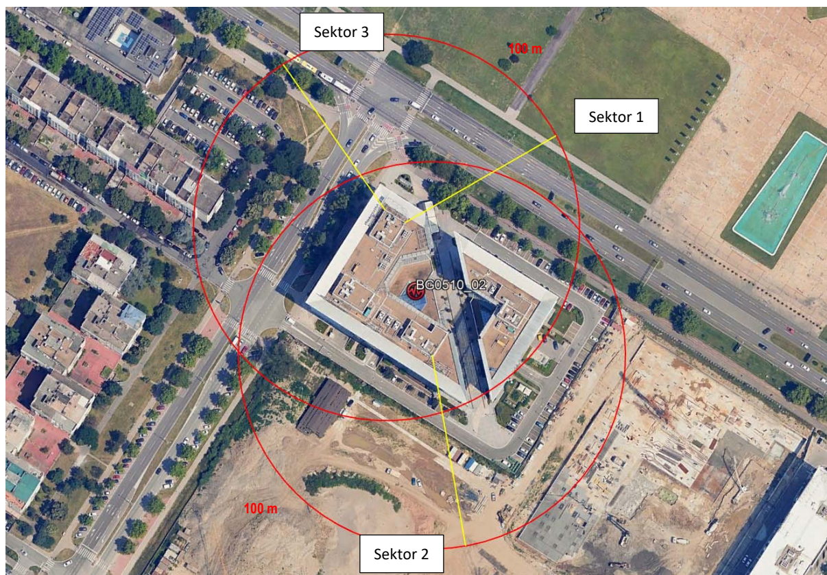
Slika 2.6 Pravci zračenja antenskih sistema predmetne bazne stanice
