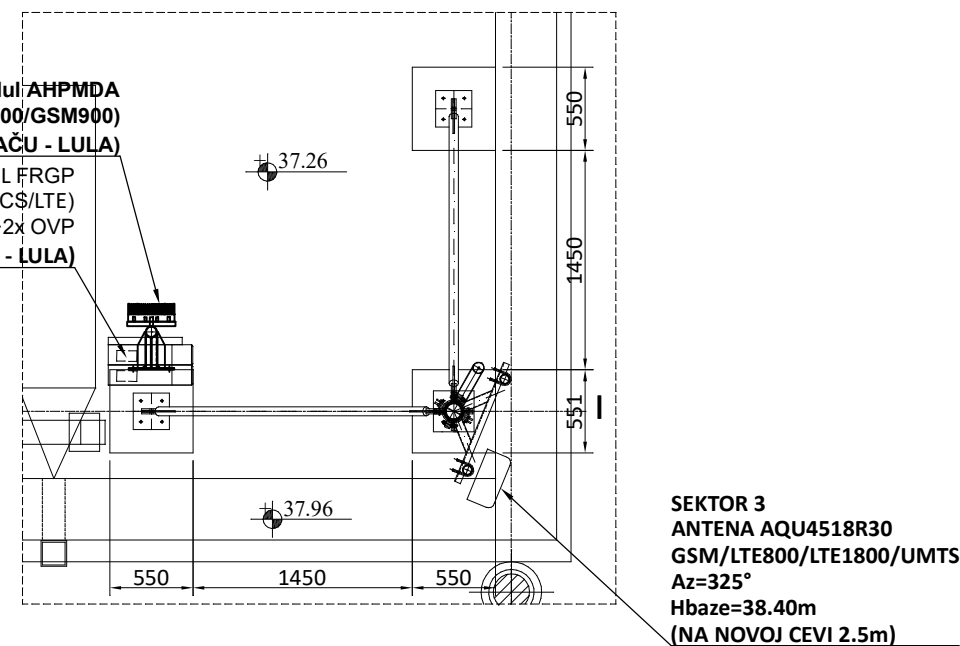
DISPOZICIJA OPREME NA LOKACIJI DETALJ "D" SA CRTEŽA 1
