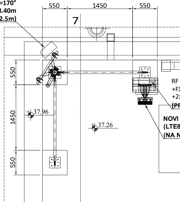
ANTENSKI SEKTOR 2 DETALJ "B" SA CRTEŽA 1
