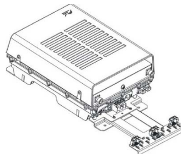
Slika 3.4 Izgled jednostrukih Nokia Flexi radio modula
