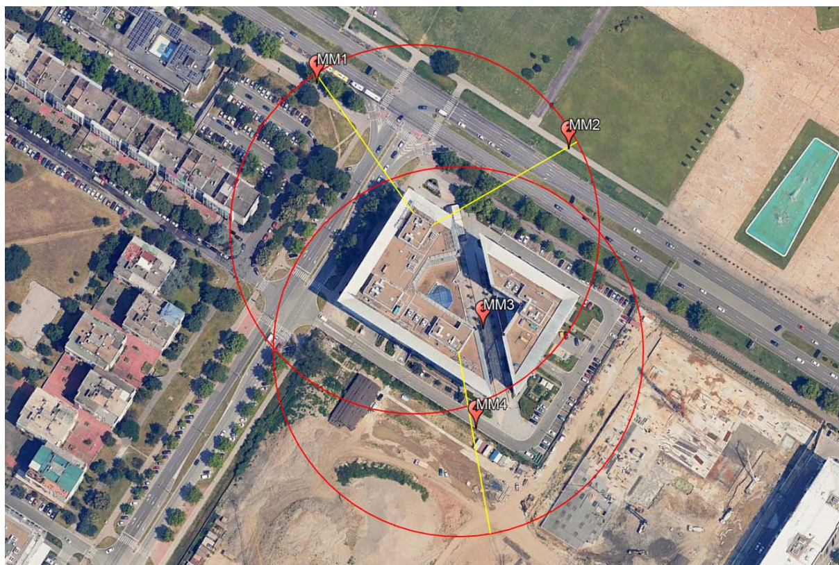
Slika 4.1 Prikaz pozicije mernih mesta u kojima su izvršena merenja nivoa EMP (crveni krugovi poluprečnika 100 m)
