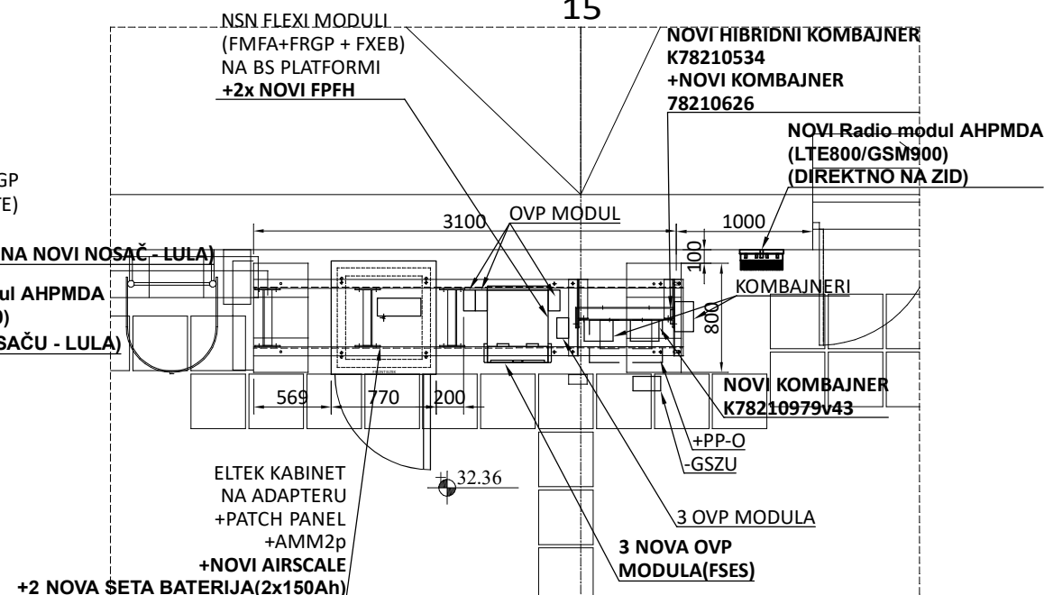
DISPOZICIJA OPREME NA LOKACIJI DETALJ "D" SA CRTEŽA 1
