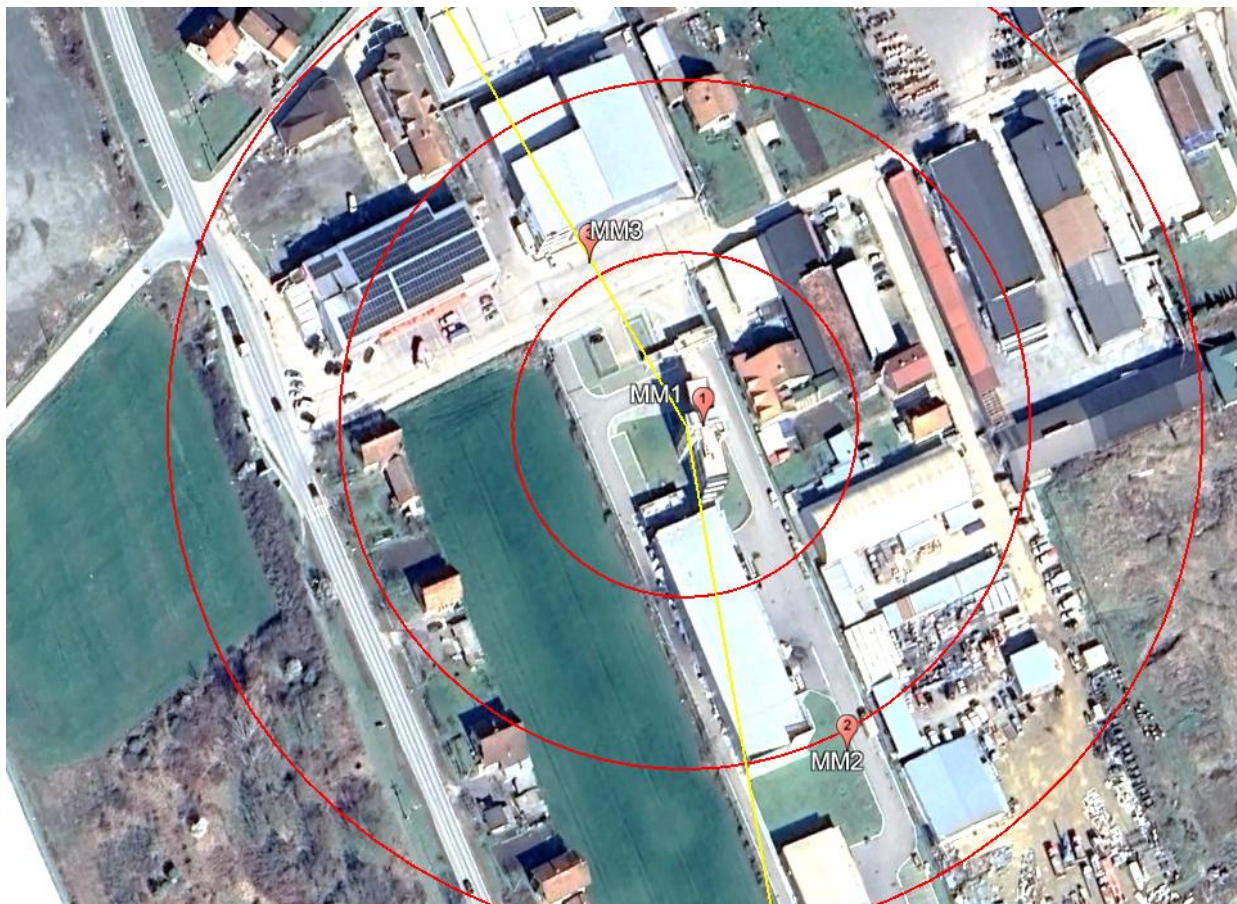
Slika 7: Prikaz Mernih Mesta u lokalnoj zoni Cetin BS Dobanovci Squadra
