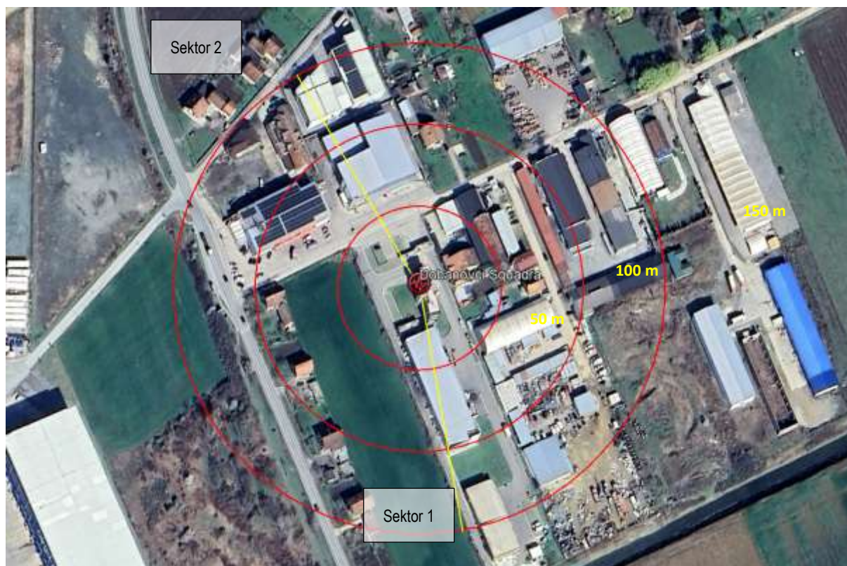
Slika 2.6 Pravci zračenja antenskog sistema BS Dobanovci Squadra
