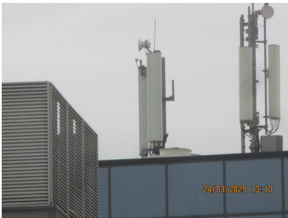
Slika 4 : Prikaz antene sektora 1 Cetin BS
