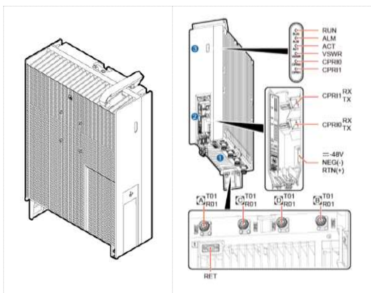
Slika 3.6 RRU5502 jedinica
