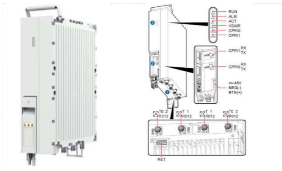
Slika 3.7 RRU5509t jedinica
