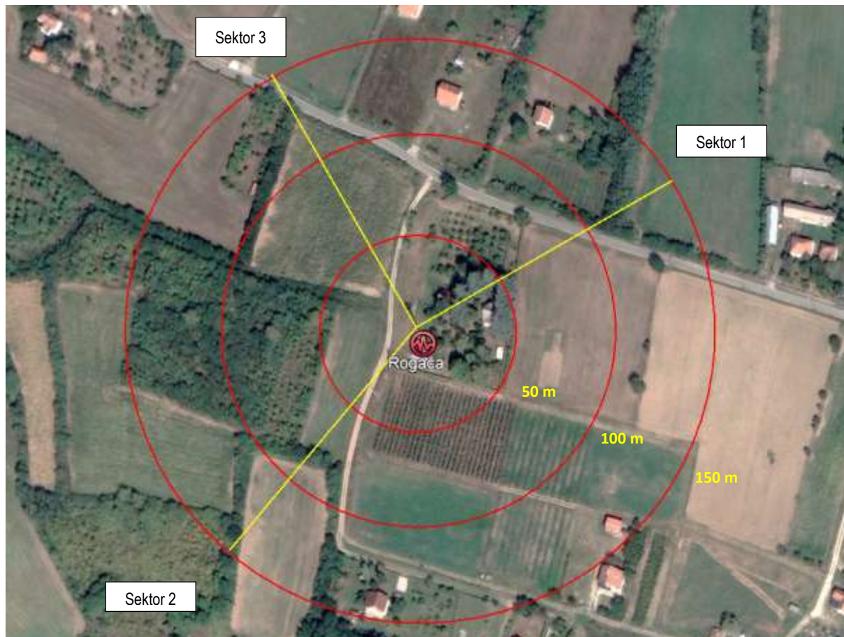
Slika 2.5 Pravci zračenja budućeg antenskog sistema BS ROGAČA
