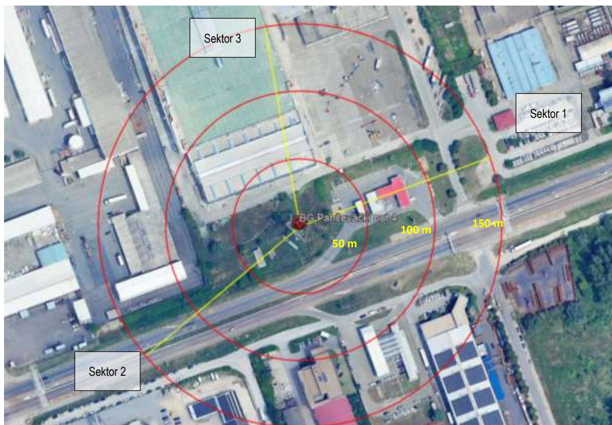
Slika 2.6 Pravci zračenja antenskog sistema BS BG PANČEVAČKI PUT 4
