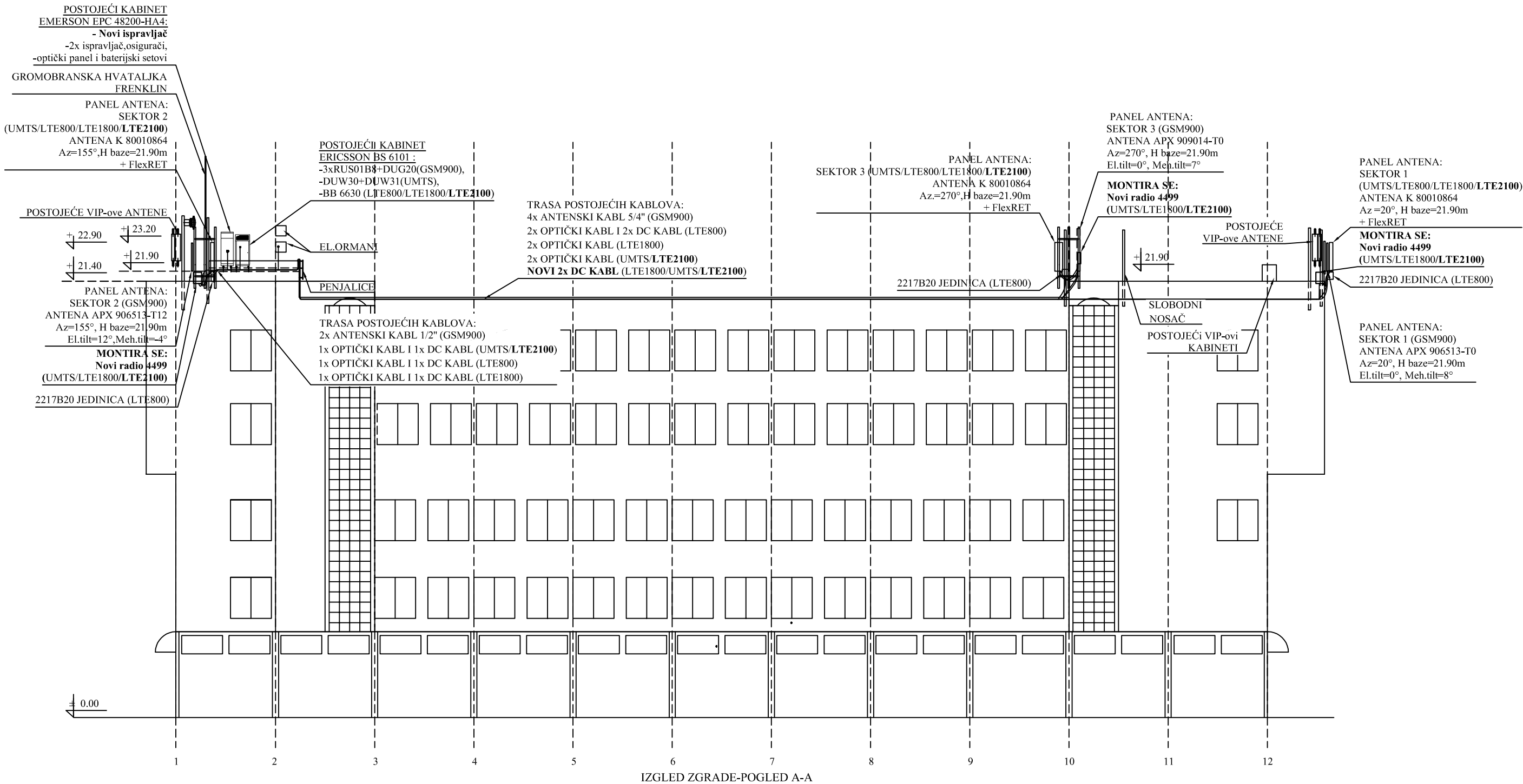
IZGLED ZGRADE-POGLED A-A
