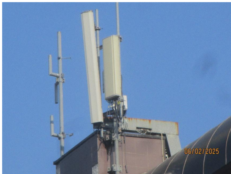
Slika 6 : Prikaz antena i radio modula sektora 3
