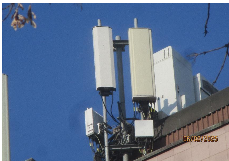
Slika 5 : Prikaz antena i radio modula sektora 2
