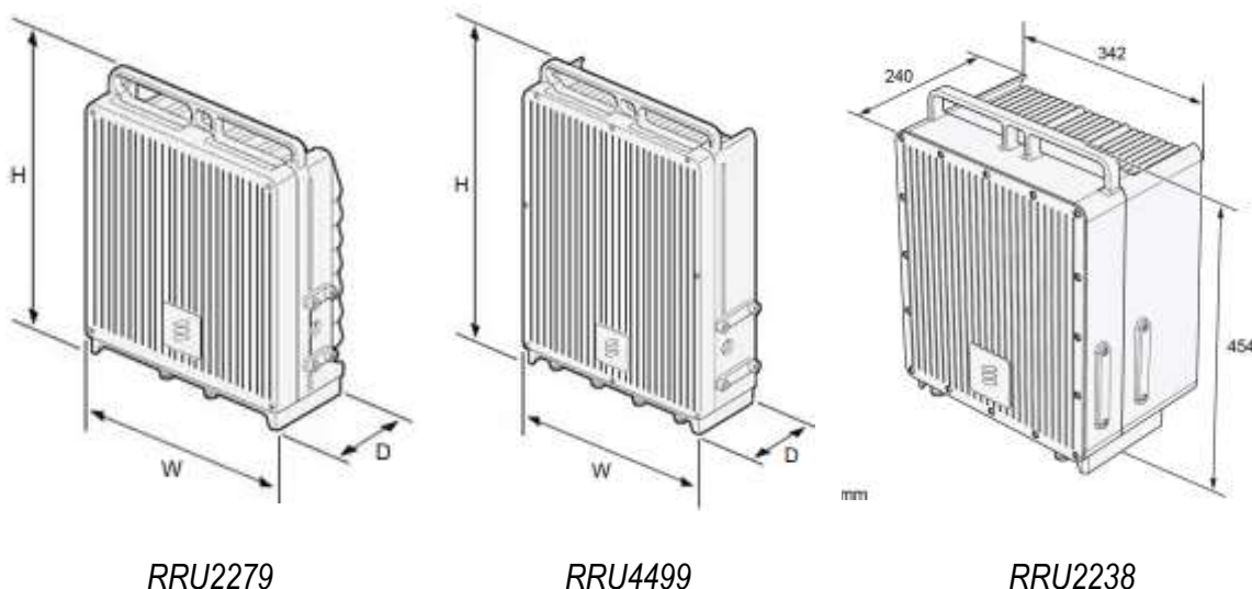
Slika 3.7 Izgled Radio modula
