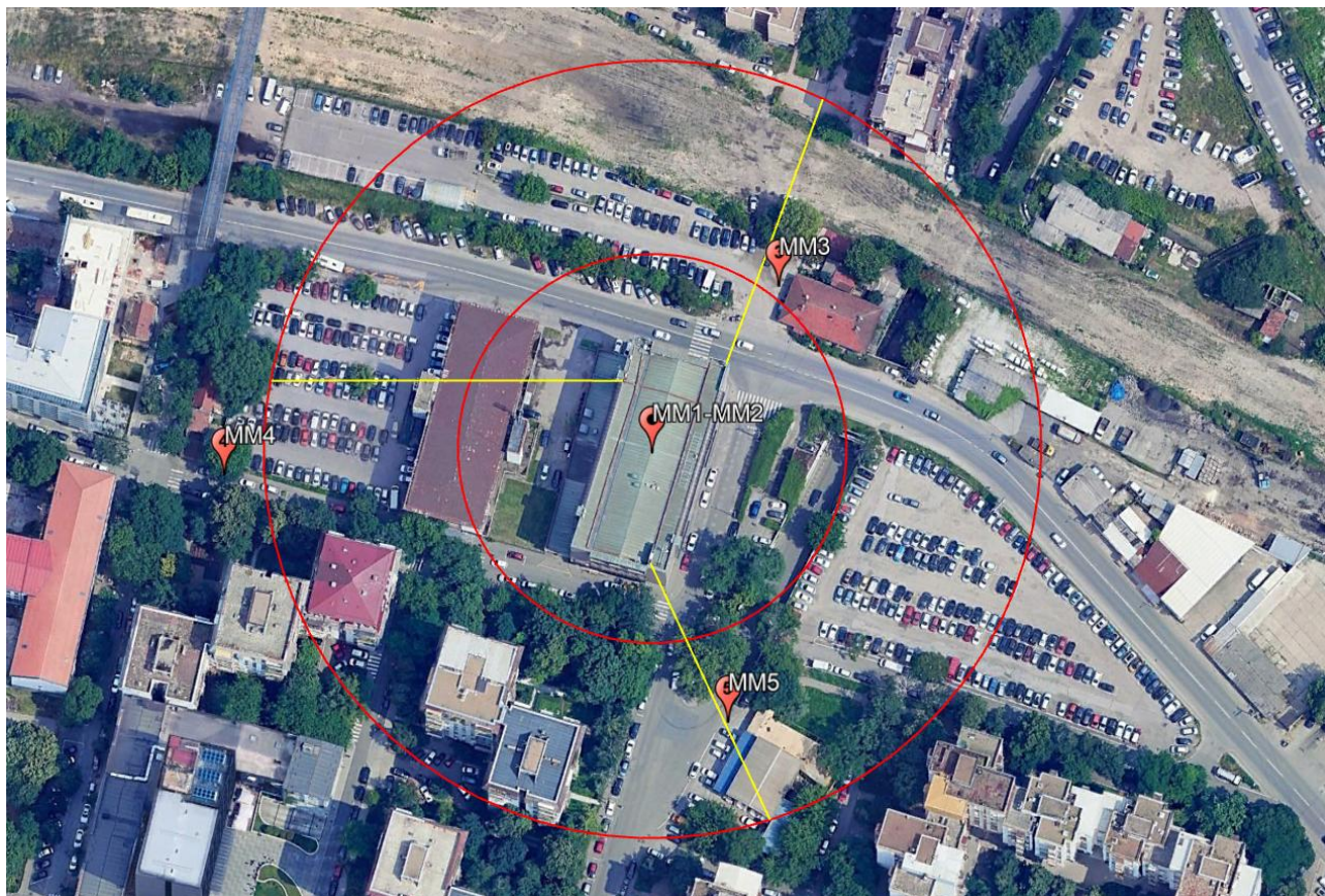
Slika 8: Prikaz mernih mesta u lokalnoj zoni BS Telekom Srbija BG-Dubrovačka
