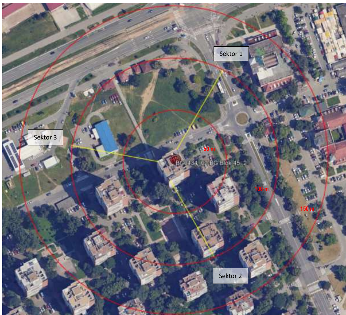
Slika 2.5 Pravci zračenja antenskih sistema predmetne bazne stanice
