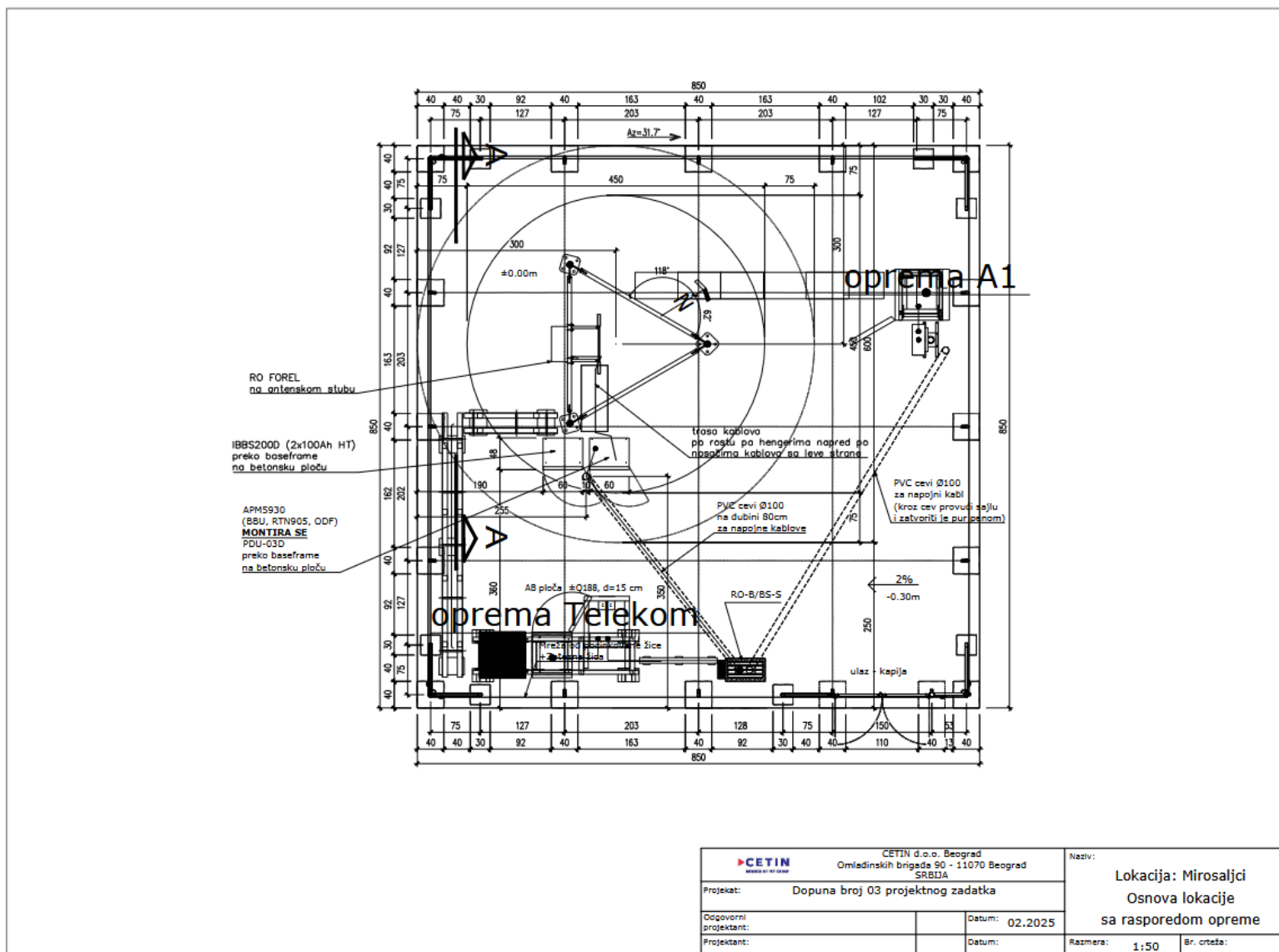
Слика 8.1. Идејно решење – Основа локације са распоредом опреме – ново стање
