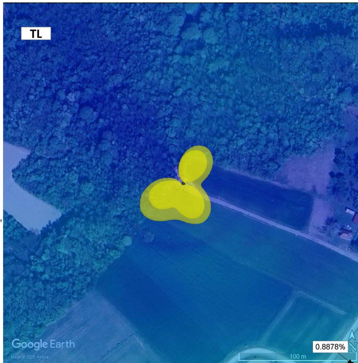
Слика 4.9. Фактор изложености на тлу када сви радио-системи свих оператора раде максималним капацитетом
