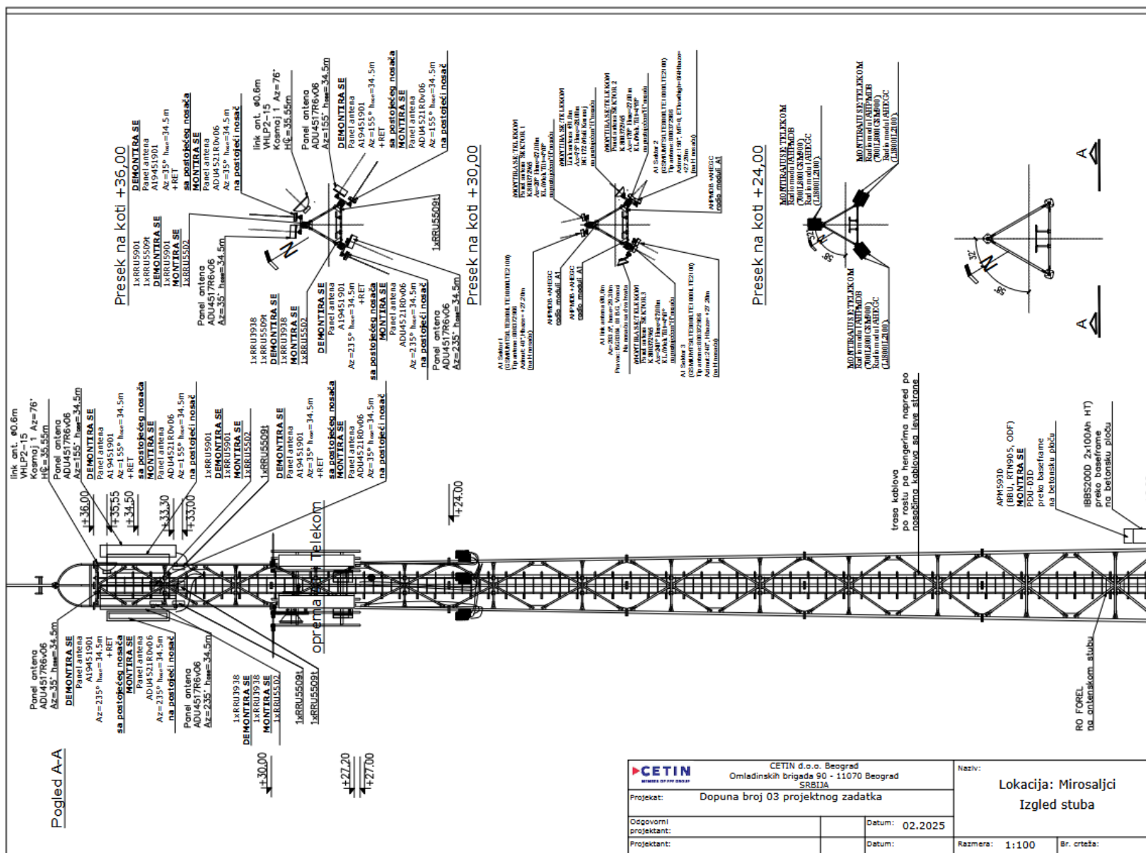
Слика 8.2. Идејно решење – Изглед стуба
