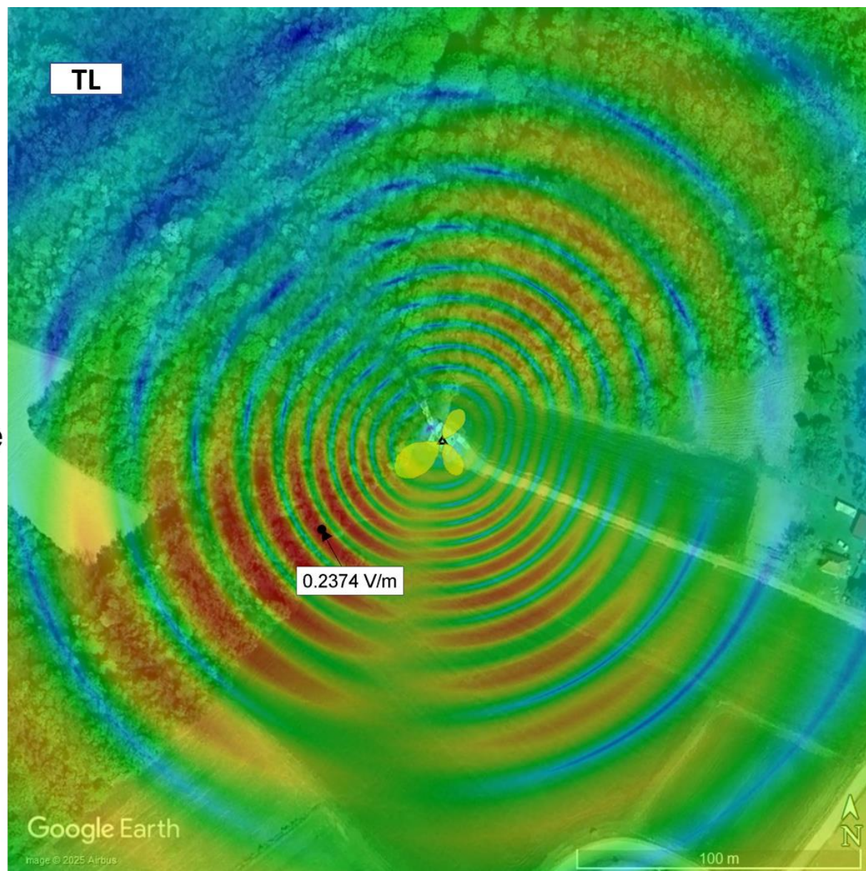
Слика 4.7. Јачина електричног поља на тлу када радио-систем LTE2100 оператора Cetin ради максималним капацитетом
