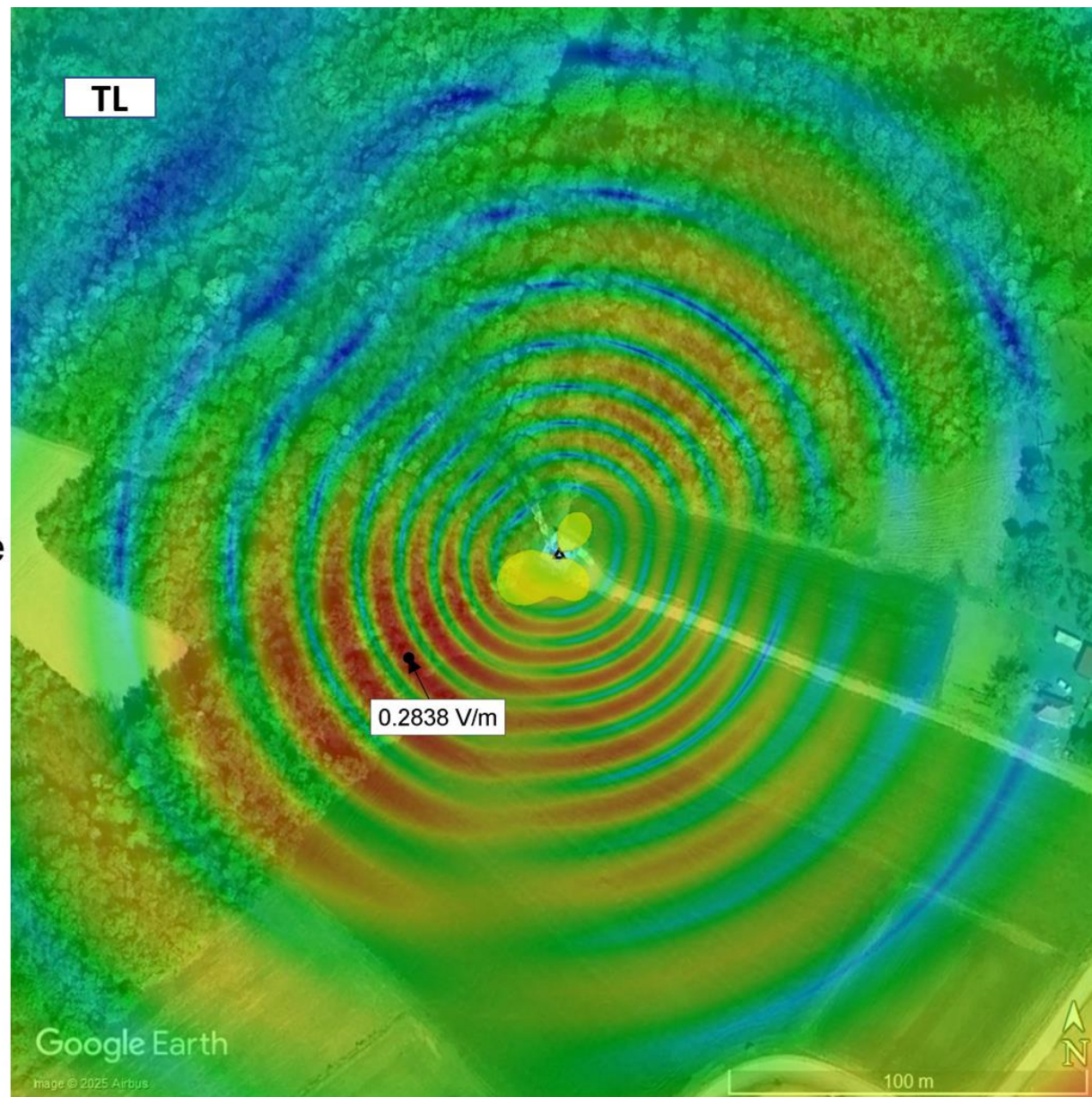
Слика 4.6. Јачина електричног поља на тлу када радио-систем LTE1800 оператора Cetin ради максималним капацитетом
