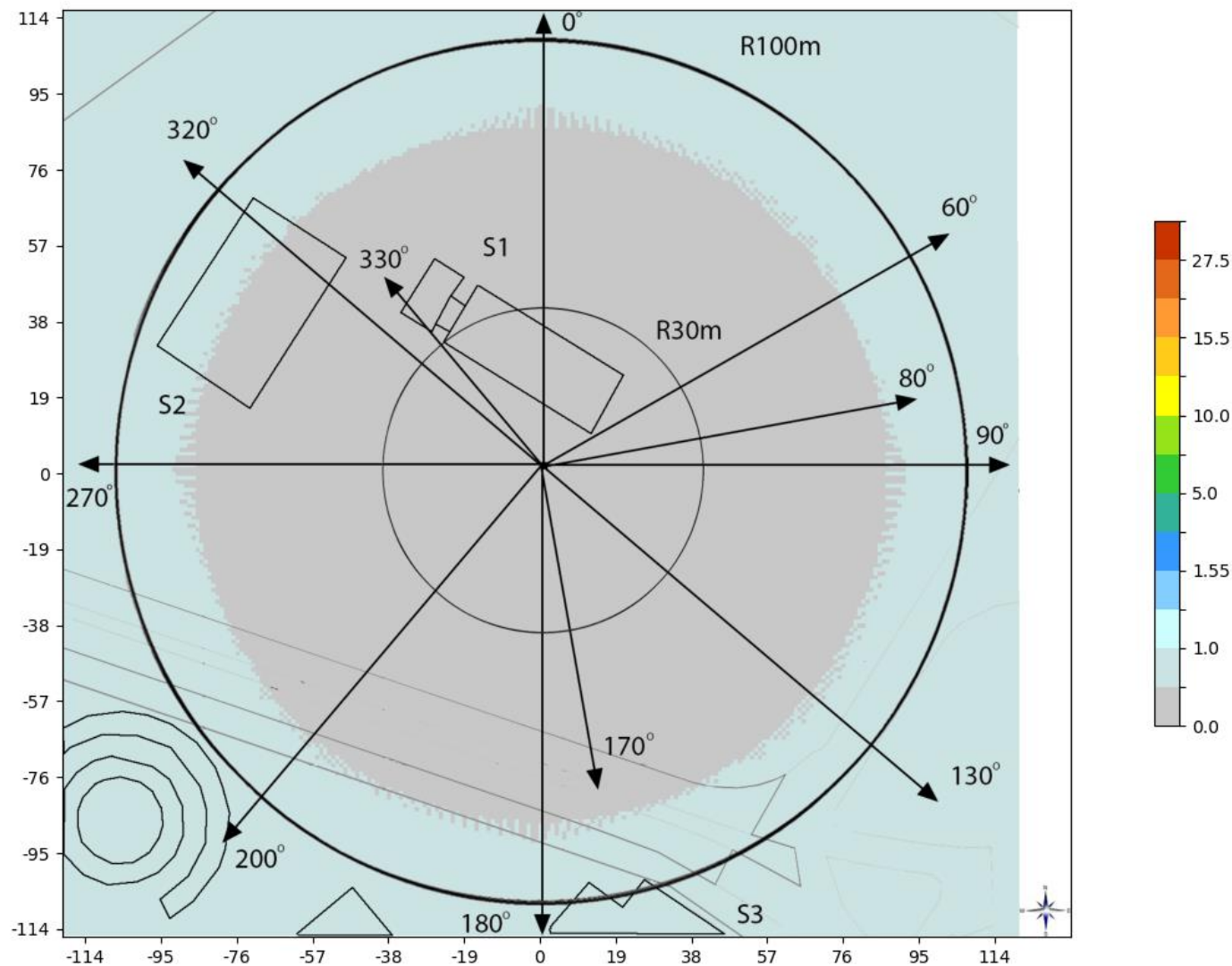
Slika 6.9. Rezultati proračuna jačine električnog polja na tlu, za slučaj kada LTE800 bazna stanica operatora A1 radi sa maks. kapacitetom.
