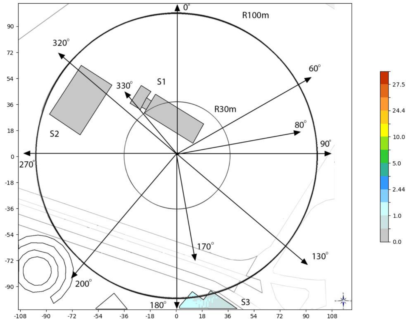
Slika 6.4. Rezultati proračuna jačine električnog polja na tlu, unutar objekata, kada LTE2100 bazna stanica operatora A1 radi sa maks. kapacitetom.
