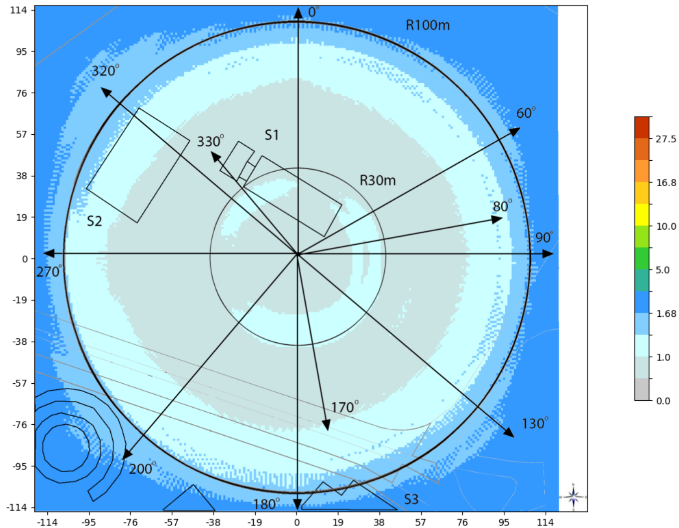
Slika 6.15. Rezultati proračuna jačine električnog polja na tlu, za slučaj kada sve stanice svih operatora rade sa maks. kapacitetom.
