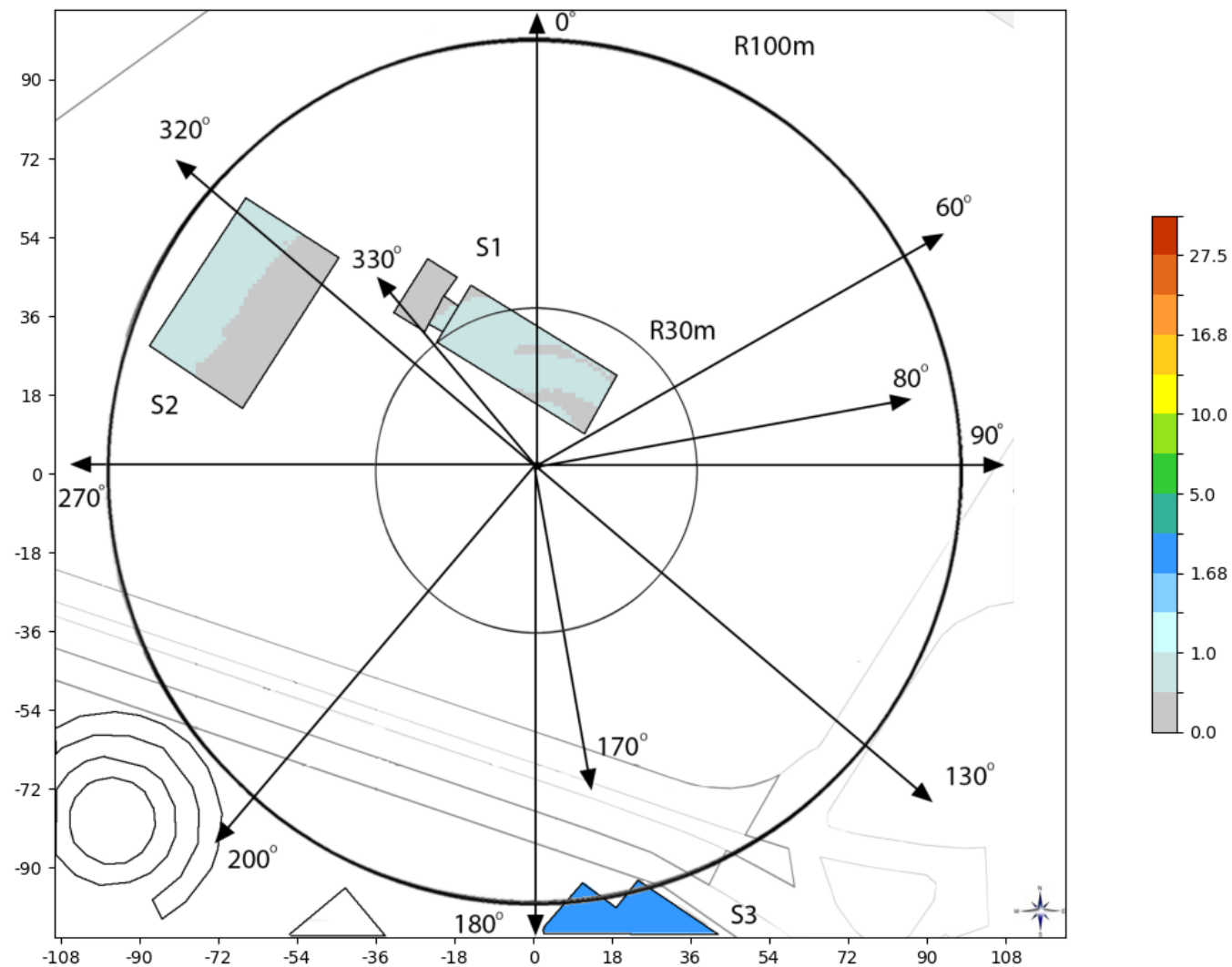
Slika 6.5. Rezultati proračuna jačine električnog polja unutar objekata, kada svi sistemi operatora A1 na lokaciji rade sa maksimalnim kapacitetom.
