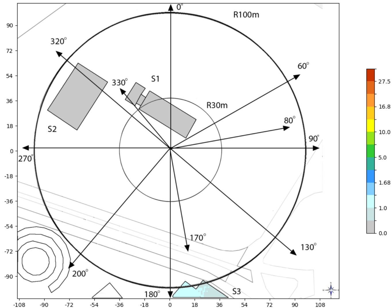
Slika 6.3. Rezultati proračuna jačine električnog polja na tlu, unutar objekata, kada GSM900 bazna stanica operatora A1 radi sa maks. kapacitetom.
