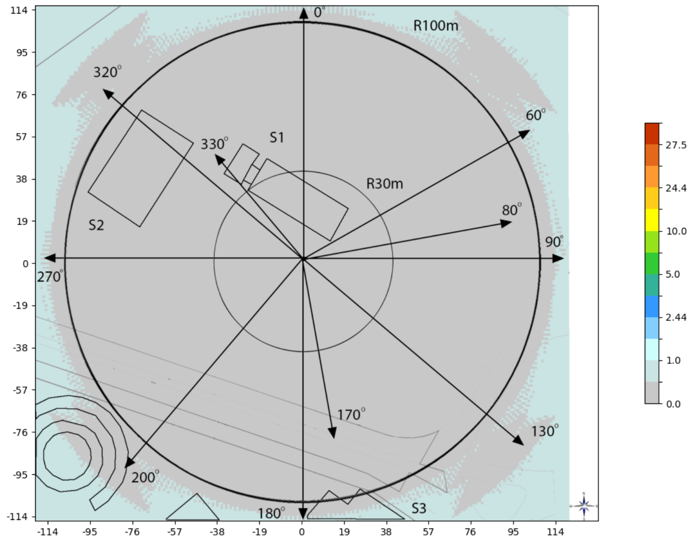
Slika 6.7. Rezultati proračuna jačine električnog polja na tlu, za slučaj kada LTE2100 bazna stanica operatora A1 radi sa maks. kapacitetom.
