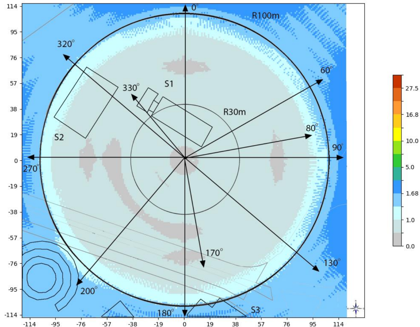
Slika 6.13. Rezultati proračuna jačine električnog polja na tlu, za slučaj kada sve stanice operatora A1 rade sa maks. kapacitetom.
