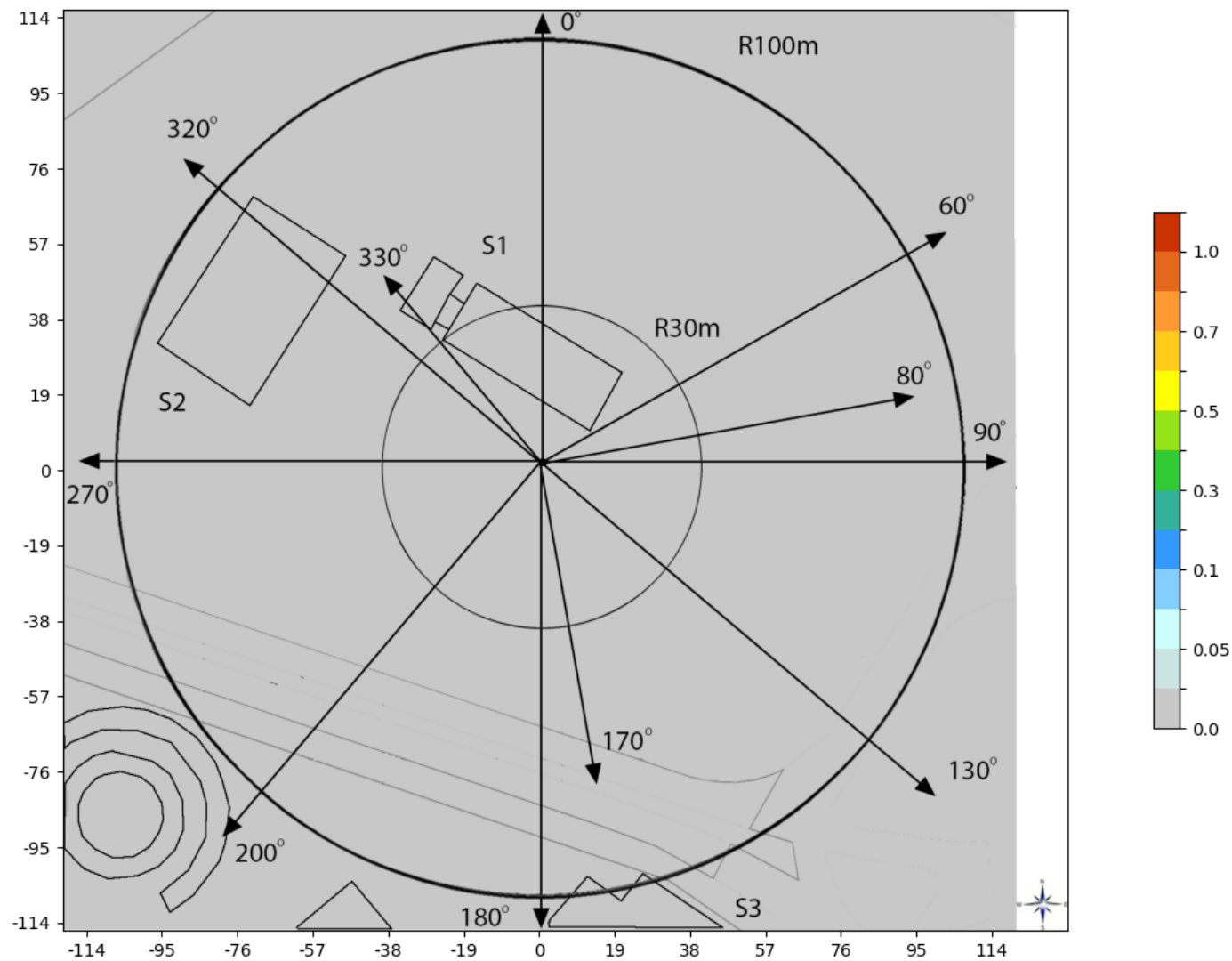
Slika 6.8. Rezultati proračuna faktora izlaganja na tlu, za slučaj kada svi sistemi svih operatora na lokaciji rade sa maksimalnim kapacitetom
