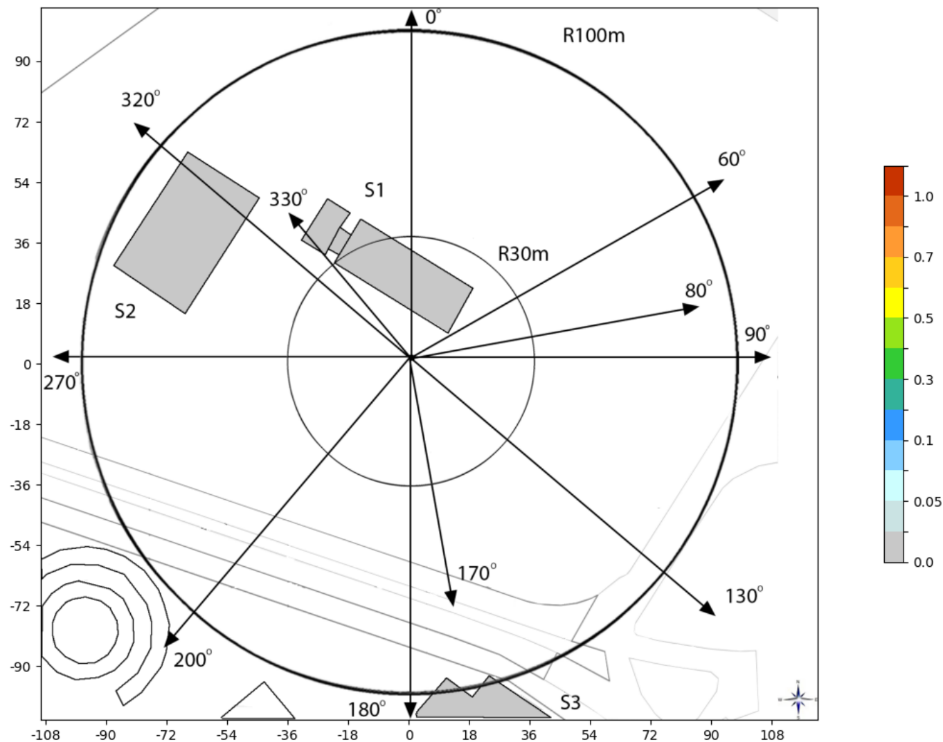
Slika 6.6. Rezultati proračuna faktora izlaganja unutar objekata, kada svi sistemi operatora A1 na lokaciji rade sa maksimalnim kapacitetom.
