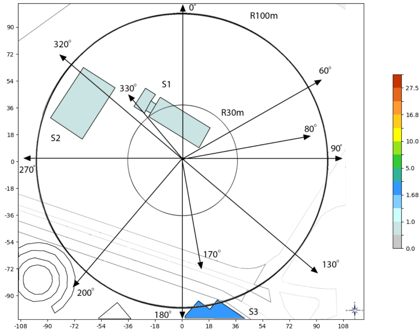
Slika 6.7. Rezultati proračuna jačine električnog polja unutar objekata, kada svi sistemi svih operatora na lokaciji rade sa maksimalnim kapacitetom.
