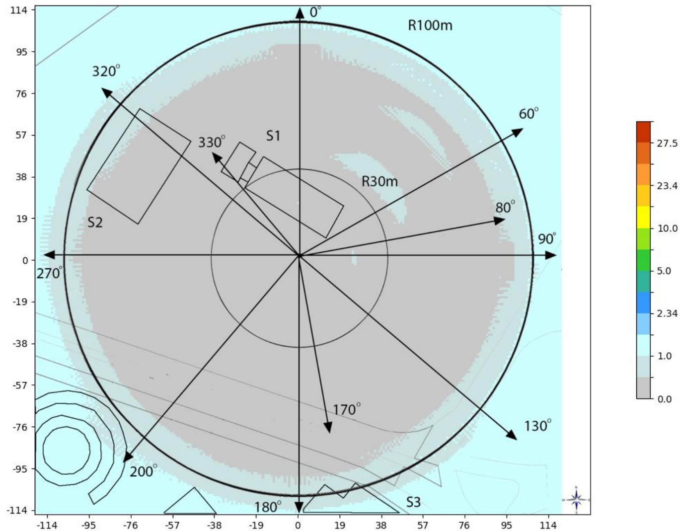
Slika 6.10. Rezultati proračuna jačine električnog polja na tlu, za slučaj kada LTE1800 bazna stanica operatora A1 radi sa maks. kapacitetom.
