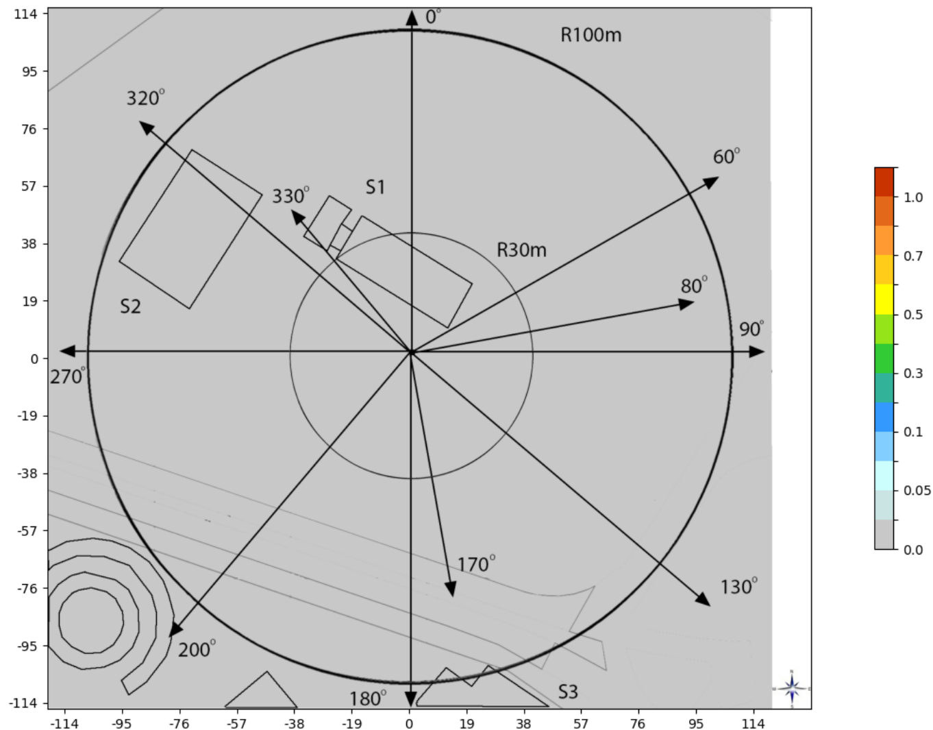
Slika 6.14. Rezultati proračuna faktora izlaganja na tlu, za slučaj kada svi sistemi operatora A1 na lokaciji rade sa maksimalnim kapacitetom
