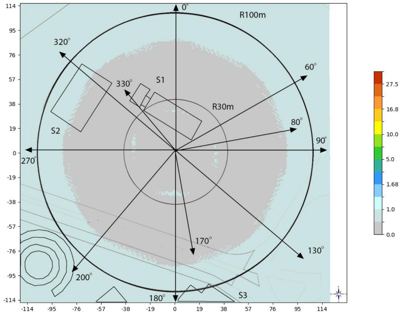
Slika 6.11. Rezultati proračuna jačine električnog polja na tlu, za slučaj kada GSM900 bazna stanica operatora A1 radi sa maks. kapacitetom.
