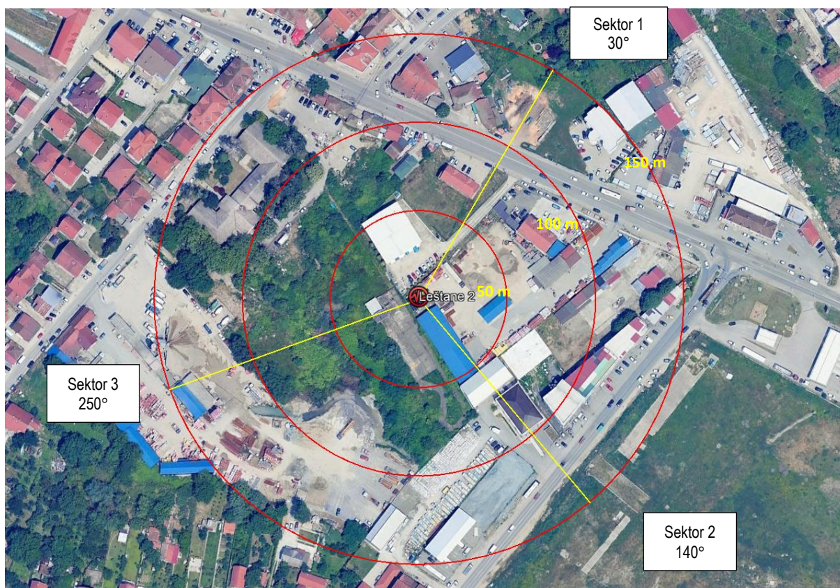
Slika 2.7 Pravci zračenja antenskog sistema buduće BS LEŠTANE 2
