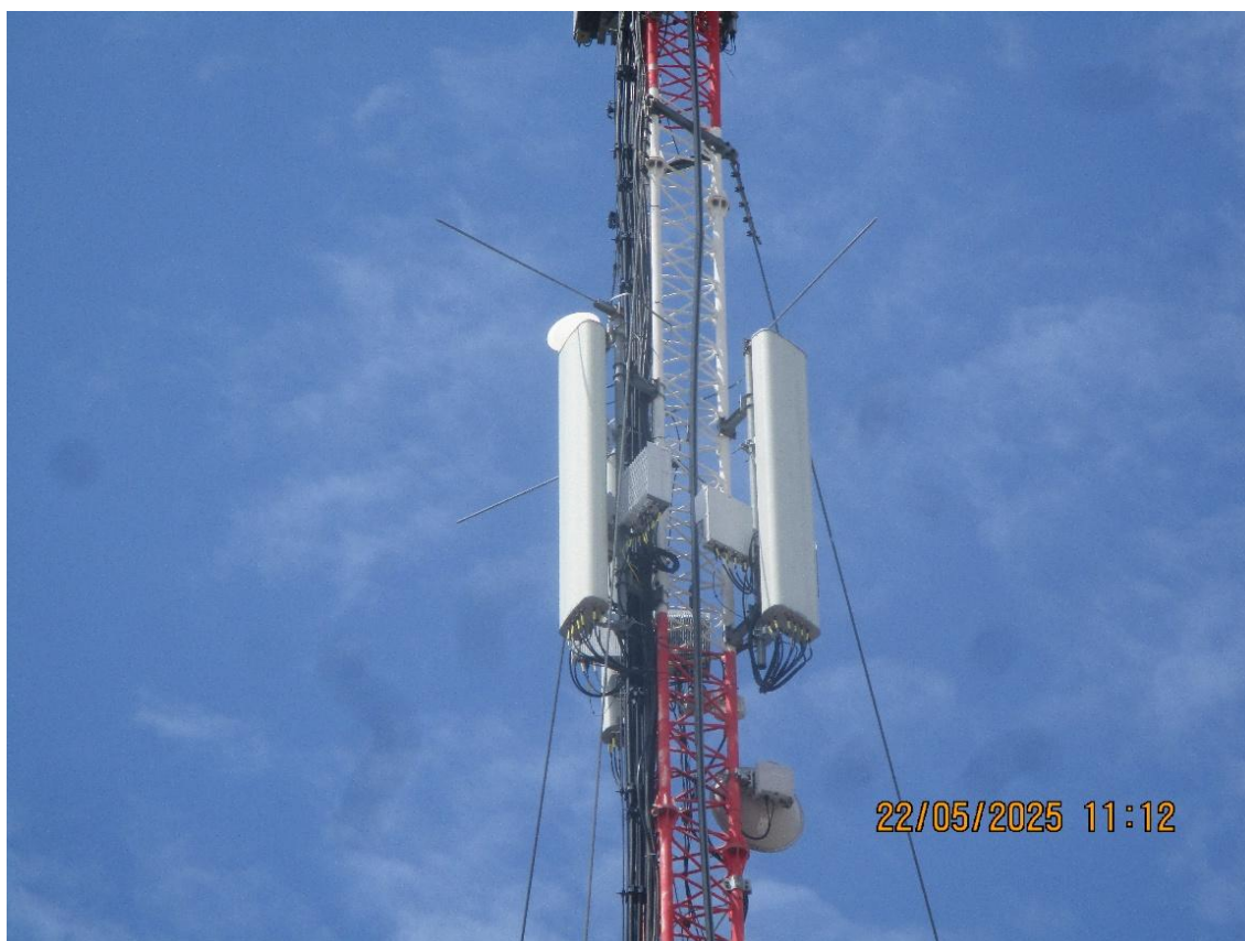
Slika 2.6 Kabinet i antenski sistem BS
