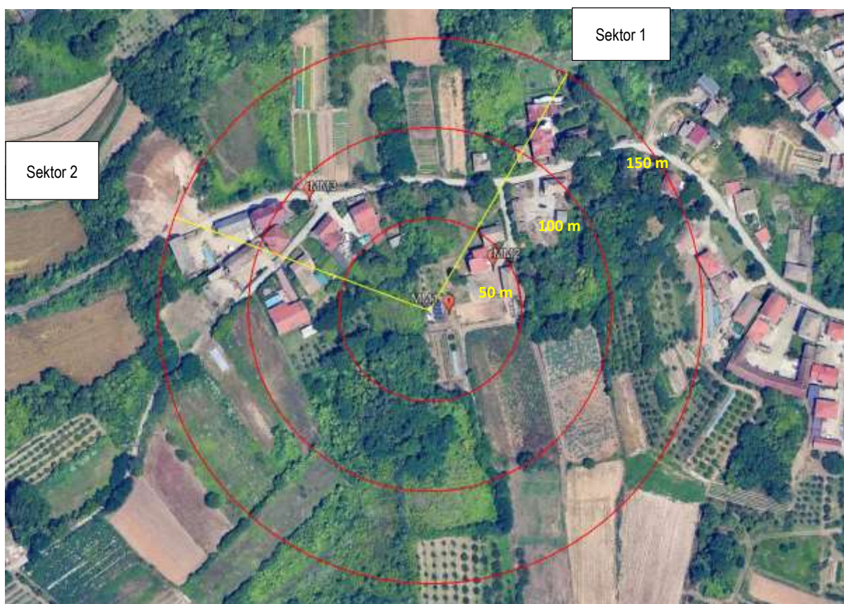
Slika 2.6 Pravci zračenja antenskog sistema buduće BS SLANCI 2
