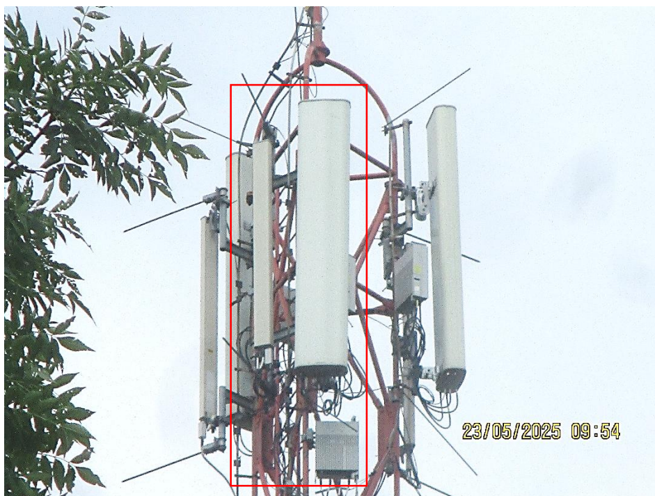
Slika 4 : Prikaz antenskog sistema sektora 1
