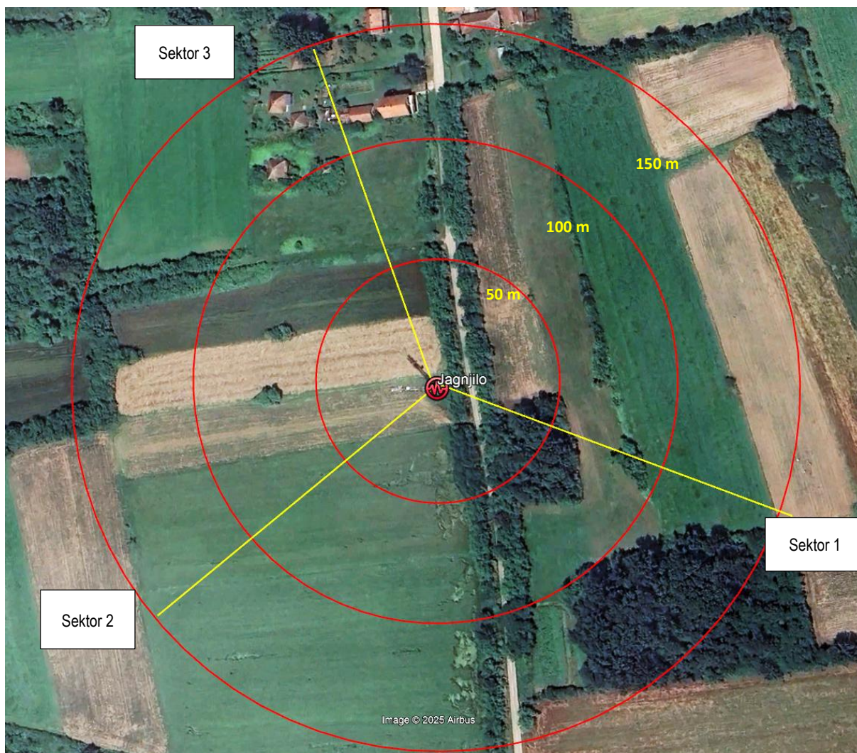
Slika 2.5 Pravci zračenja antenskog sistema BS JAGNJILO
