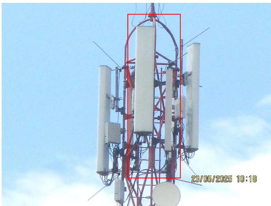
Slika 6 : Prikaz antenskog sistema sektora 3
