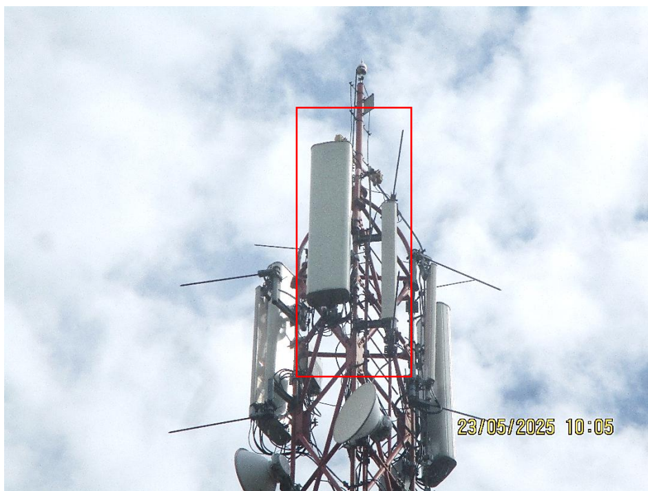
Slika 5 : Prikaz antenskog sistema sektora 2
