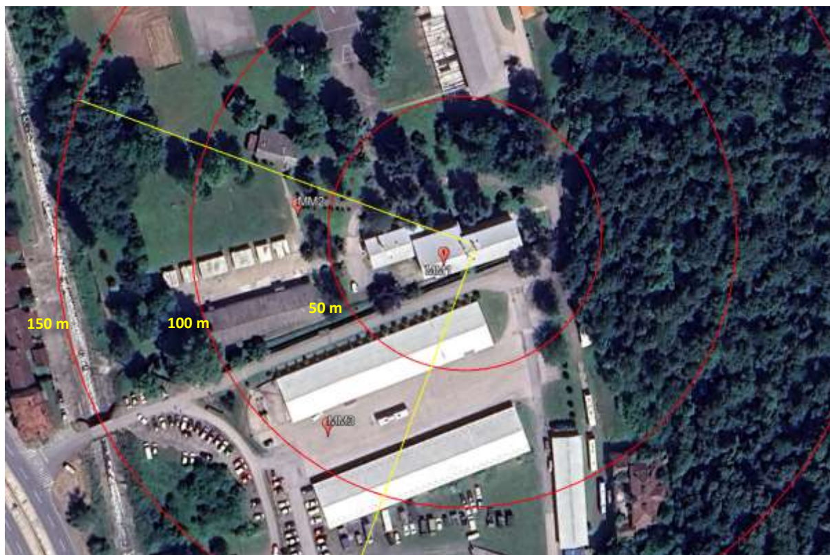
Slika 4.1 Prikaz pozicije mernih mesta u kojima su izvršena merenja nivoa EMP (crveno – krugovi poluprečnika 50, 100 i 150 m)
