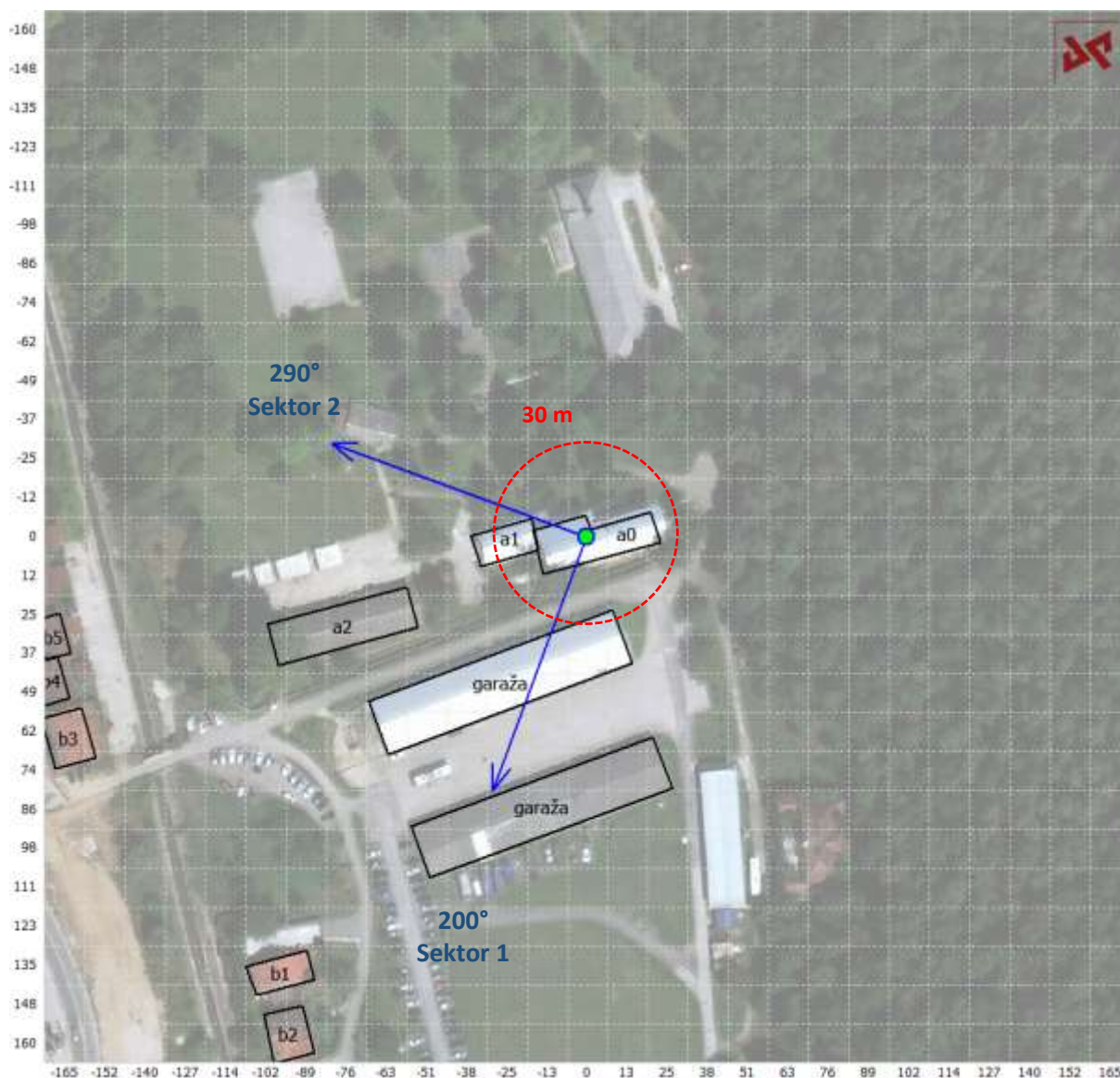
Slika 2.7 Prikaz pravaca zračenja antena bazne stanice i pozicije okolnih objekata
