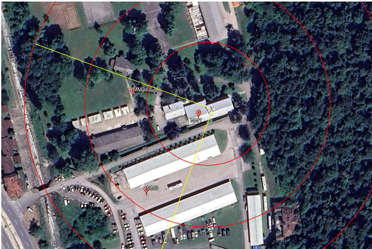
Slika 5: Prikaz Mernih Mesta u lokalnoj zoni Cetin BS BG Rakovički put
