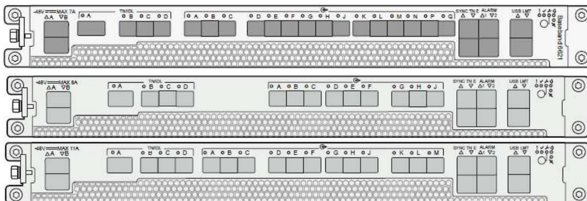
Slika 3.3 Izgled Baseband 6621 / 6631 jedinice
