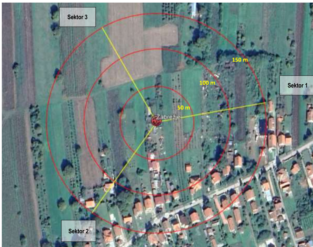
Slika 2.6 Pravci zračenja antenskog sistema buduće BS ZABREŽJE
