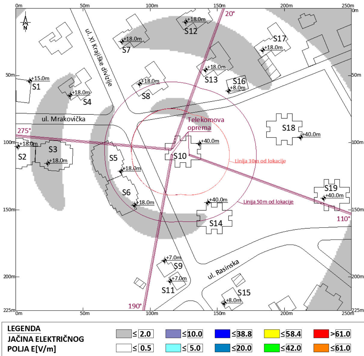
Slika 4.13 Rezultati proračuna jačine električnog polja u široj okolini lokacije bazne stanice na javnom području, na visini +1.70m (prosečna visina čoveka) u odnosu na nivo tla za slučaj rada sistema LTE800 (sistem koji se rekonstruiše) operatora Telekom Srbija .
