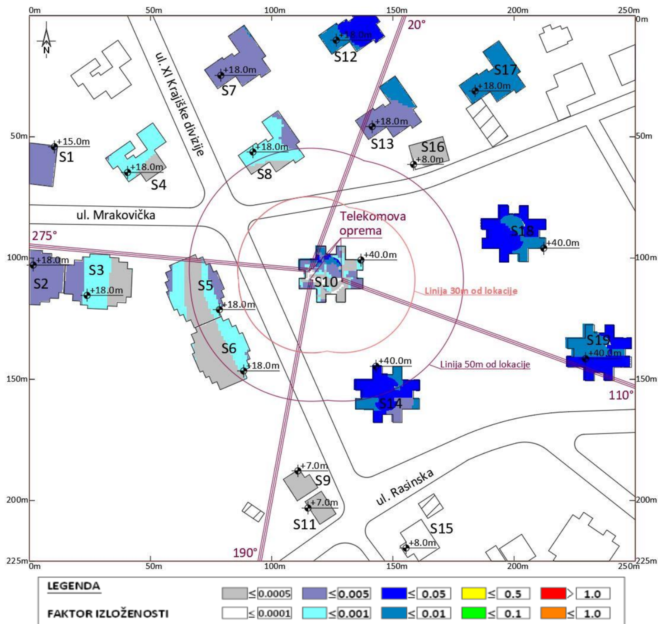
Slika 4.8 Rezultati proračuna faktora izloženosti za slučaj rada svih sistema na lokaciji- GSM900, GSM1800, UMTS2100, LTE1800, LTE800 i LTE2100 operatora Telekom Srbija , u zonama povećane osetljivosti
