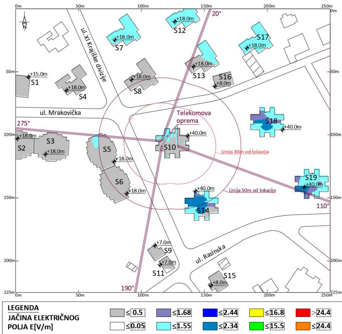
Slika 4.4 Rezultati proračuna jačine električnog polja sistema LTE1800 operatora Telekom Srbija , u zonama povećane osetljivosti (sistem koji se rekonstruiše)
