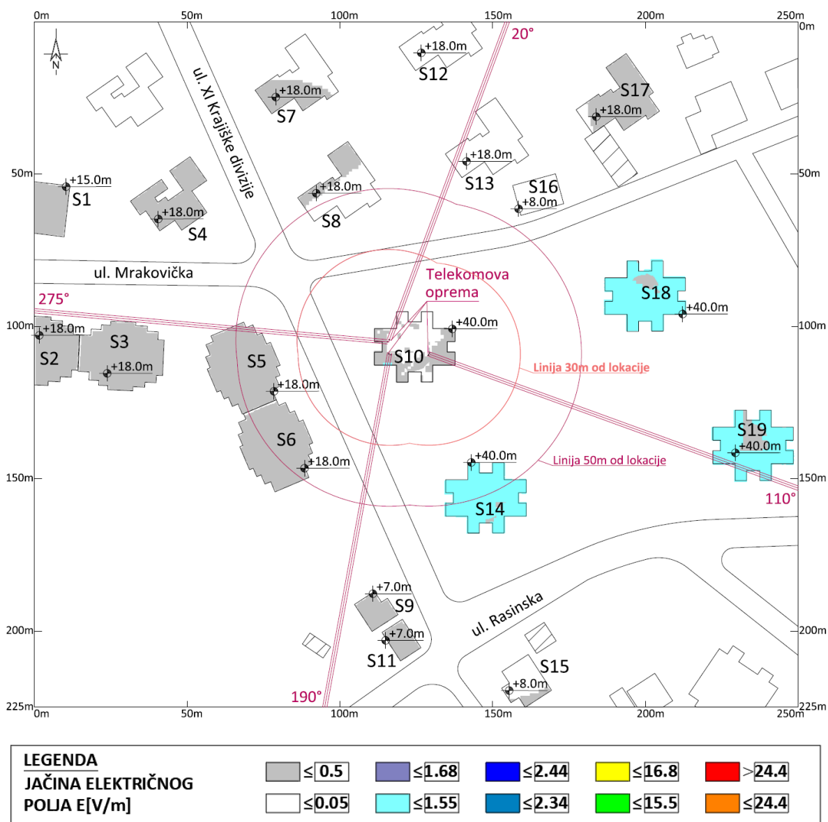
Slika 4.1 Rezultati proračuna jačine električnog polja sistema GSM900 operatora Telekom Srbija , u zonama povećane osetljivosti
