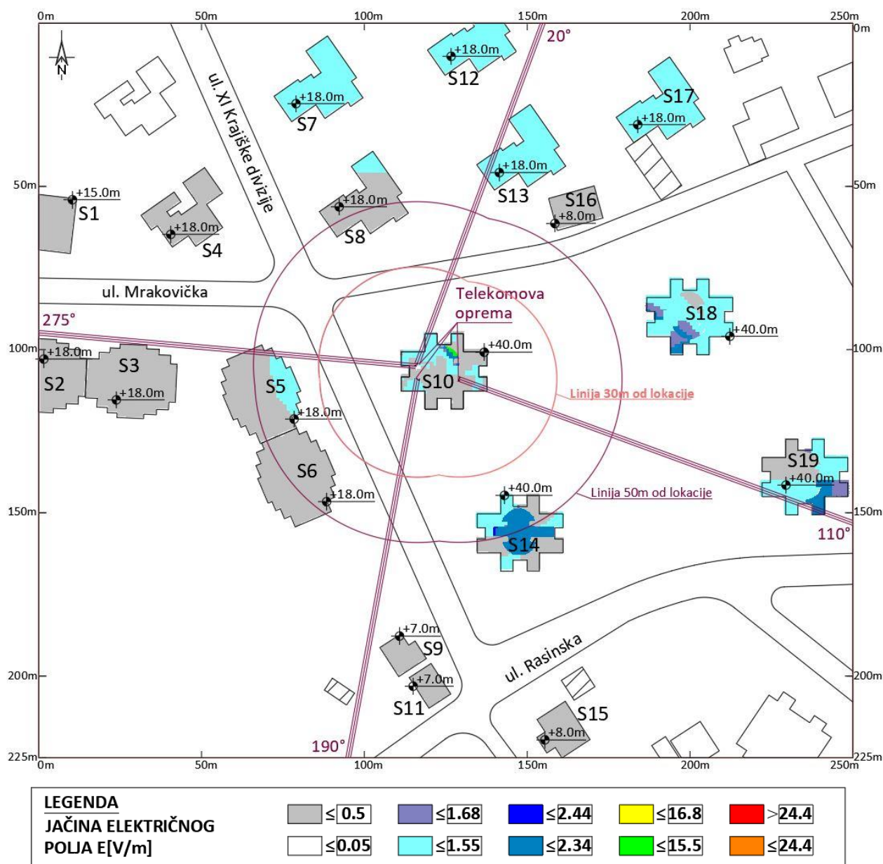
Slika 4.6 Rezultati proračuna jačine električnog polja sistema LTE2100 operatora Telekom Srbija , u zonama povećane osetljivosti (sistem koji se rekonstruiše)
