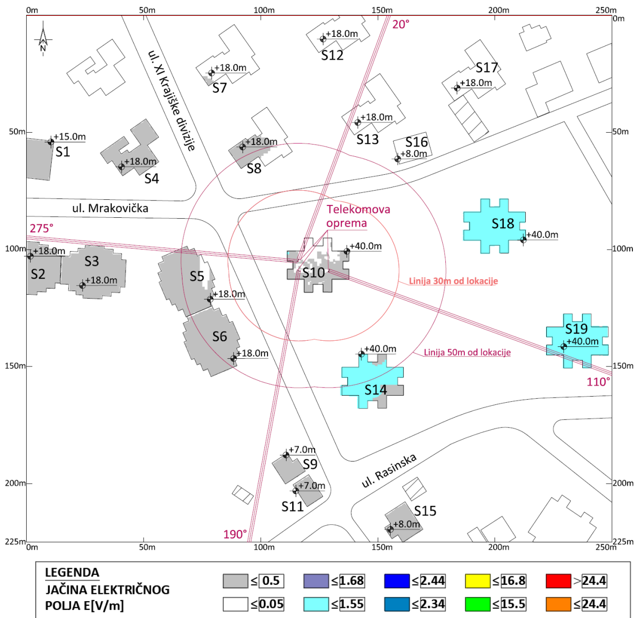
Slika 4.2 Rezultati proračuna jačine električnog polja sistema GSM1800 operatora Telekom Srbija , u zonama povećane osetljivosti
