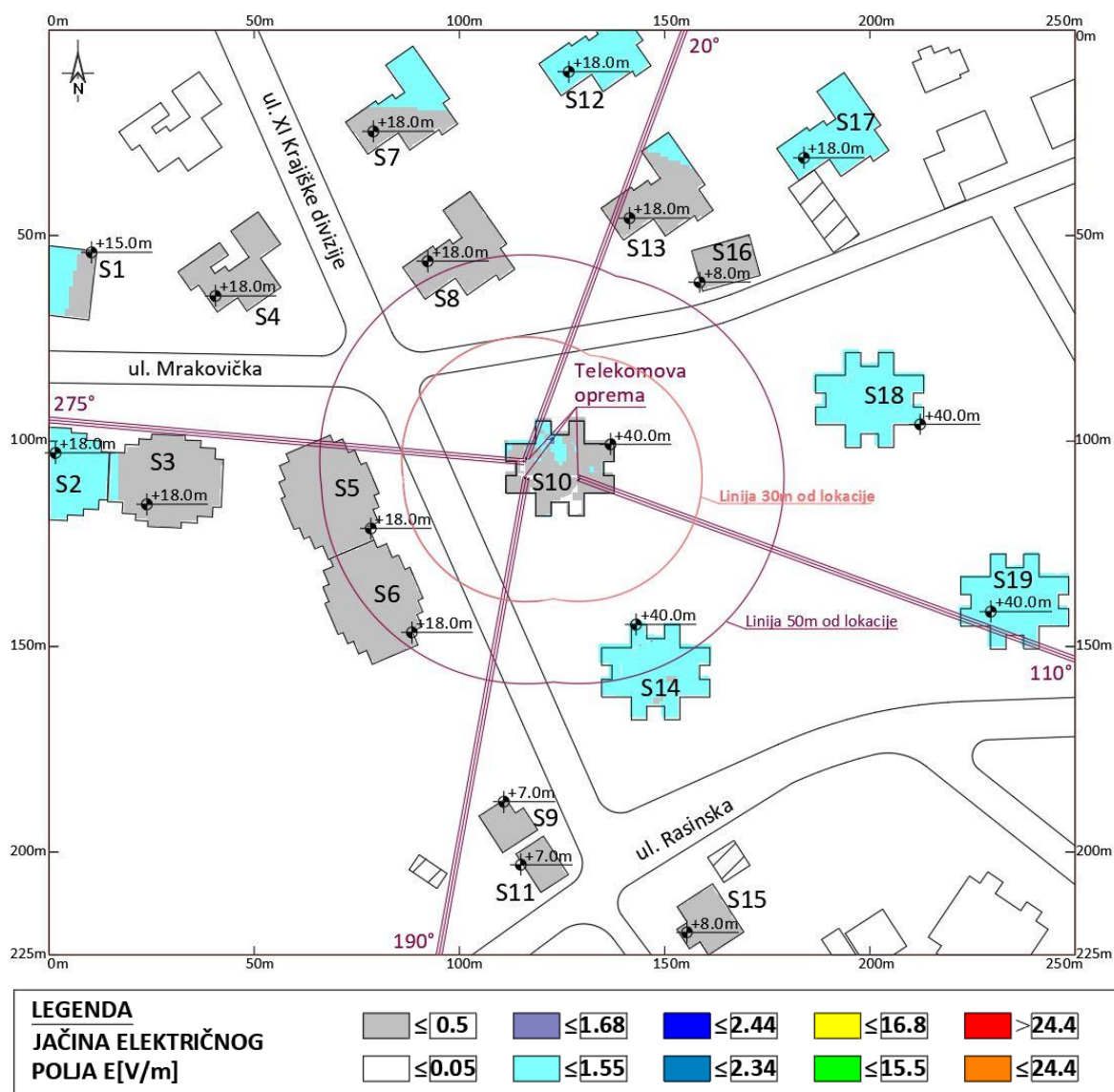
Slika 4.5 Rezultati proračuna jačine električnog polja sistema LTE800 operatora Telekom Srbija , u zonama povećane osetljivosti ( sistem koji se rekonstruiše )
