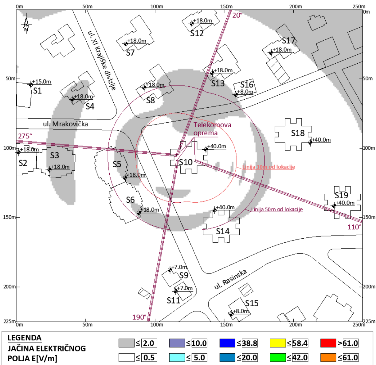
Slika 4.12 Rezultati proračuna jačine električnog polja u široj okolini lokacije bazne stanice na javnom području , na visini +1.70m (prosečna visina čoveka) u odnosu na nivo tla za slučaj rada sistema LTE1800 (sistem koji se rekonstruiše) operatora Telekom Srbija .
