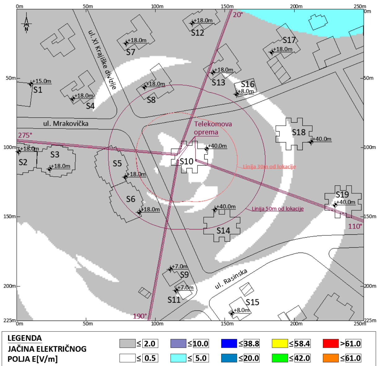
Slika 4.15 Rezultati proračuna jačine električnog polja u široj okolini lokacije bazne stanice na javnom području, na visini +1.70m (prosečna visina čoveka) u odnosu na nivo tla za slučaj rada sistema GSM900, GSM1800, UMTS2100, LTE1800, LTE800 i LTE2100 operatora Telekom Srbija . Maksimalna proračunata vrednost jačine električnog polja iznosi E=2.53 V/m .
