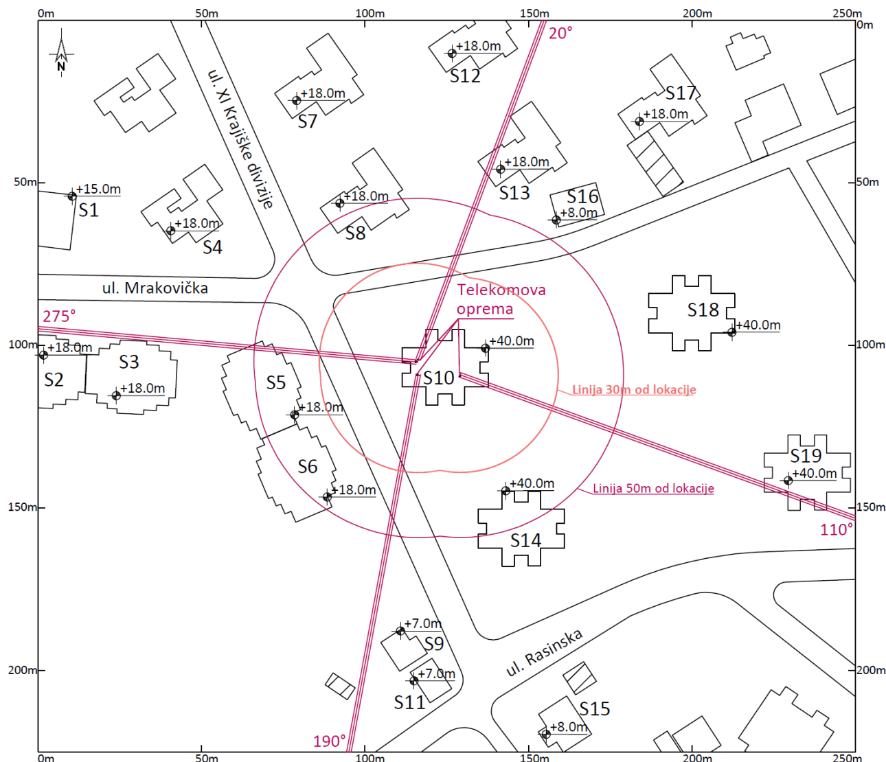
Slika 2.5 Dijagram objekata u okruženju radio bazne stanice „BG - Petlovo brdo“- BG83/BGH83/BGU83/BGL83/BGO83/BGI83
