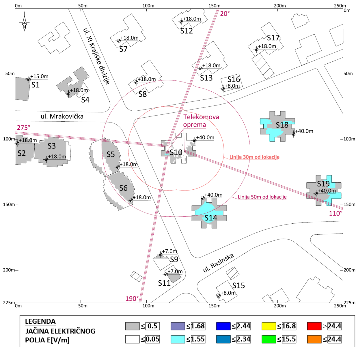
Slika 4.3 Rezultati proračuna jačine električnog polja sistema UMTS2100 operatora Telekom Srbija , u zonama povećane osetljivosti
