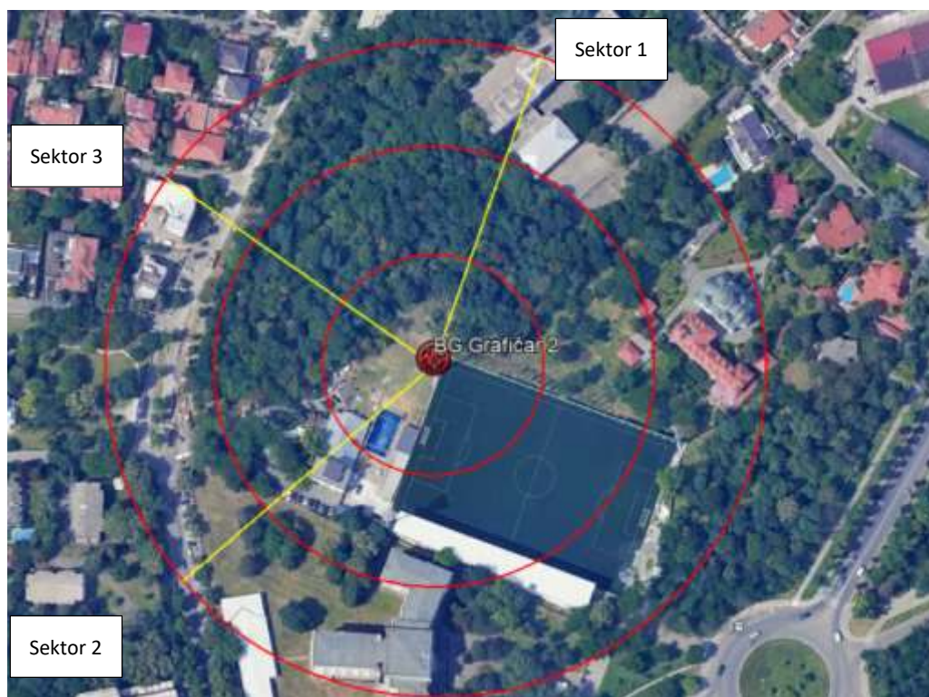
Slika 2.6 Pravci zračenja antenskih sistema predmetne bazne stanice
