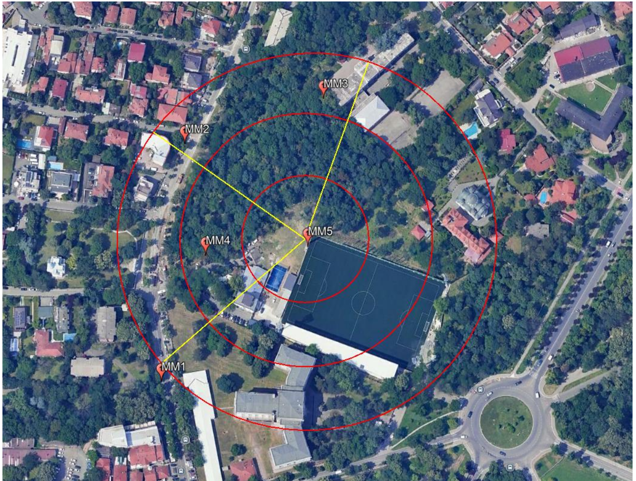
Slika 6: Prikaz mernih mesta u lokalnoj zoni BS Telekom Srbija BG-Grafičar 2
