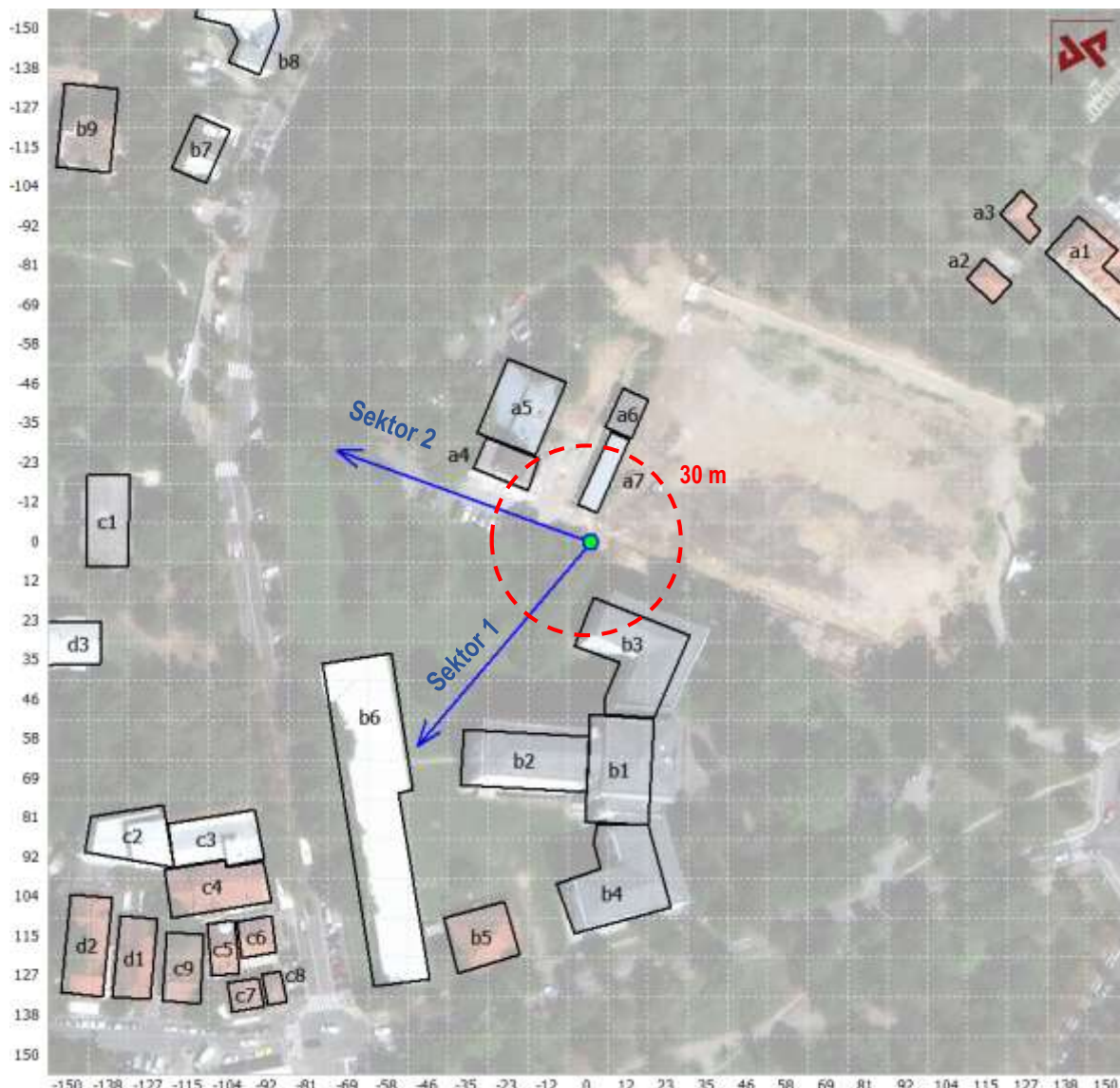
Slika 2.8 Prikaz pravaca zračenja antena i pozicije okolnih objekata
