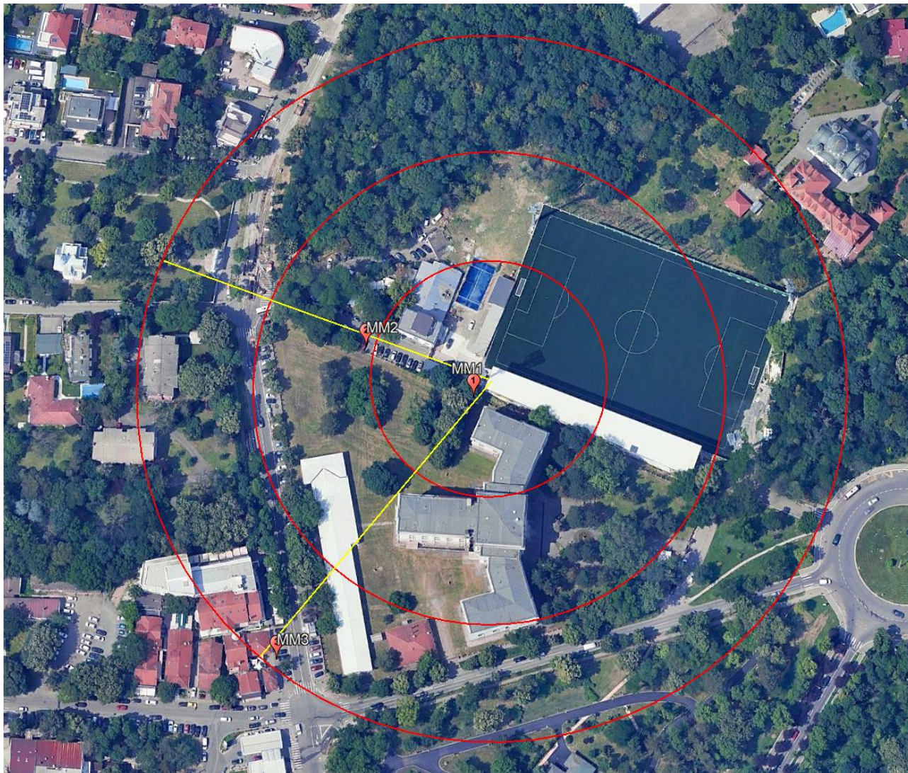
Slika 6: Prikaz mernih mesta u lokalnoj zoni BS Telekom Srbija BG-Gračar 3
