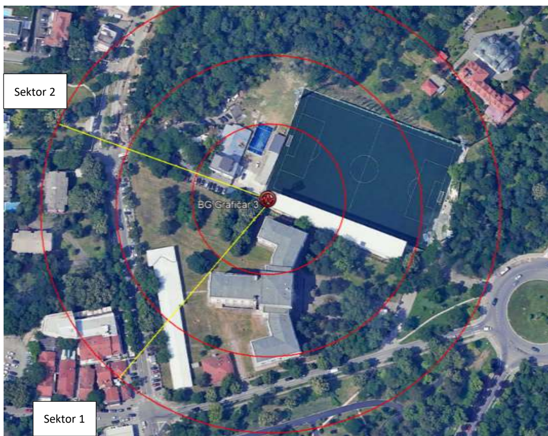
Slika 2.7 Pravci zračenja antenskih sistema predmetne bazne stanice
