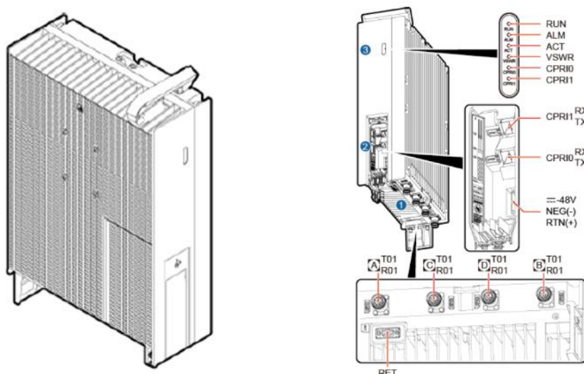
Slika 3.5 RRU5502 jedinica
