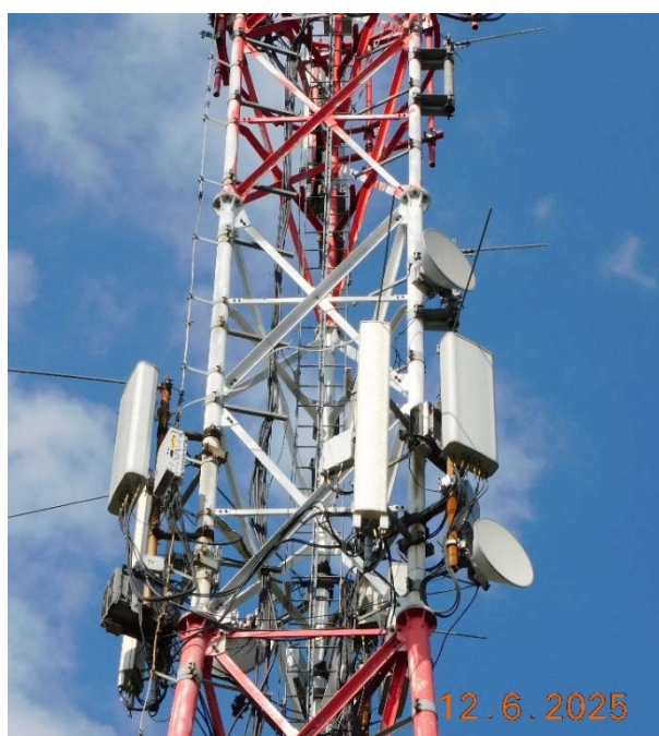
Slika 2.5 Kabinet i antenski sistem BS
