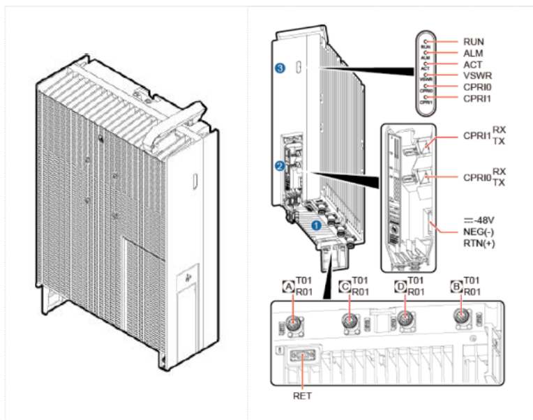
Slika 3.3 RRU5502 jedinica
