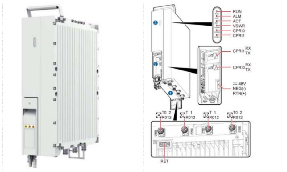
Slika 3.4 RRU5509t jedinica
