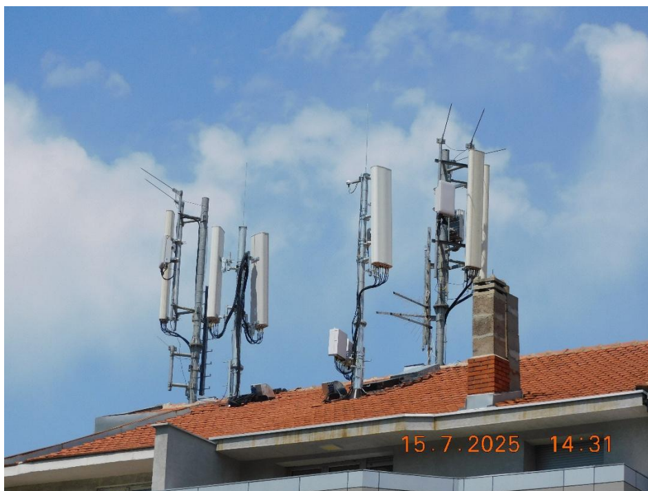
Slika 4 : Prikaz antenskog sistema
