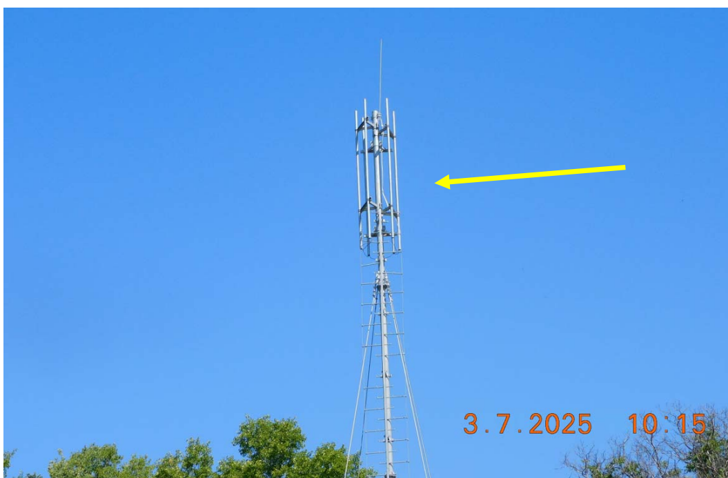
Slika 2.5 Prikaz antenskih nosača na antenskom stubu
