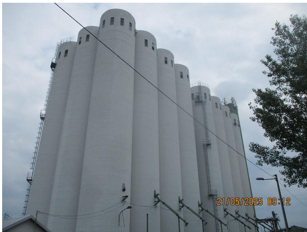
Slika 3: Prikaz silosa na kom se nalazi antenski sistem bazne stanice
