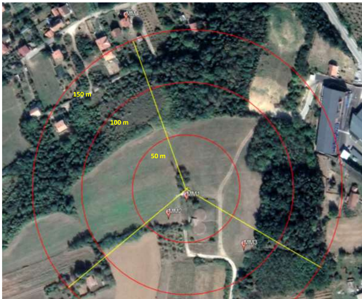
Slika 4.1 Prikaz pozicije mernih mesta u kojima su izvršena merenja nivoa EMP (crveno – krugovi poluprečnika 50, 100 i 150 m)
