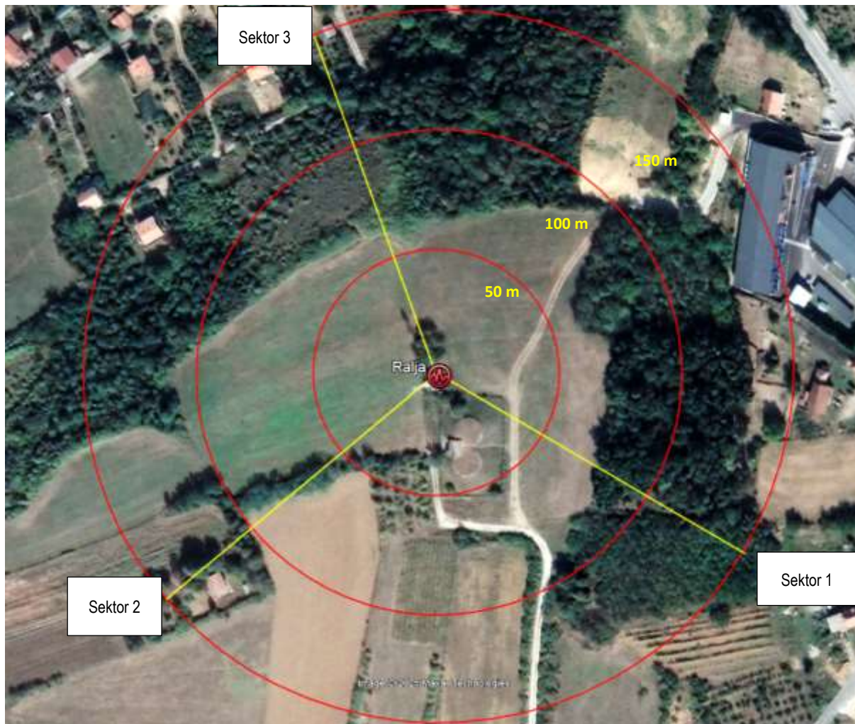
Slika 2.7 Pravci zračenja antenskog sistema buduće BS RALJA
