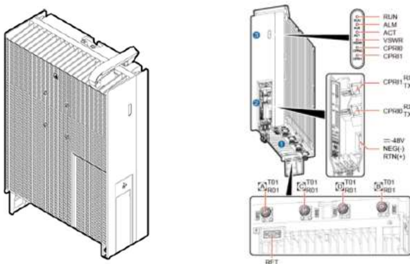
Slika 3.5 RRU5502 jedinica
