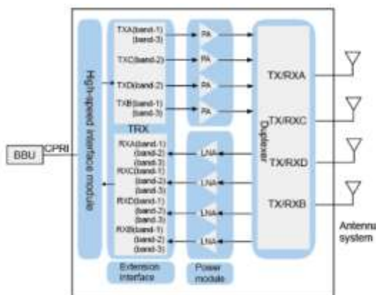
Slika 3.4 Struktura RRU jedinice
