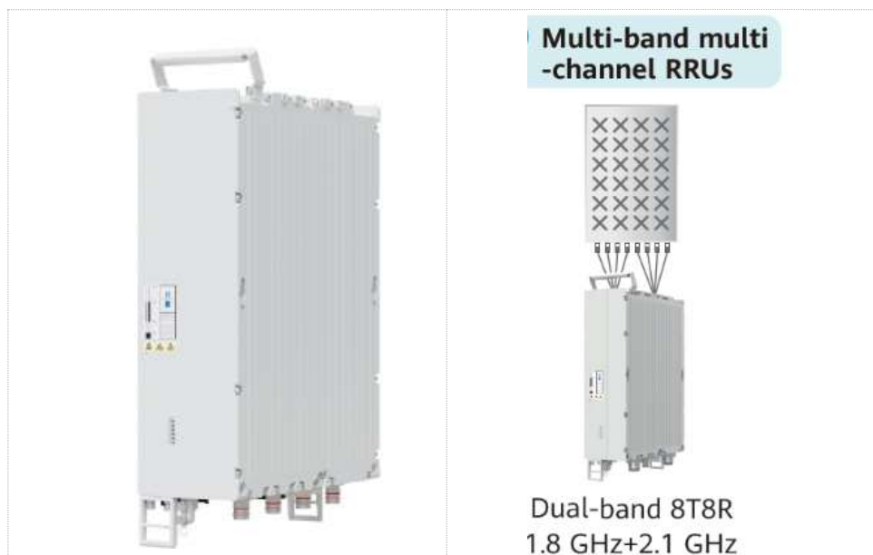
Slika 3.7 RRU5513t jedinica
