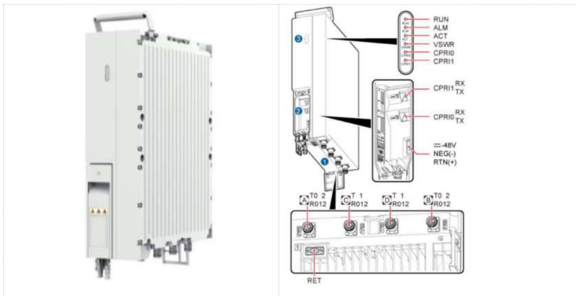
Slika 3.6 RRU5509t jedinica
