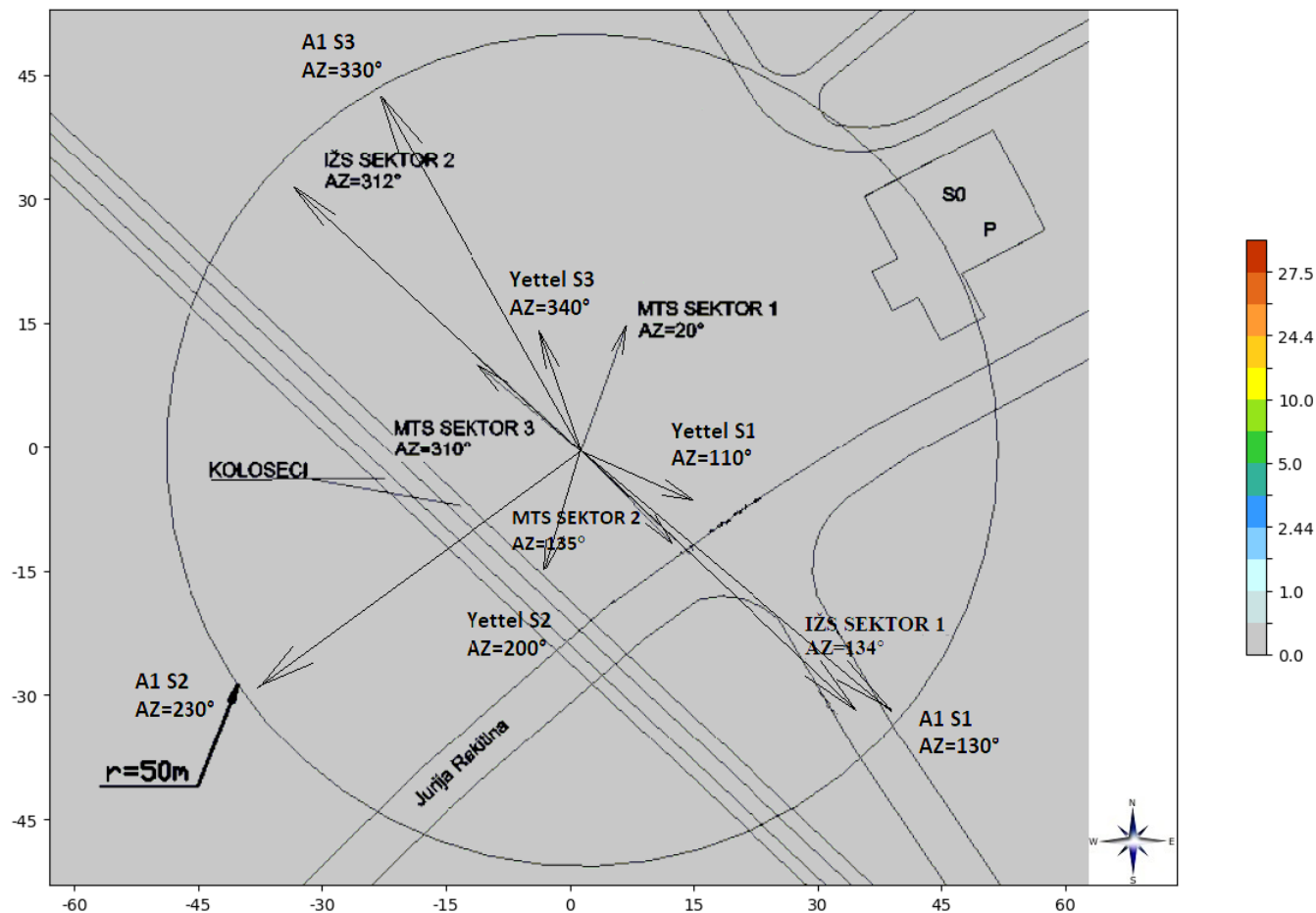
Slika 6.13. Rezultati proračuna jačine električnog polja na tlu sa uvažavanom prosečnom visinom čoveka, za slučaj kada bazna stanica LTE2100 A1 Srbija radi sa maksimalnim kapacitetom.
