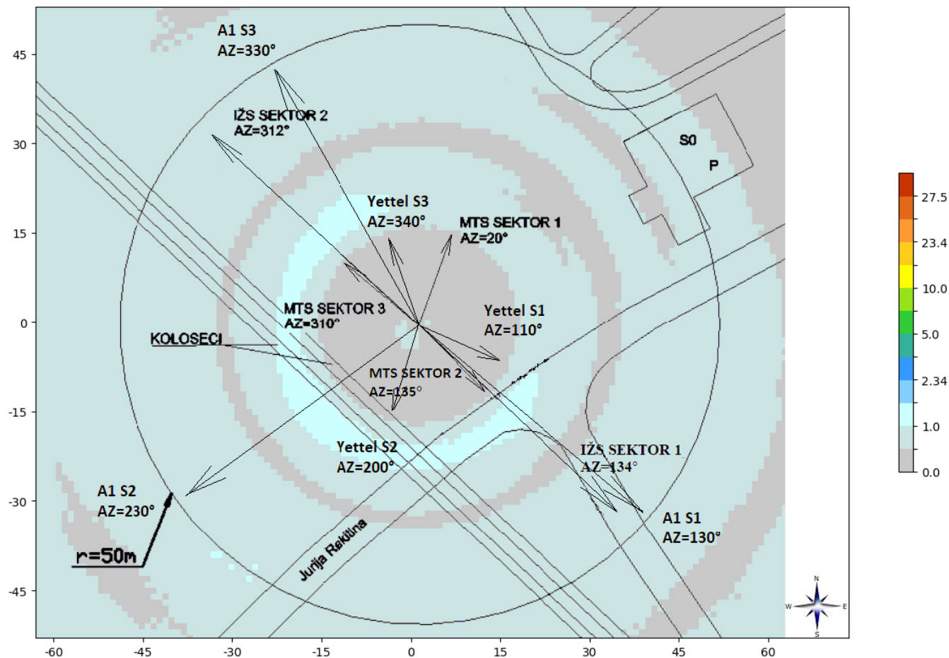
Slika 6.10. Rezultati proračuna jačine električnog polja na tlu sa uvažanom prosečnom visinom čoveka, za slučaj kada bazna stanica LTE1800 A1 Srbija radi sa maksimalnim kapacitetom.
