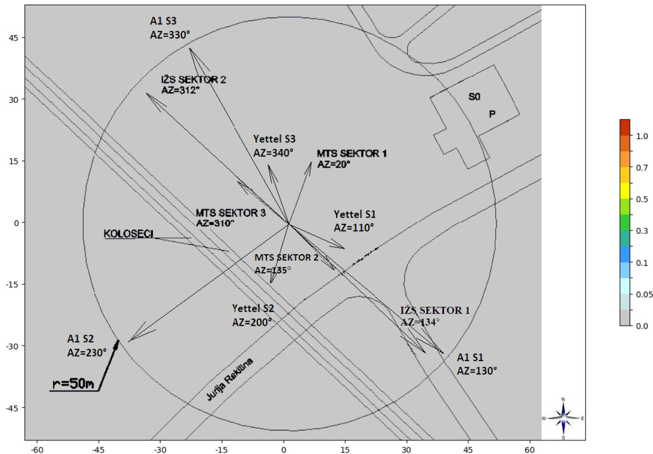
Slika 6.14. Rezultati proračuna faktora izlaganja na tlu sa uvažanom prosečnom visinom čoveka, za slučaj kada svi sistemi A1 Srbija na lokaciji rade sa maksimalnim kapacitetom.
