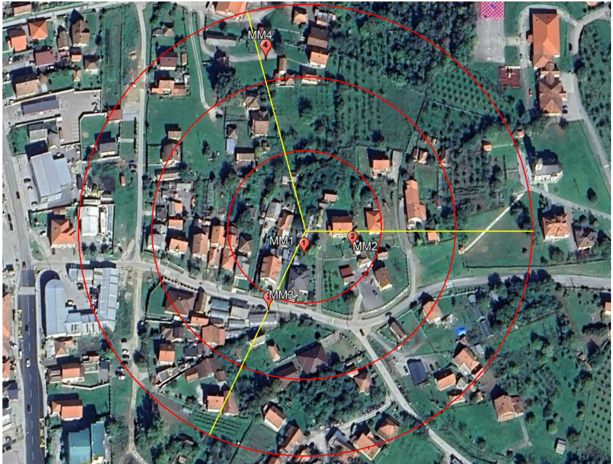
Slika 6: Prikaz mernih mesta u lokalnoj zoni BS Telekom Srbija Lazarevac 3 (ETS)
