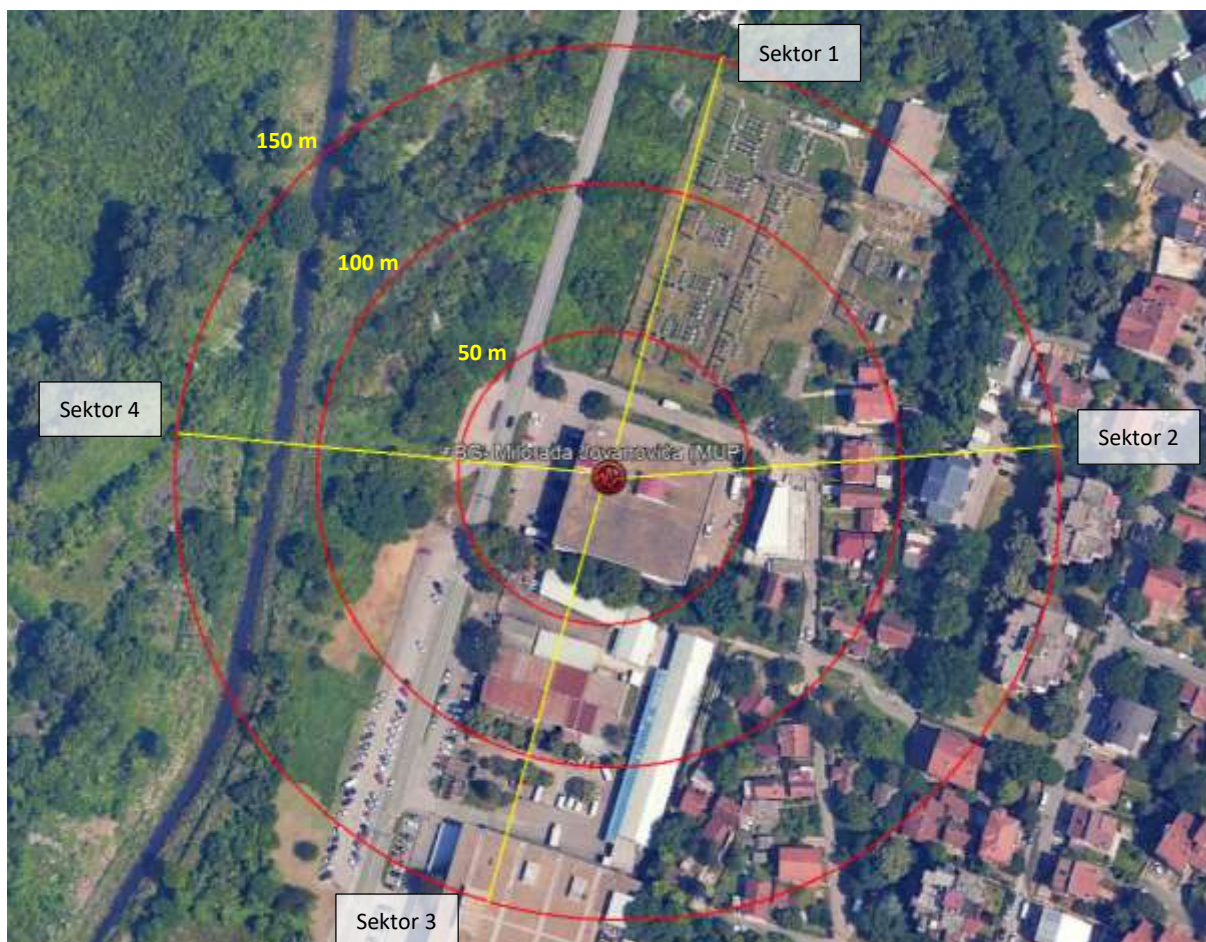
Slika 2.5 Pravci zračenja antenskih sistema predmetne bazne stanice
