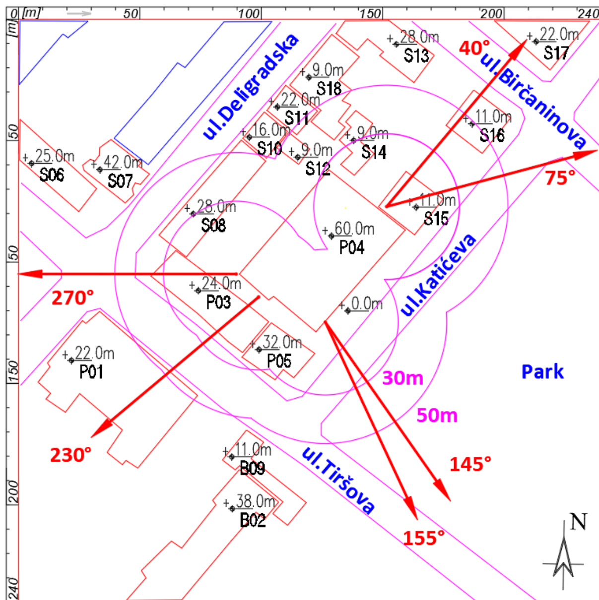
Slika 2.5 Dijagram objekata u okruženju radio bazne stanice „BG-TK Centar“- BG02/BGH02/BGU02/BGL02/BGO02/BGJ02
