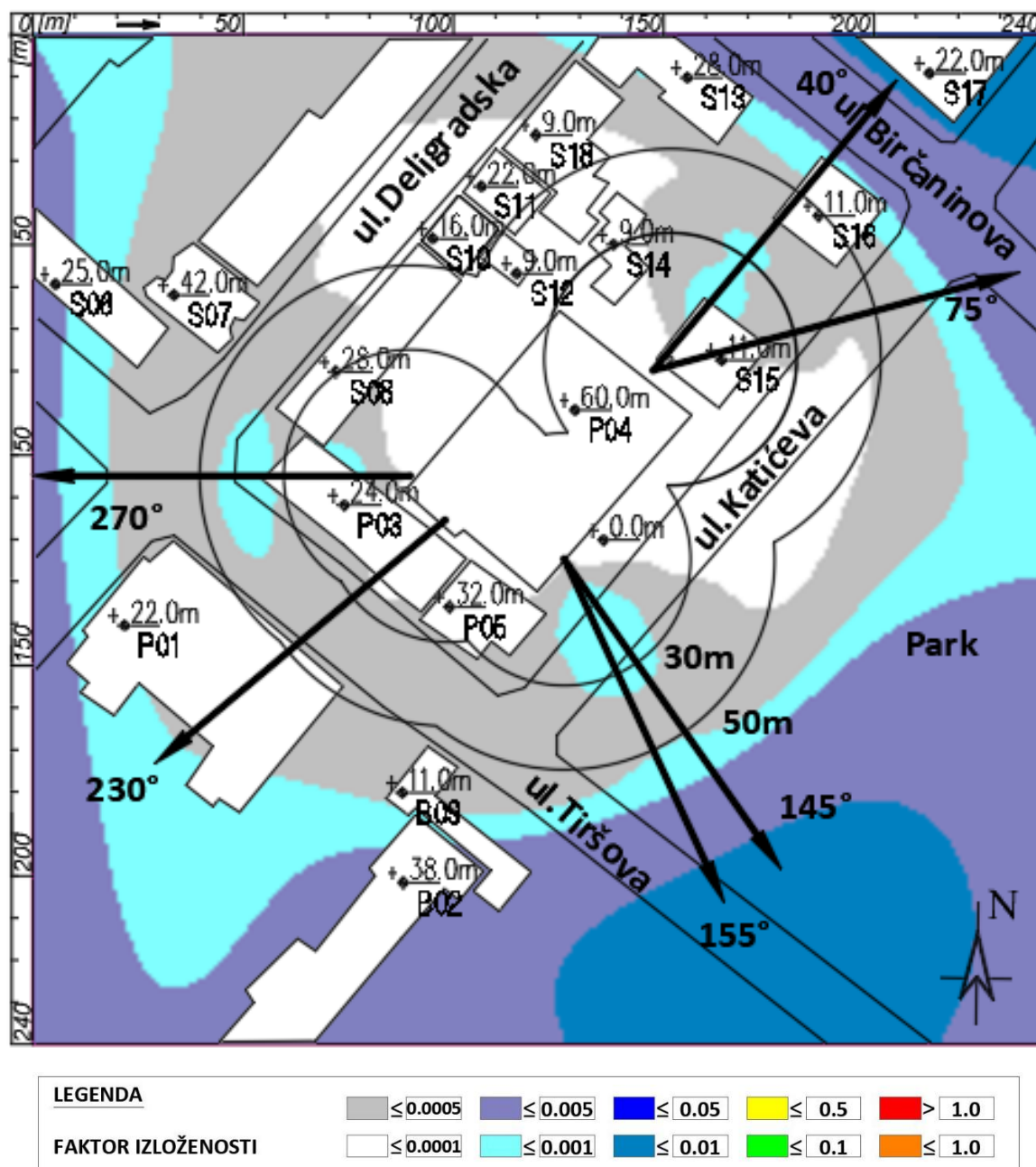
Slika 4.18 Maksimalna proračunata vrednost ukupnog faktora izloženosti na nivou tla u slučaju rada svih sistema na predmetnoj lokaciji operatora TELEKOM I Cetin iznosi: 0.0081
