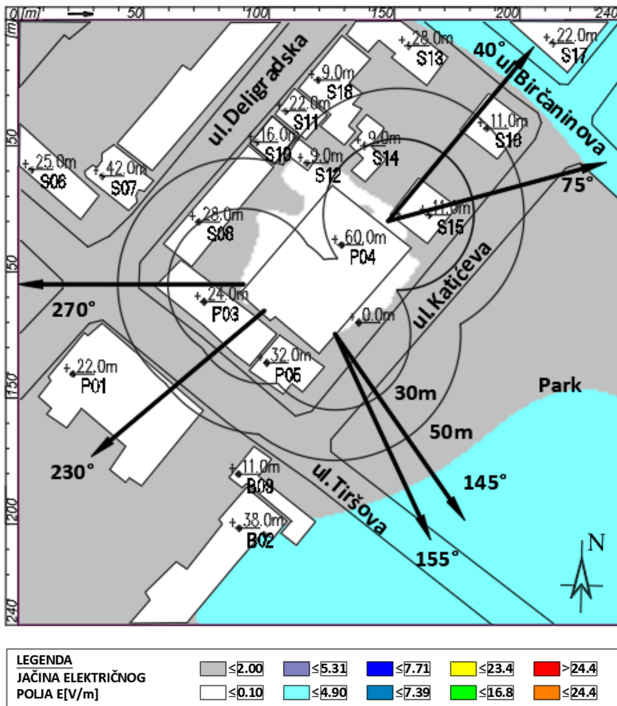
Slika 4.16 Maksimalna proračunata vrednost električnog polja na nivou tla u slučaju rada svih sistema na predmetnoj lokaciji operatora TELEKOM iznosi: 4.73 V/m.
