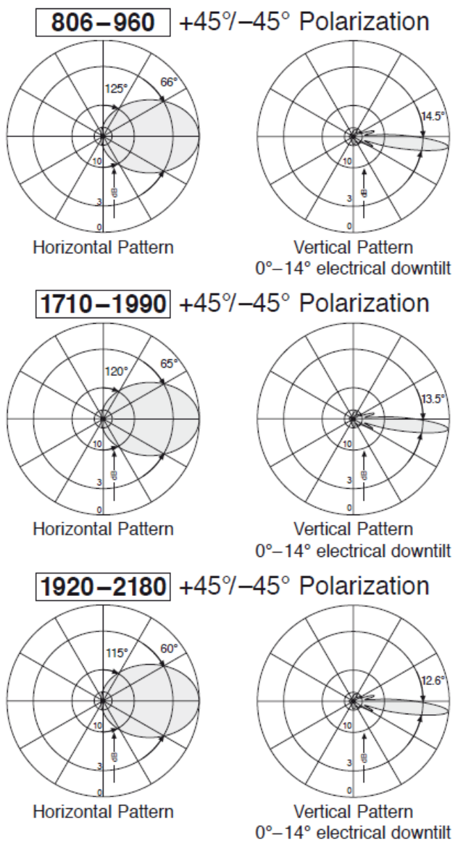
Slika 8.6 Dijagram zračenja antene K80010290
