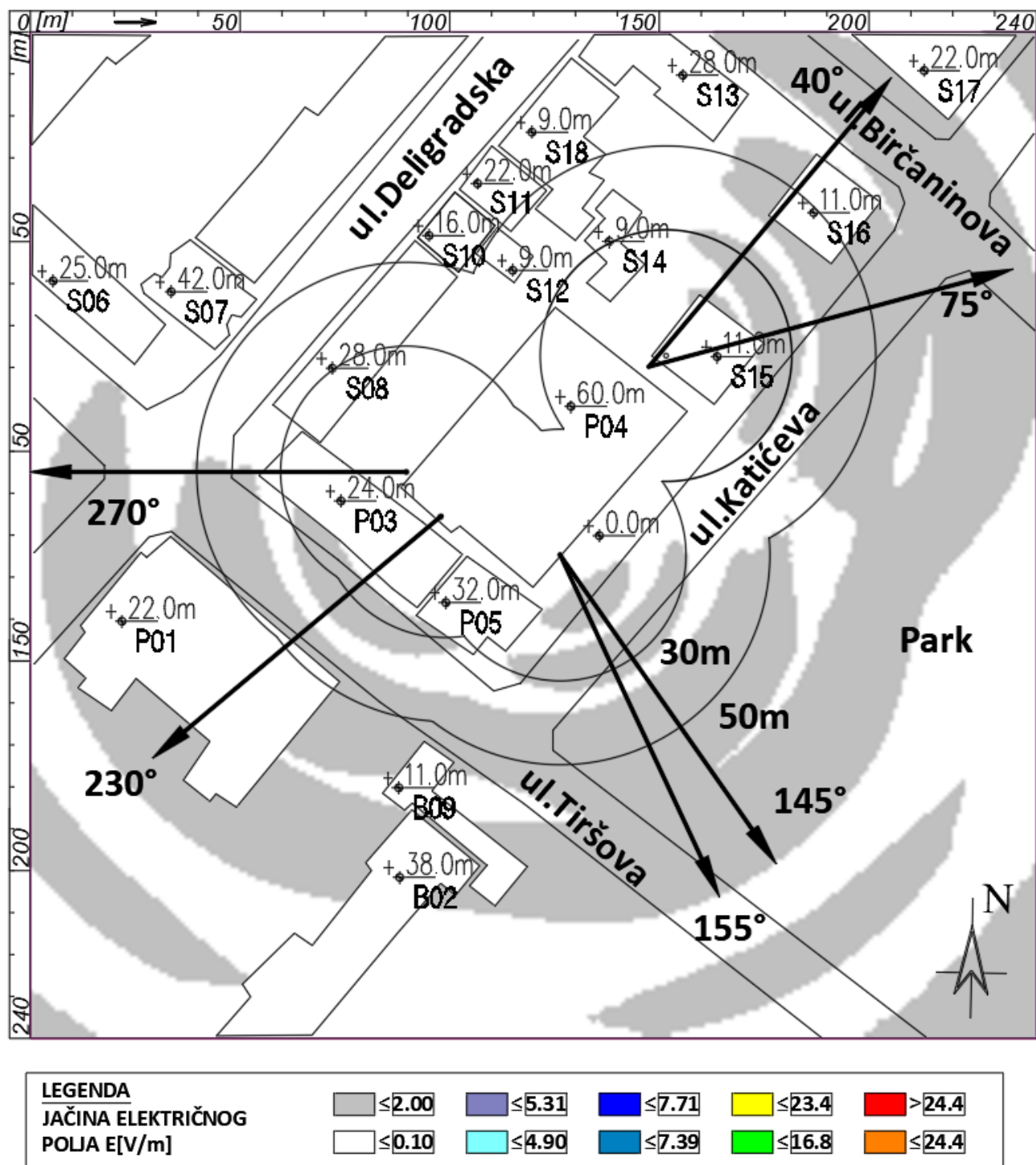
Slika 4.11 Maksimalna proračunata vrednost električnog polja na nivou tla u slučaju rada sistema DCS1800 operatora TELEKOM iznosi: 0.37 V/m Maksimalni faktor izloženosti na nivou tla u slučaju rada sistema DCS1800 operatora TELEKOM iznosi: 0.00004
