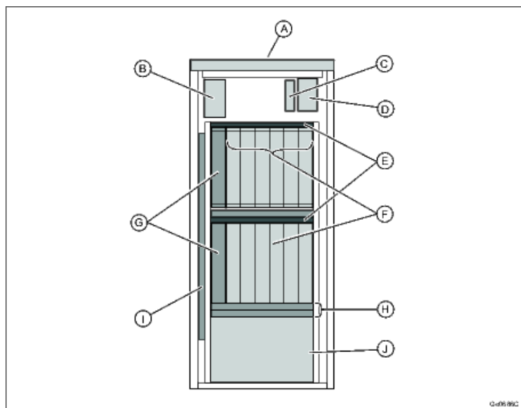
Slika 8.3 Hardver kabineta BS6201 (-48 V DC)
