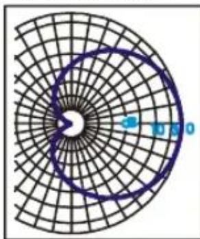
Slika 8.5 Dijagram zračenja antene APX186515-T6
