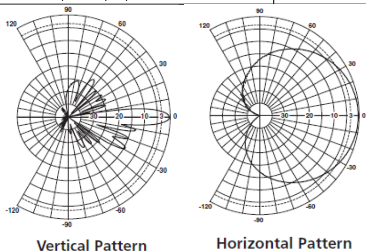
Slika 8.4 Dijagram zračenja antene APX906516-T9
