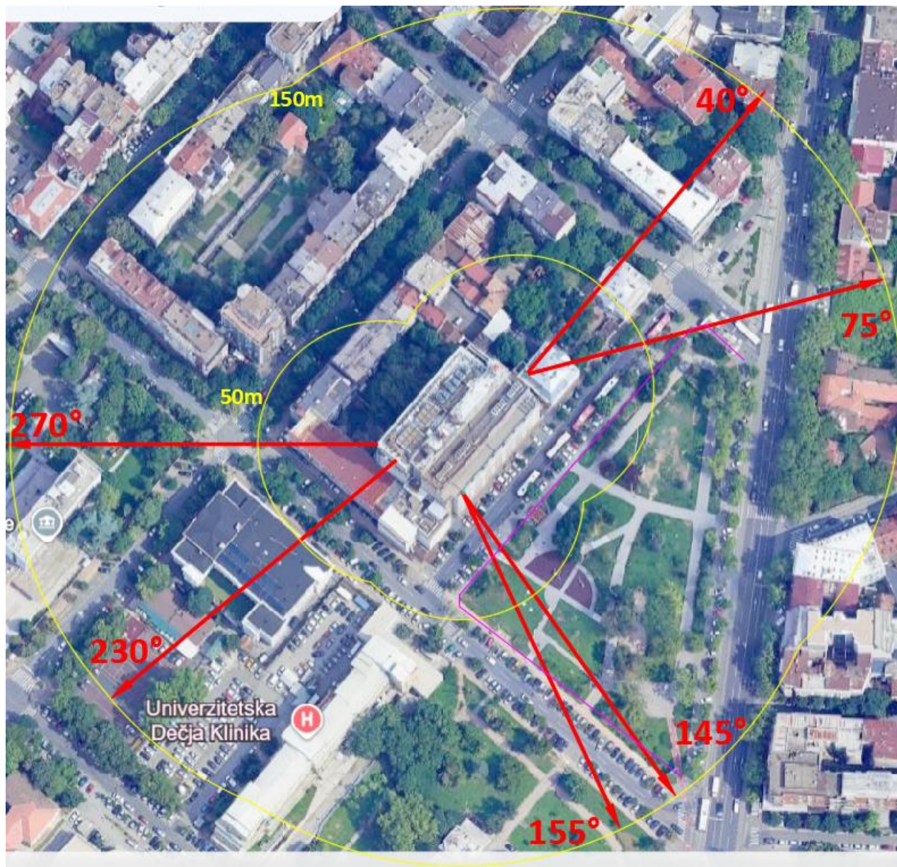
Slika 2.4 Dijagram zračenja radio bazne stanice „BG-TK Centar“- BG02/BGH02/BGU02/BGL02/BGO02/BGJ02 3
