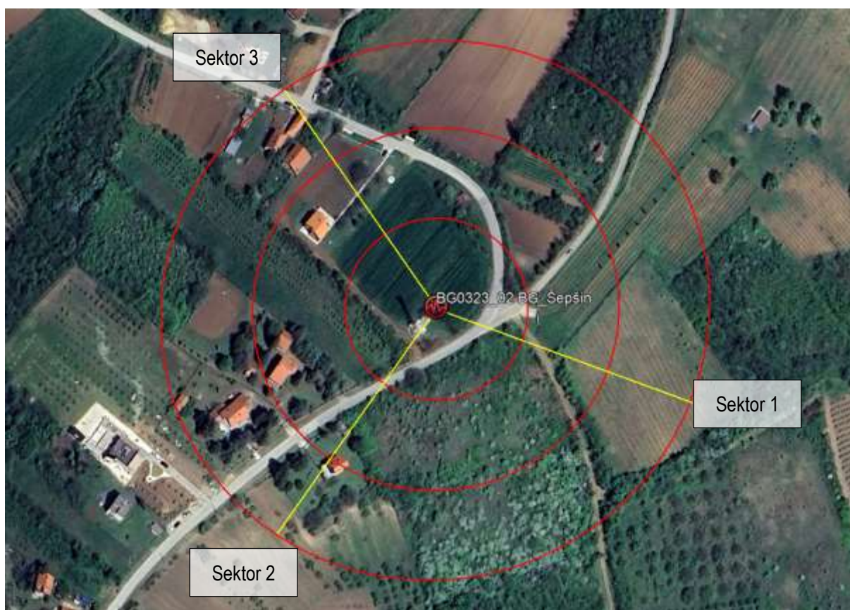
Slika 2.5 Pravci zračenja antenskog sistema predmetne bazne stanice
