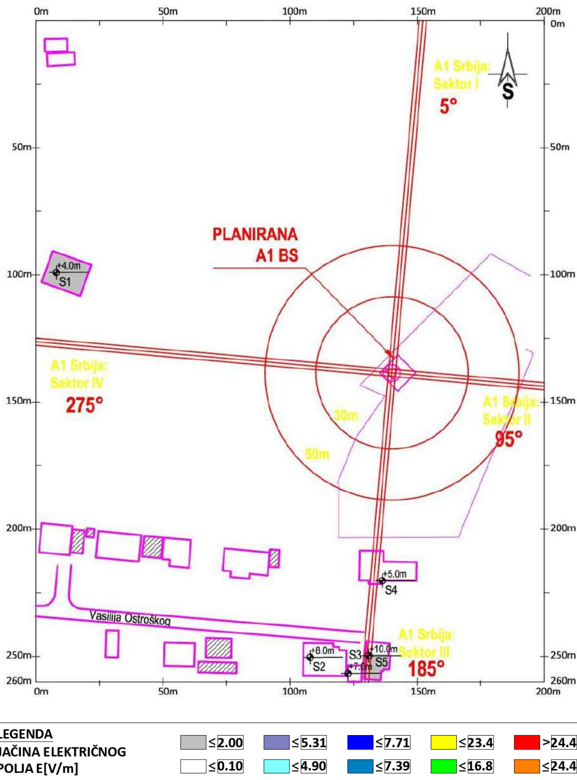
Slika 4.1 Rezultati proračuna jačine električnog polja sistema GSM900 operatora A1 Srbija , u zonama povećane osetljivosti
