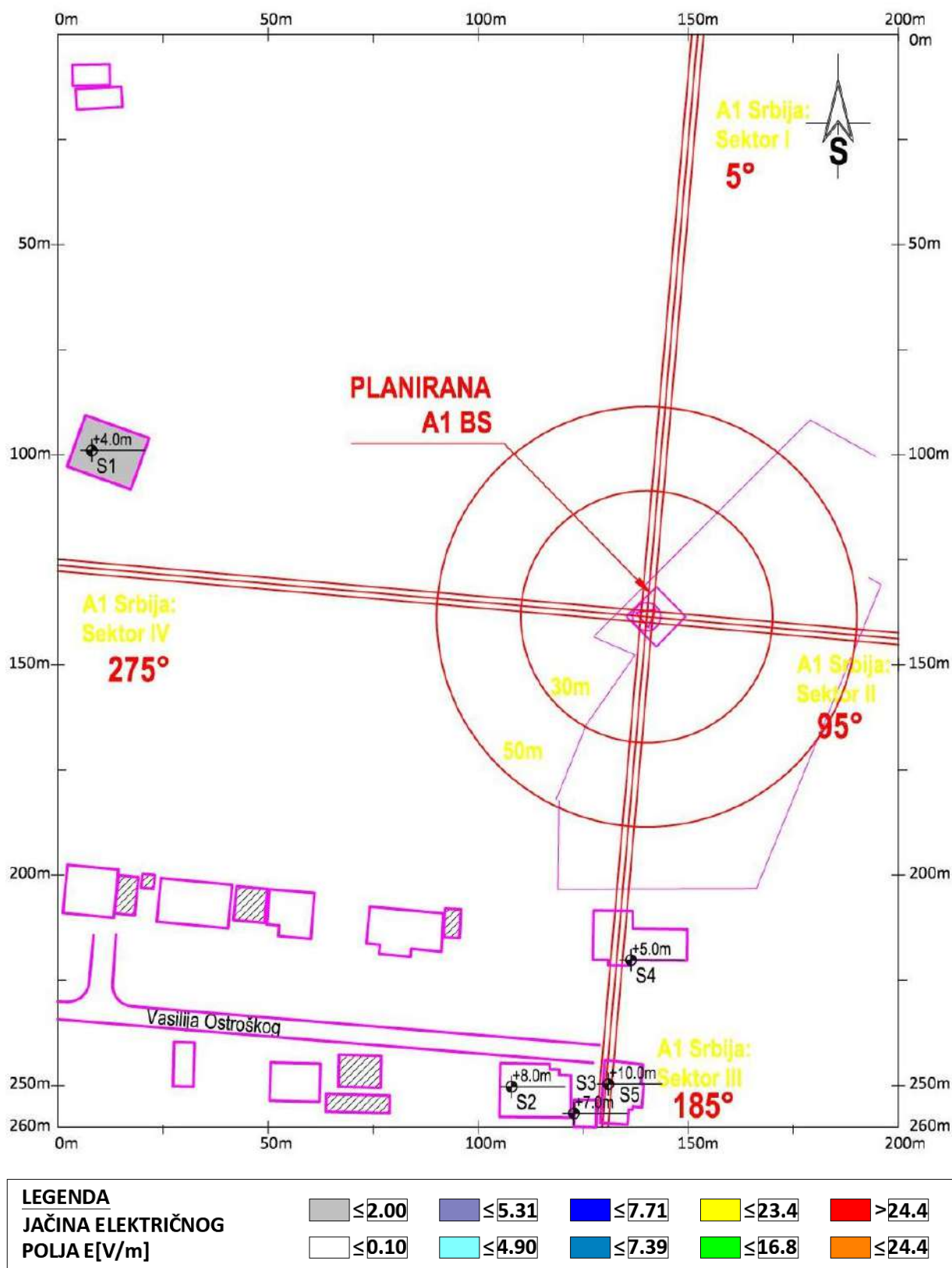
Slika 4.4 Rezultati proračuna jačine električnog polja sistema LTE2100 operatora A1 Srbija , u zonama povećane osetljivosti
