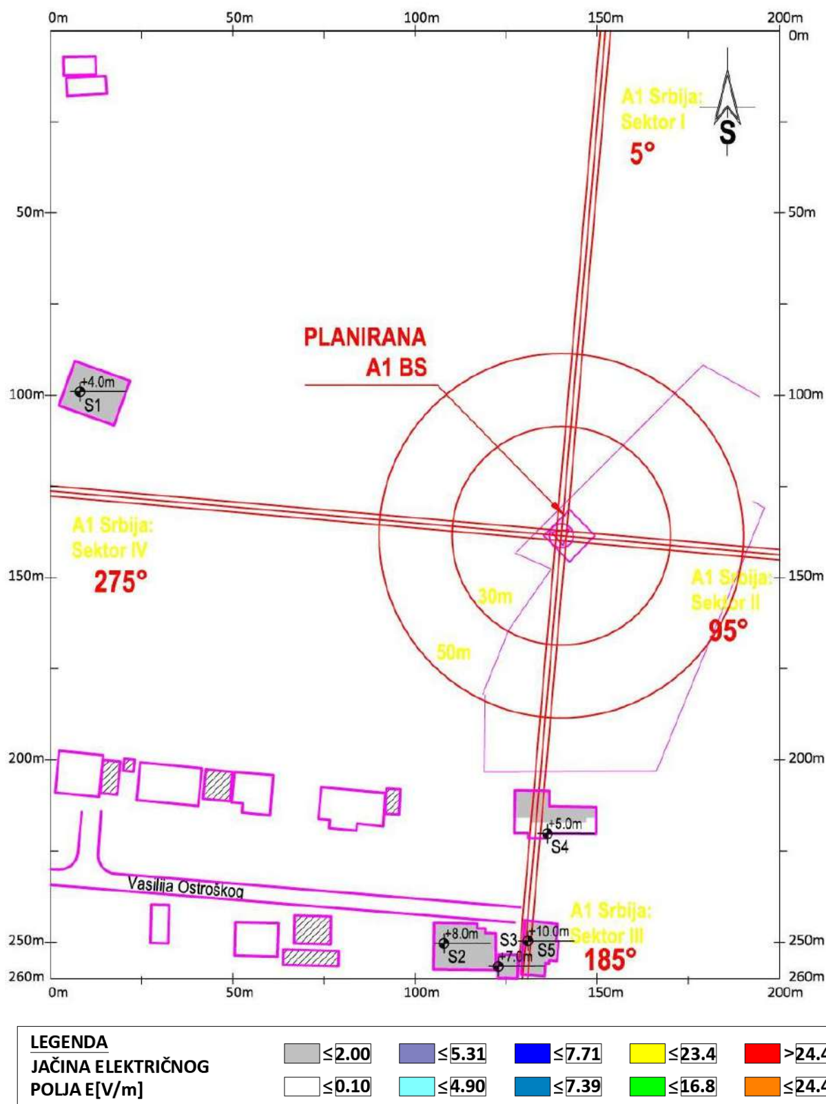
Slika 4.3 Rezultati proračuna jačine električnog polja sistema LTE800 operatora A1 Srbija , u zonama povećane osetljivosti
