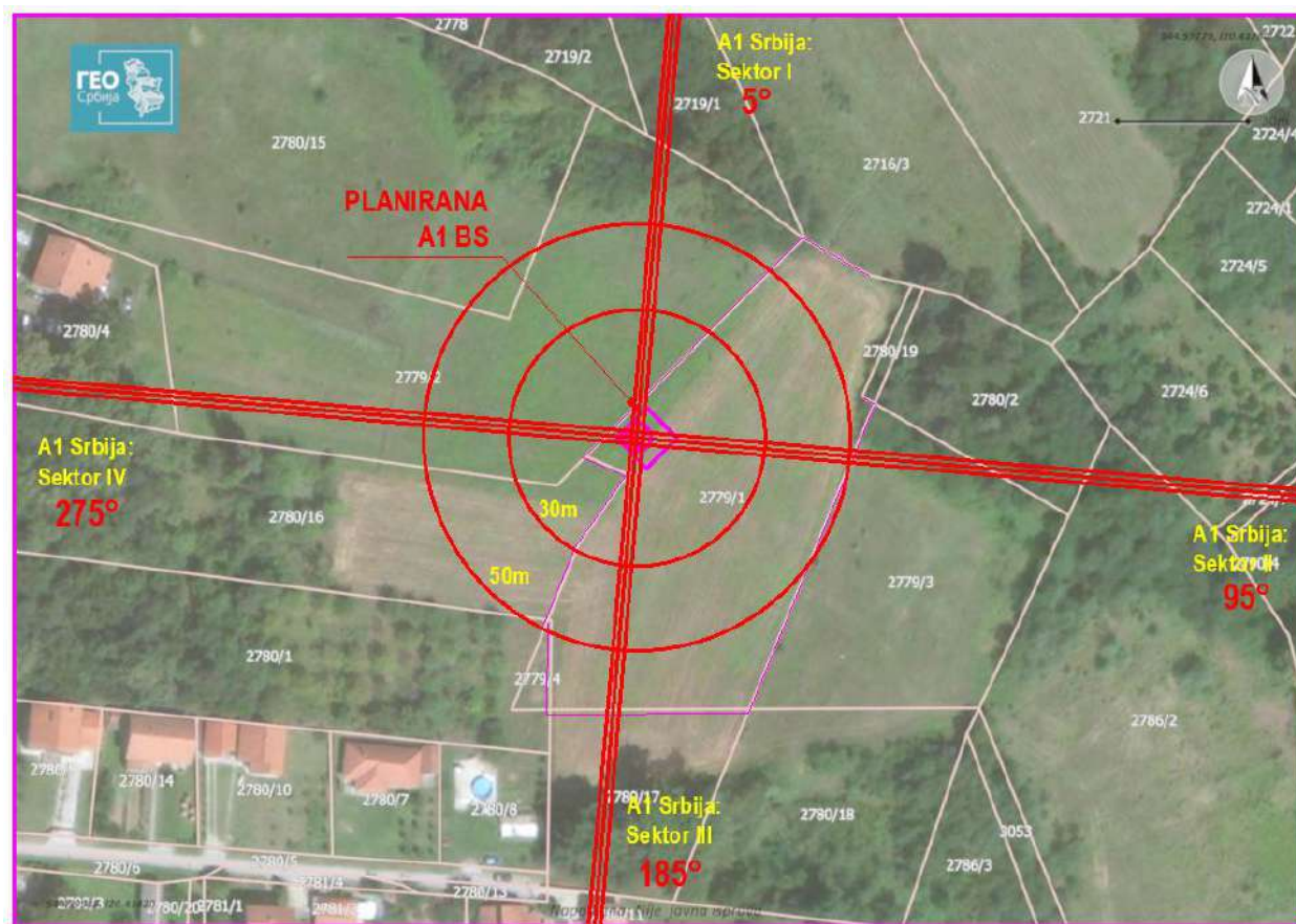
Slika 2.4 Dijagram zračenja planirane radio bazne stanice „BG0934_02 BG_Barajevo_2“ 3
