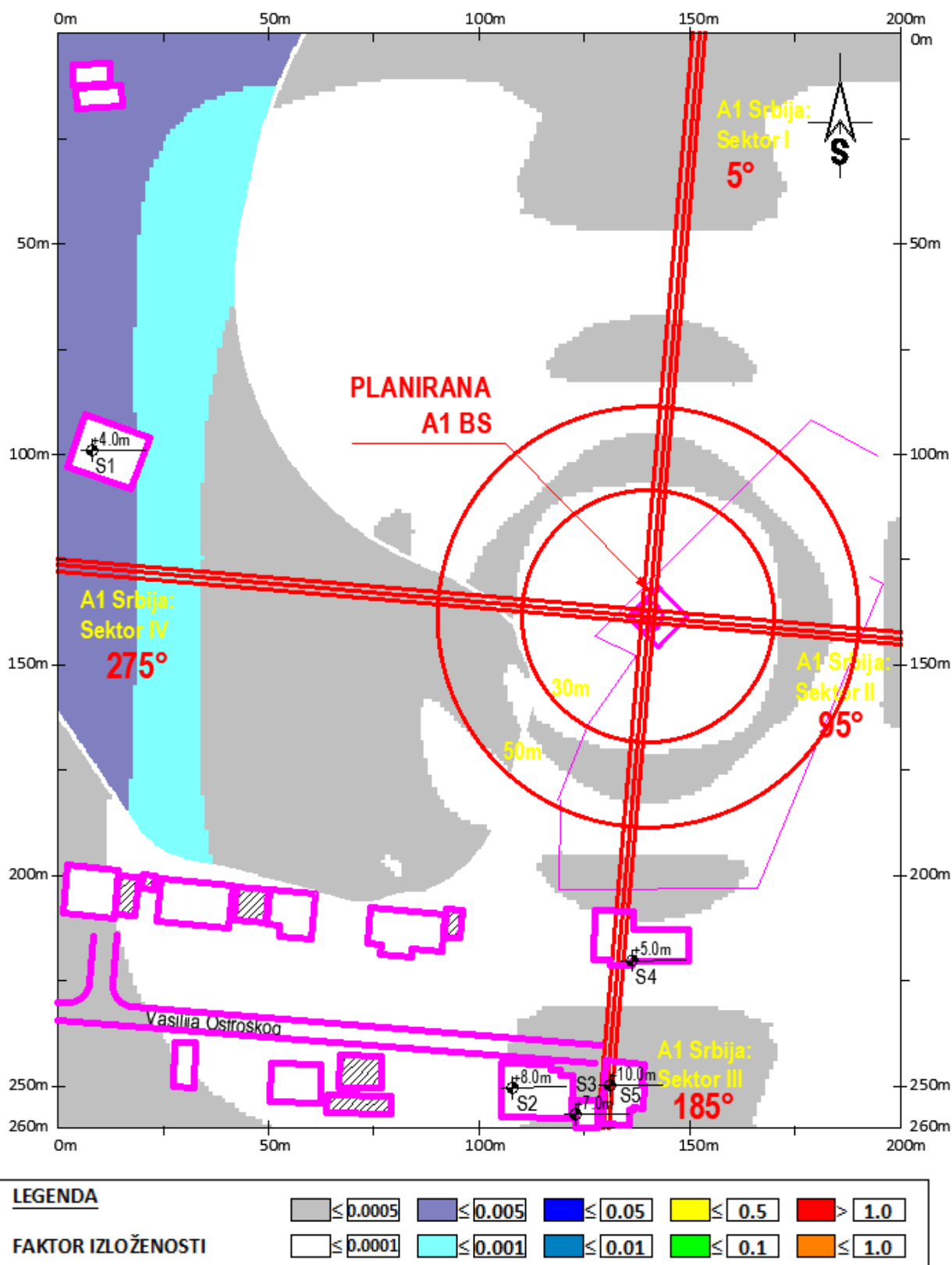
Slika 4.12 Rezultati proračuna faktora izloženosti u široj okolini lokacije bazne stanice na javnom području, na visini +1.70m (prosečna visina čoveka) u odnosu na nivo tla za slučaj rada sistema GSM900, LTE1800, LTE800 i LTE2100 operatora A1 Srbija .
