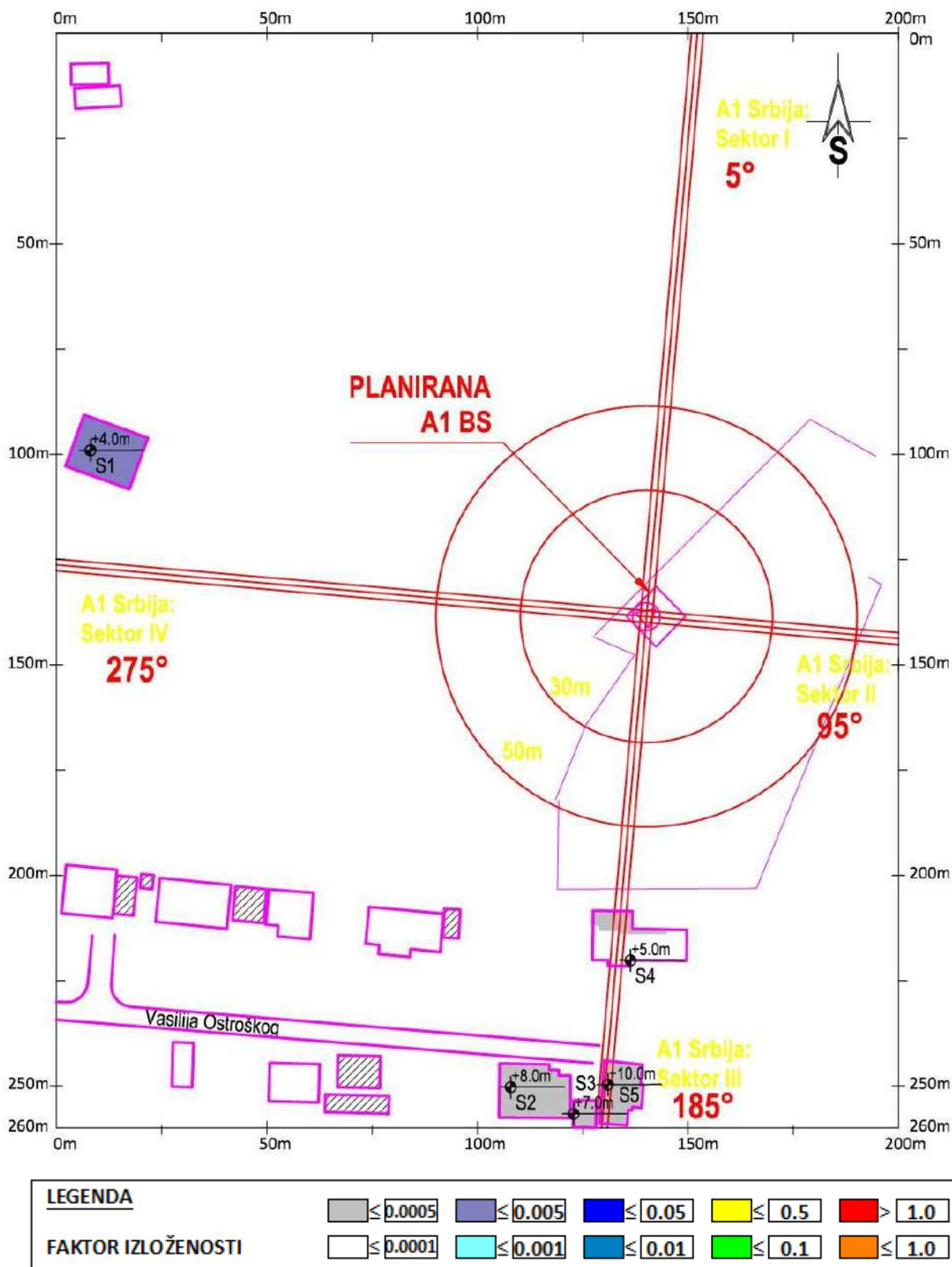
Slika 4.6 Rezultati proračuna faktora izloženosti za slučaj rada svih planiranih sistema na lokaciji- GSM900, LTE1800, LTE800 i LTE2100 operatora A1 Srbija , u zonama povećane osetljivosti
