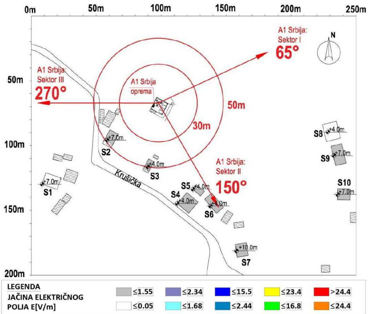
Slika 4.2 Rezultati proračuna jačine električnog polja u objektima na najizloženijim spratovima za slučaj rada sistema LTE1800 operatora A1 Srbija
