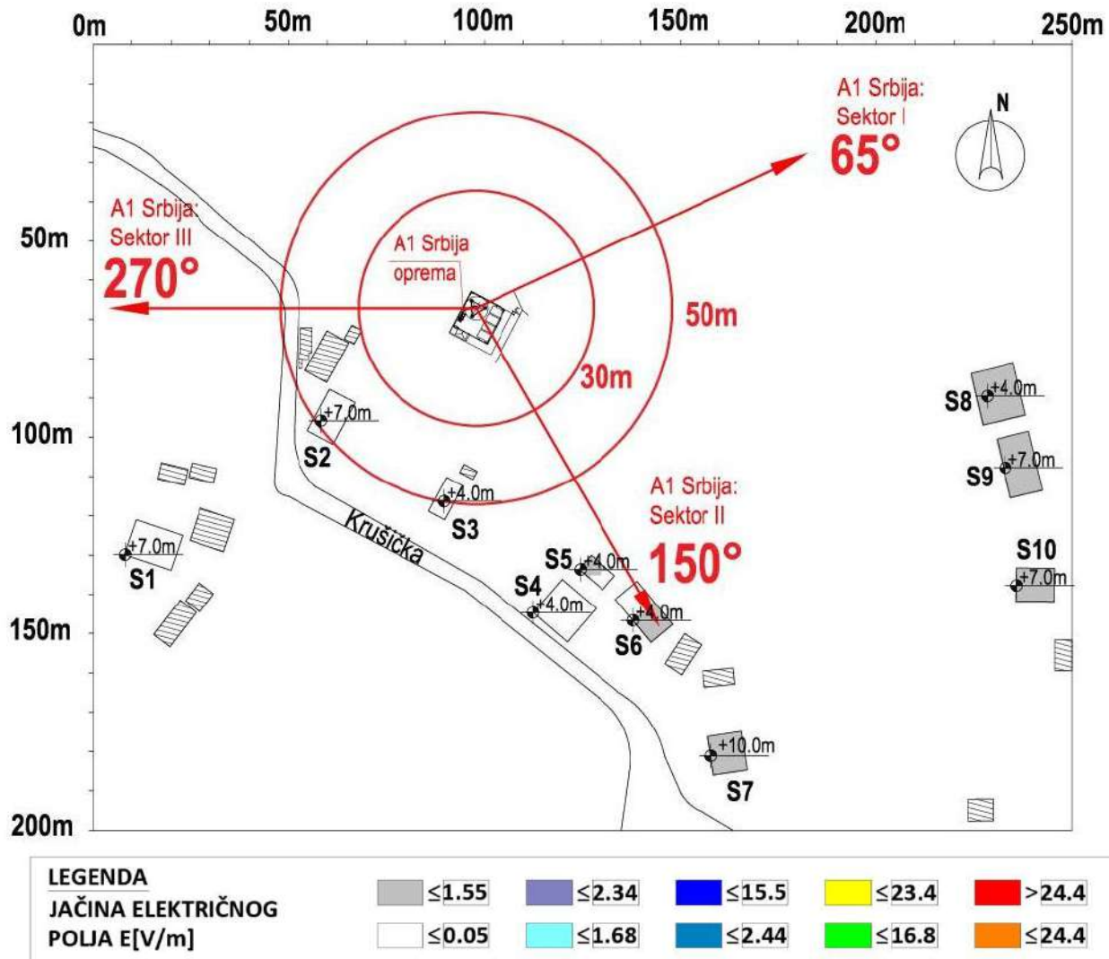
Slika 4.1 Rezultati proračuna jačine električnog polja u objektima na najizloženijim spratovima za slučaj rada sistema GSM900 operatora A1 Srbija
