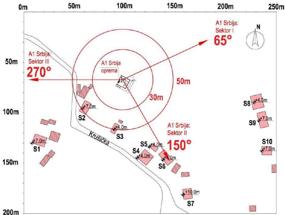
Slika 2.5 Dijagram objekata u okruženju radio bazne stanice "BG0784_02 BG_Boždarevac"
