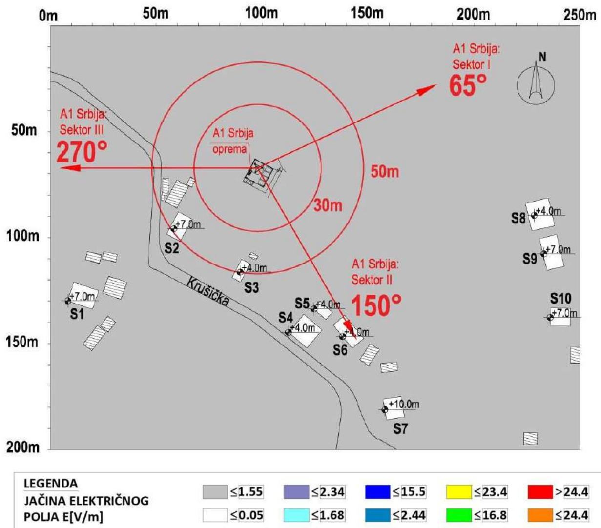
Slika 4.11 Rezultati proračuna jačine električnog polja u široj okolini lokacije bazne stanice na visini +1.70m (prosečna visina čoveka) u odnosu na nivo tla za slučaj rada GSM900/LTE1800/LTE800/LTE2100 operatora A1 Srbija . Maksimalna proračunata vrednost jačine električnog polja iznosi E=0.89V/m .
