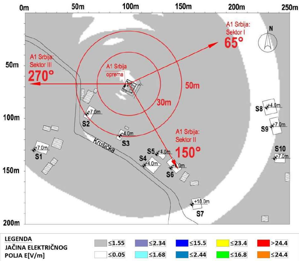
Slika 4.10 Rezultati proračuna jačine električnog polja u široj okolini lokacije bazne stanice na visini +1.70m (prosečna visina čoveka) u odnosu na nivo tla za slučaj rada LTE2100 operatora A1 Srbija . Maksimalna proračunata vrednost jačine električnog polja iznosi E=0.50 V/m. Maksimalna proračunata vrednost faktora izloženosti iznosi 0.00006 .
