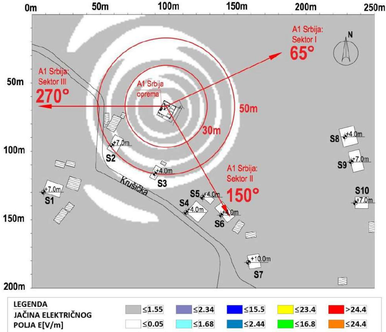
Slika 4.7 Rezultati proračuna jačine električnog polja u široj okolini lokacije bazne stanice na visini +1.70m (prosečna visina čoveka) u odnosu na nivo tla za slučaj rada sistema GSM900 operatora A1 Srbija .
