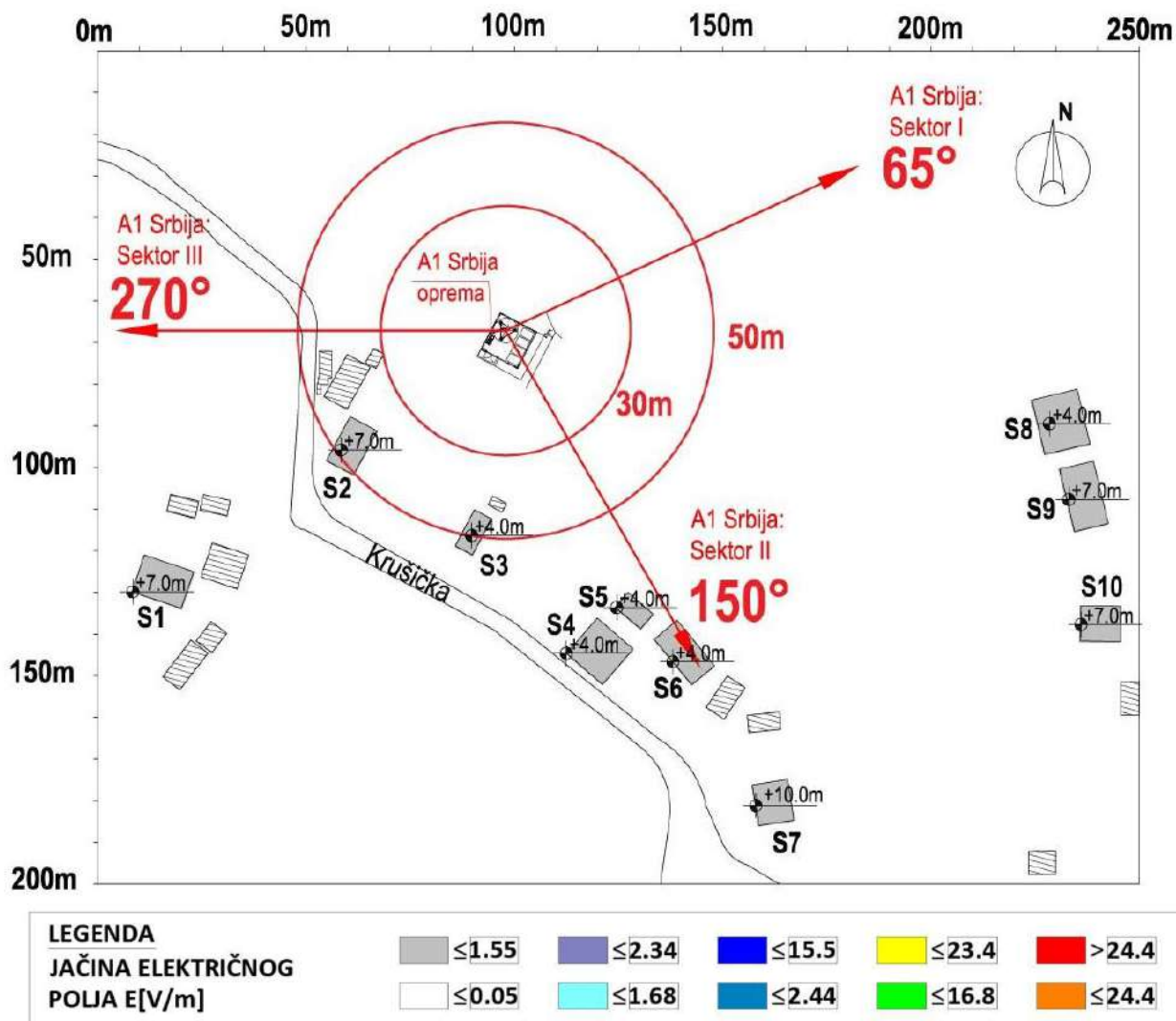
Slika 4.3 Rezultati proračuna jačine električnog polja u objektima na najizloženijim spratovima za slučaj rada sistema LTE800 operatora A1 Srbija
