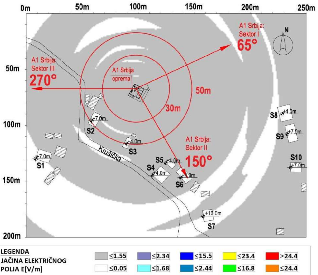
Slika 4.8 Rezultati proračuna jačine električnog polja u široj okolini lokacije bazne stanice na visini +1.70m (prosečna visina čoveka) u odnosu na nivo tla za slučaj rada sistema LTE1800 operatora A1 Srbija .
