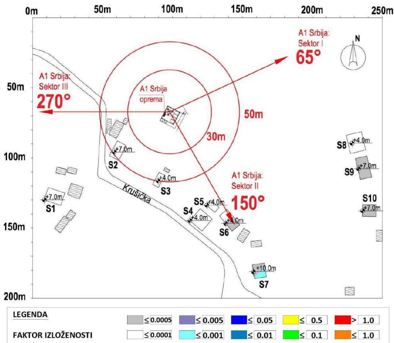
Slika 4.6 Rezultati proračuna faktora izloženosti u objektima na najizloženijim spratovima za slučaj rada sistema GSM900/LTE1800/LTE800/LTE2100 operatora A1 Srbija
