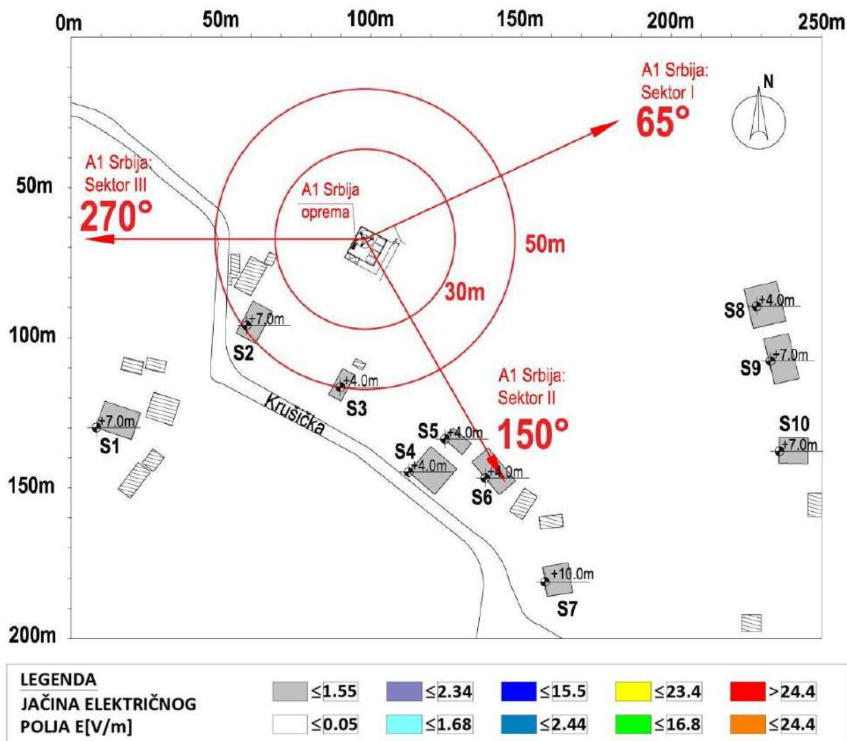
Slika 4.5 Rezultati proračuna jačine električnog polja u objektima na najizloženijim spratovima za slučaj rada sistema GSM900/LTE1800/LTE800/LTE2100 operatora A1 Srbija
