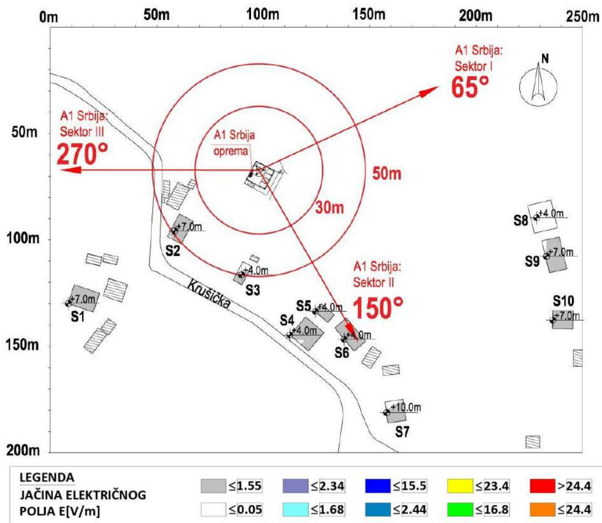
Slika 4.4 Rezultati proračuna jačine električnog polja u objektima na najizloženijim spratovima za slučaj rada sistema LTE2100 operatora A1 Srbija
