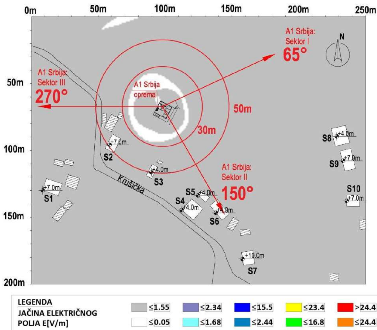
Slika 4.9 Rezultati proračuna jačine električnog polja u široj okolini lokacije bazne stanice na visini +1.70m (prosečna visina čoveka) u odnosu na nivo tla za slučaj rada LTE800 operatora A1 Srbija . Maksimalna proračunata vrednost jačine električnog polja iznosi E=0.57 \text{ V/m} .
