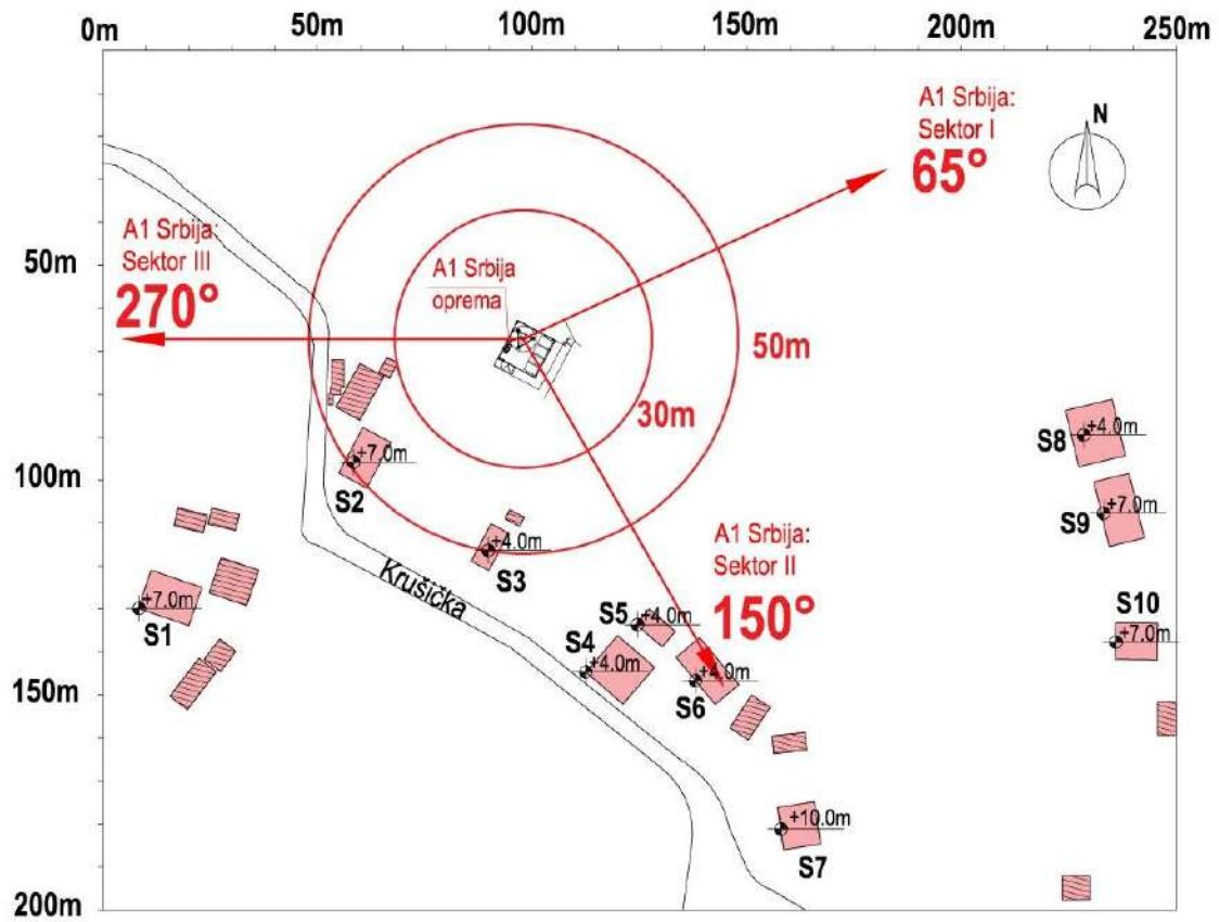
Slika 5.2 Dijagram objekata u okruženju radio bazne stanice «BG0784_02 BG_Boždarevac»
