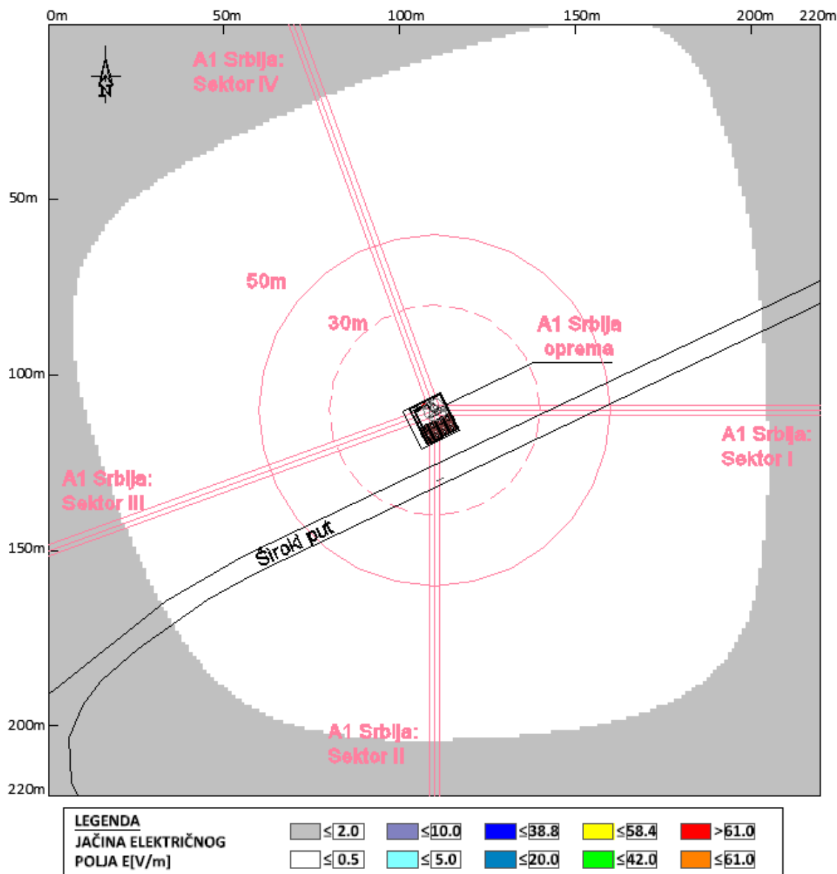
Slika 4.3 Rezultati proračuna jačine električnog polja u široj okolini lokacije bazne stanice na javnom području, na visini +1.70m (prosečna visina čoveka) u odnosu na nivo tla za slučaj rada sistema LTE800 operatora A1 Srbija .
