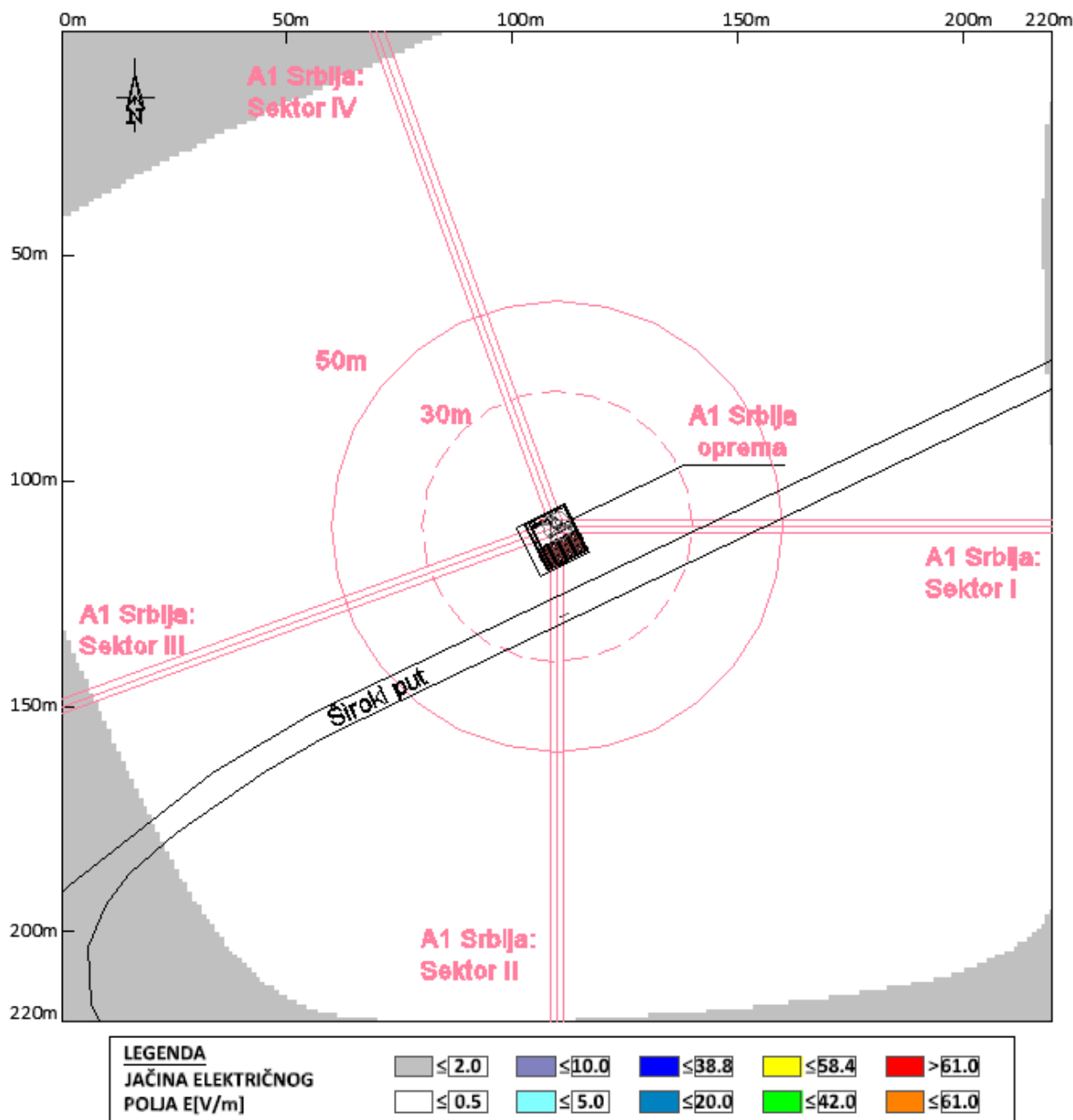
Slika 4.1 Rezultati proračuna jačine električnog polja u široj okolini lokacije bazne stanice na javnom području , na visini +1.70m (prosečna visina čoveka) u odnosu na nivo tla za slučaj rada sistema GSM900 operatora A1 Srbija .
