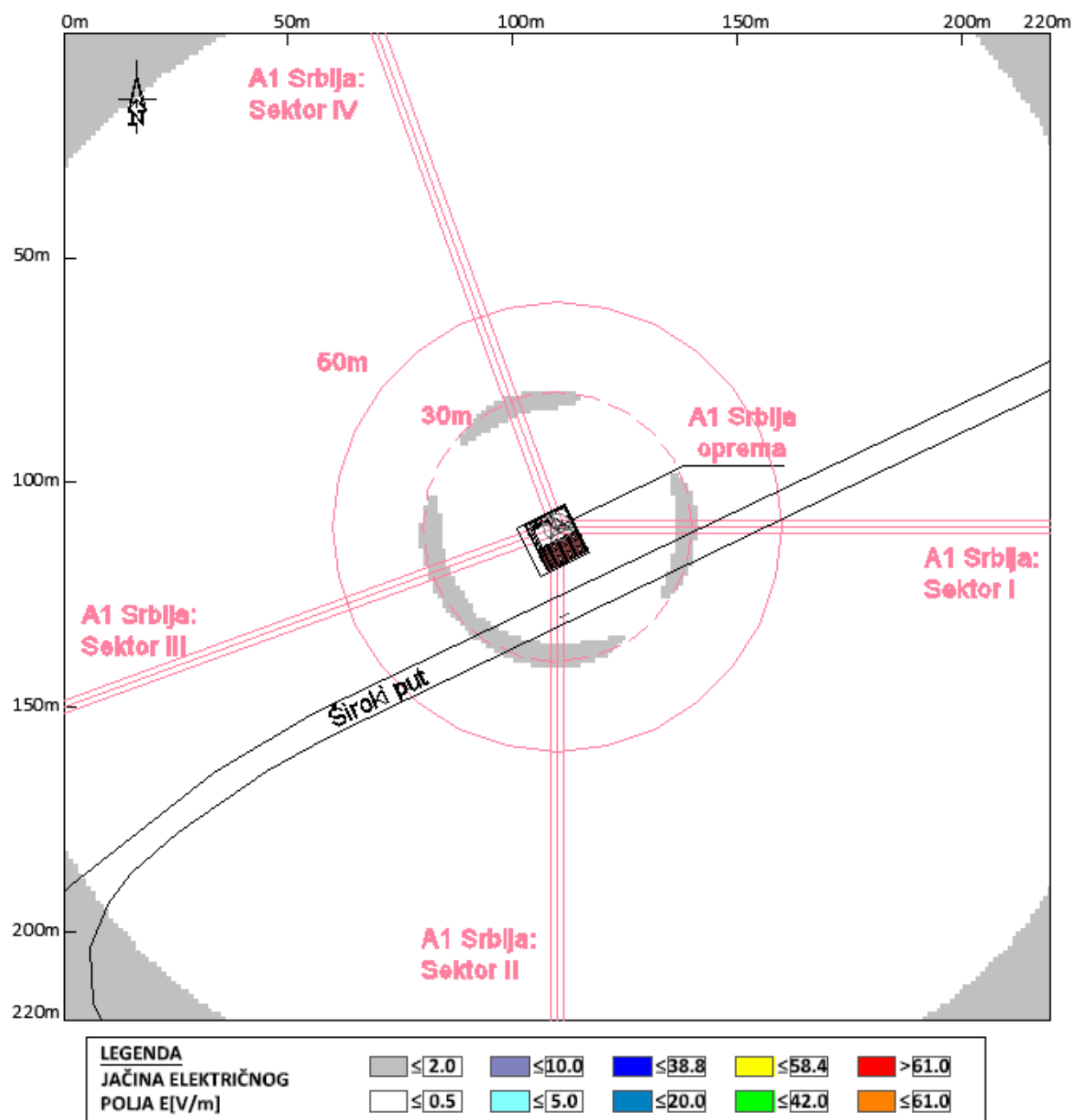
Slika 4.2 Rezultati proračuna jačine električnog polja u široj okolini lokacije bazne stanice na javnom području , na visini +1.70m (prosečna visina čoveka) u odnosu na nivo tla za slučaj rada sistema LTE1800 operatora A1 Srbija .
