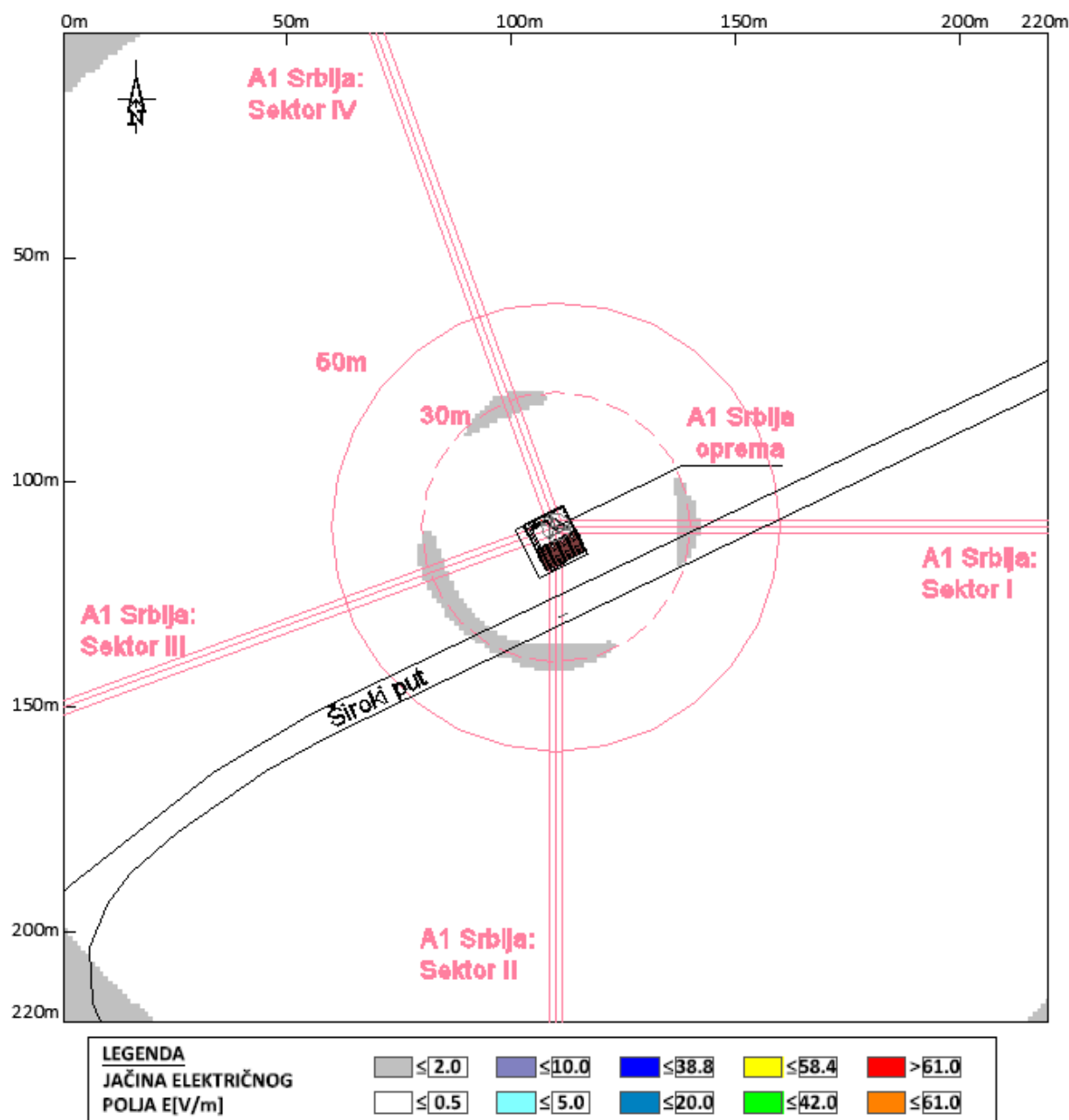
Slika 4.4 Rezultati proračuna jačine električnog polja u široj okolini lokacije bazne stanice na javnom području, na visini +1.70m (prosečna visina čoveka) u odnosu na nivo tla za slučaj rada sistema LTE2100 operatora A1 Srbija .
