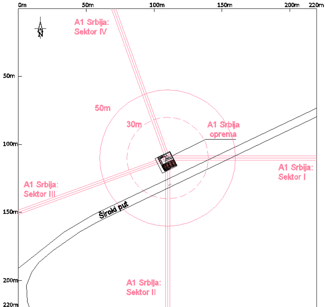
Slika 5.2 Dijagram objekata u okruženju radio bazne stanice «BG0551_02 BG_Batajnica_Eko_Unija»
