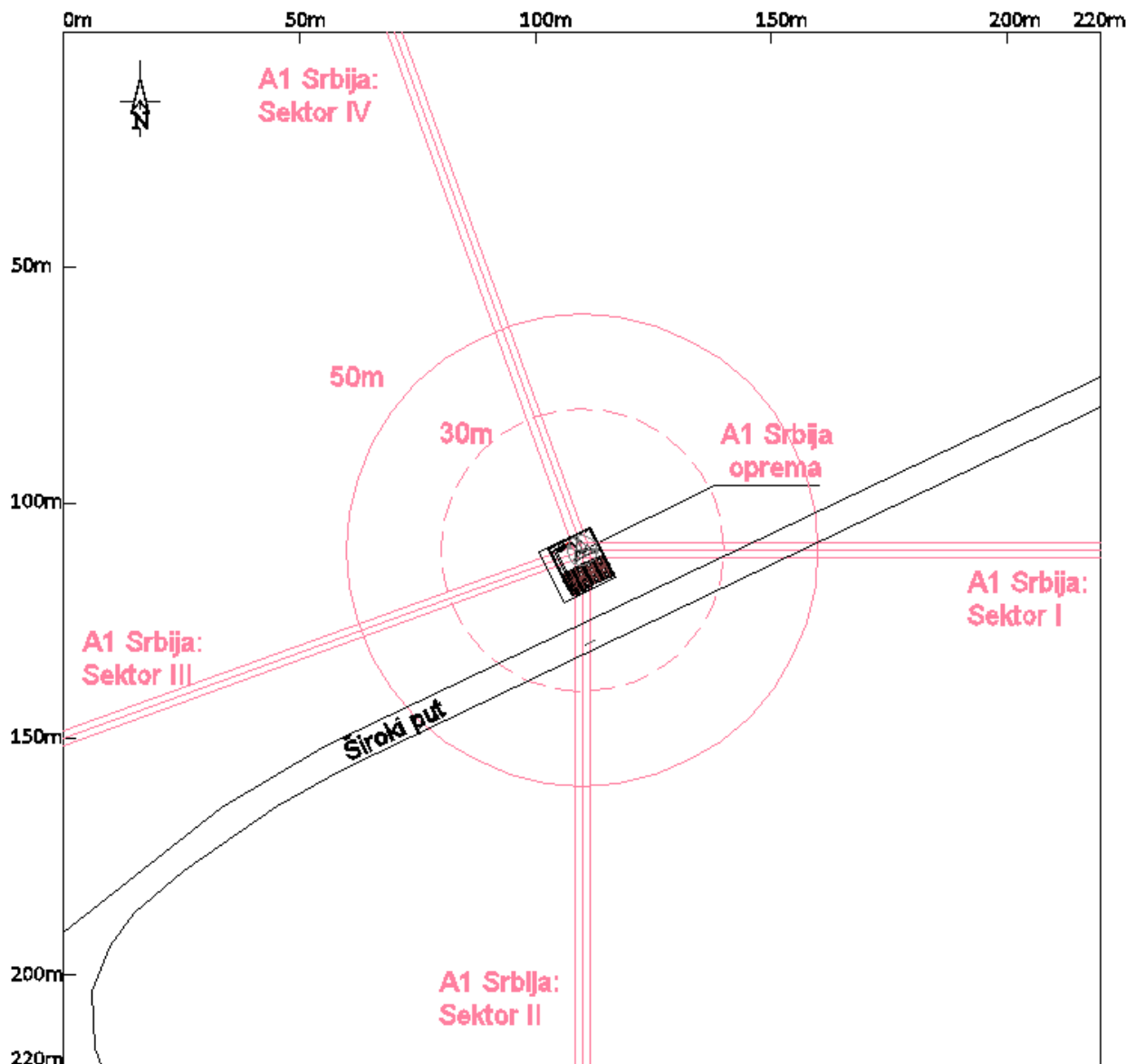
Slika 2.5 Dijagram objekata u okruženju radio bazne stanice "BG0551_02 BG_Batajnica_Eko_Unija"
