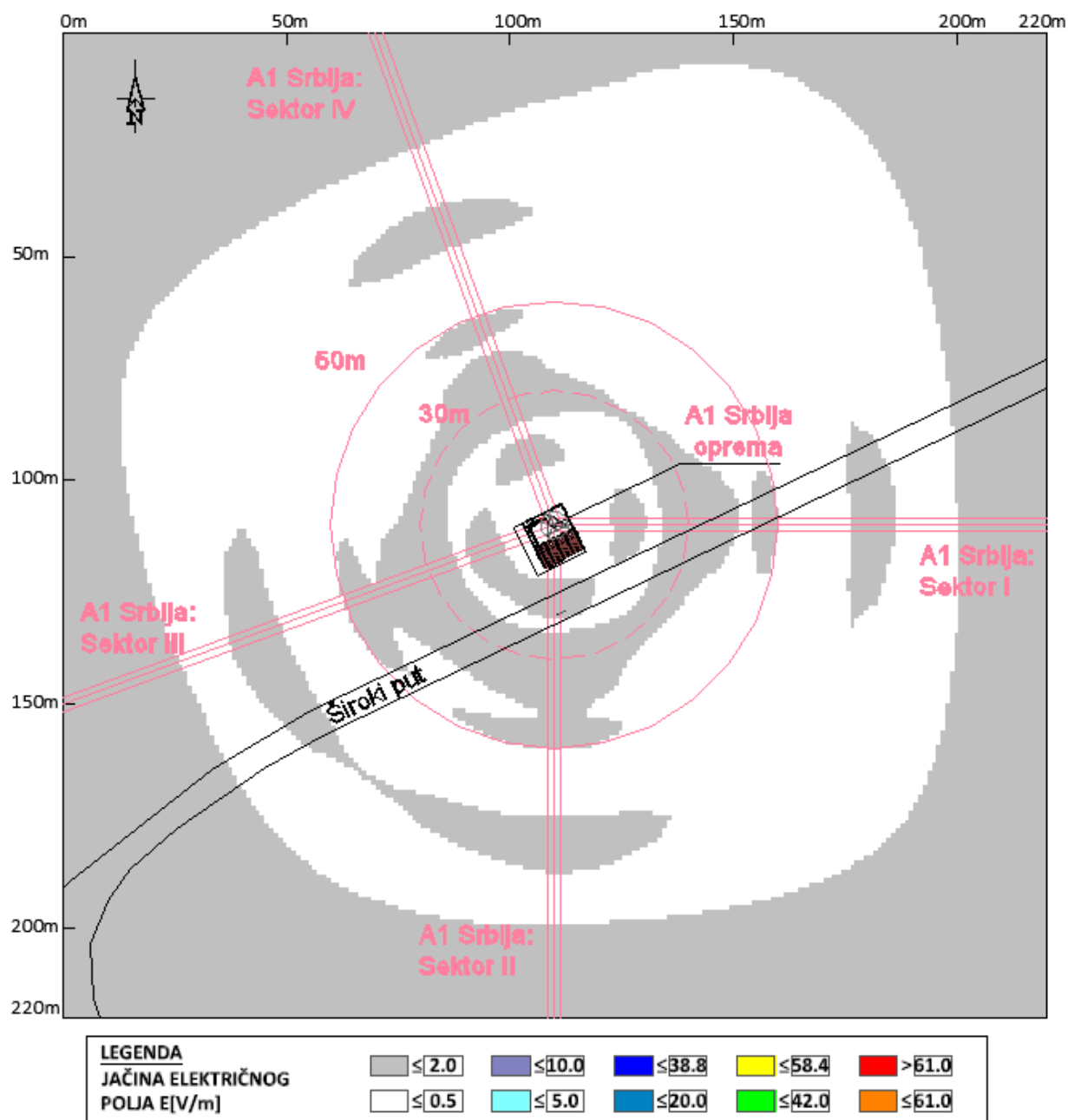
Slika 4.5 Rezultati proračuna jačine električnog polja u široj okolini lokacije bazne stanice na javnom području, na visini +1.70m (prosečna visina čoveka) u odnosu na nivo tla za slučaj rada sistema GSM900, LTE1800, LTE800 i LTE2100 operatora A1 Srbija . Maksimalna proračunata vrednost jačine električnog polja iznosi E=1.79 V/m .
