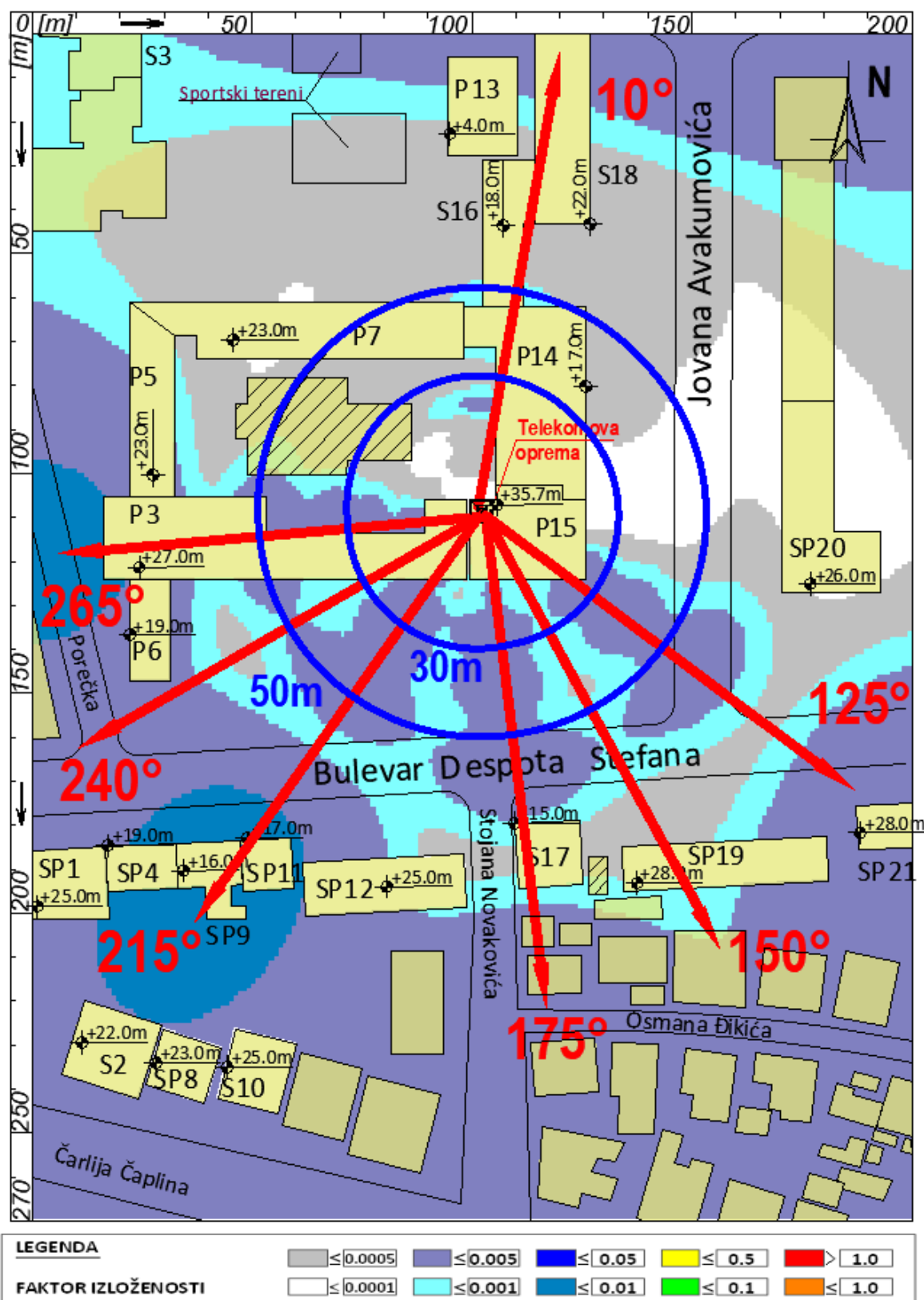
Slika 4.15 Rezultati proračuna faktora izloženosti u široj okolini lokacije bazne stanice na javnom području, na visini +1.70m (prosečna visina čoveka) u odnosu na nivo tla za slučaj rada sistema GSM900, UMTS2100, LTE1800, LTE800 i LTE2100 operatora Telekom Srbija . Maksimalna proračunata vrednost faktora izloženosti iznosi FI=0.0075 .
