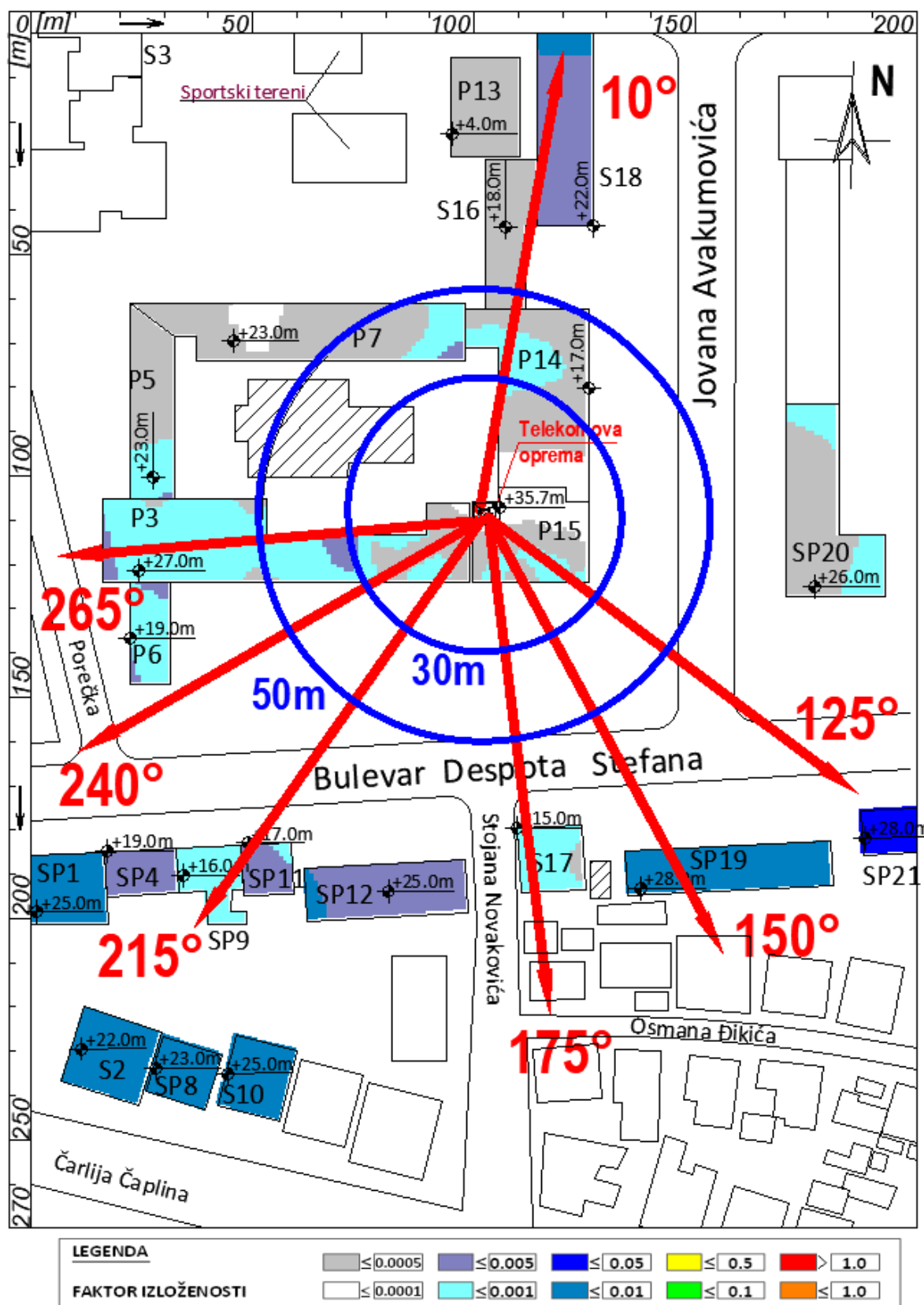
Slika 4.7 Rezultati proračuna faktora izloženosti za slučaj rada svih sistema na lokaciji GSM900, UMTS2100, LTE1800, LTE800 i LTE2100 operatora Telekom Srbija , u zonama povećane osetljivosti
