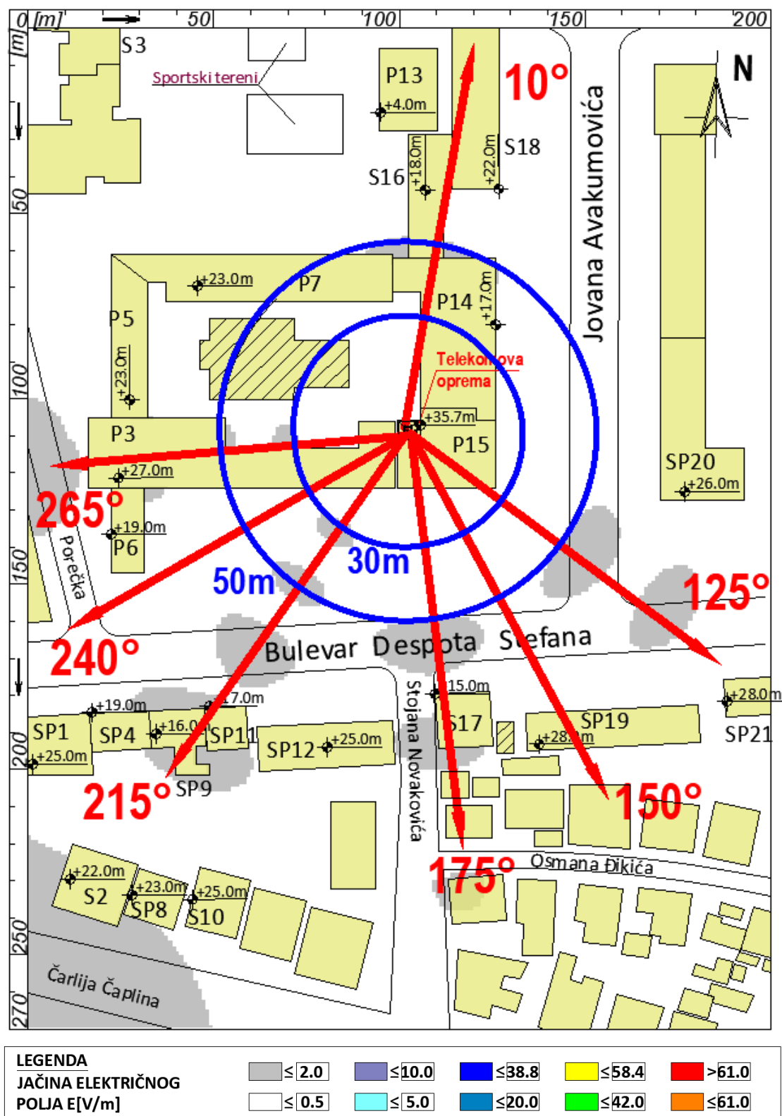
Slika 4.10 Rezultati proračuna jačine električnog polja u široj okolini lokacije bazne stanice na javnom području, na visini +1.70m (prosečna visina čoveka) u odnosu na nivo tla za slučaj rada sistema UMTS2100 operatora Telekom Srbija .
