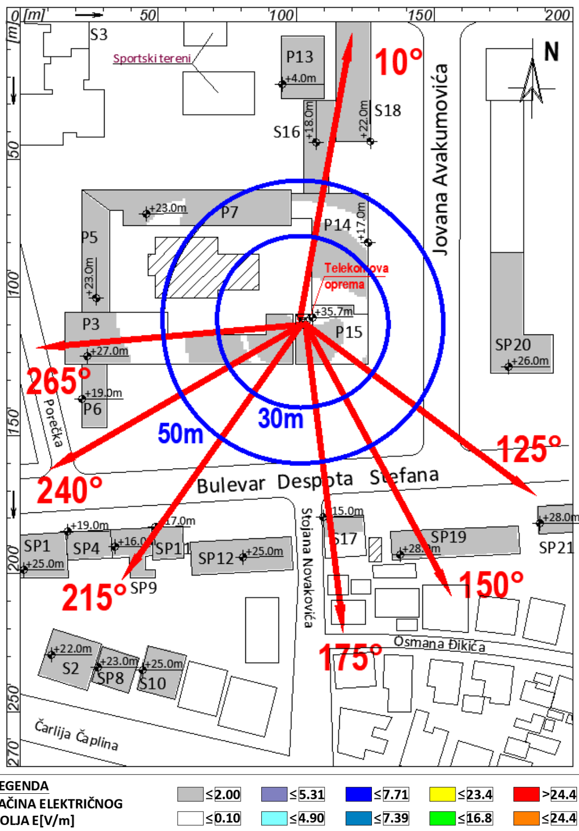
Slika 4.4 Rezultati proračuna jačine električnog polja sistema LTE800 operatora Telekom Srbija , u zonama povećane osetljivosti
