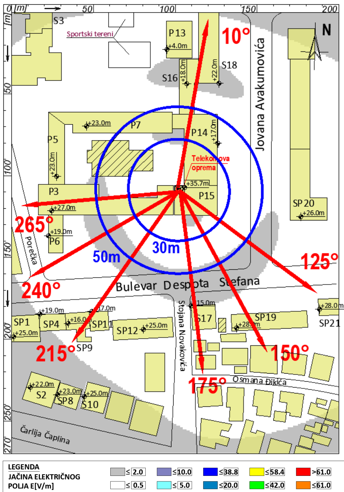
Slika 4.12 Rezultati proračuna jačine električnog polja u široj okolini lokacije bazne stanice na javnom području, na visini +1.70m (prosečna visina čoveka) u odnosu na nivo tla za slučaj rada sistema LTE800 operatora Telekom Srbija .
