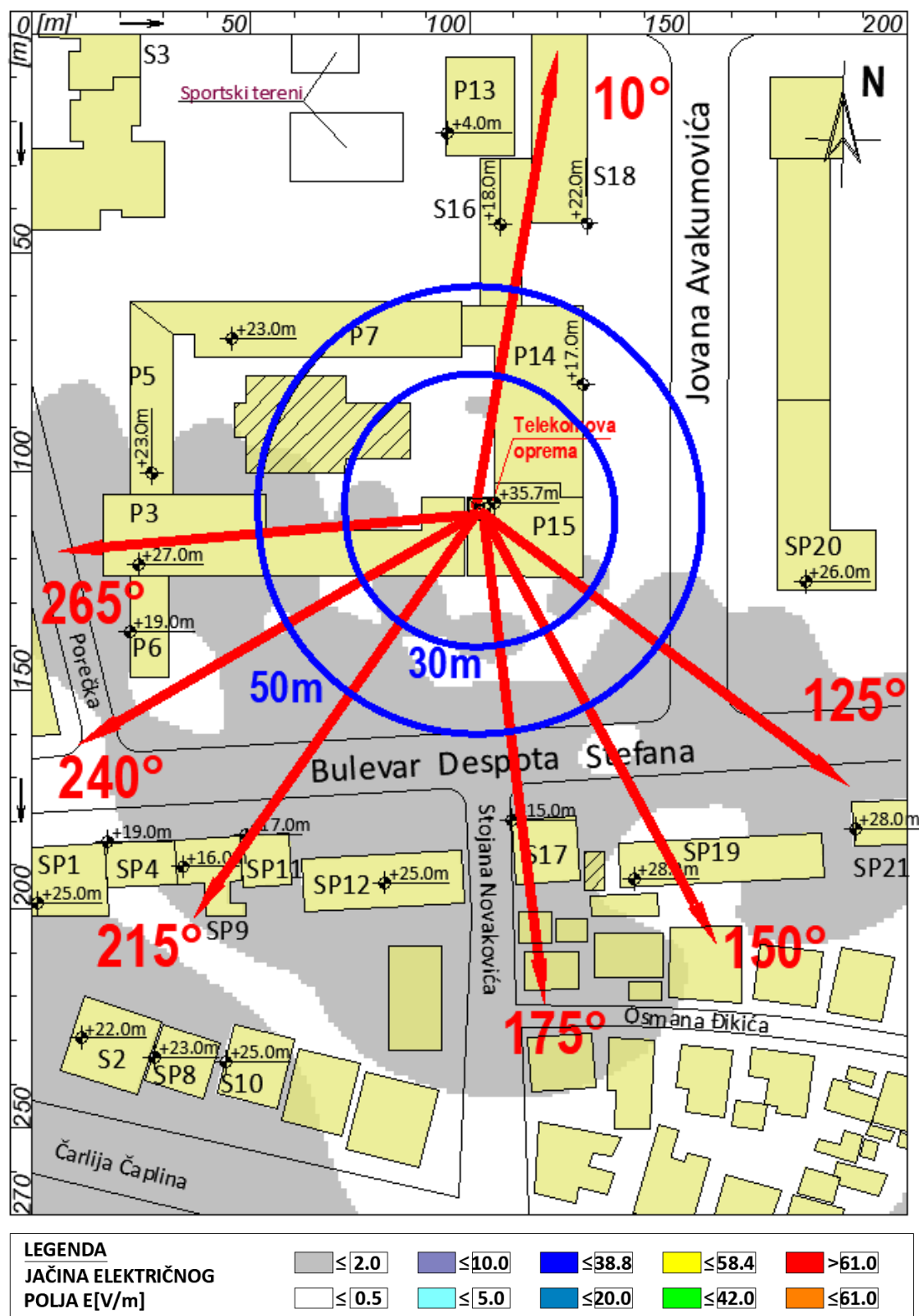
Slika 4.11 Rezultati proračuna jačine električnog polja u široj okolini lokacije bazne stanice na javnom području , na visini +1.70m (prosečna visina čoveka) u odnosu na nivo tla za slučaj rada sistema LTE1800 operatora Telekom Srbija .
