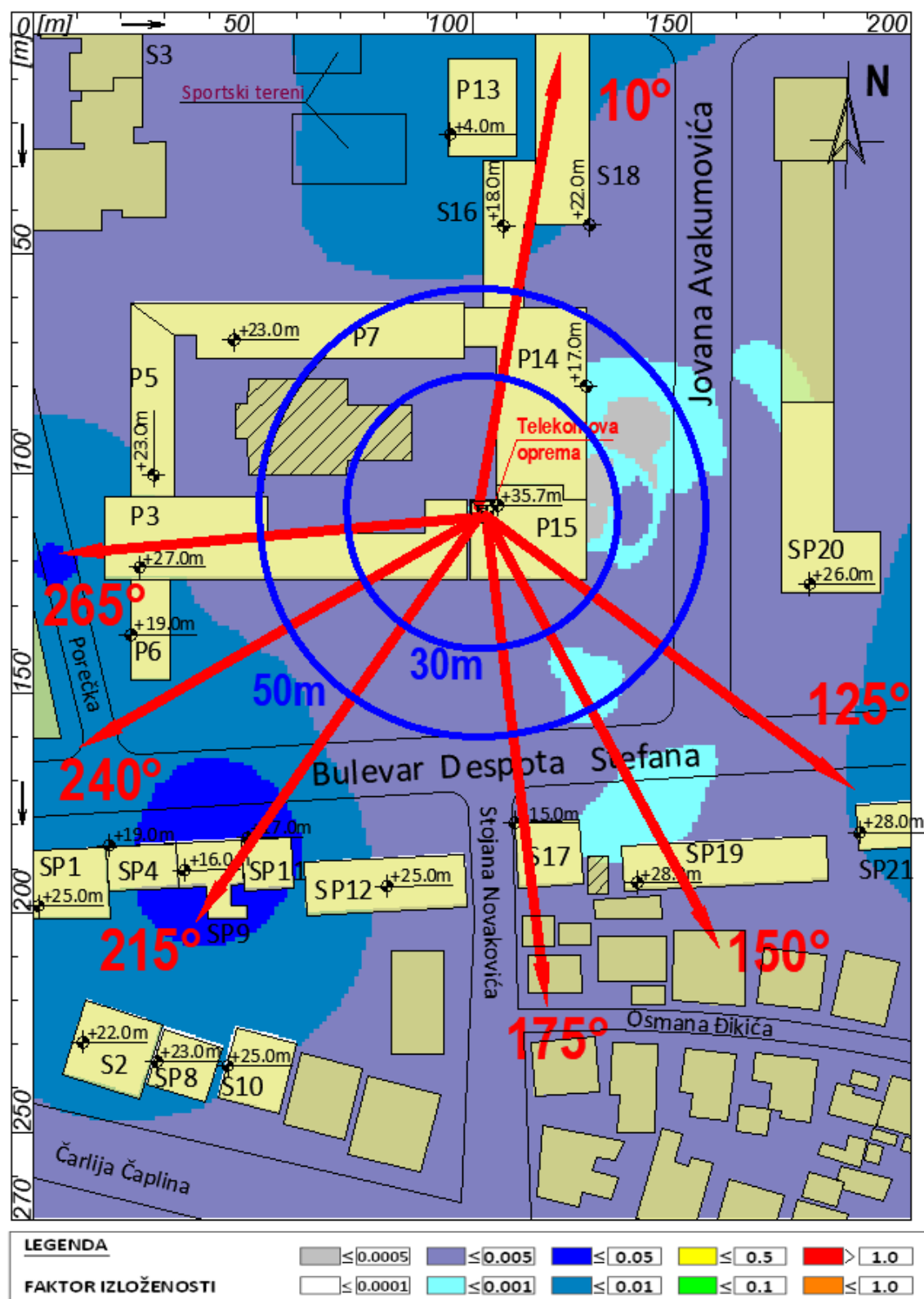
Slika 4.16 Rezultati proračuna faktora izloženosti u široj okolini lokacije bazne stanice na javnom području, na visini +1.70m (prosečna visina čoveka) u odnosu na nivo tla za slučaj rada sistema GSM900, UMTS2100, LTE1800, LTE800 i LTE2100 operatora Telekom Srbija i postojećih sistema operatora A1 Srbija .
