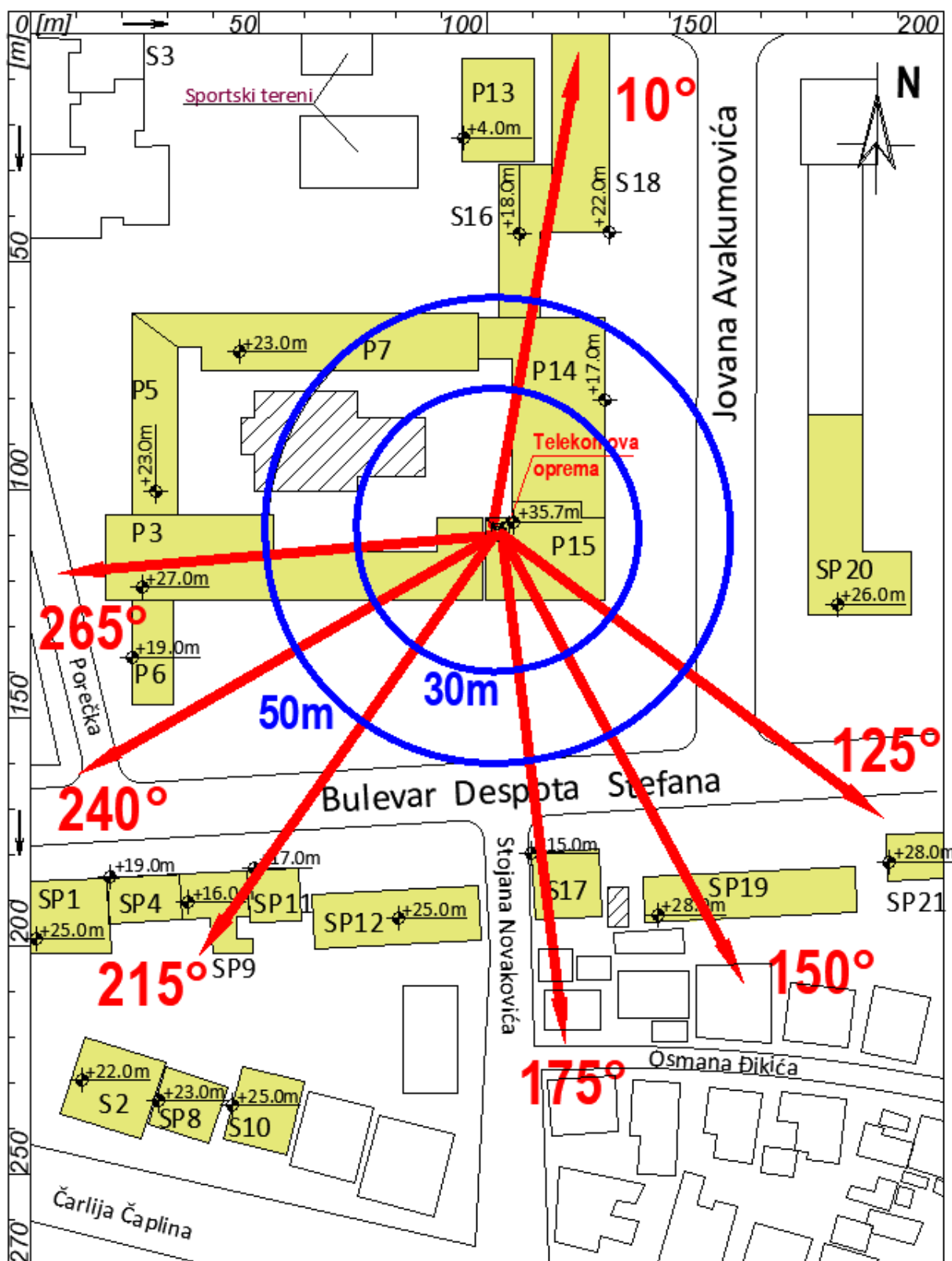
Slika 2.5 Dijagram objekata u okruženju radio bazne stanice „BG-29. novembra MUP“ - BG211/BGU211/BGL211/BGO211/BGJ211
