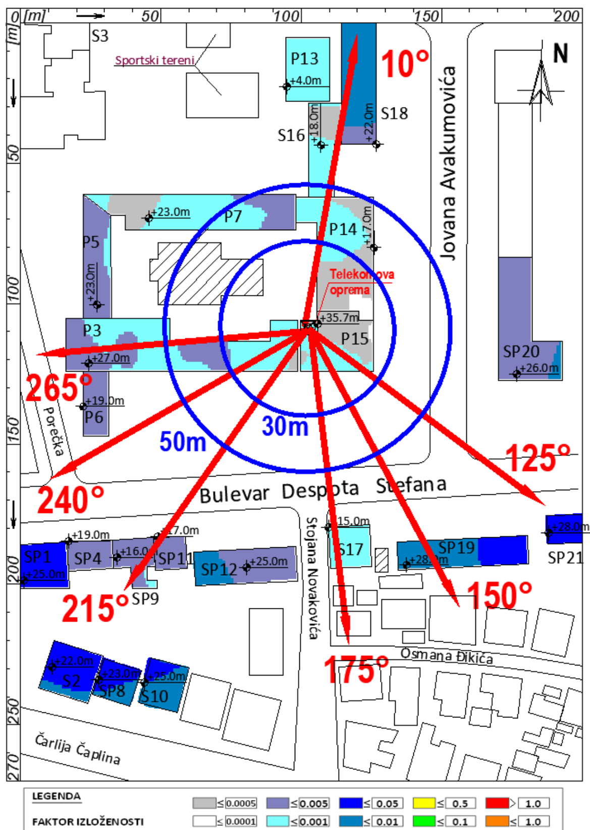
Slika 4.8 Rezultati proračuna faktora izloženosti za slučaj rada svih sistema na lokaciji GSM900, UMTS2100, LTE1800, LTE800 i LTE2100 operatora Telekom Srbija i postojećih sistema operatora A1 Srbija , u zonama povećane osetljivosti
