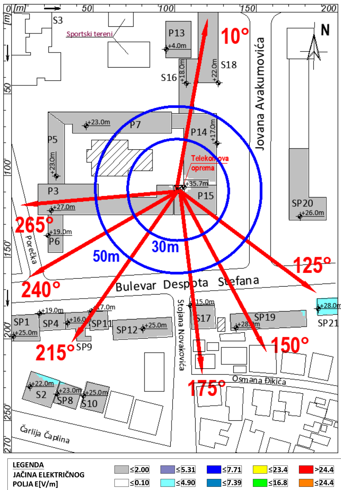
Slika 4.6 Rezultati proračuna jačine električnog polja za slučaj rada svih sistema na lokaciji GSM900, UMTS2100, LTE1800, LTE800 i LTE2100 operatora Telekom Srbija , u zonama povećane osetljivosti
