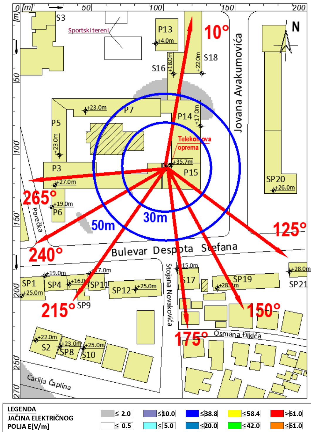
Slika 4.9 Rezultati proračuna jačine električnog polja u široj okolini lokacije bazne stanice na javnom području, na visini +1.70m (prosečna visina čoveka) u odnosu na nivo tla za slučaj rada sistema GSM900 operatora Telekom Srbija.
