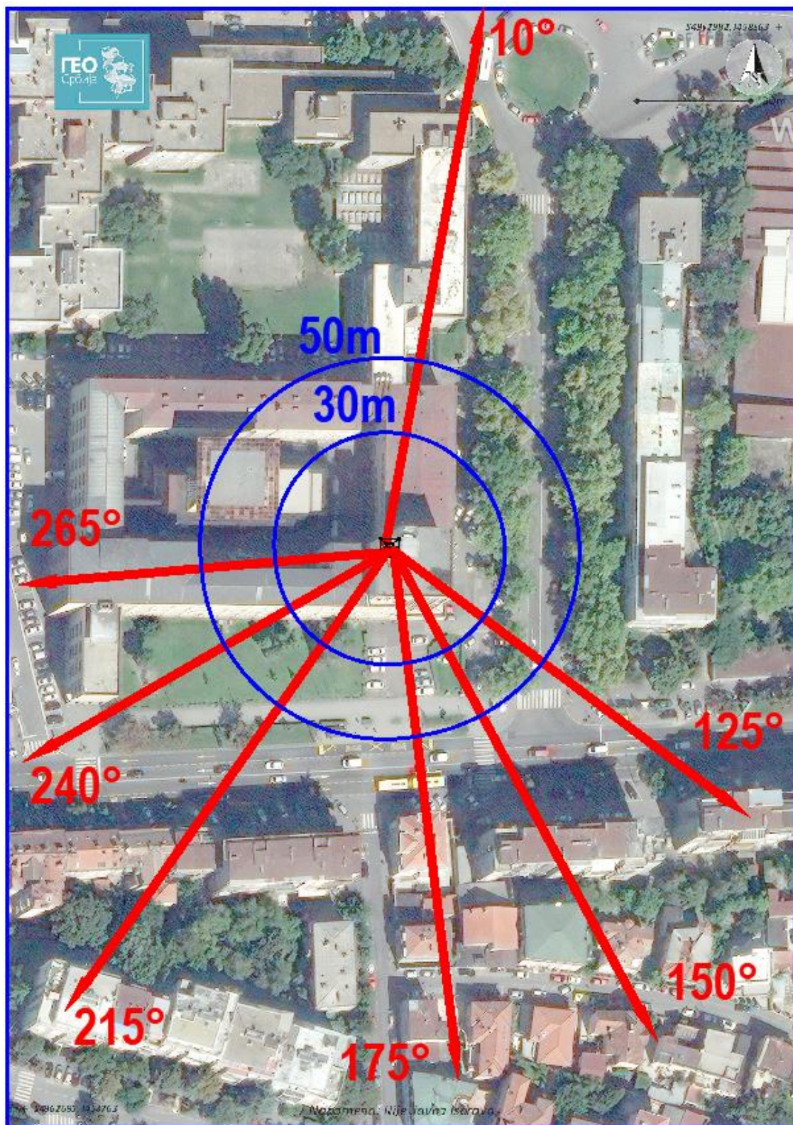
Slika 2.4 Dijagram zračenja predmetne radio bazne stanice „BG-29. novembra MUP“ - BG211/BGU211/BGL211/BGO211/BGJ211 3
