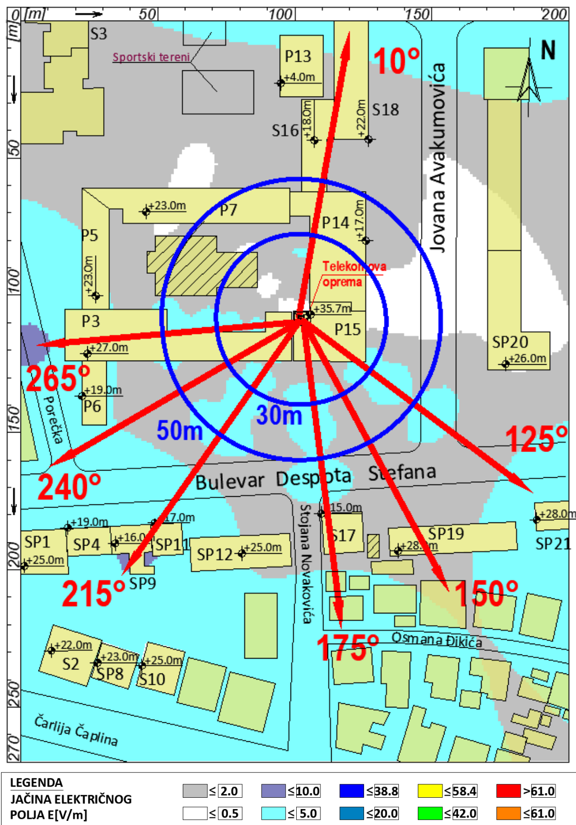
Slika 4.14 Rezultati proračuna jačine električnog polja u široj okolini lokacije bazne stanice na javnom području, na visini +1.70m (prosečna visina čoveka) u odnosu na nivo tla za slučaj rada sistema GSM900, UMTS2100, LTE1800, LTE800 i LTE2100 operatora Telekom Srbije . Maksimalna proračunata vrednost jačine električnog polja iznosi E= 5.17 V/m .
