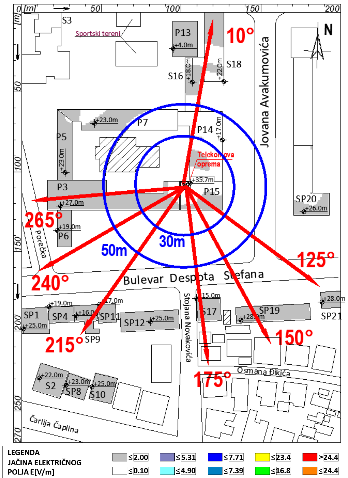
Slika 4.3 Rezultati proračuna jačine električnog polja sistema LTE1800 operatora Telekom Srbija , u zonama povećane osetljivosti
