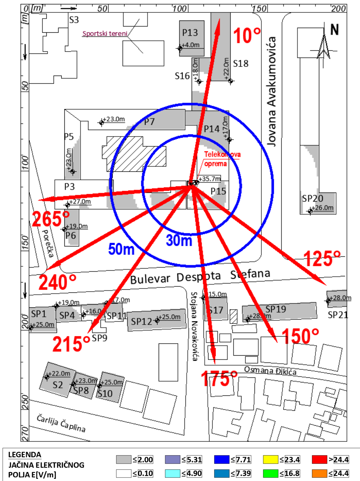
Slika 4.1 Rezultati proračuna jačine električnog polja sistema GSM900 operatora Telekom Srbija , u zonama povećane osetljivosti
