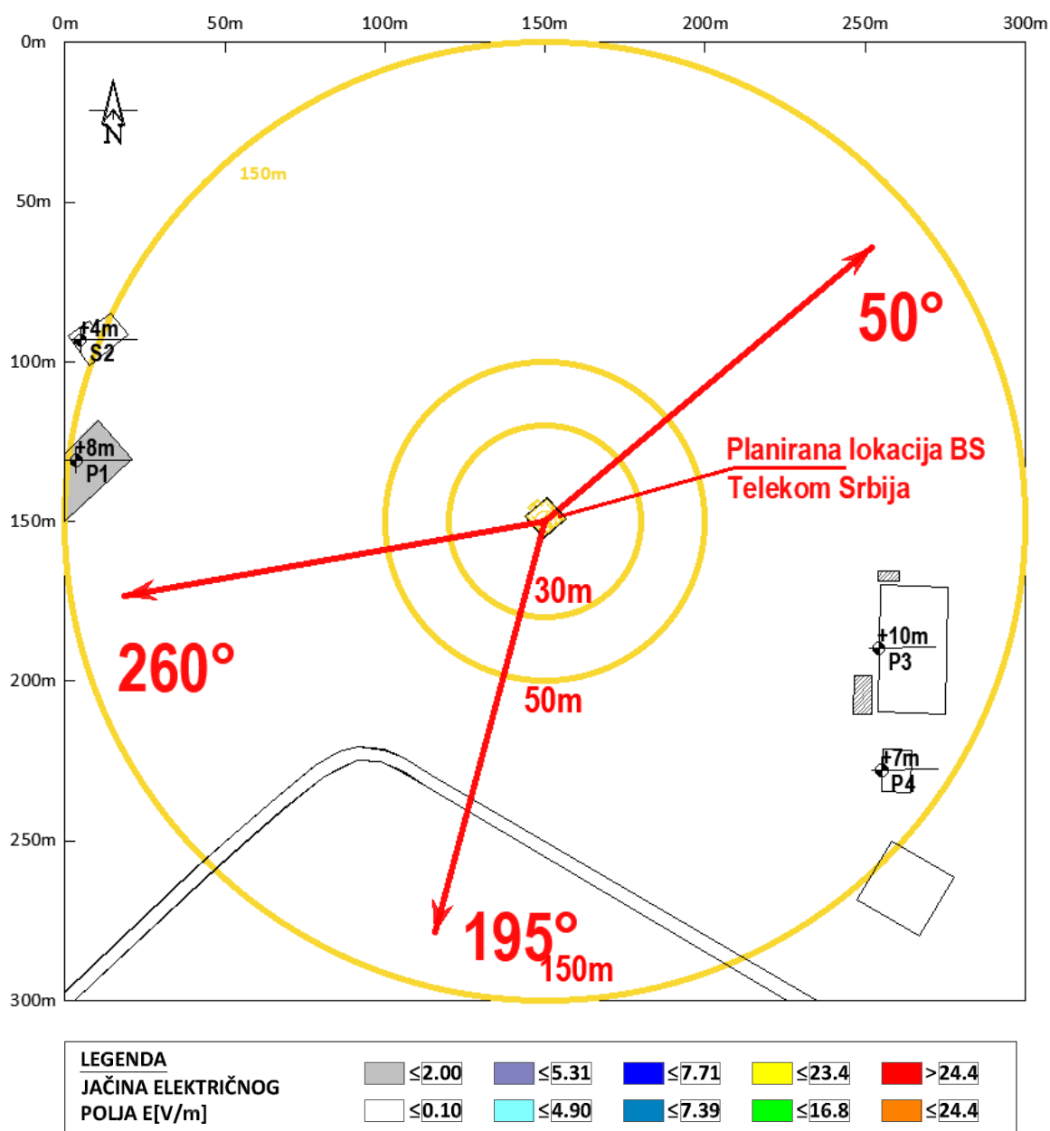
Slika 4.1 Rezultati proračuna jačine električnog polja sistema GSM900 operatora Telekom Srbija , u zonama povećane osetljivosti
