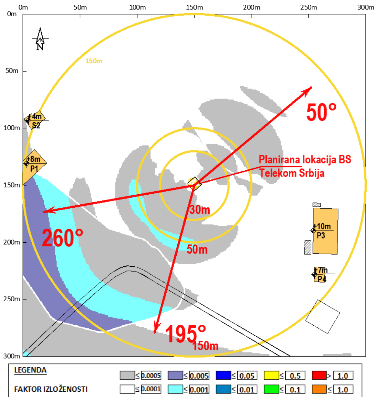
Slika 4.12 Rezultati proračuna faktora izloženosti u široj okolini lokacije bazne stanice na javnom području, na visini +1.70m (prosečna visina čoveka) u odnosu na nivo tla za slučaj rada sistema GSM900, LTE1800, LTE800 i LTE2100 operatora Telekom Srbija .
