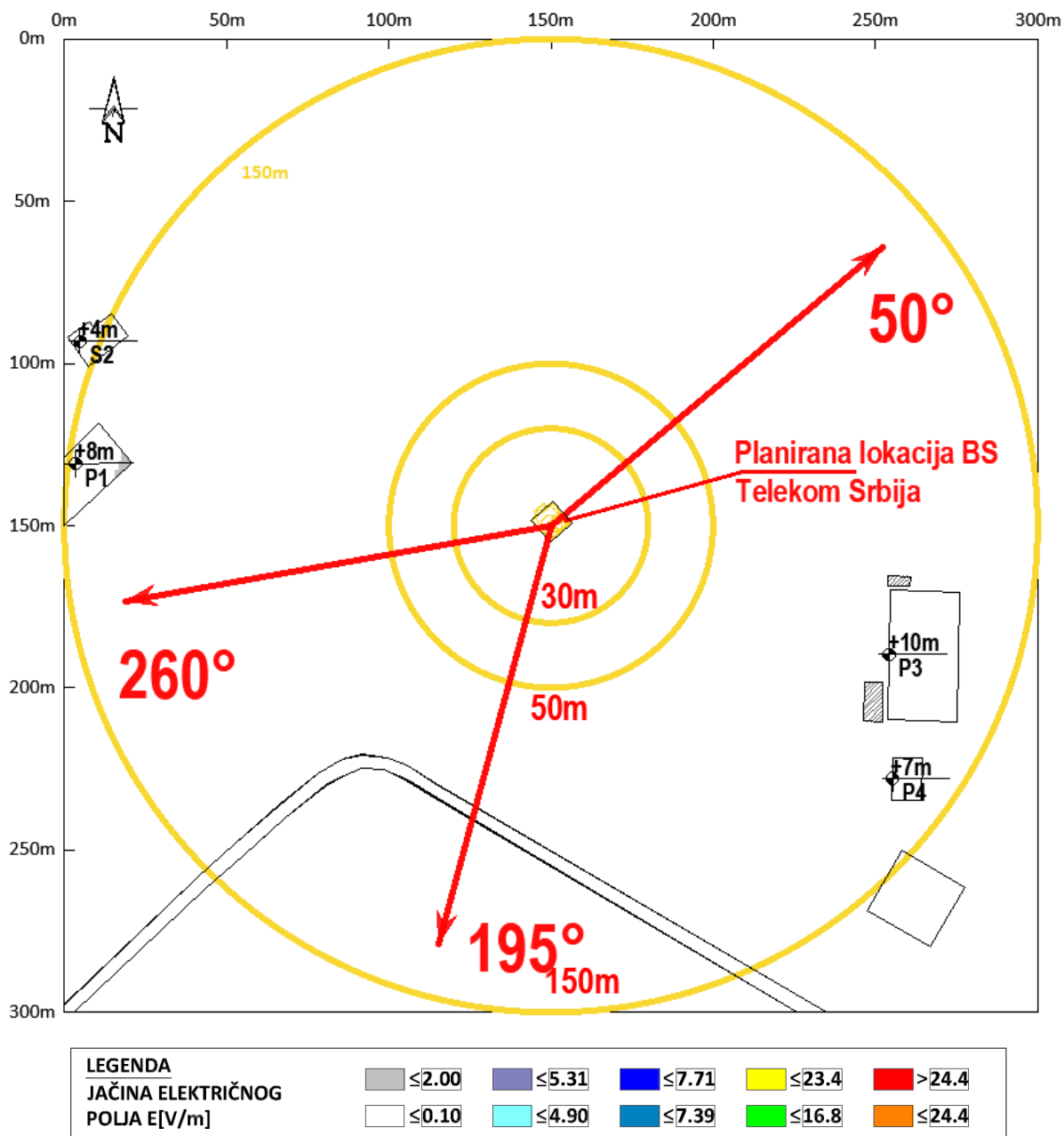
Slika 4.2 Rezultati proračuna jačine električnog polja sistema LTE1800 operatora Telekom Srbija , u zonama povećane osetljivosti
