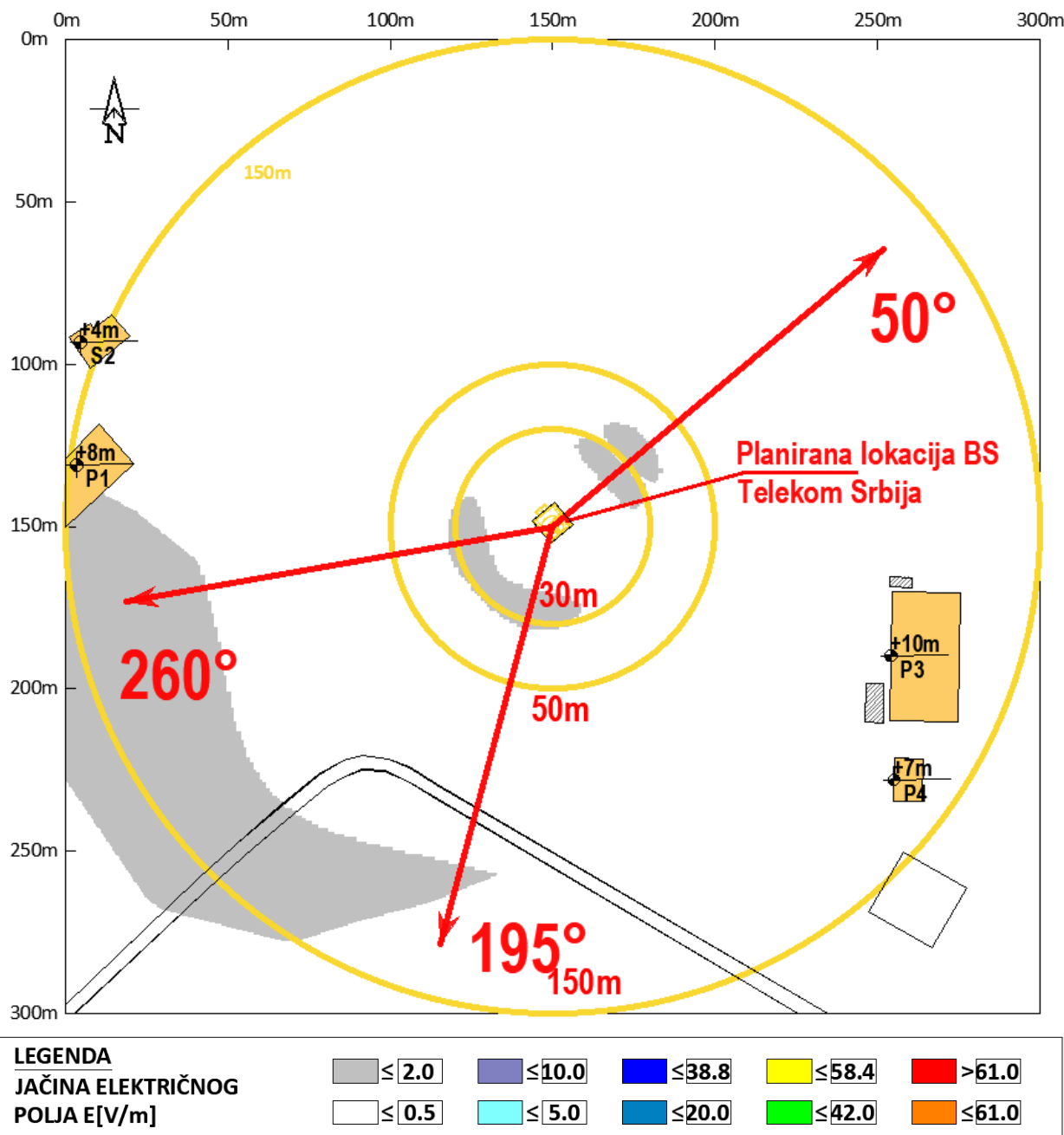
Slika 4.7 Rezultati proračuna jačine električnog polja u široj okolini lokacije bazne stanice na javnom području , na visini +1.70m (prosečna visina čoveka) u odnosu na nivo tla za slučaj rada sistema GSM900 operatora Telekom Srbija .
