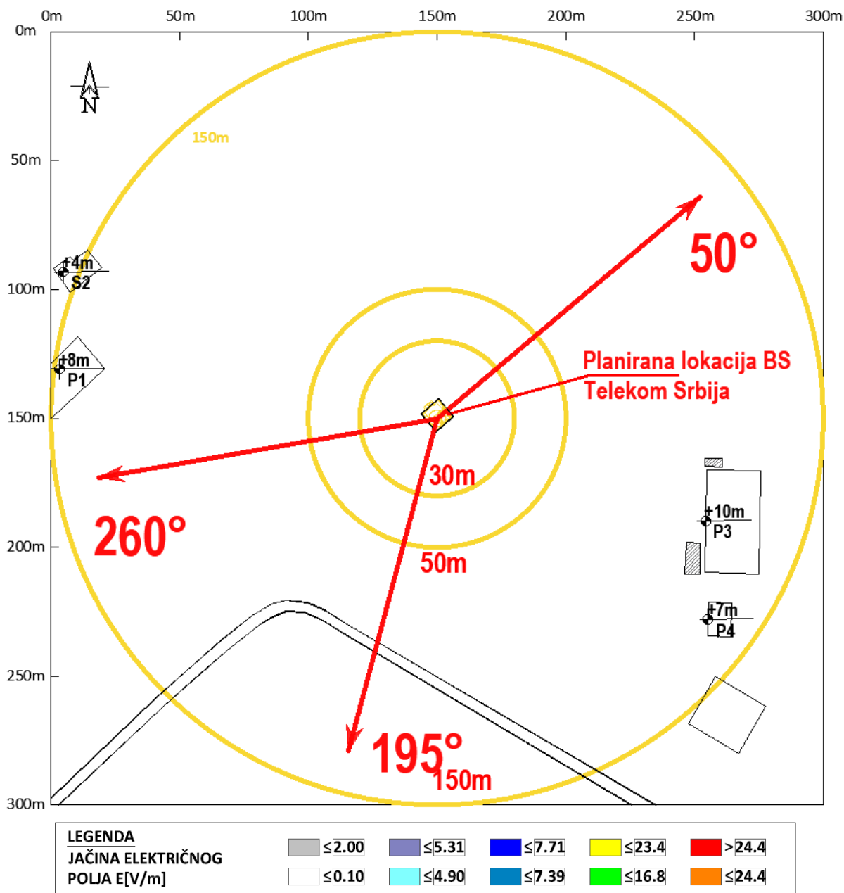
Slika 4.4 Rezultati proračuna jačine električnog polja sistema LTE2100 operatora Telekom Srbija, u zonama povećane osetljivosti
