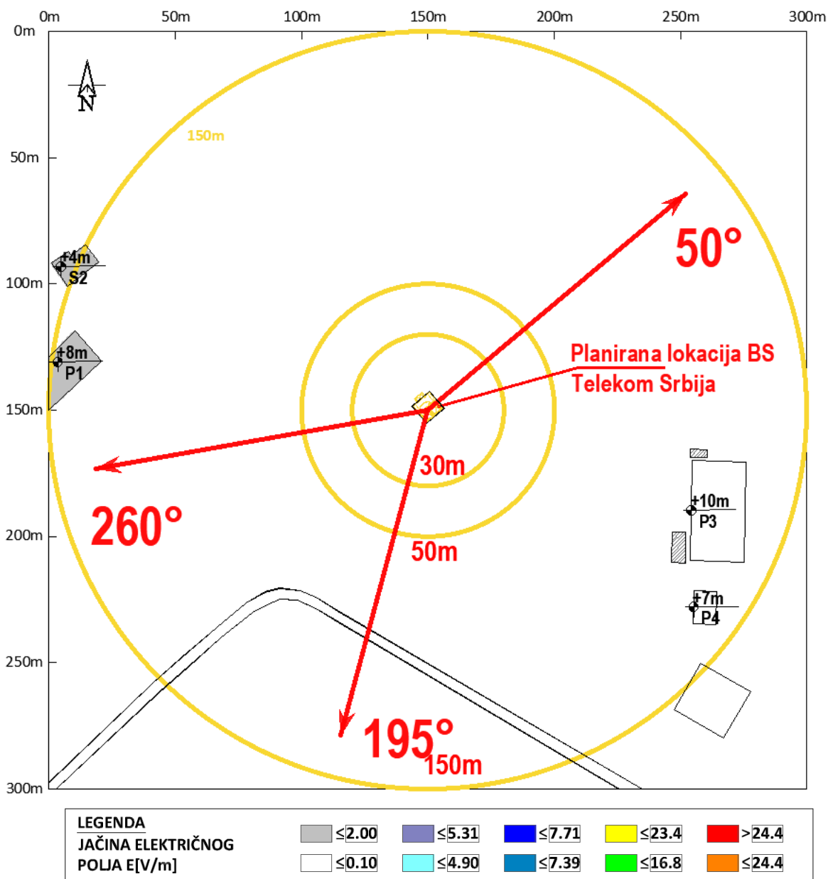
Slika 4.5 Rezultati proračuna jačine električnog polja za slučaj rada svih planiranih sistema na lokaciji- GSM900, LTE1800, LTE800 i LTE2100 operatora Telekom Srbija , u zonama povećane osetljivosti
