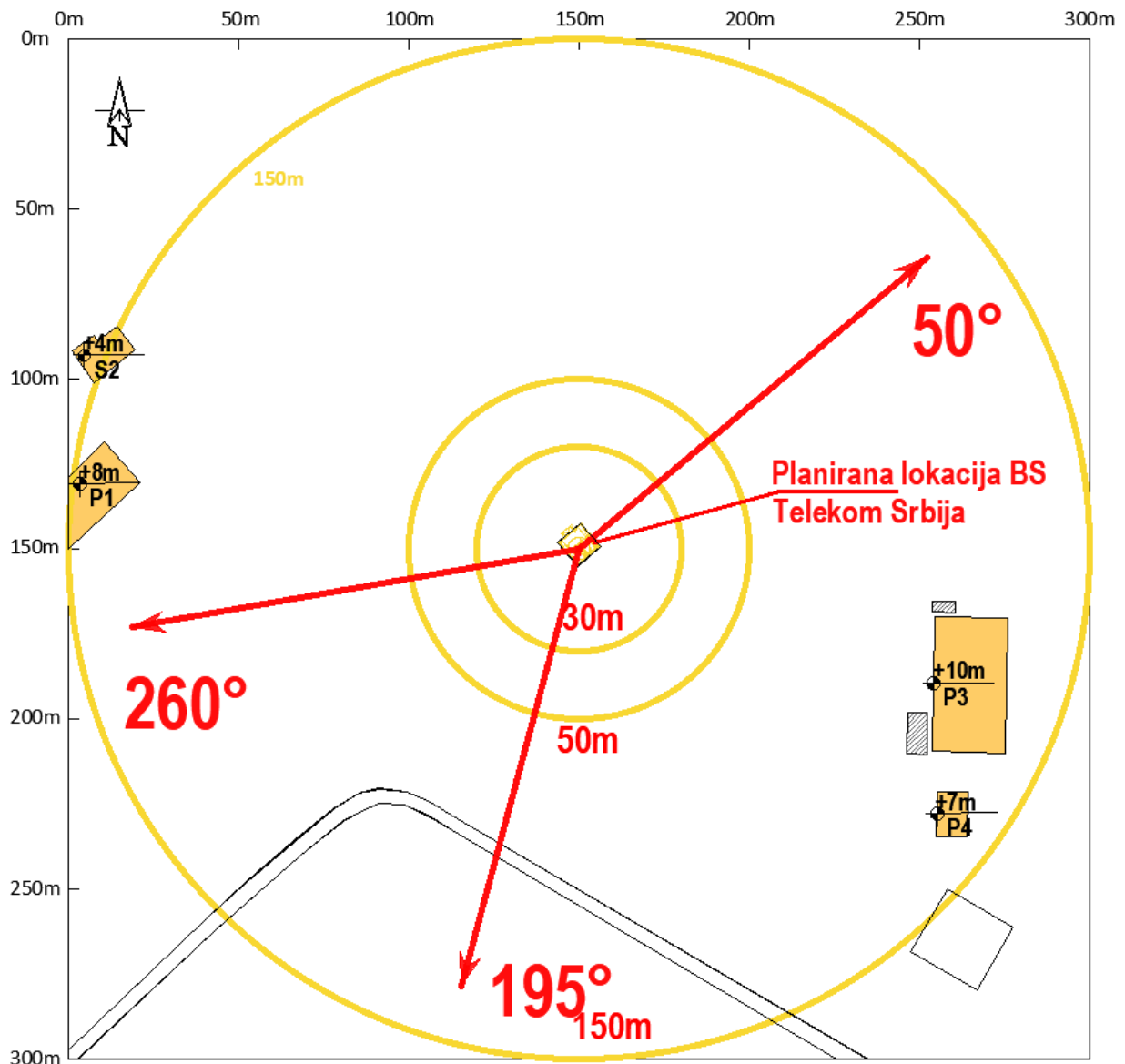
Slika 2.5 Dijagram objekata u okruženju radio bazne stanice "Guncati (CT)"- B1477/BL1477/BO1477/BJ1477
