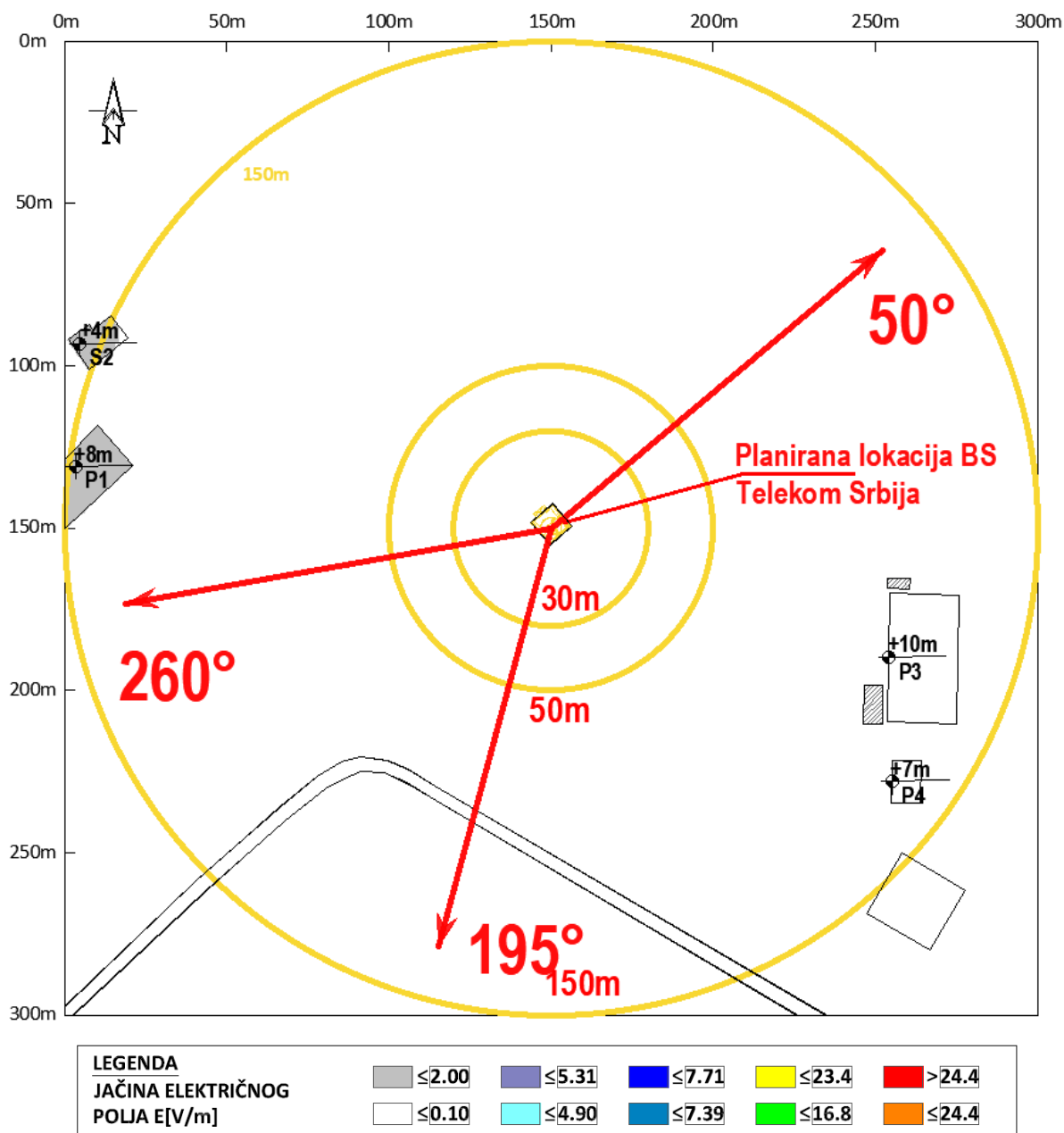
Slika 4.3 Rezultati proračuna jačine električnog polja sistema LTE800 operatora Telekom Srbija , u zonama povećane osetljivosti
