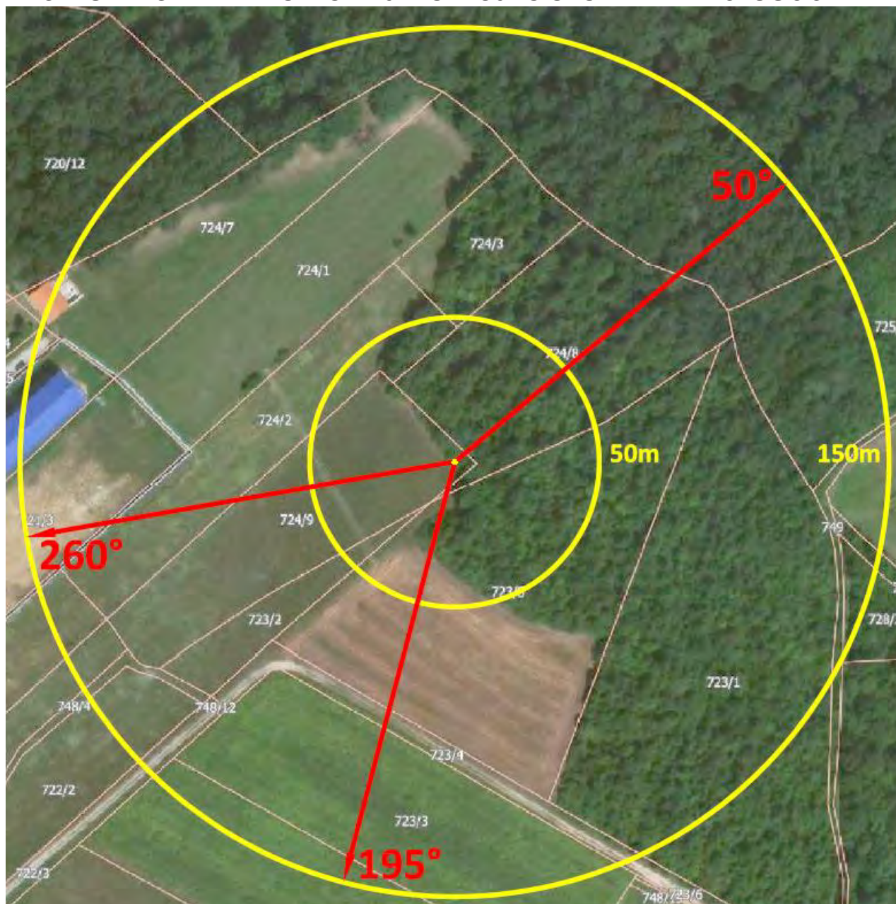
Slika 2.4 Dijagram zračenja planirane radio bazne stanice "Guncati (CT)"-B1477/BL1477/BO1477/BJ1477 ‡
