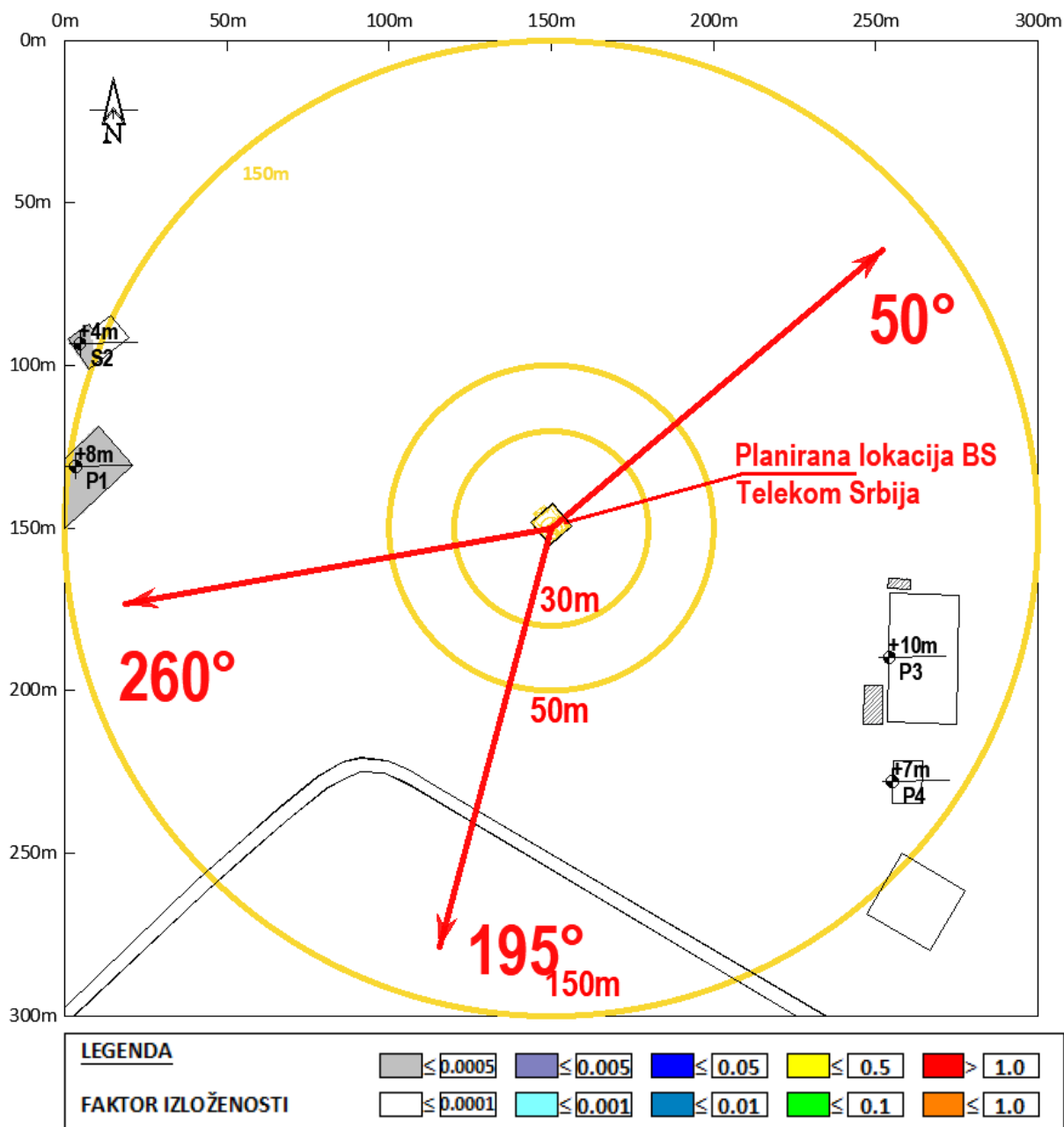
Slika 4.6 Rezultati proračuna faktora izloženosti za slučaj rada svih planiranih sistema na lokaciji- GSM900, LTE1800, LTE800 i LTE2100 operatora Telekom Srbija , u zonama povećane osetljivosti
