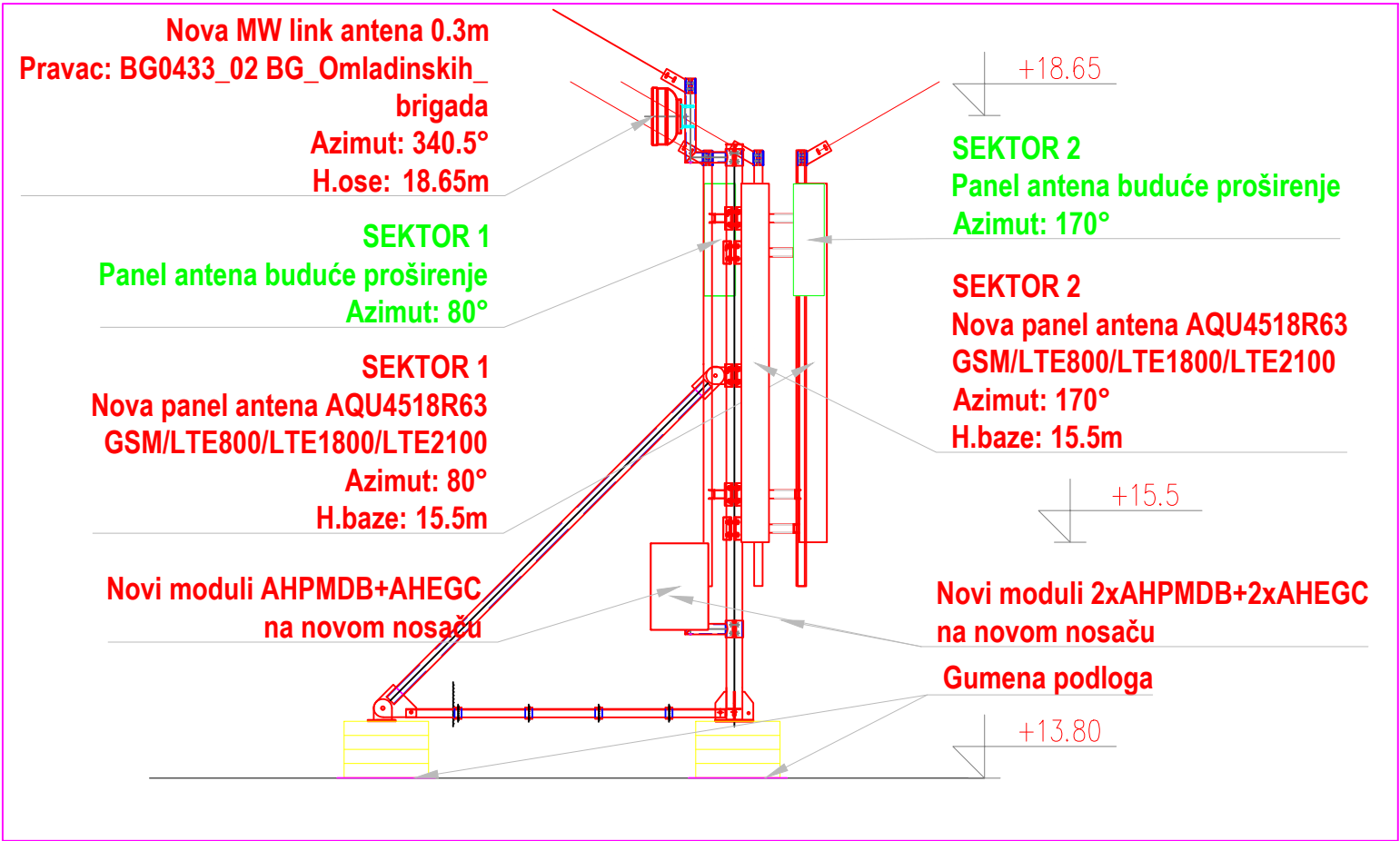
Pogled 1-1 Razmera: 1:50
