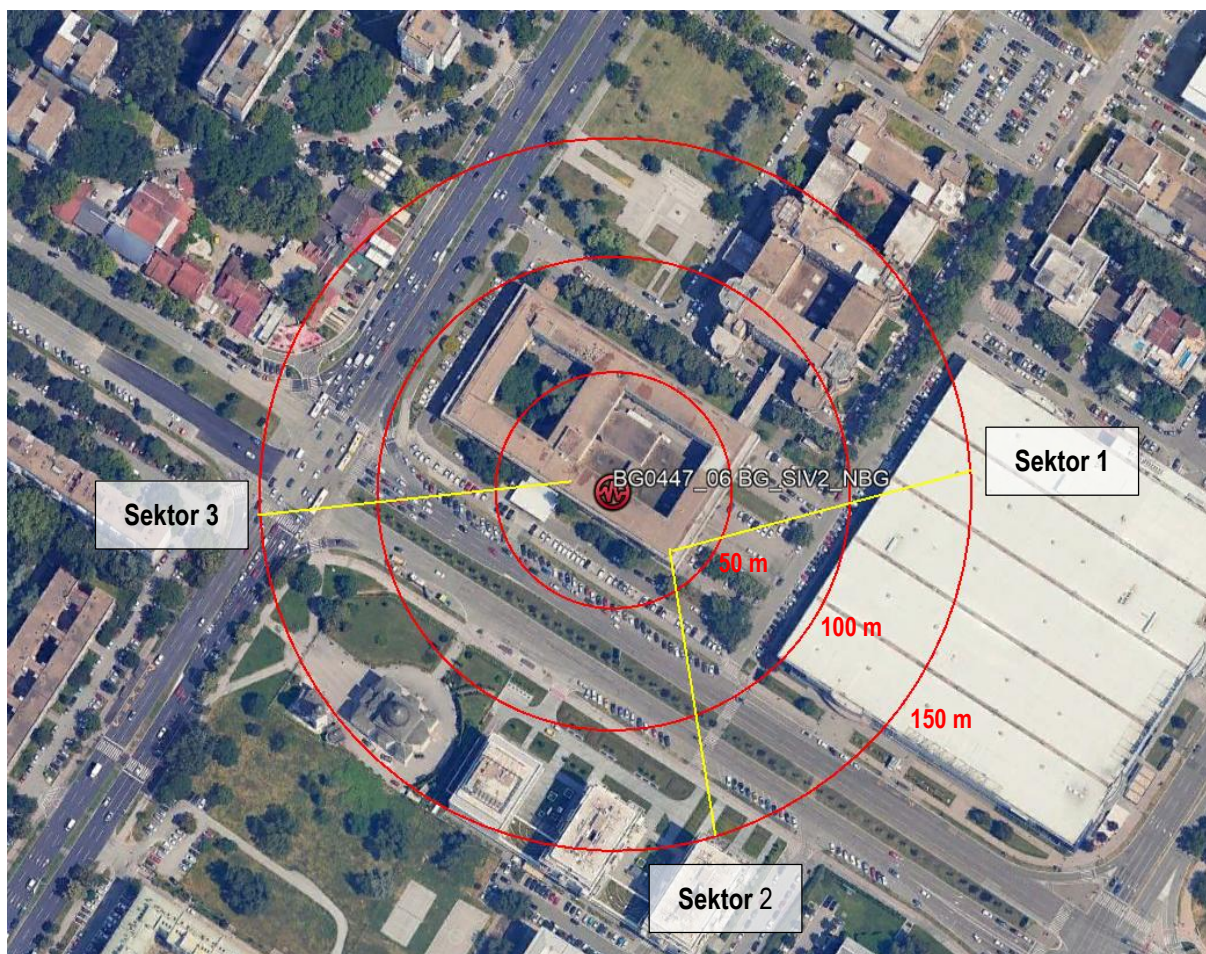
Slika 2.5 Pravci zračenja antenskog sistema predmetne bazne stanice
