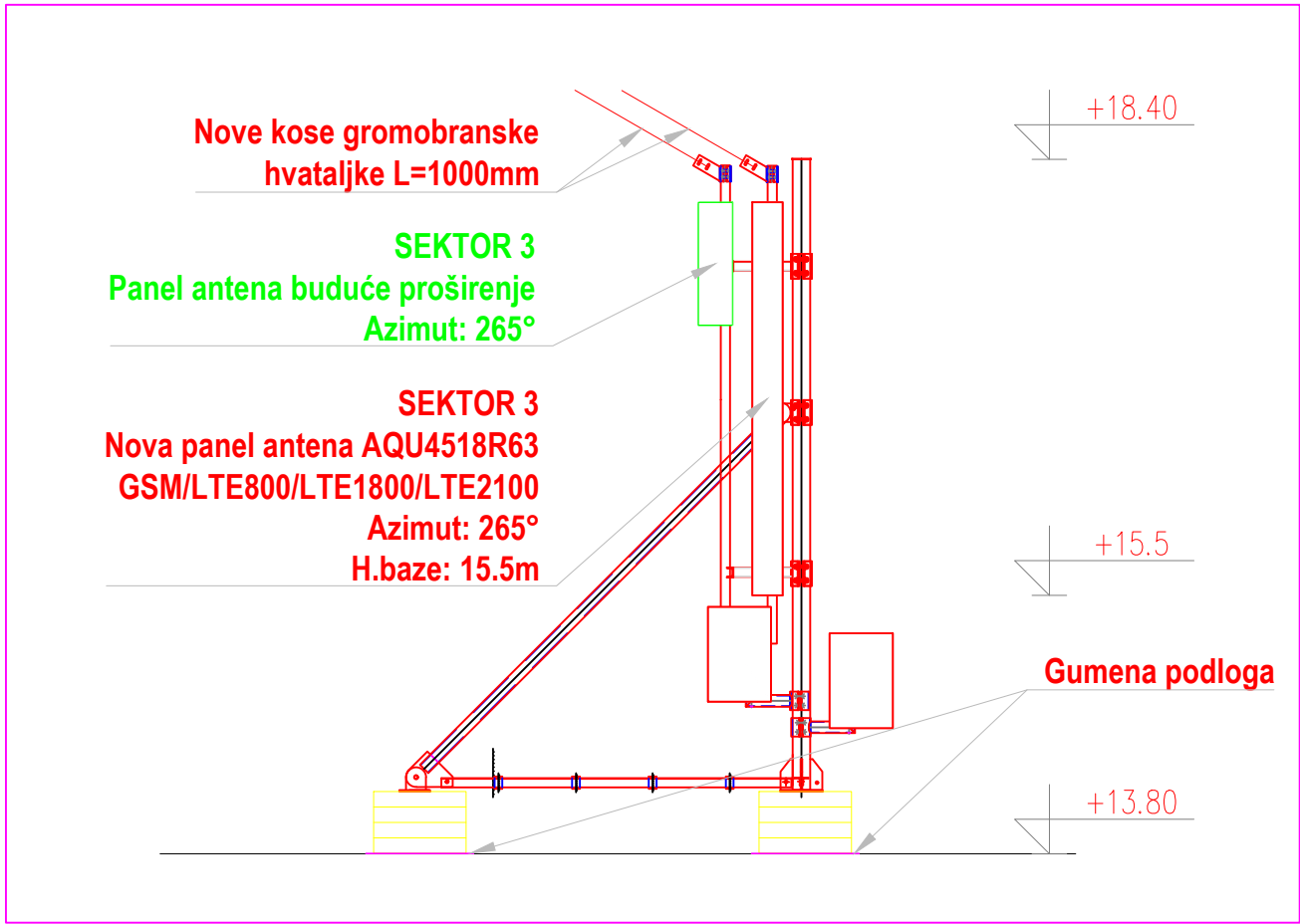
Pogled 2-2 Razmera: 1:50
