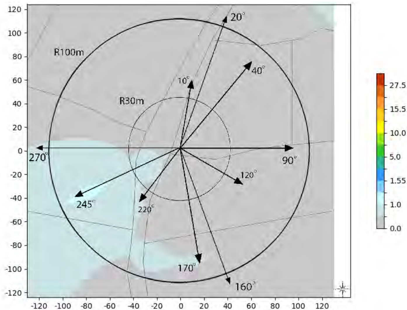
Slika 6.1. Rezultati proračuna jačine električnog polja na tlu, za slučaj kada LTE800 bazna stanica operatora MTS radi sa maks. kapacitetom.
