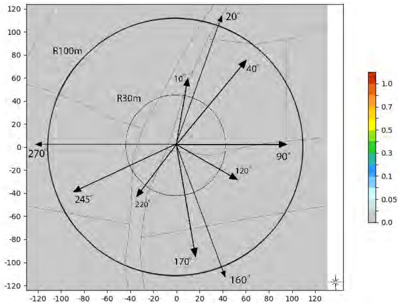
Slika 6.9. Rezultati proračuna jačine električnog polja na tlu, za slučaj kada sve stanice svih operatora rade sa maks. kapacitetom.
