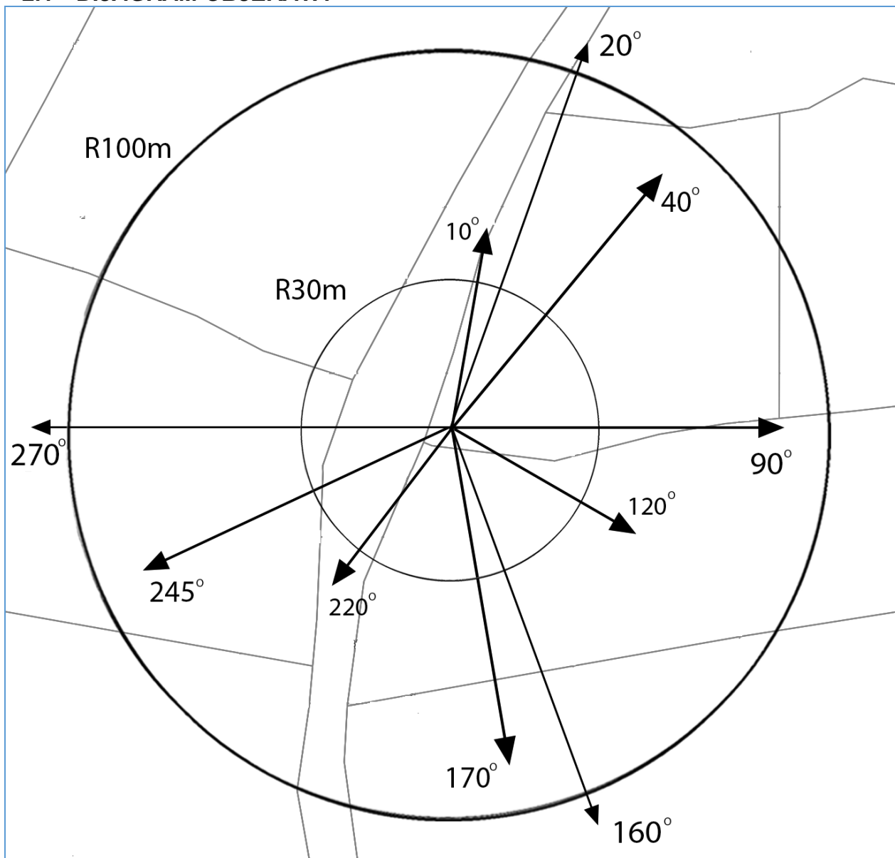
Slika 2.3 Dispozicija objekata u okruženju bazne stanice u krugu 100m od izvora Ucrtani su azimuti antena MTS 40°-90°-170°-245° Na istom stubu su i operateri A1 20°-160°-270°. i YETTEL 10°-120°-220°. Objekata u okruženju nema.
