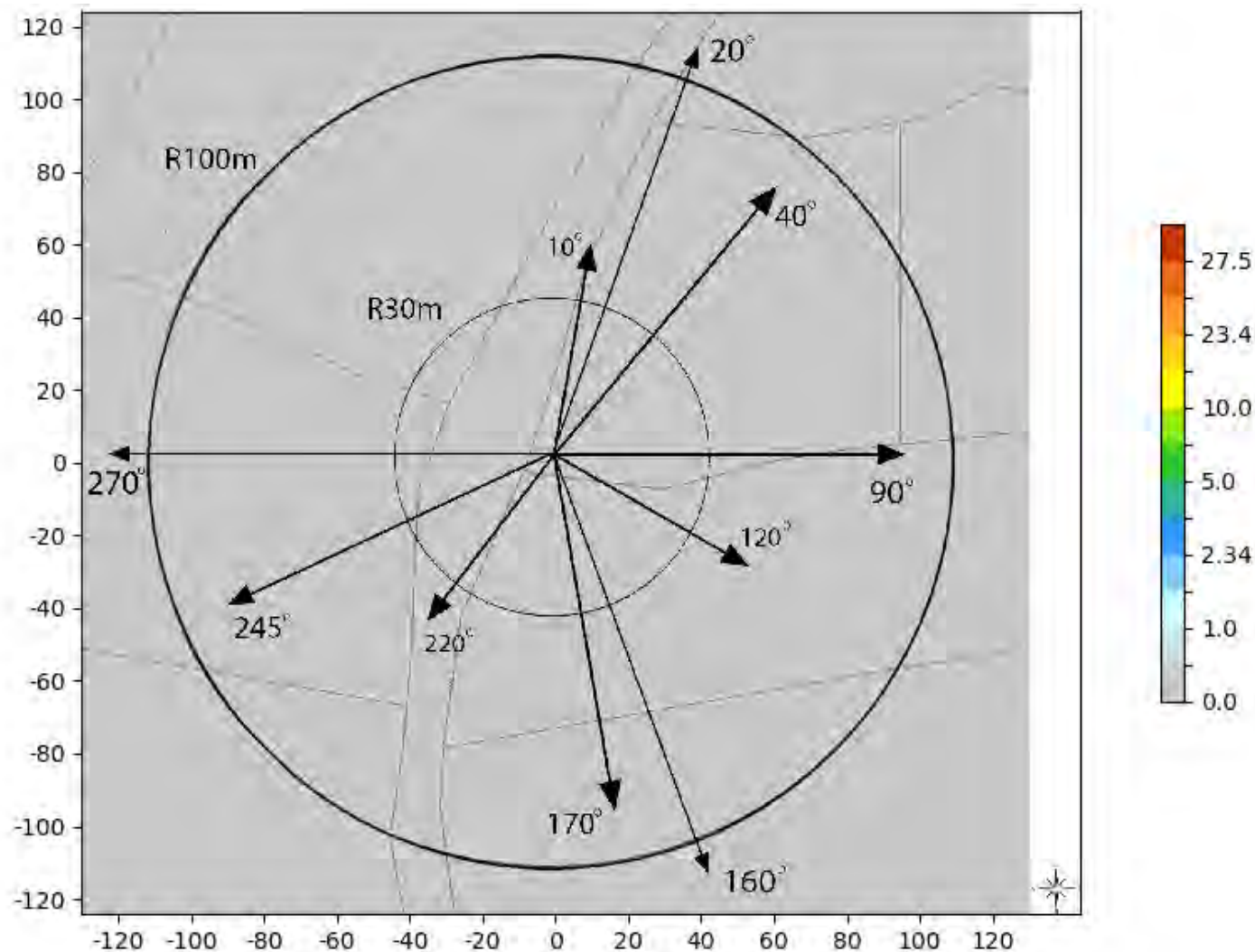
Slika 6.2. Rezultati proračuna jačine električnog polja na tlu, za slučaj kada LTE1800 bazna stanica operatora MTS radi sa maks. kapacitetom.
