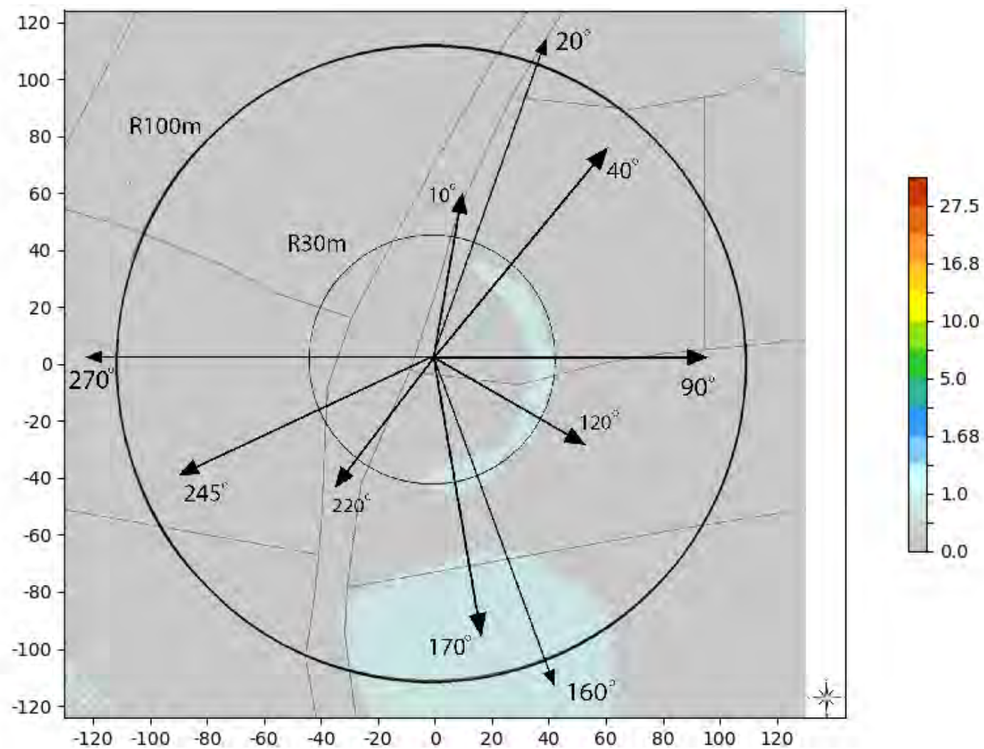
Slika 6.3. Rezultati proračuna jačine električnog polja na tlu, za slučaj kada GSM900 bazna stanica operatora MTS radi sa maks. kapacitetom.
