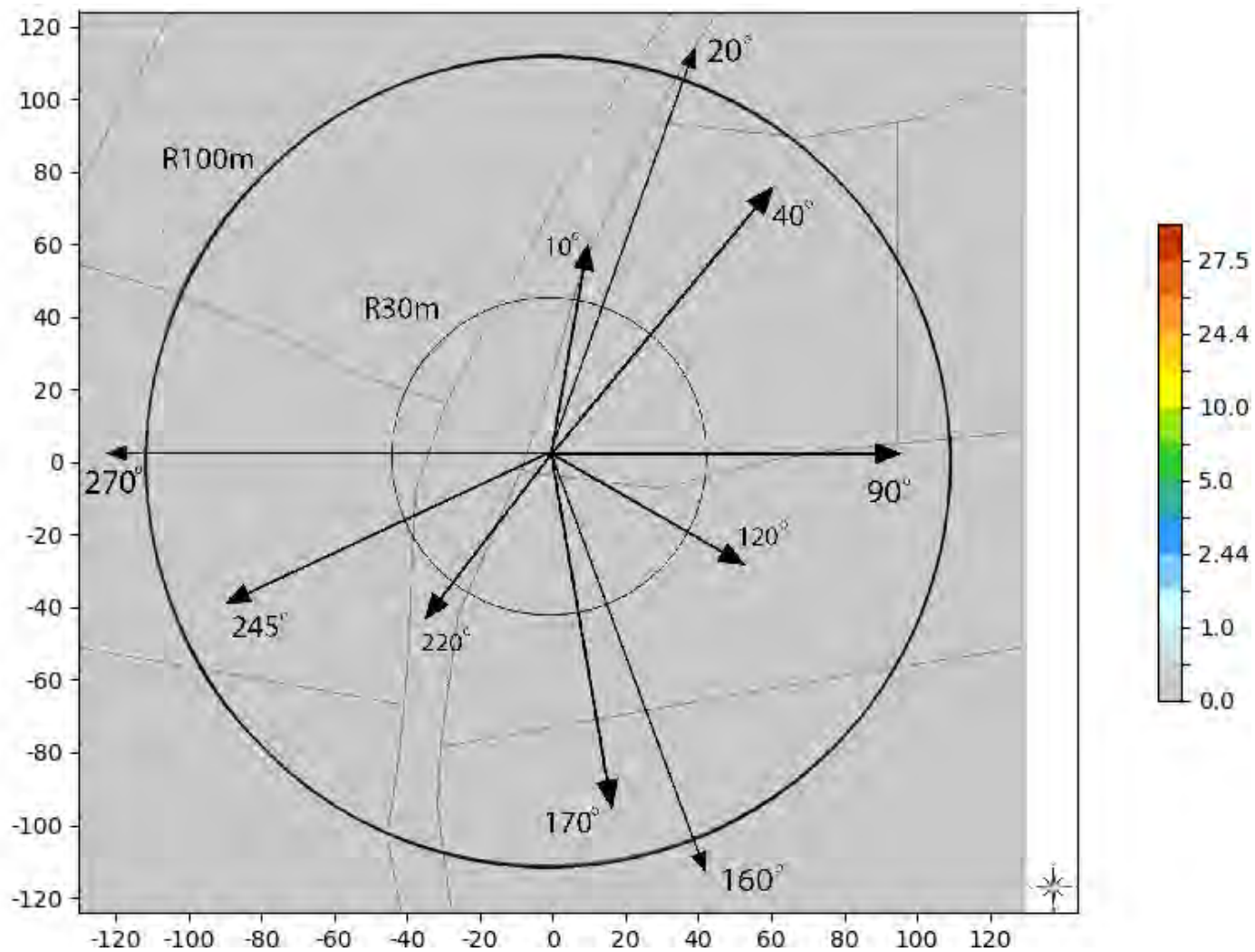
Slika 6.5. Rezultati proračuna jačine električnog polja na tlu, za slučaj kada UMTS2100 bazna stanica operatora MTS radi sa maks. kapacitetom.
