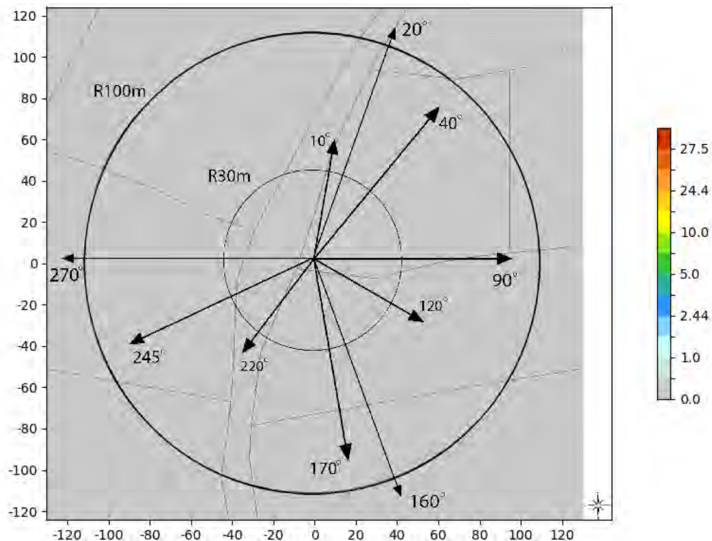
Slika 6.4. Rezultati proračuna jačine električnog polja na tlu, za slučaj kada LTE2100 bazna stanica operatora MTS radi sa maks. kapacitetom.
