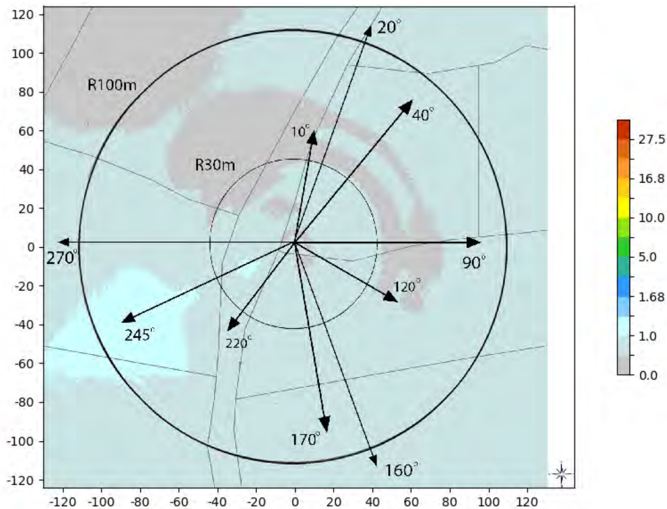
Slika 6.6. Rezultati proračuna jačine električnog polja na tlu, za slučaj kada sve stanice operatora MTS rade sa maks. kapacitetom.
