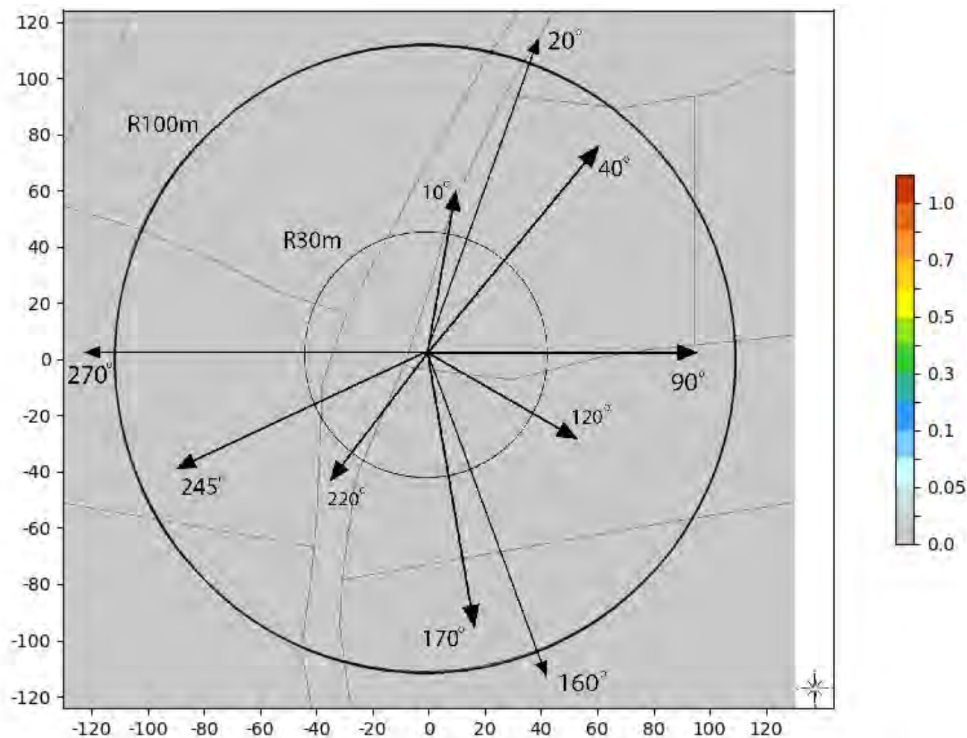
Slika 6.7. Rezultati proračuna faktora izlaganja na tlu, za slučaj kada svi sistemi operatora MTS na lokaciji rade sa maksimalnim kapacitetom
