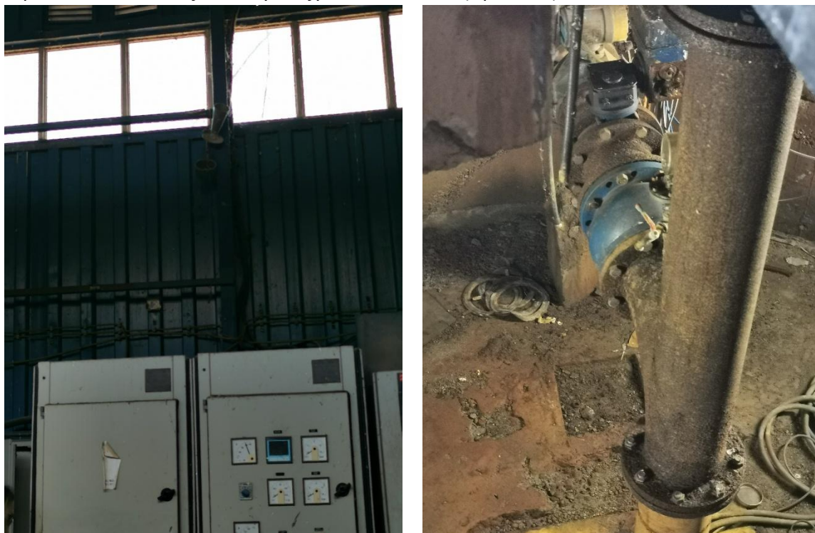
Слика 3. Рени бунар РБ-50, машинска сала и затварачница
