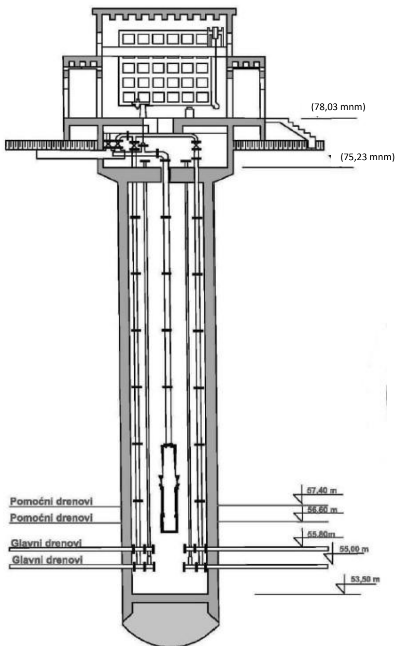
Слика 4. Шематски приказ бунара РБ-50 (Архив ЈКП. „Београдски водовод и канализација“).
