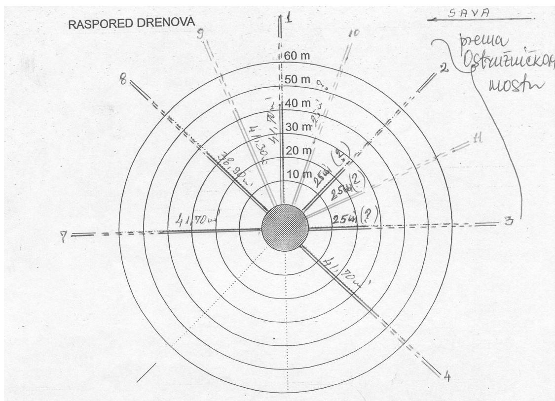
Слика 3 - Положај дренава бунара РБ-50 (Архив ЈКП „Београдски водовод и канализација“)
