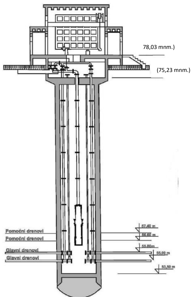
Слика 5 – Шематски приказ шахта бунара РБ-50 (Архив ЈКП „Београдски водовод и канализација“)
