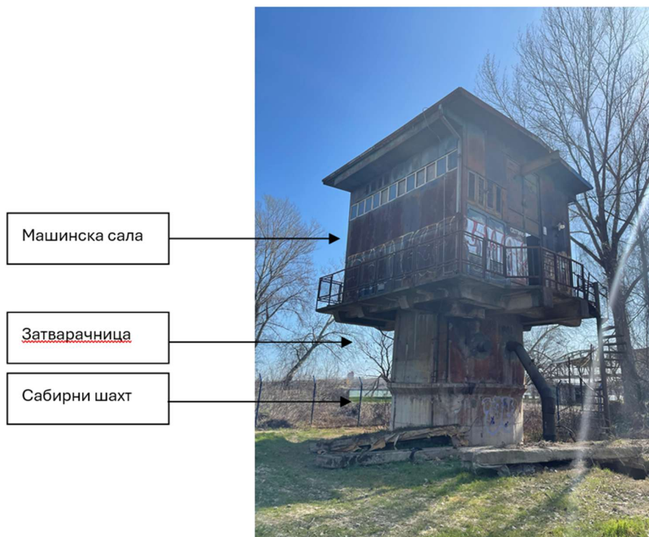
Слика 1. Надземни део рени бунара РБ 51
