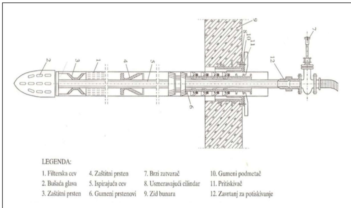
Слика 3.1. Утискивање хоризонталних дренава по Рени методи („Бунари са хоризонталним дренавима“, Д.Бабац, 1993.год.)
