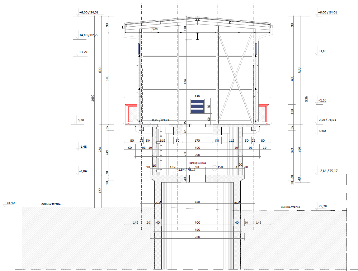
Сл.1.5.1.5.1. Попречни пресек кроз Рени бунар РБ-51
