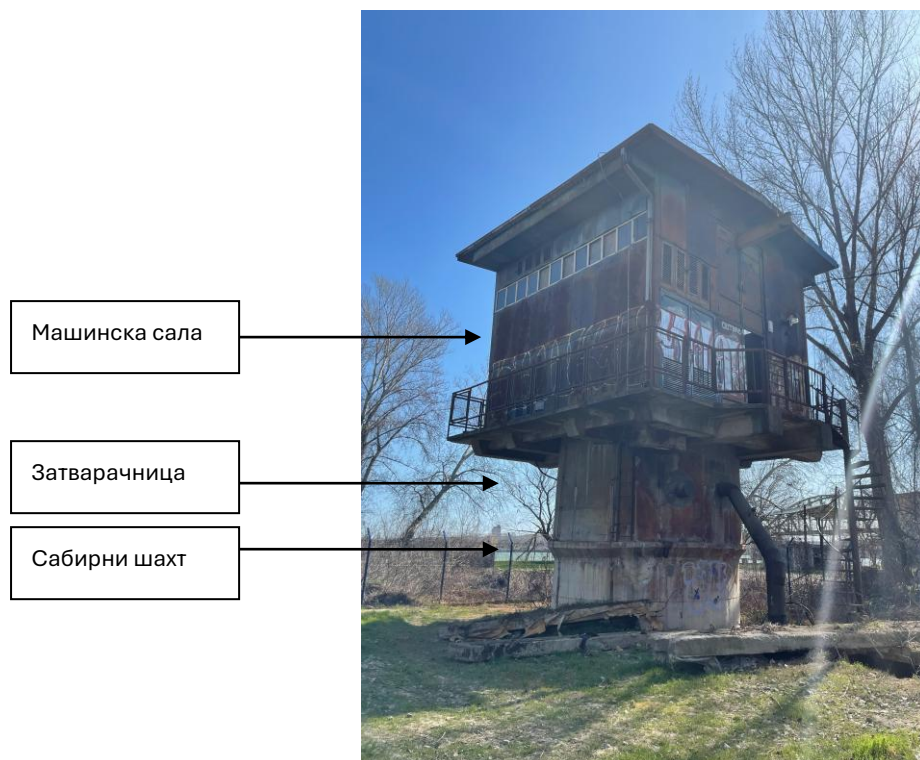
Слика 4 – Надземни део бунара РБ-51 - машинска сала и затварајница (снимак 2026 год.)
