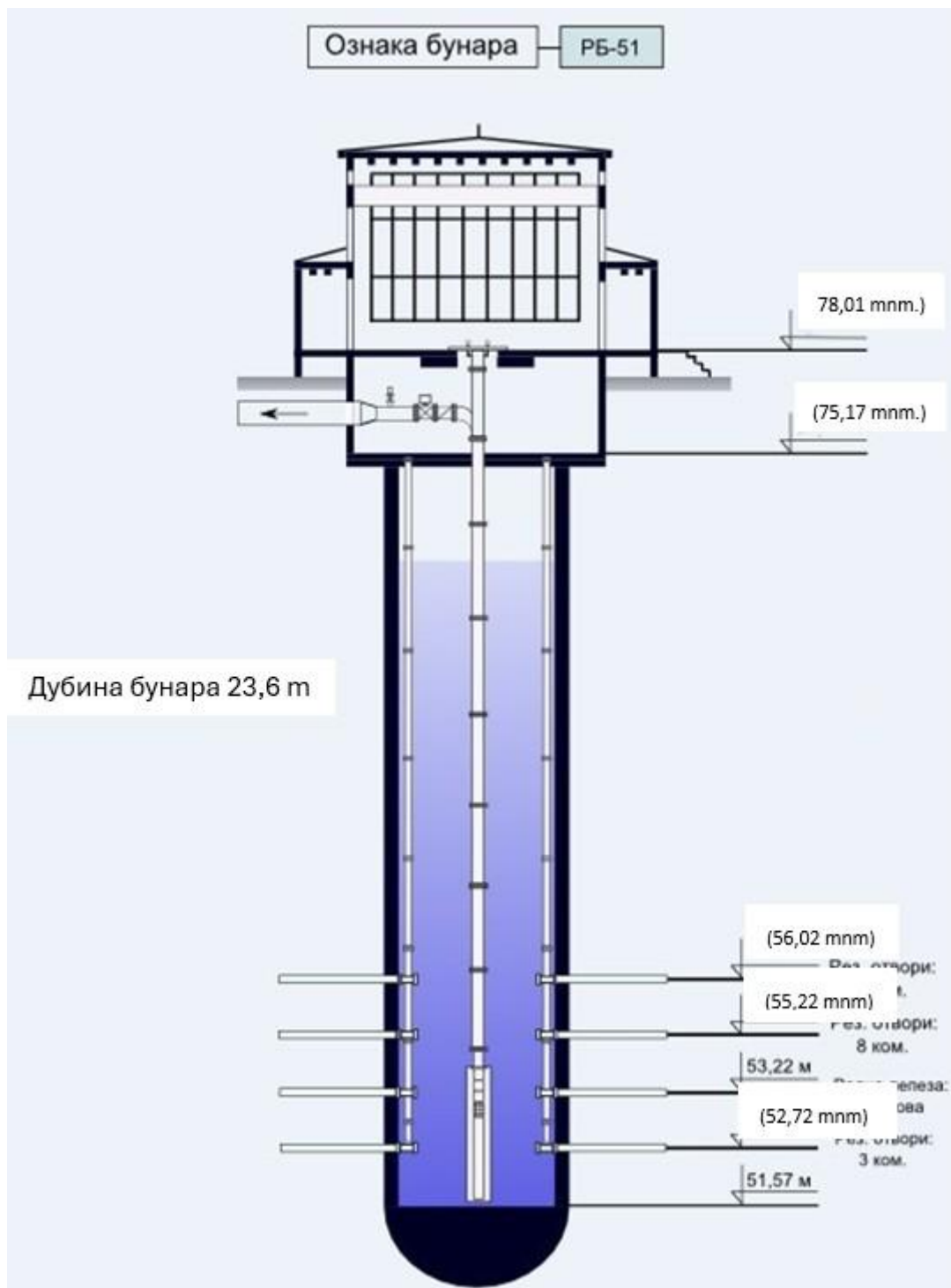
Слика 1. Шематски приказ бунара РБ-51 (Архив ЈКП „Београдски водовод и канализација“)
