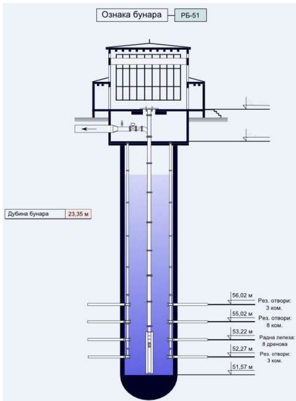
Слика 3. Шематски приказ шахта бунара РБ-51 (Архив ЈКП „Београдски водовод и канализација“)
