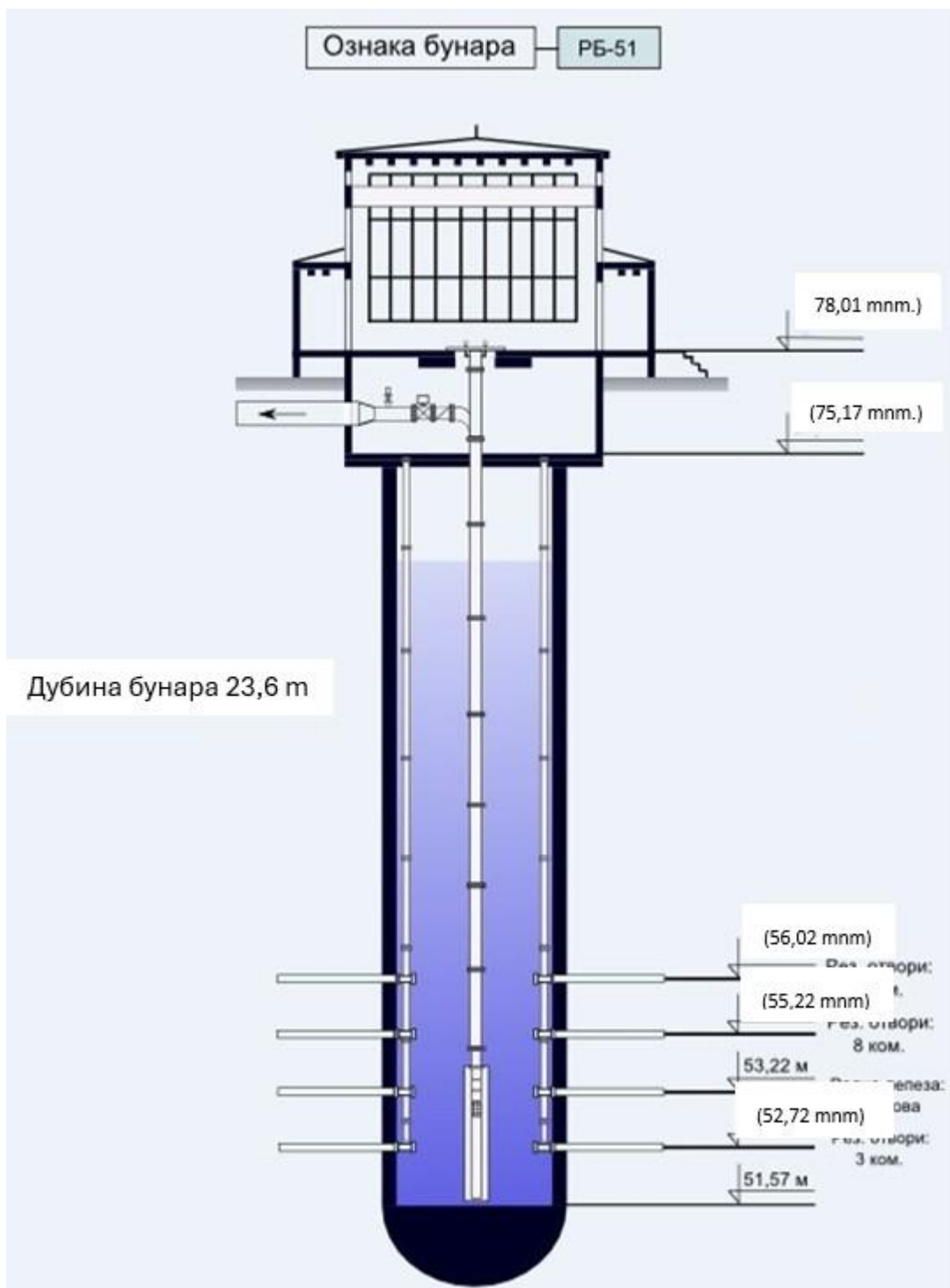
Слика 5 – Шематски приказ шахта бунара РБ-51 (Архив ЈКП „Београдски водовод и канализација“)
