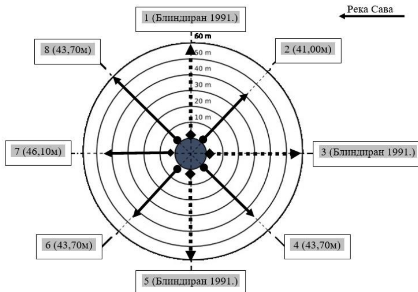
Слика 3 - Положај дрена бунара РБ-51 (Архив ЈКП „Београдски водовод и канализација“)
