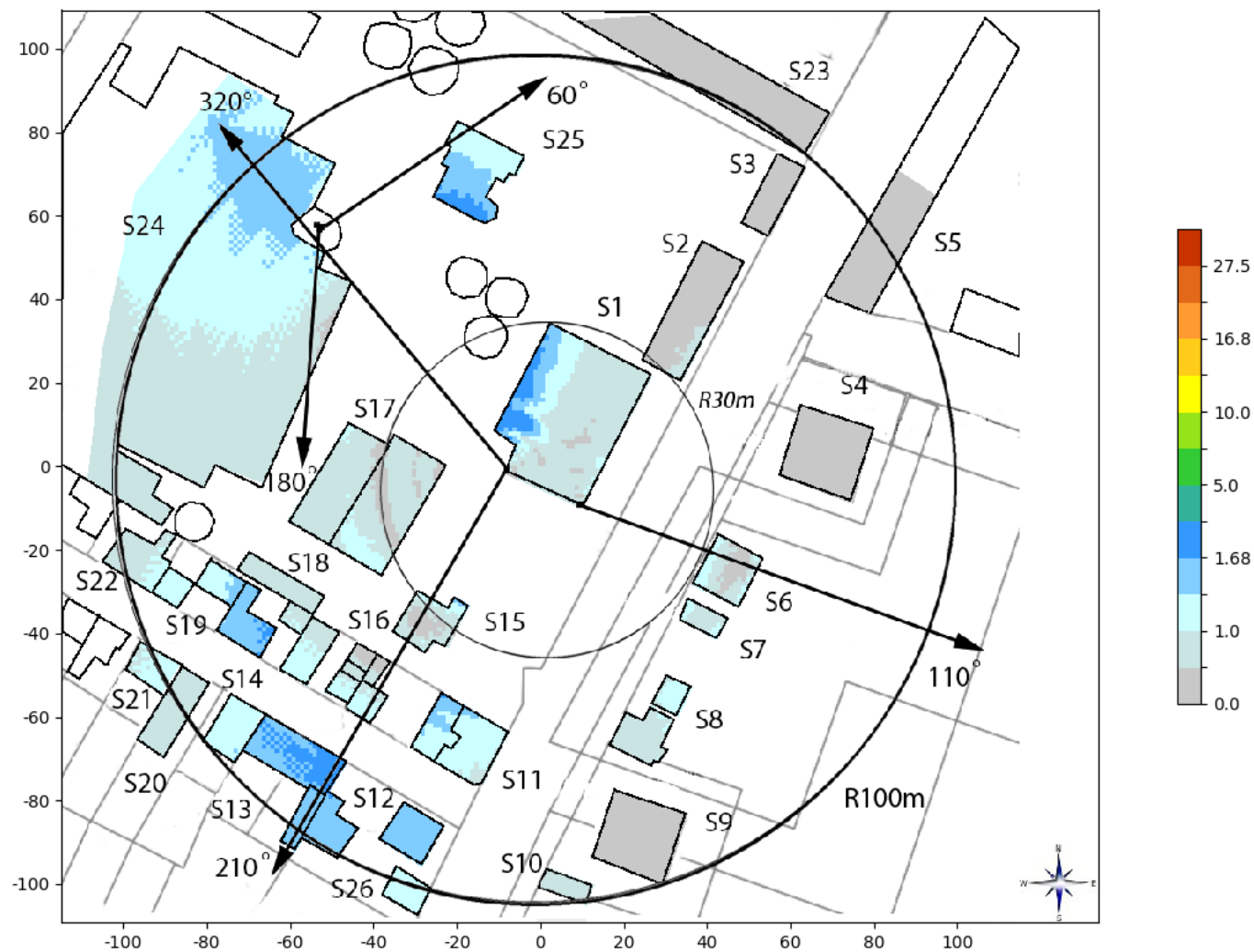
Slika 6.13: Rezultati proračuna jačine električnog polja unutar okolnih objekata za slučaj kada stanica GSM900 Telekom Srbije radi sa maks. kapacitetom.
