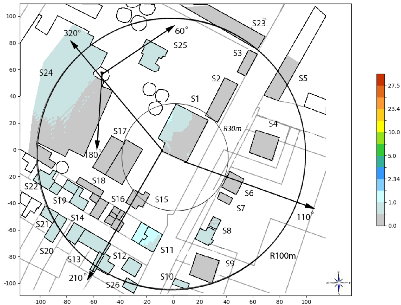
Slika 6.12: Rezultati proračuna jačine električnog polja unutar okolnih objekata za slučaj kada stanica LTE1800 Telekom Srbije radi sa maks. kapacitetom.
