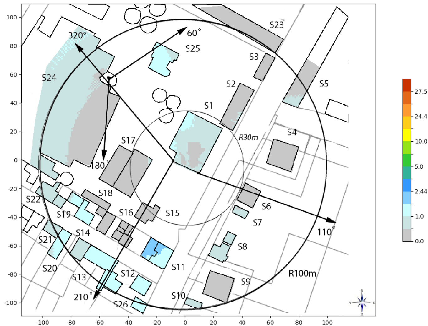
Slika 6.11: Rezultati proračuna jačine električnog polja unutar okolnih objekata za slučaj kada stanica UMTS2100 Telekom Srbije radi sa maks. kapacitetom.
