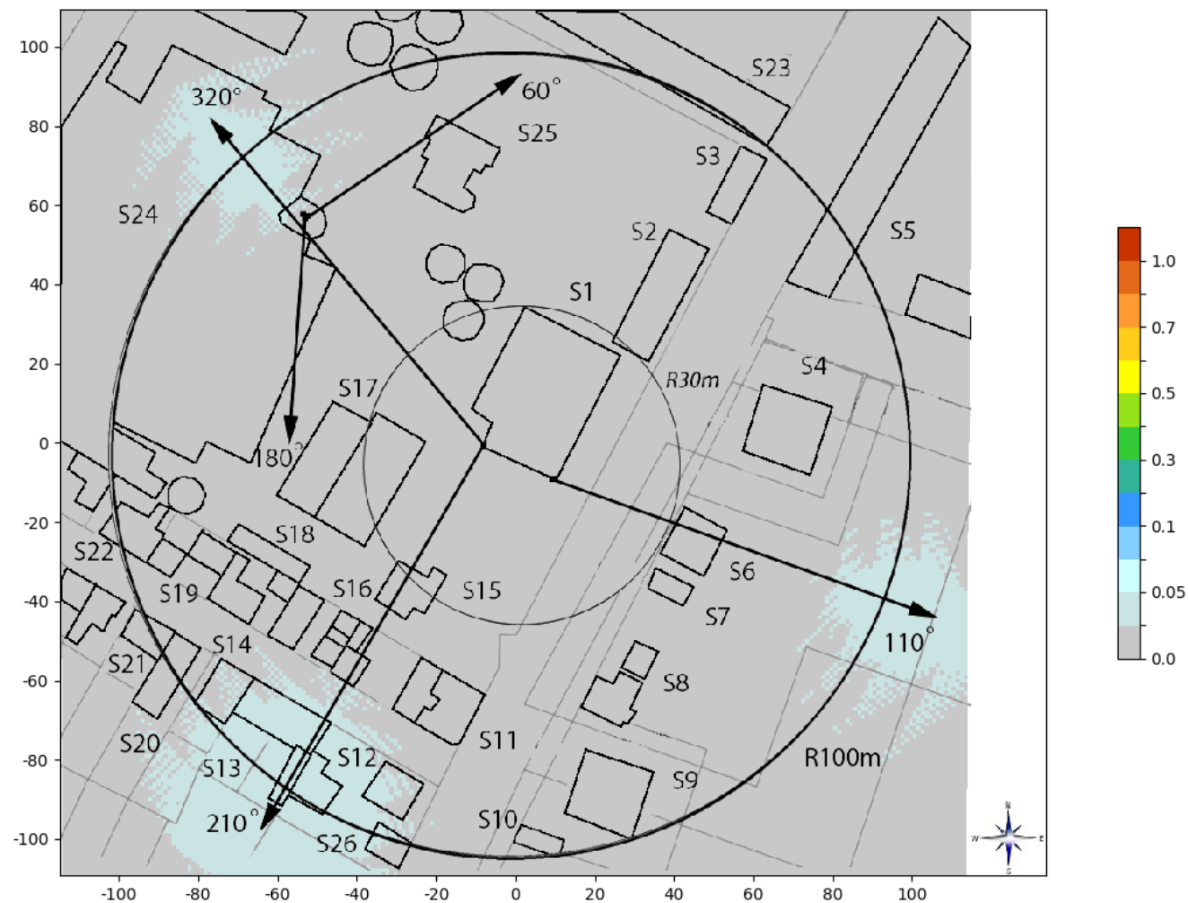
Slika 6.9: Rezultati proračuna faktora izlaganja na tlu, za slučaj kada svi sistemi operatora MTS i CETIN na lokaciji rade sa maksimalnim
