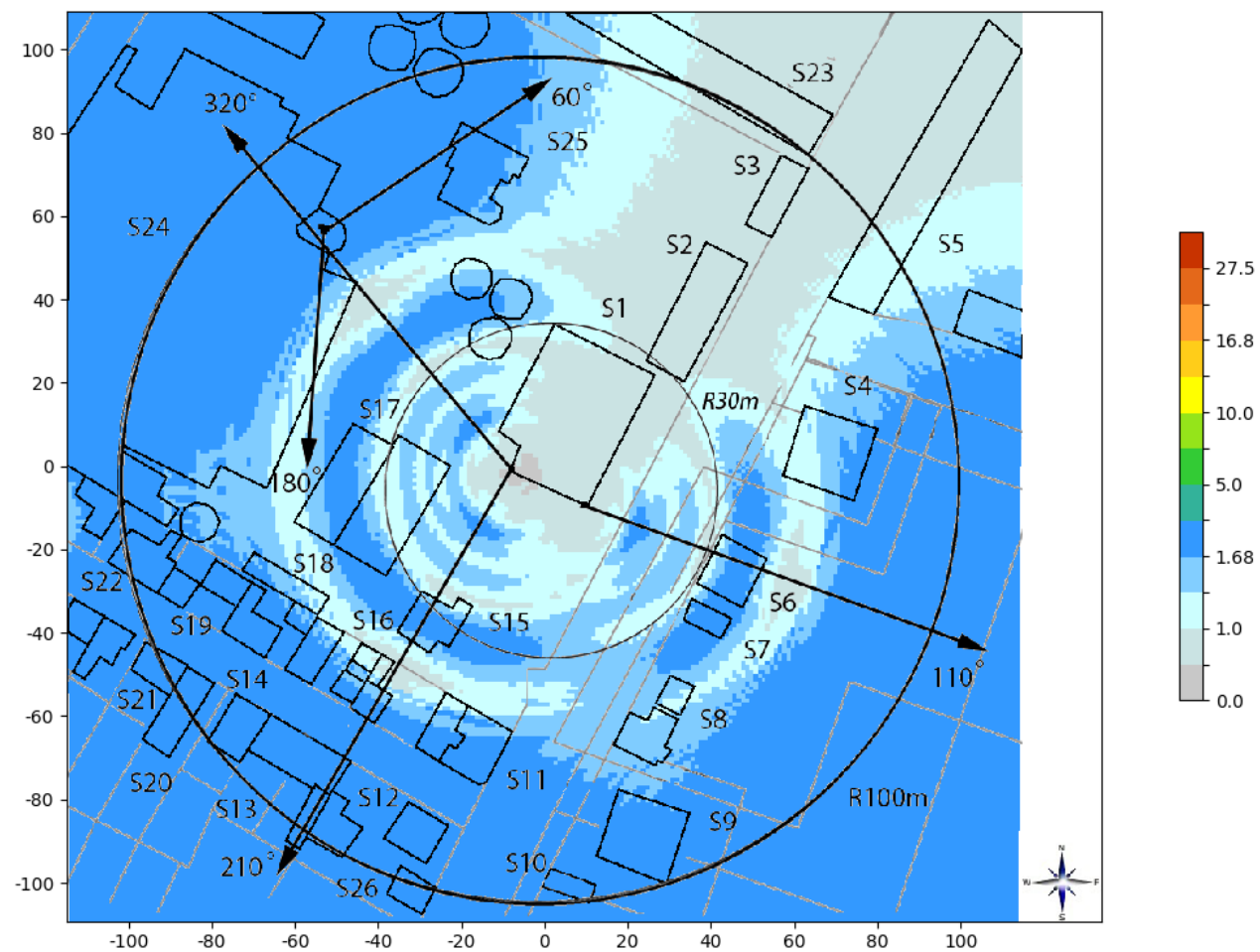
Slika 6.6: Rezultati proračuna jačine električnog polja na nivou tla sa uračunatom prosečnom visinom čoveka od 1.7m, kada svi sistemi Telekom Srbija rade sa maks. kapacitetom.
