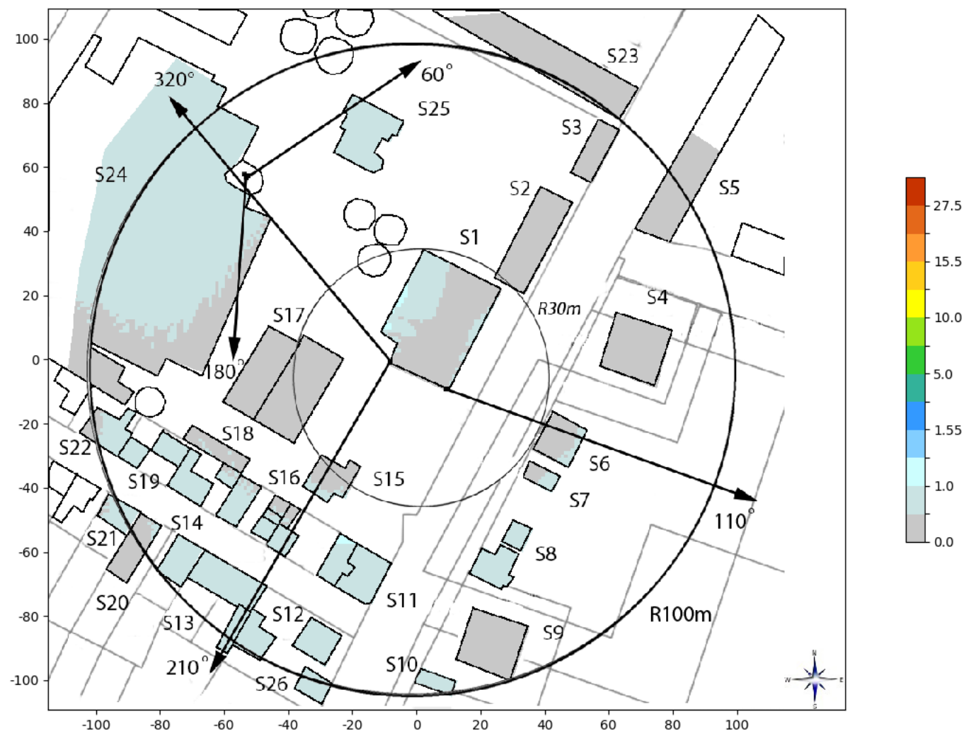
Slika 6.10: Rezultati proračuna jačine električnog polja unutar okolnih objekata za slučaj kada stanica LTE800 Telekom Srbije radi sa maks. kapacitetom.
