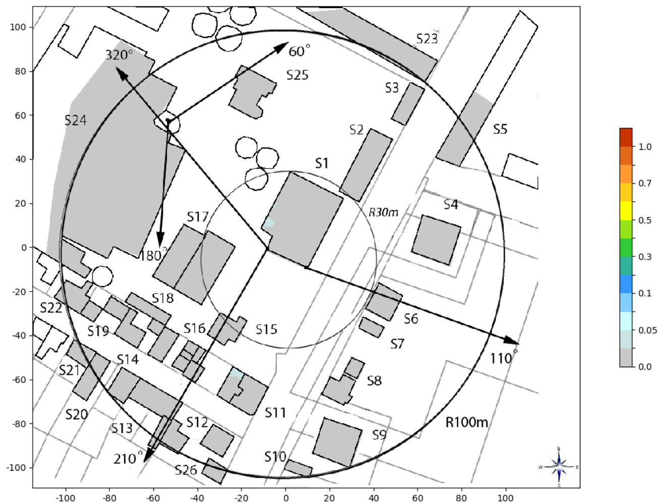
Slika 6.17: Rezultati proračuna faktora izlaganja u objektima, za slučaj kada svi sistemi operatora MTS i Cetin na lokaciji rade sa maks. kapacitetom
