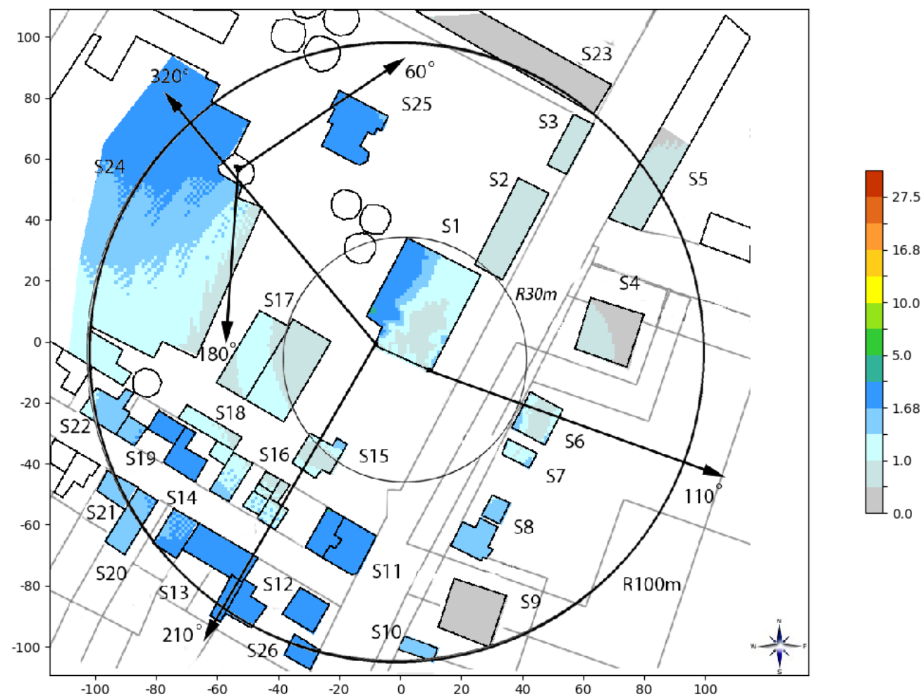
Slika 6.14: Rezultati proračuna jačine električnog polja unutar okolnih objekata za slučaj kada svi sistemi Telekom Srbije rade sa maks. kapacitetom.
