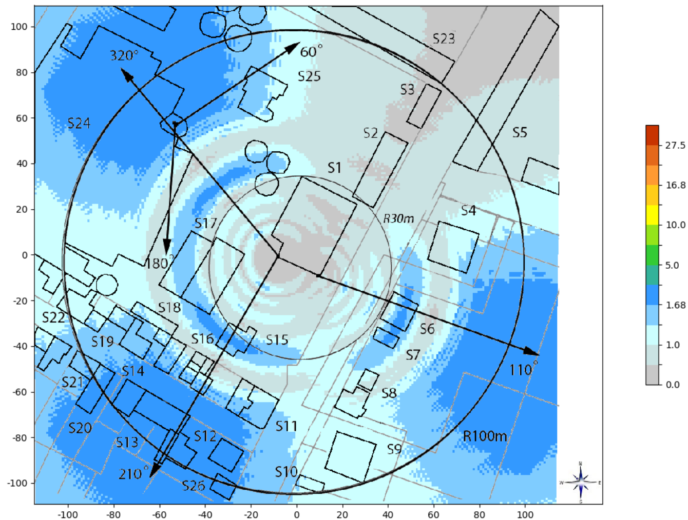
Slika 6.5: Rezultati proračuna jačine električnog polja na nivou tla sa uračunatom prosečnom visinom čoveka od 1.7m, kada bazna stanica GSM900 Telekom Srbije radi sa maks. kapacitetom.
