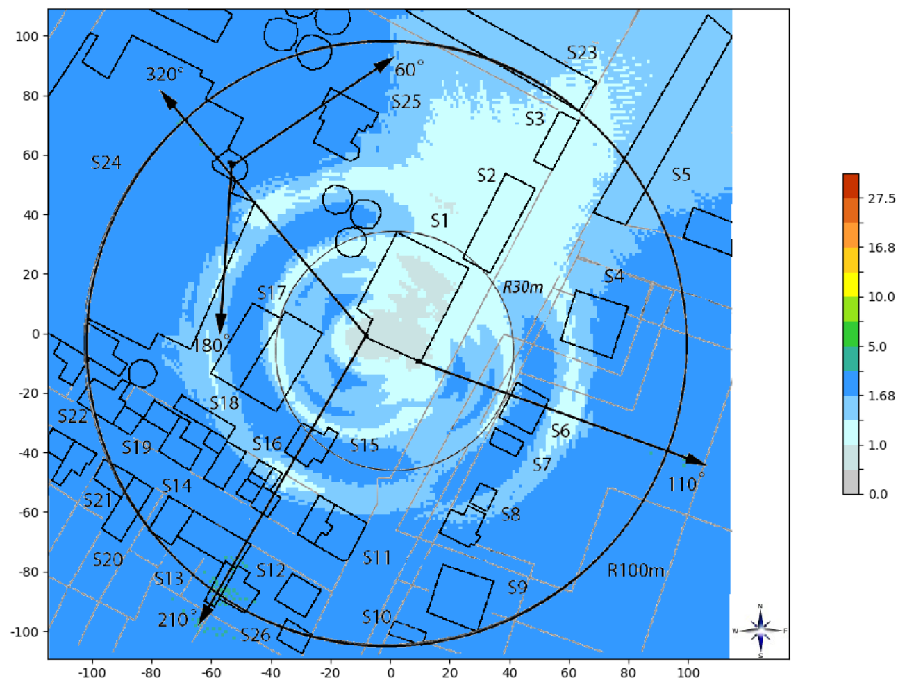
Slika 6.8: Rezultati proračuna jačine električnog polja na tlu, za slučaj kada svi sistemi operatora MTS i Cetin na lokaciji rade sa maksimalnim kapacitetom.
