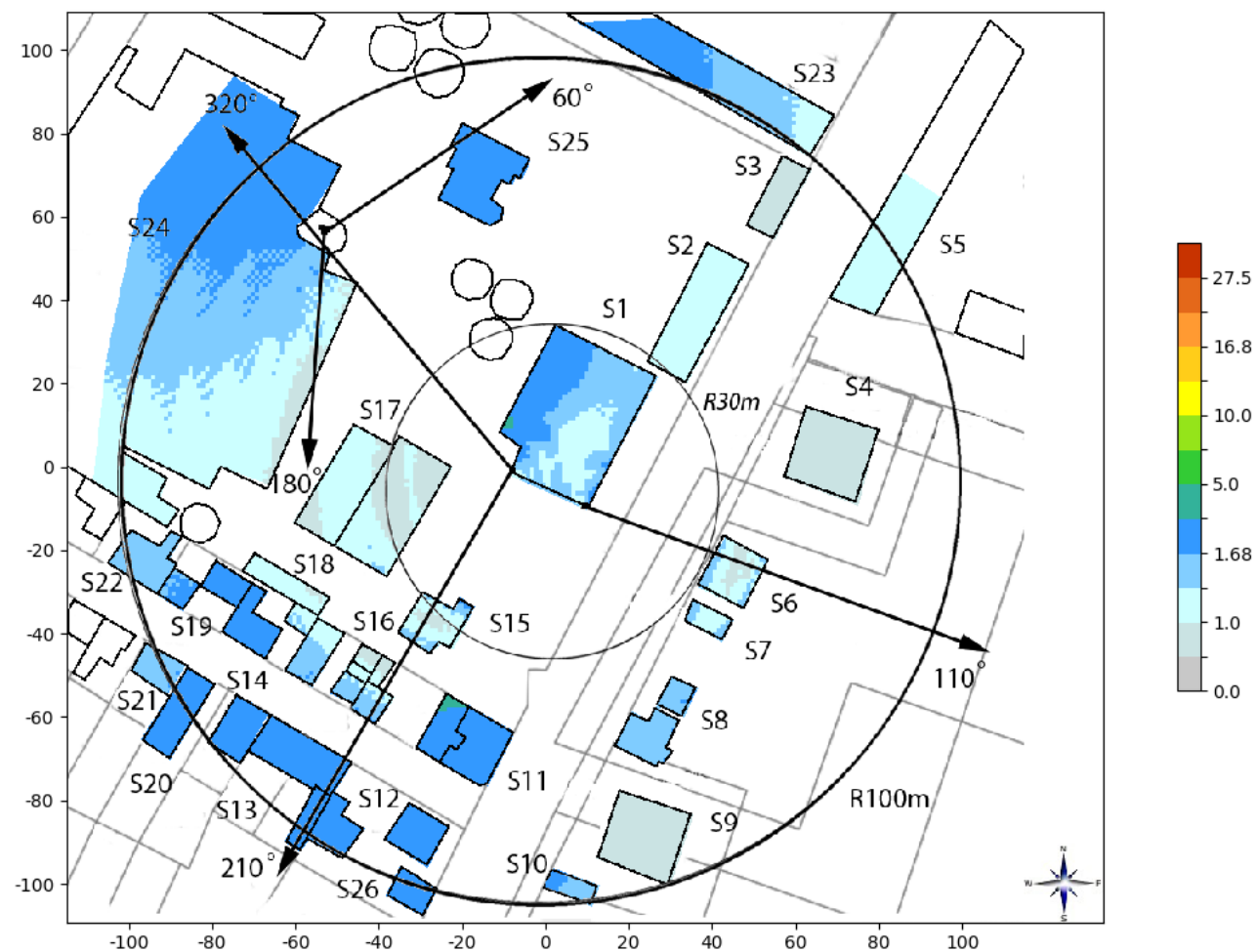
Slika 6.16: Rezultati proračuna jačine električnog polja u objektima, za slučaj kada sve stanice operatora MTS i Cetin rade sa maks. kapacitetom.
