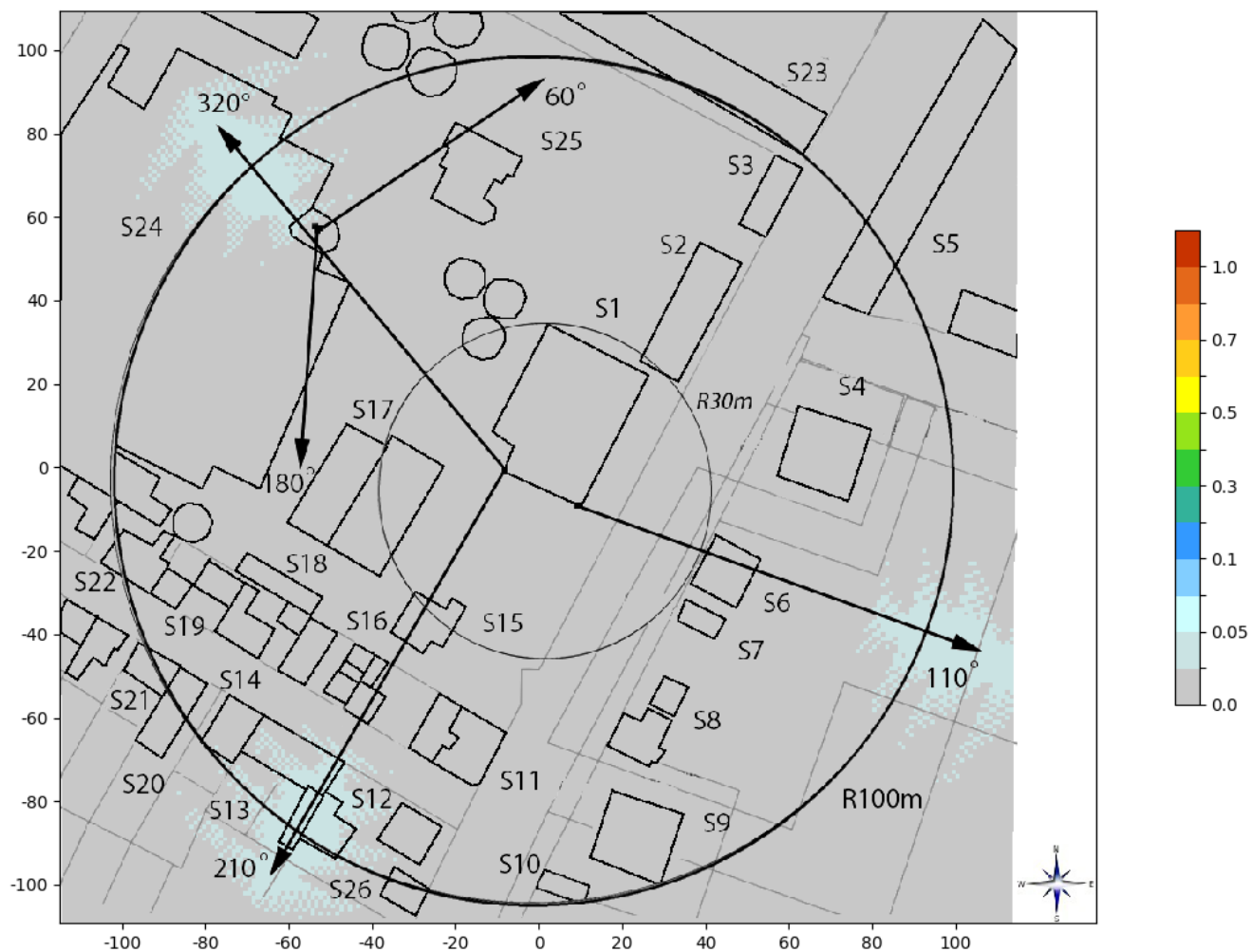
Slika 6.7: Rezultati proračuna faktora izlaganja na nivou tla sa uračunatom prosečnom visinom čoveka od 1.7m za slučaj kada svi sistemi Telekom Srbije rade sa maks. kapacitetom.
