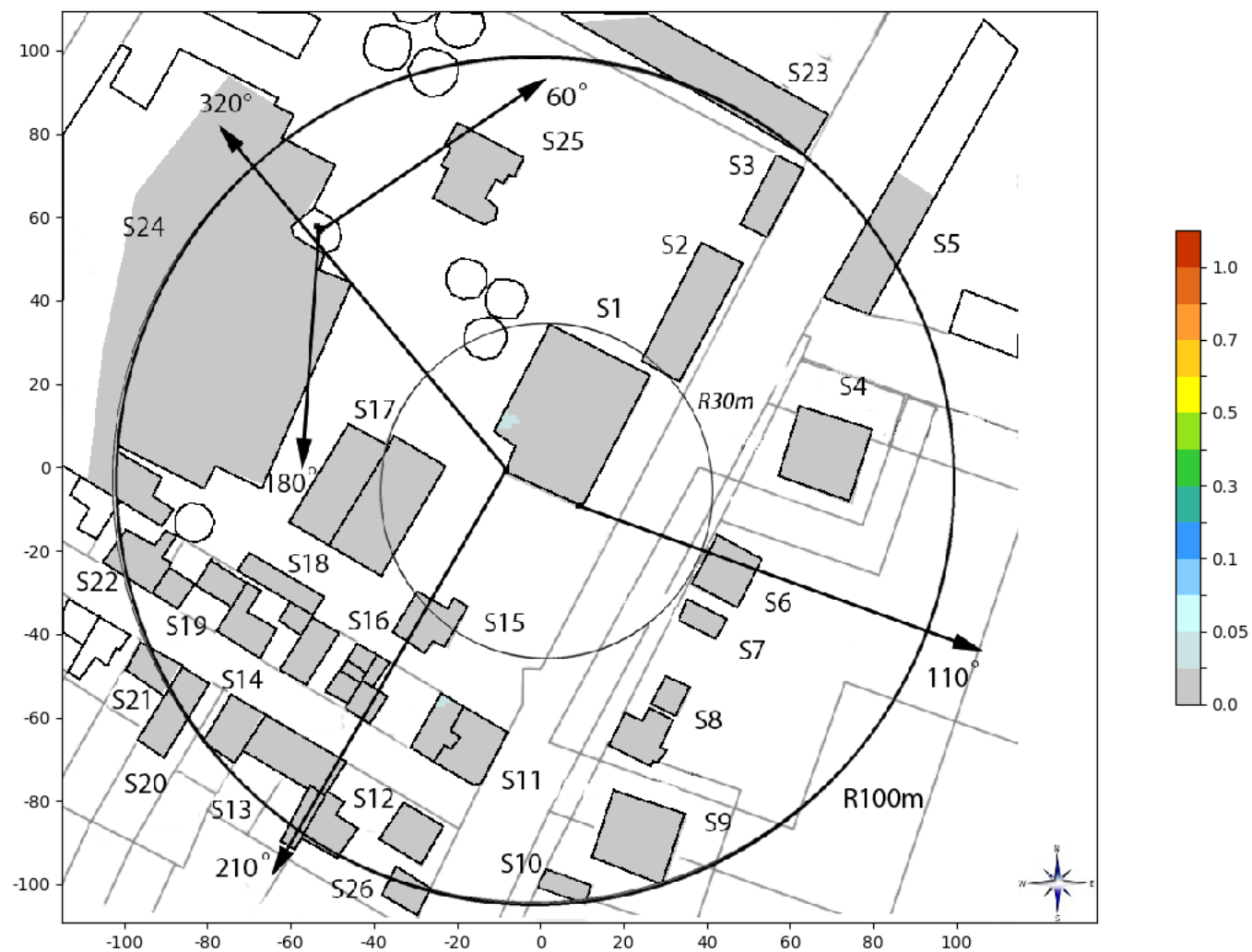
Slika 6.15: Rezultati proračuna faktora izlaganja unutar okolnih objekata za slučaj kada svi sistemi Telekom Srbija rade sa maksimalnim kapacitetom
