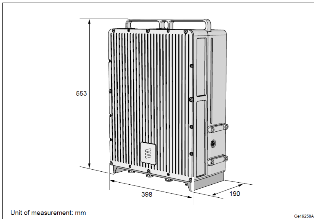
Slika 9.3. Dimenzije radio modula 2479/4499
