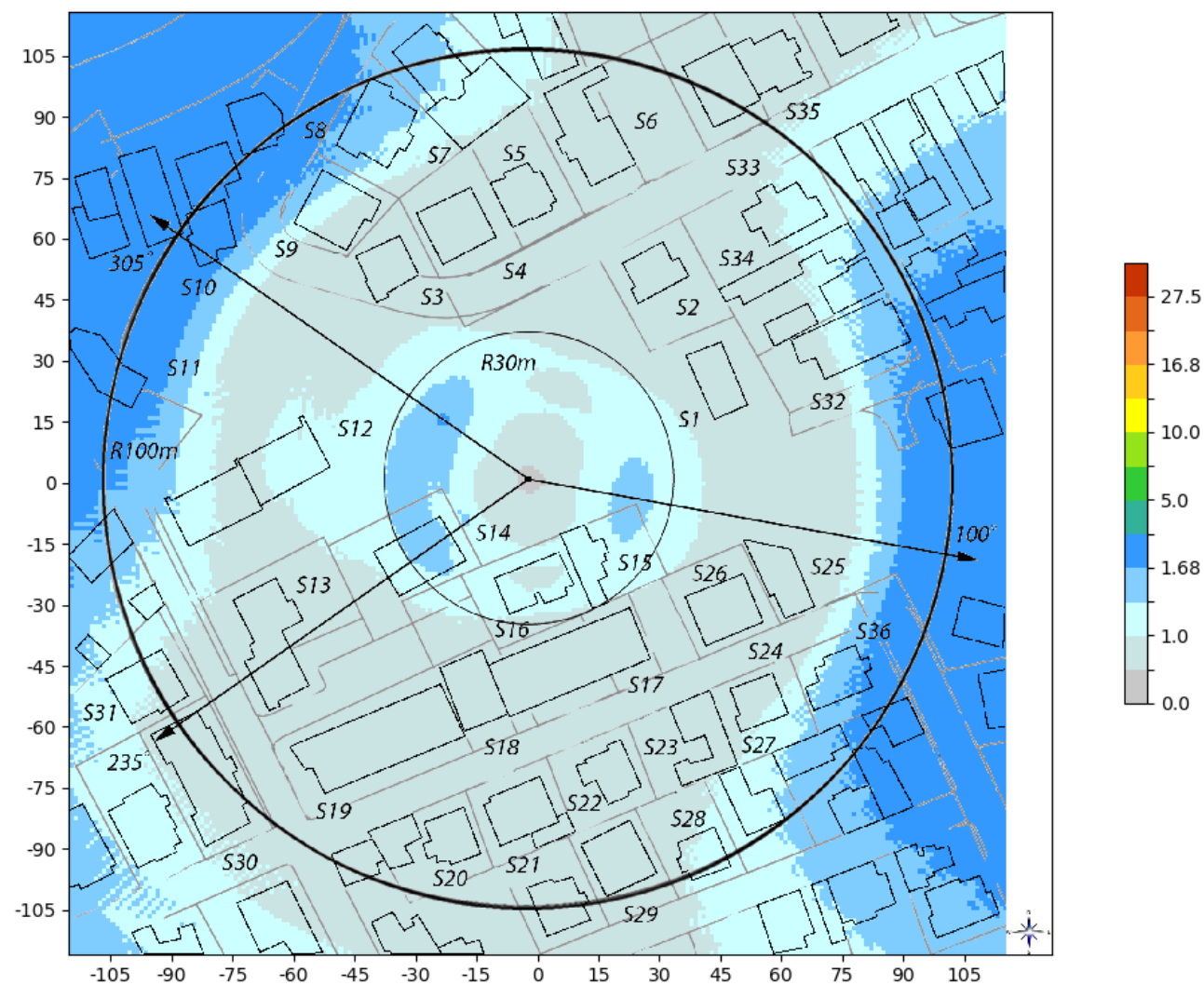
Slika 6.6: Rezultati proračuna jačine električnog polja na nivou tla sa uvažanom prosečnom visinom čoveka od 1.7m, kada svi sistemi Telekom Srbija rade sa maks. kapacitetom.
