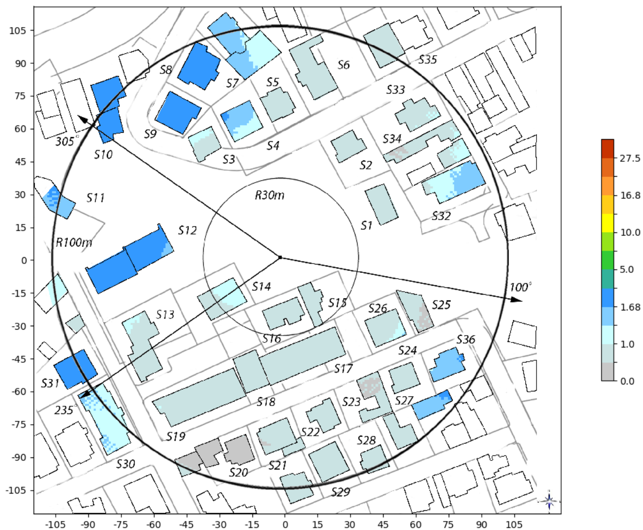
Slika 6.16: Rezultati proračuna jačine električnog polja unutar okolnih objekata za slučaj kada svi sistemi MTS i GSM-R rade sa maks. kapacitetom.
