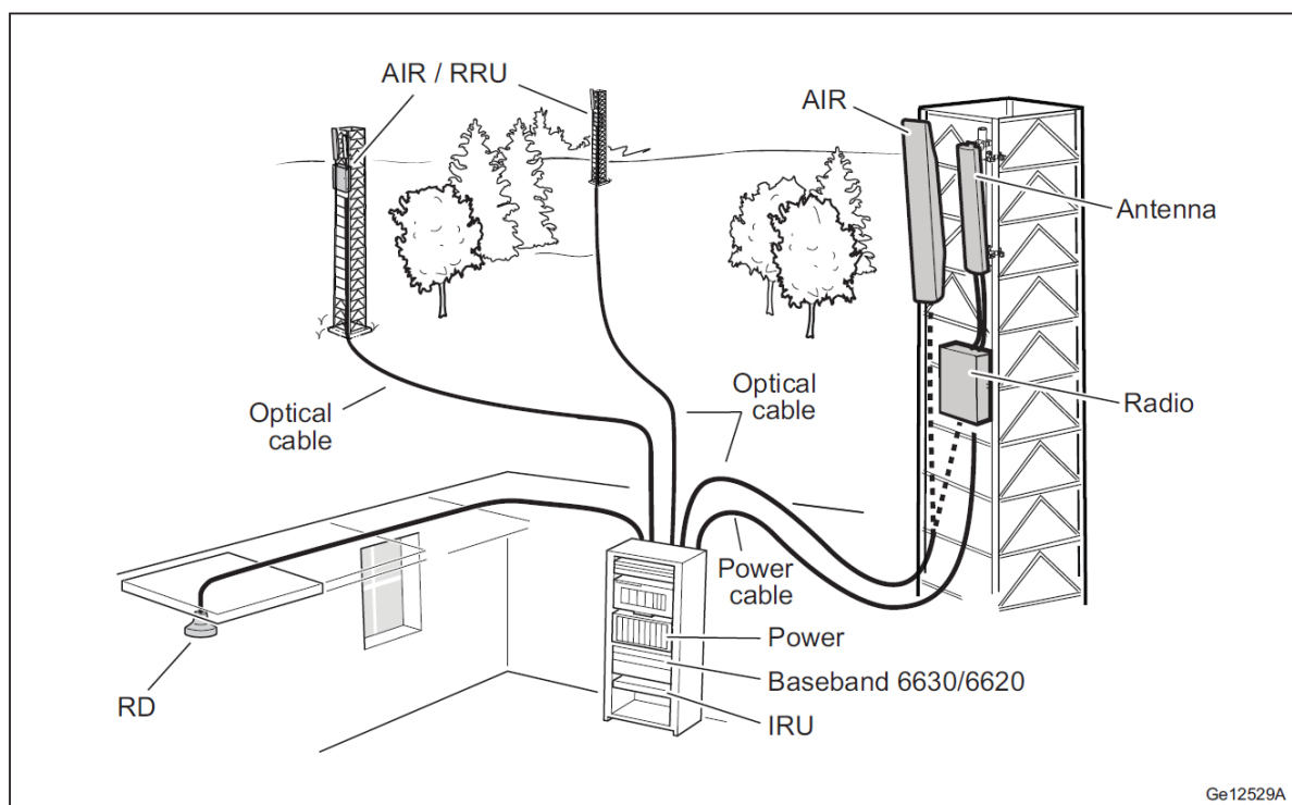
Sl. 9.1. Shema bazne stanice
