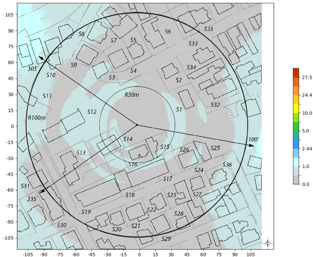
Slika 6.3: Rezultati proračuna jačine električnog polja na nivou tla sa uračunatom prosečnom visinom čoveka od 1.7m, kad bazna stanica UMTS2100 Telekom Srbija radi sa maks. kapacitetom.
