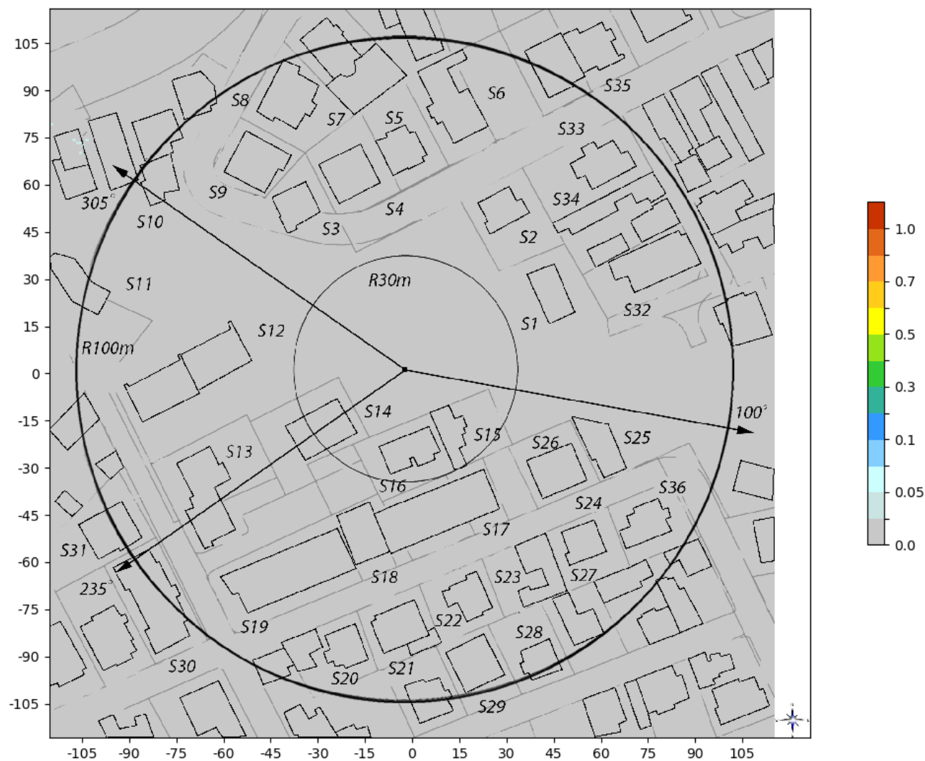
Slika 6.7: Rezultati proračuna faktora izlaganja na nivou tla sa uračunatom prosečnom visinom čoveka od 1.7m za slučaj kada svi sistemi Telekom Srbije rade sa maks. kapacitetom.
