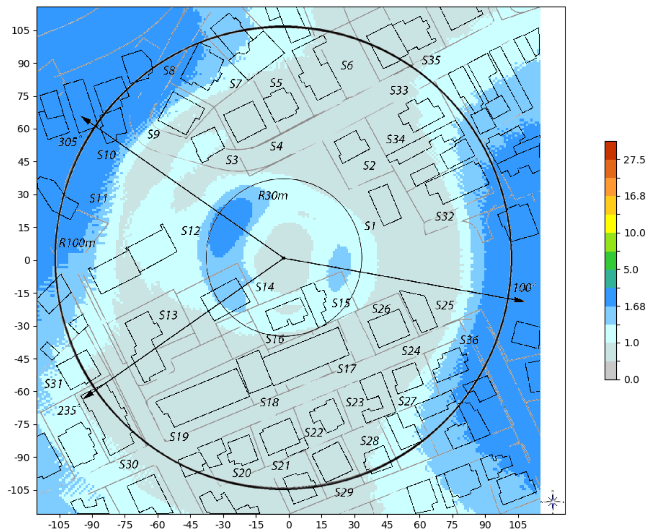
Slika 6.8: Rezultati proračuna jačine električnog polja na nivou tla sa uračunatom prosečnom visinom čoveka od 1.7m, kada sistemi MTS i GSM-R rade sa maks. kapacitetom.
