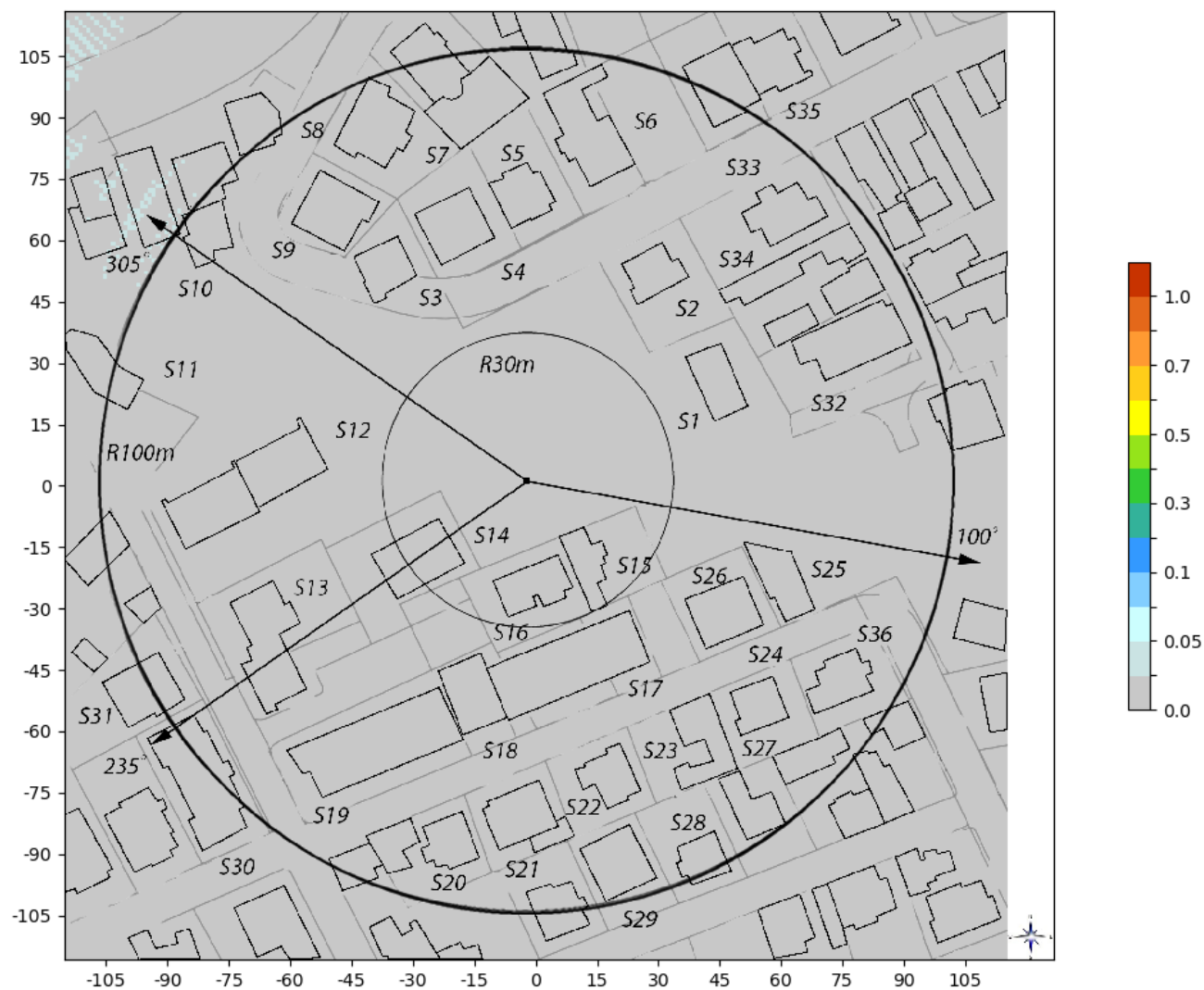
Slika 6.9: Rezultati proračuna faktora izlaganja na nivou tla sa uračunatom prosečnom visinom čoveka od 1.7m za slučaj kada sistemi MTS i GSM-R rade sa maks. kapacitetom.
