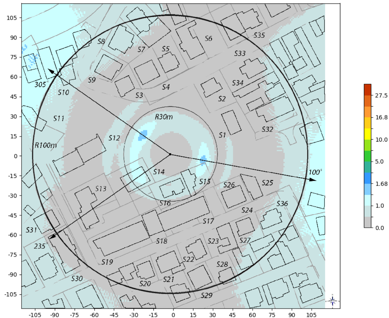
Slika 6.5: Rezultati proračuna jačine električnog polja na nivou tla sa uračunatom prosečnom visinom čoveka od 1.7m, kada bazna stanica GSM900 Telekom Srbije radi sa maks. kapacitetom.
