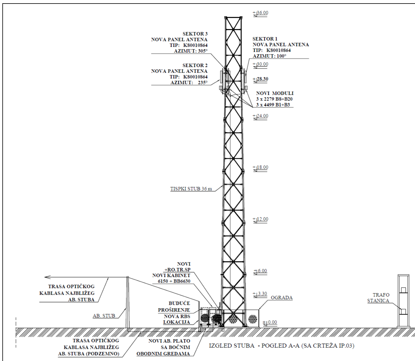
Slika 3.2.1. Projektovano stanje – osnova
