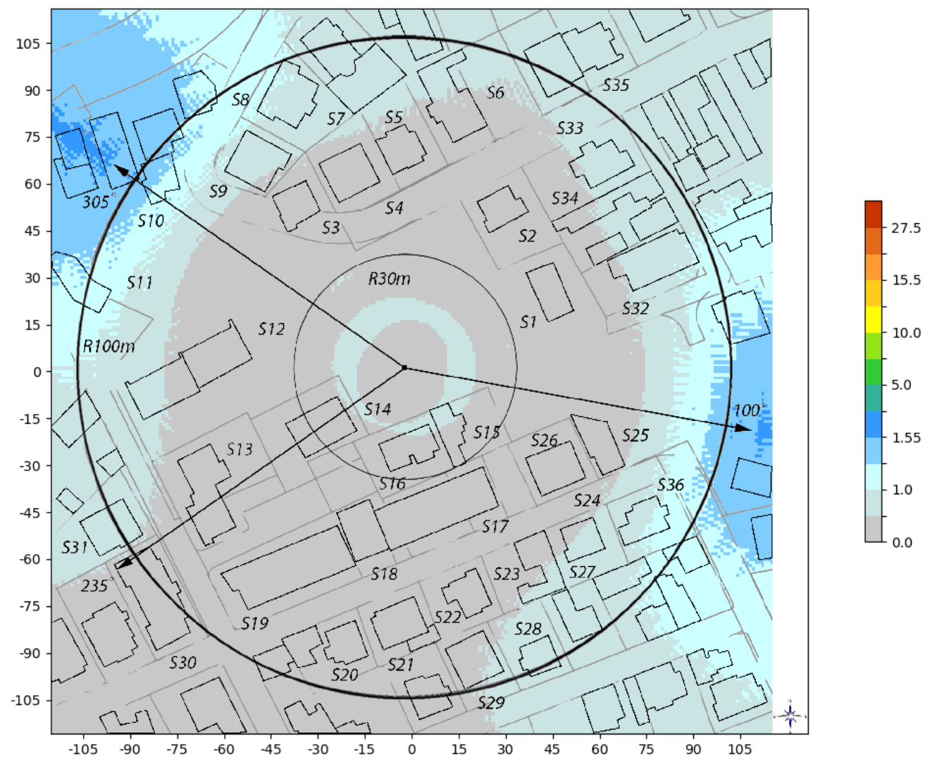
Slika 6.2: Rezultati proračuna jačine električnog polja na nivou tla sa uračunatom prosečnom visinom čoveka od 1.7m, kada bazna stanica LTE800 Telekom Srbija radi sa maks. kapacitetom
