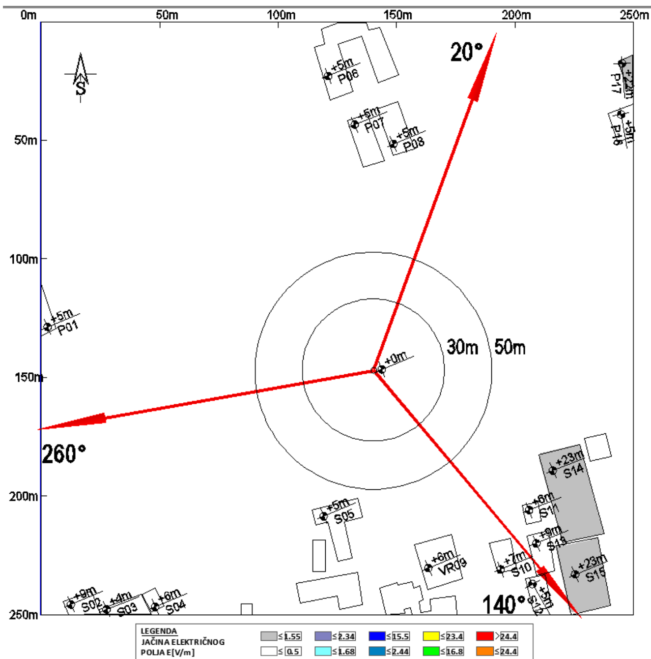
Slika 4.5 Rezultati proračuna jačine električnog polja u objektima na najizloženijim spratovima za slučaj rada sistema LTE1800 20MHz operatora A1 Srbija
