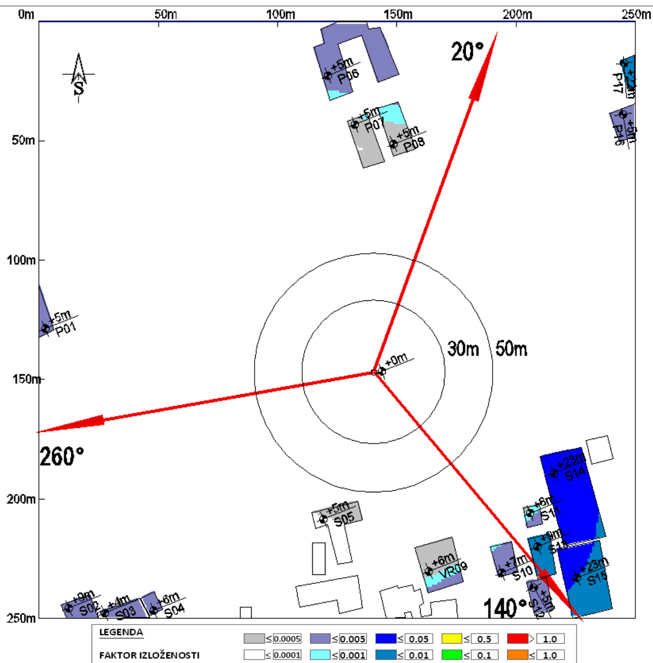
Slika 4.8 Rezultati proračuna faktora izloženosti u objektima na najizloženijim spratovima za slučaj rada sistema GSM900/UMTS2100/LTE2100/LTE1800/LTE800 operatora A1 Srbija
