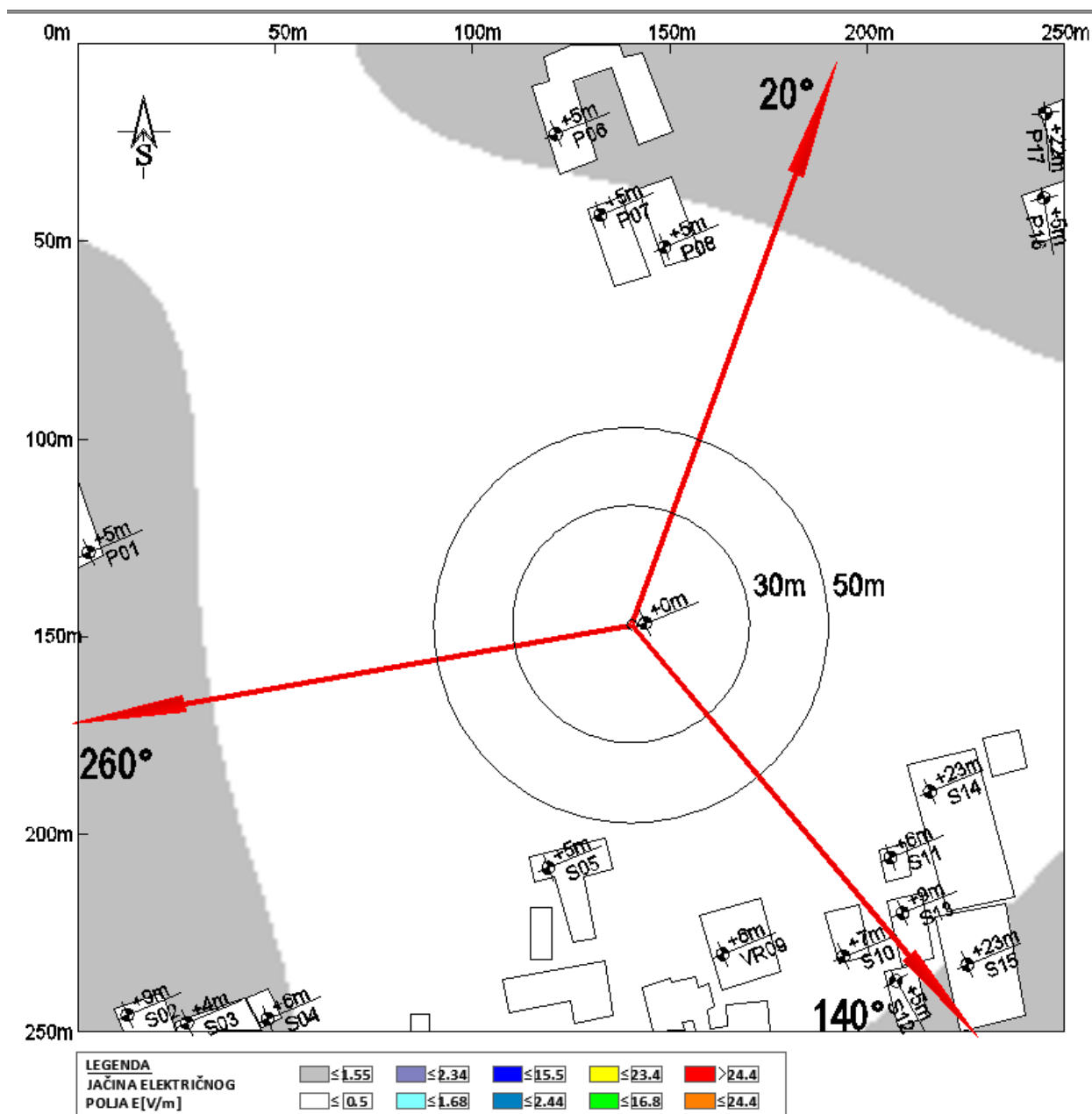
Slika 4.15 Maksimalna proračunata vrednost električnog polja na nivou tla u slučaju rada sistema LTE800 operatora A1 iznosi: 0.91 V/m
