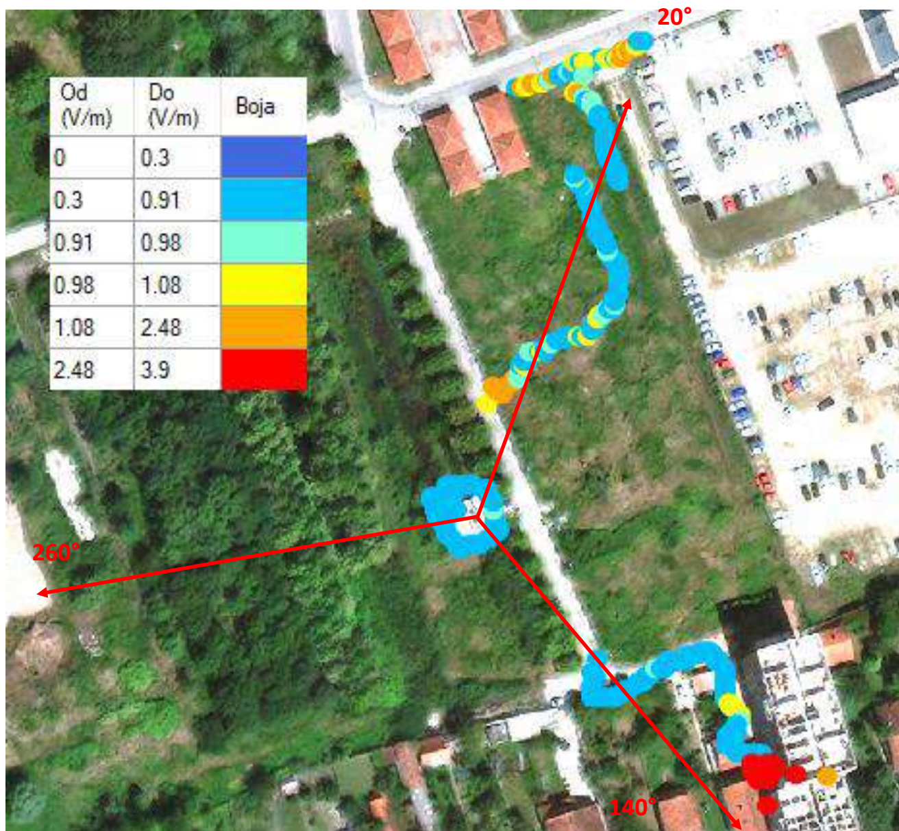
Prostorna raspodela polja u okolini antenskog sistema
