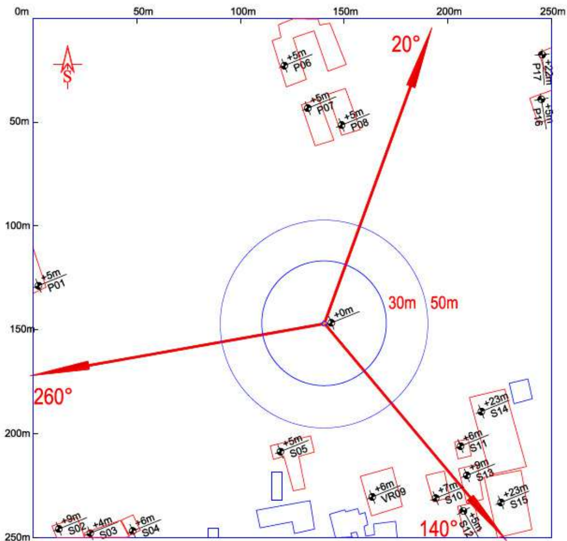
Slika 5.2 Dijagram prepreka u okruženju radio bazne stanice na lokaciji «BG0102_01 BG_Zrenjaninski put Branka Momirova»
