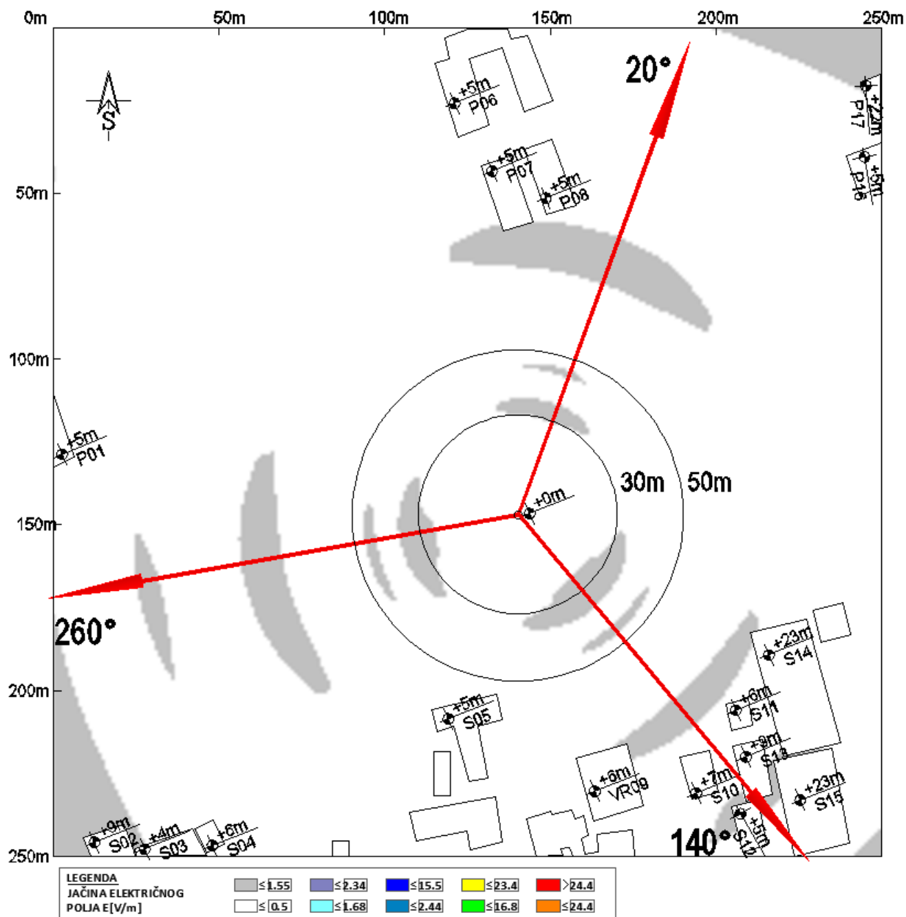
Slika 4.12 Maksimalna proračunata vrednost električnog polja na nivou tla u slučaju rada sistema UMTS2100 operatora A1 iznosi: 1.02 V/m
