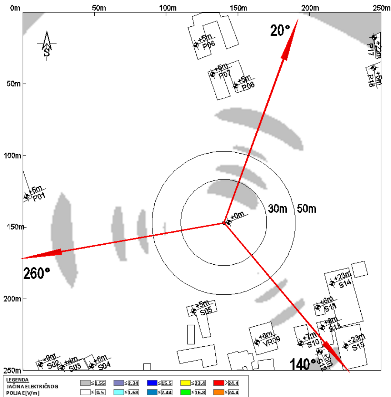
Slika 4.14 Maksimalna proračunata vrednost električnog polja na nivou tla u slučaju rada sistema LTE1800 20MHz operatora A1 iznosi: 0.96 V/m
