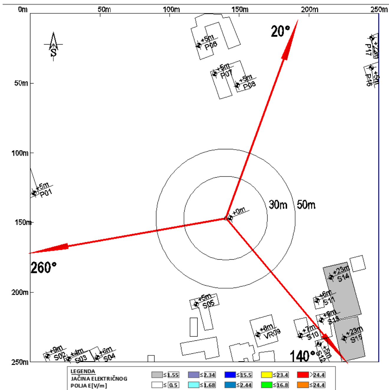
Slika 4.6 Rezultati proračuna jačine električnog polja u objektima na najizloženijim spratovima za slučaj rada sistema LTE800 operatora A1 Srbija
