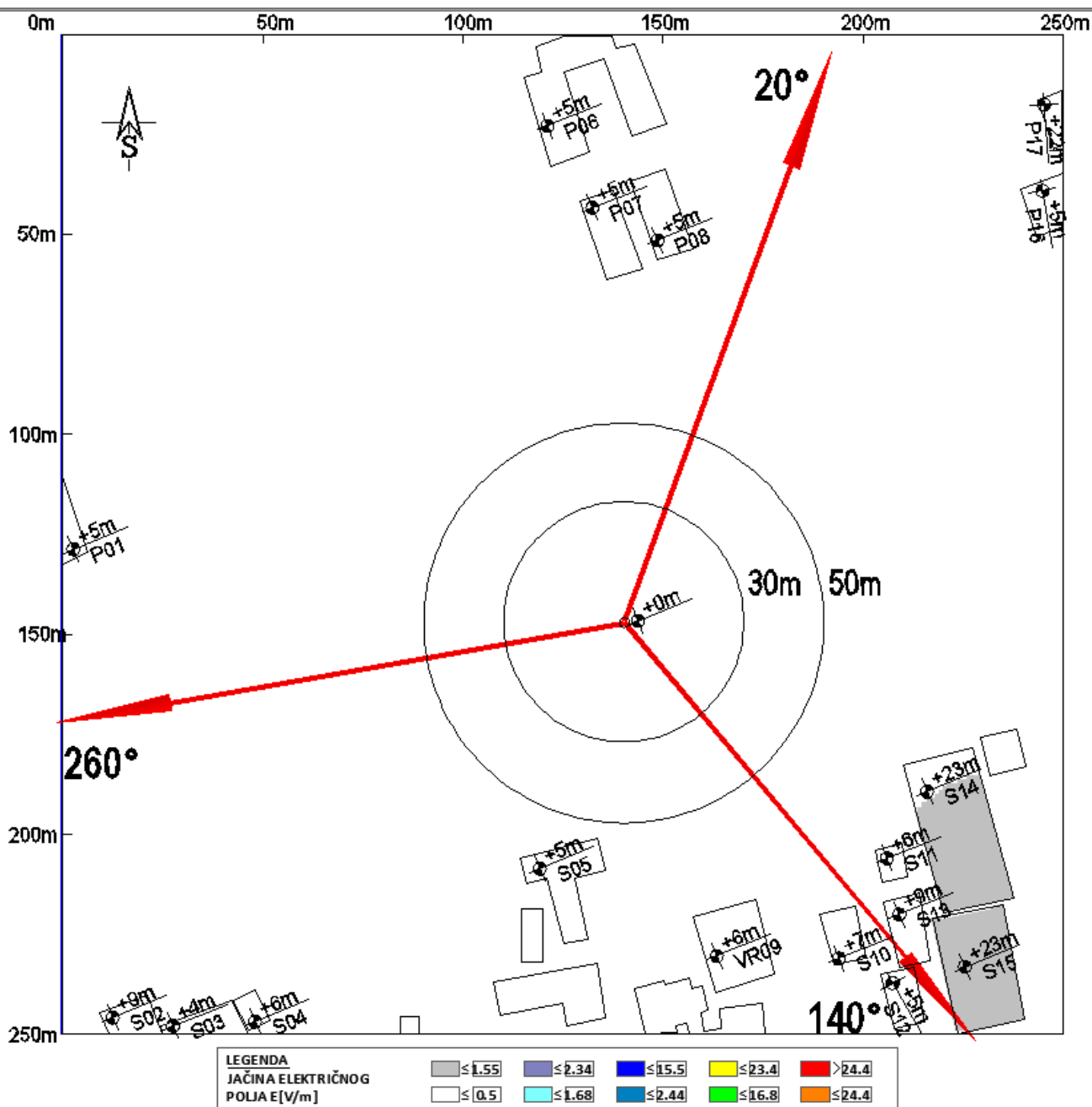
Slika 4.4 Rezultati proračuna jačine električnog polja u objektima na najizloženijim spratovima za slučaj rada sistema LTE1800 10MHz operatora A1 Srbija
