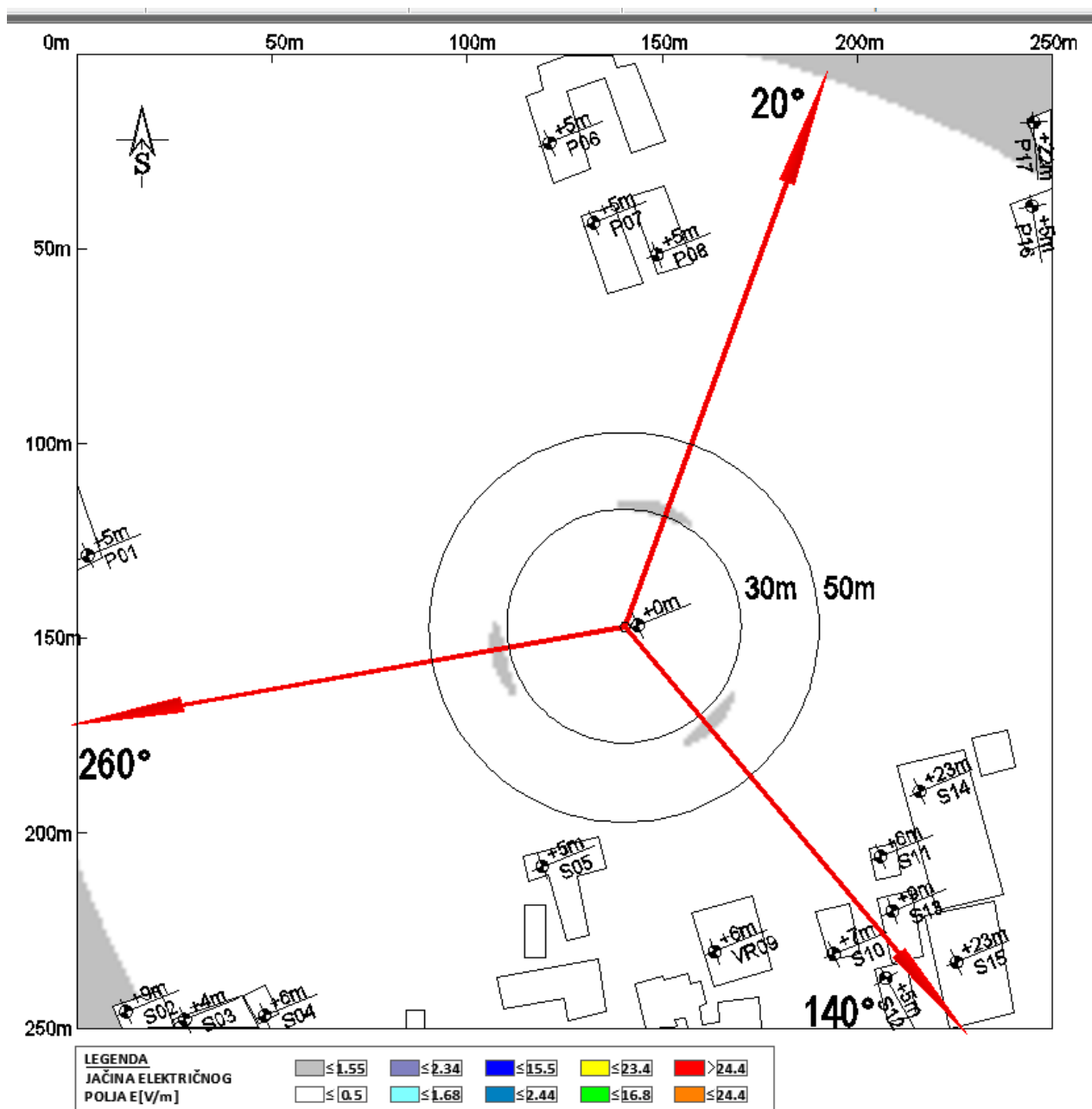
Slika 4.11 Maksimalna proračunata vrednost električnog polja na nivou tla u slučaju rada sistema LTE2100 operatora A1 iznosi: 0.79 V/m
