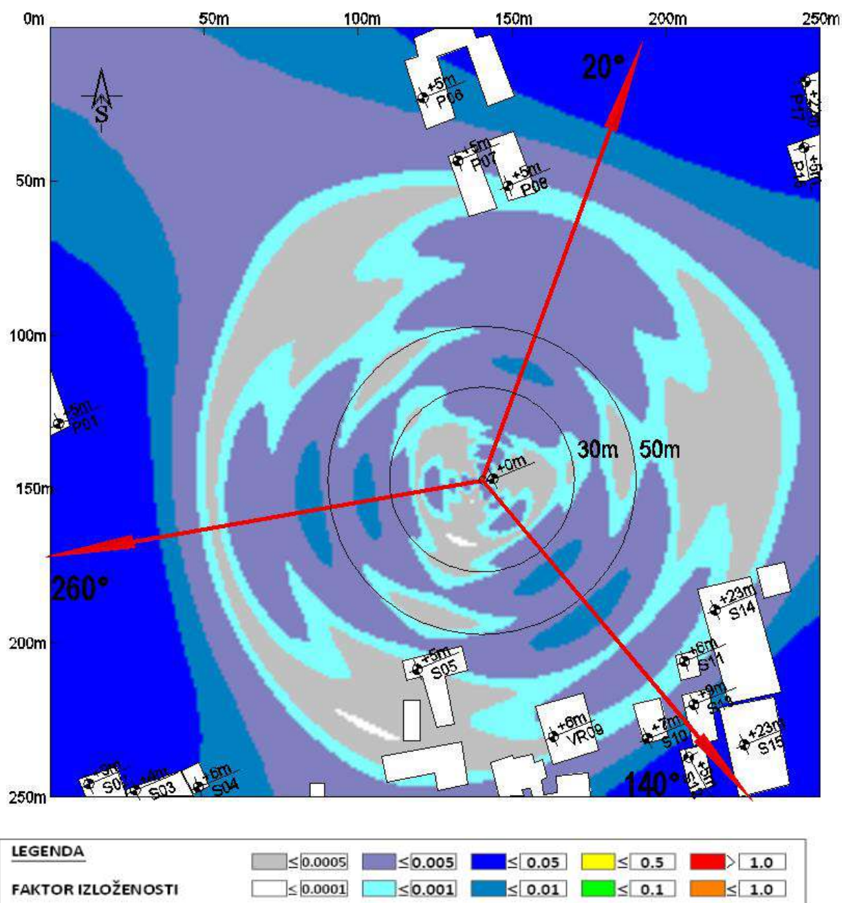
Slika 4.17 Maksimalna proračunata vrednost ukupnog faktora izloženosti na nivou tla u slučaju rada svih sistema na predmetnoj lokaciji operatora A1 iznosi: 0.0293 .
