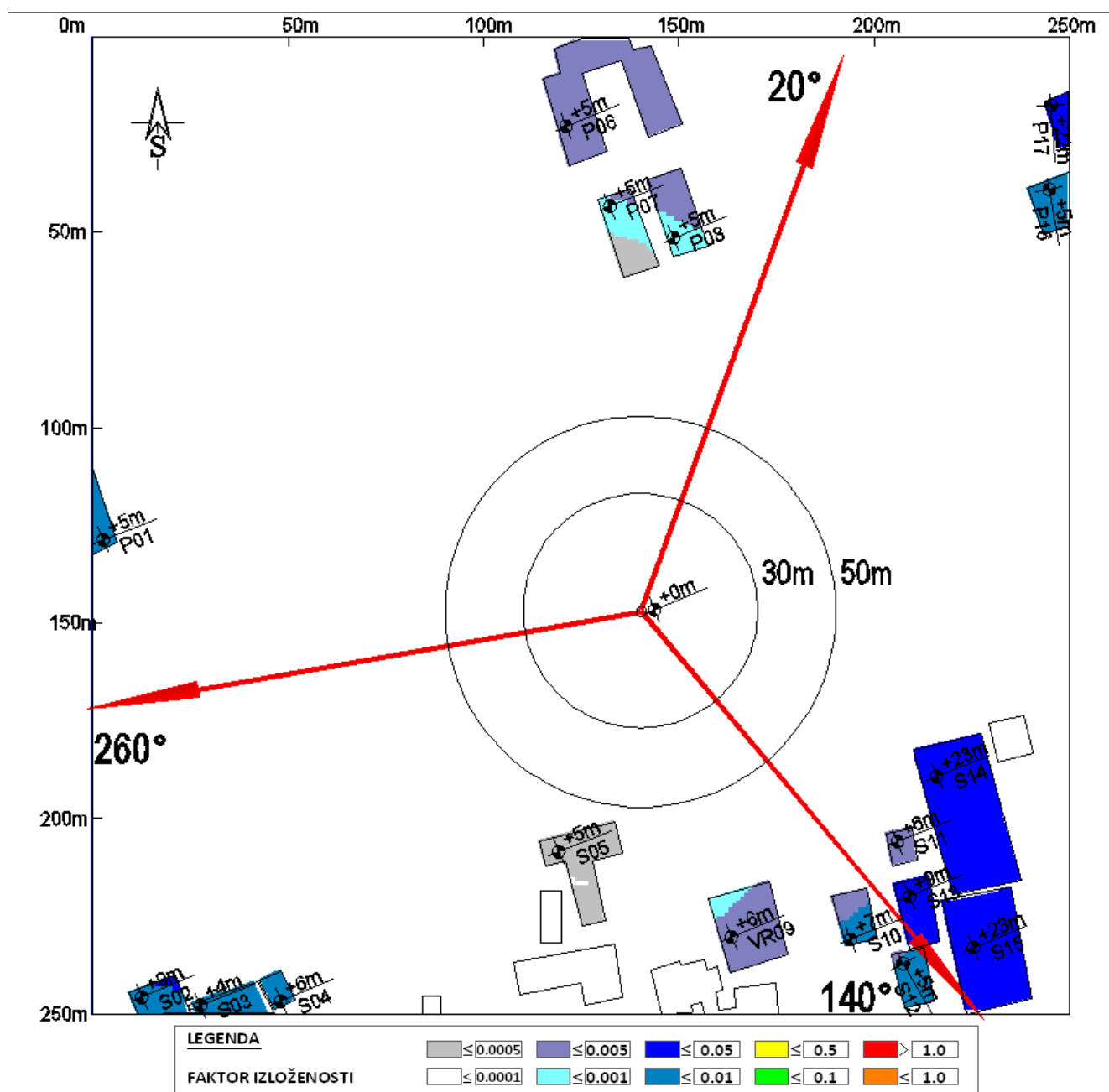
Slika 4.9 Rezultati proračuna faktora izloženosti u objektima na najizloženijim spratovima za slučaj rada sistema GSM900/UMTS2100/LTE2100/LTE1800/LTE800/UMTS900 operatora A1 I CETIN
