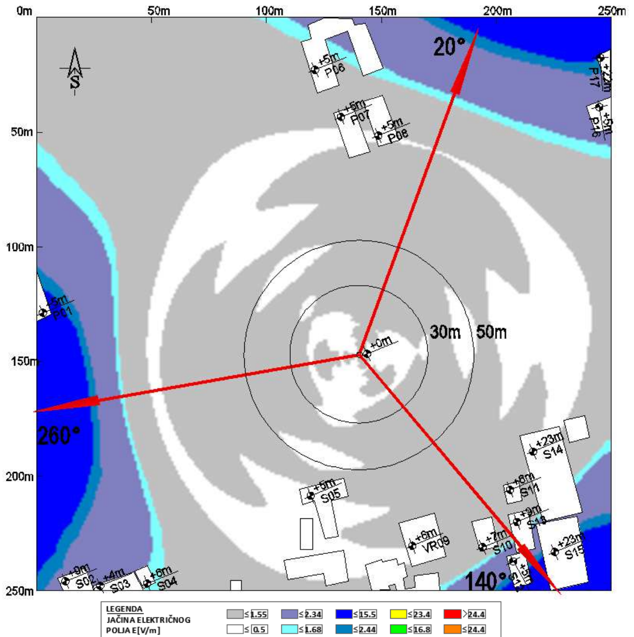
Slika 4.16 Maksimalna proračunata vrednost električnog polja na nivou tla u slučaju rada svih istema na predmetnoj lokaciji operatora A1 iznosi: 2.89 V/m .
