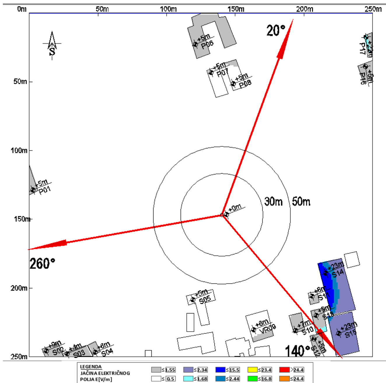
Slika 4.7 Rezultati proračuna jačine električnog polja u objektima na najizloženijim spratovima za slučaj rada sistema GSM900/UMTS2100/LTE2100/LTE1800/LTE800 operatora A1 Srbija
