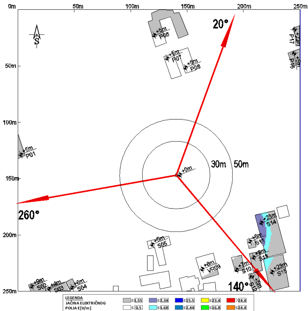
Slika 4.1 Rezultati proračuna jačine električnog polja u objektima na najizloženijim spratovima za slučaj rada sistema GSM900 operatora A1 Srbija
