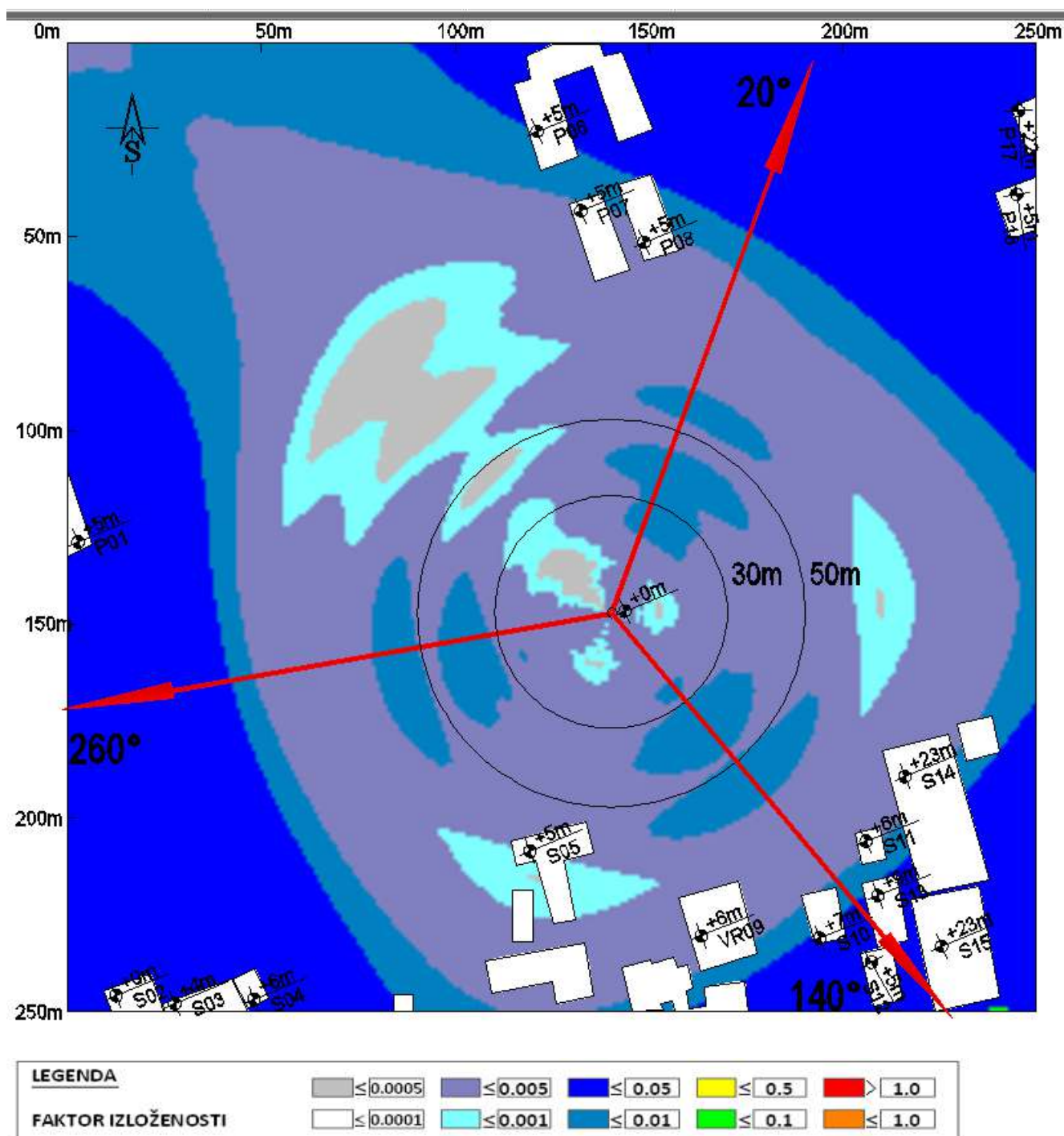
Slika 4.18 Maksimalna proračunata vrednost ukupnog faktora izloženosti na nivou tla u slučaju rada svih sistema na predmetnoj lokaciji operatora A1 I Cetin iznosi: 0.0501 .
