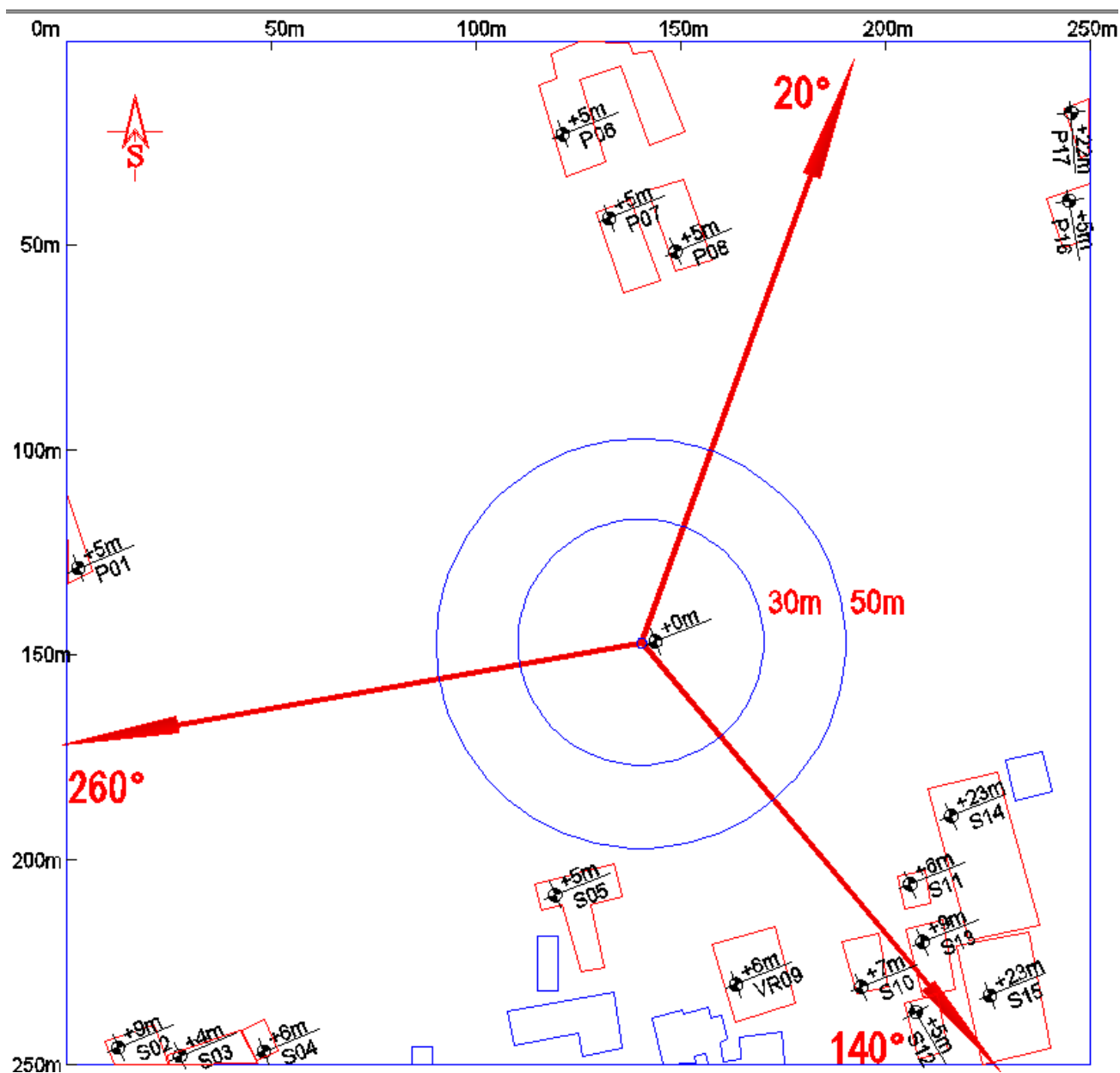
Slika 2.2 Dijagram objekata u okruženju radio bazne stanice "BG0102_01 BG_Zrenjaninski put/Branka Momirova"
