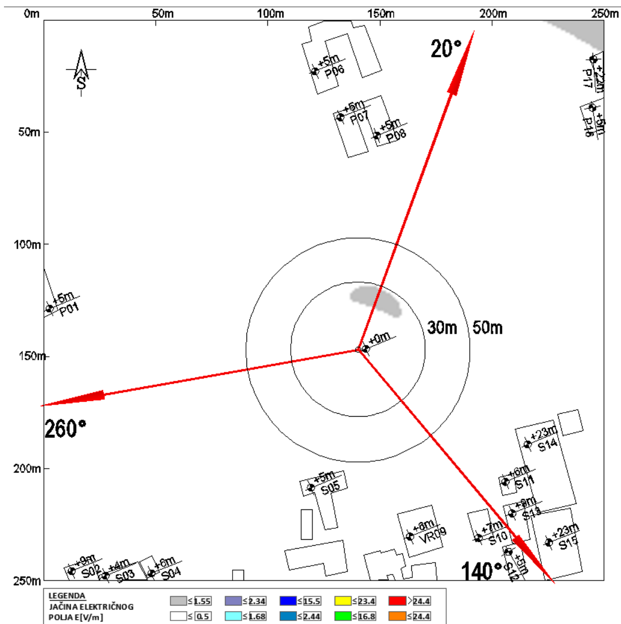
Slika 4.13 Maksimalna proračunata vrednost električnog polja na nivou tla u slučaju rada sistema LTE1800 10MHz operatora A1 iznosi: 0.68 V/m
