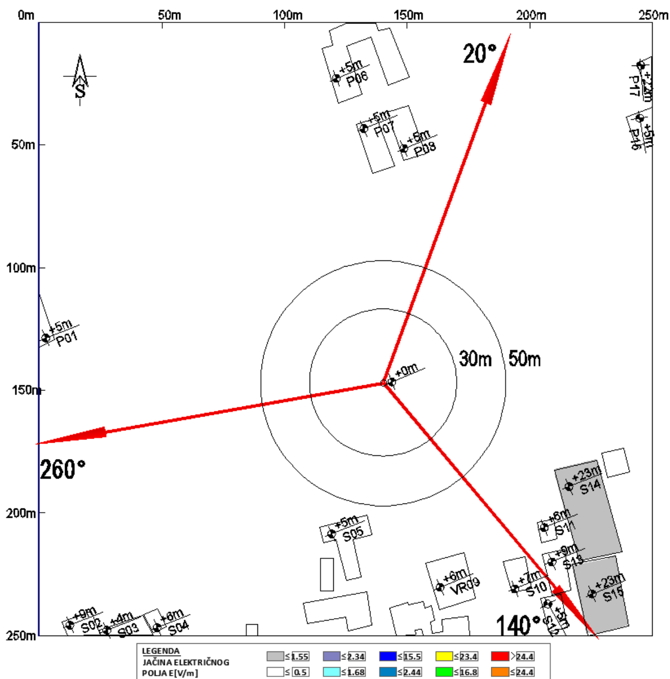
Slika 4.3 Rezultati proračuna jačine električnog polja u objektima na najizloženijim spratovima za slučaj rada sistema LTE2100 operatora A1 Srbija
