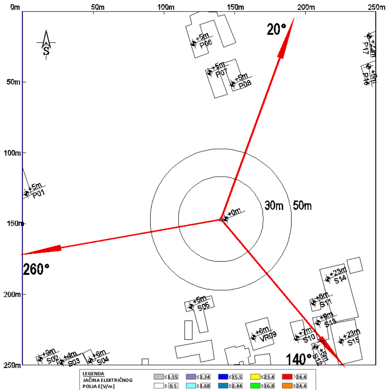
Slika 4.2 Rezultati proračuna jačine električnog polja u objektima na najizloženijim spratovima za slučaj rada sistema UMTS2100 operatora A1 Srbija
