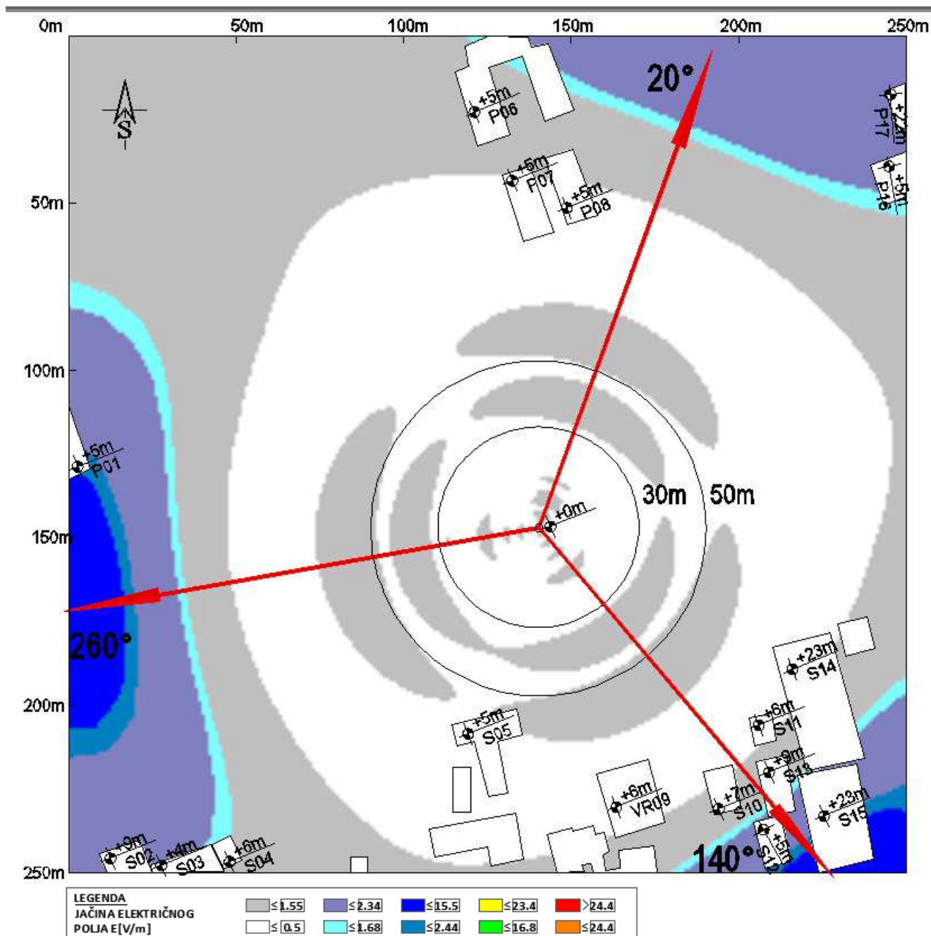
Slika 4.10 Maksimalna proračunata vrednost električnog polja na nivou tla u slučaju rada sistema GSM900 operatora A1 iznosi: 2.69 V/m
