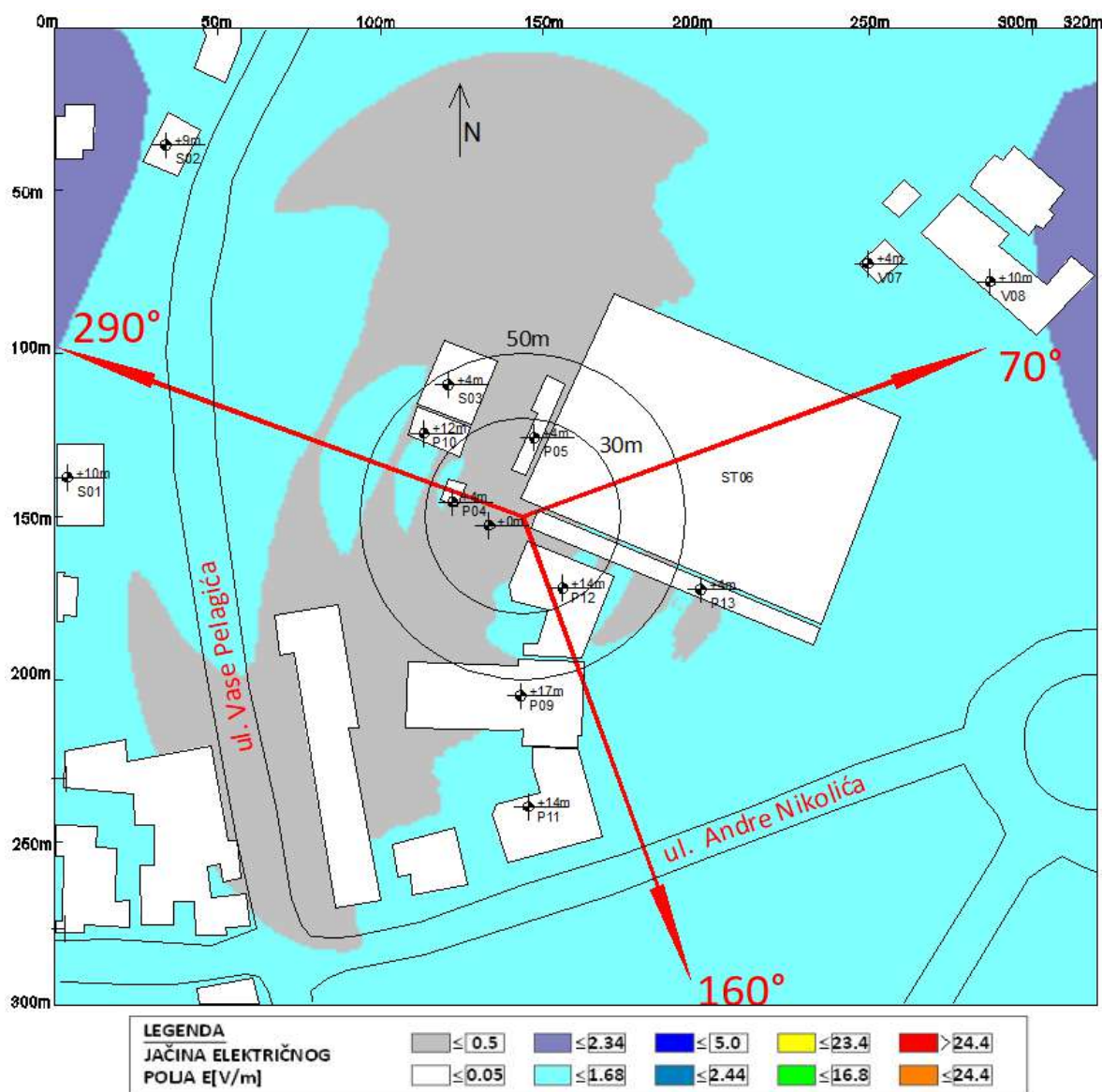
Slika 6.15 Rezultati proračuna jačine električnog polja u široj okolini lokacije bazne stanice na visini +1.70m (prosečna visina čoveka) u odnosu na nivo tla za slučaj rada svih sistema operatora A1 . Maksimalna proračunata vrednost jačine električnog polja iznosi E=2.11 V/m.
