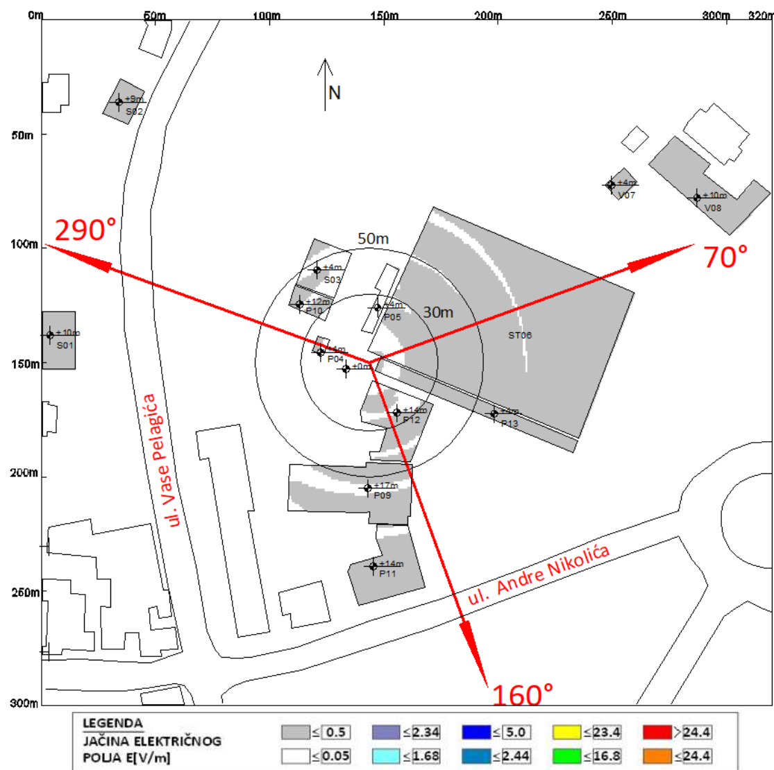
Slika 6.3 Rezultati proračuna jačine električnog polja u objektima na najizloženijim spratovima za slučaj rada sistema LTE2100 operatora A1 Srbija
