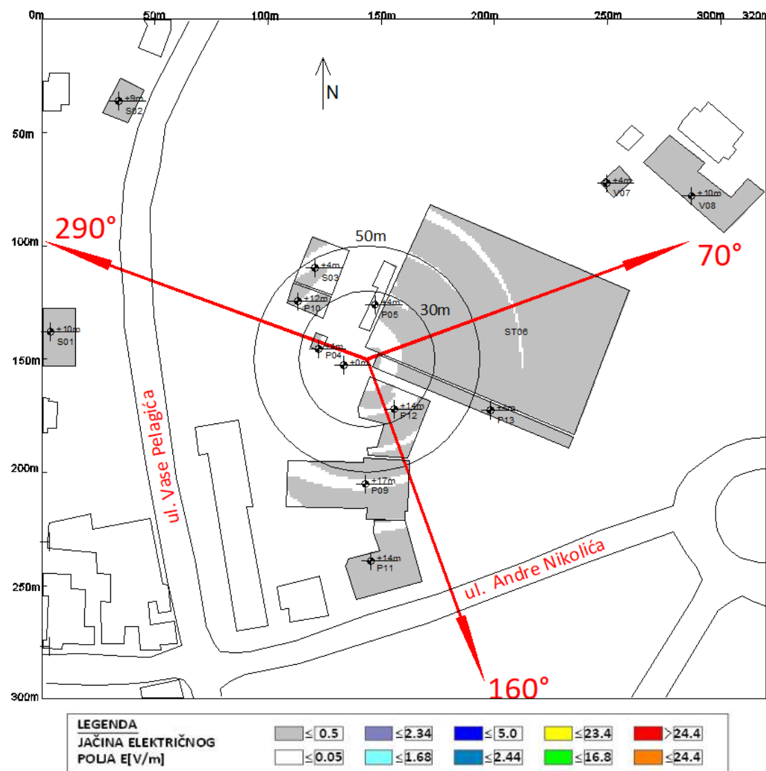
Slika 6.2 Rezultati proračuna jačine električnog polja u objektima na najizloženijim spratovima za slučaj rada sistema UMTS2100 operatora A1 Srbija
