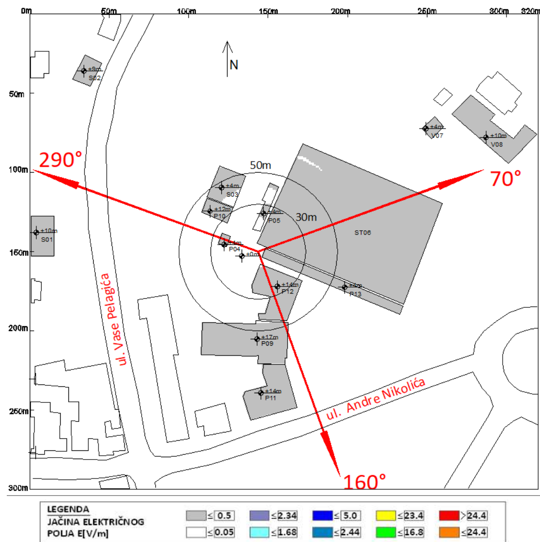
Slika 6.6 Rezultati proračuna jačine električnog polja u objektima na najizloženijim spratovima za slučaj rada sistema LTE800 operatora A1 Srbija
