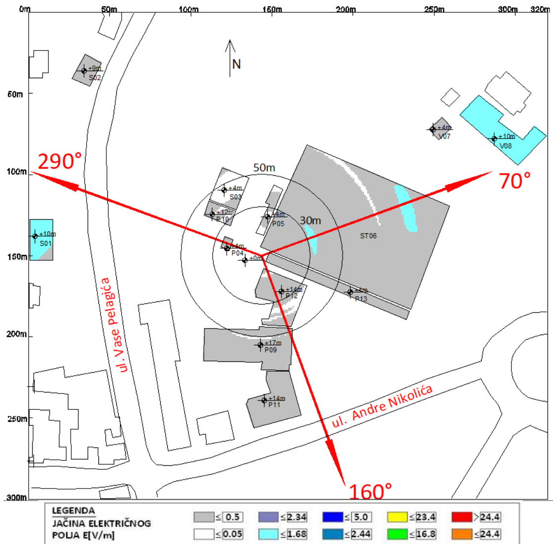
Slika 6.1 Rezultati proračuna jačine električnog polja u objektima na najizloženijim spratovima za slučaj rada sistema GSM900 operatora A1 Srbija
