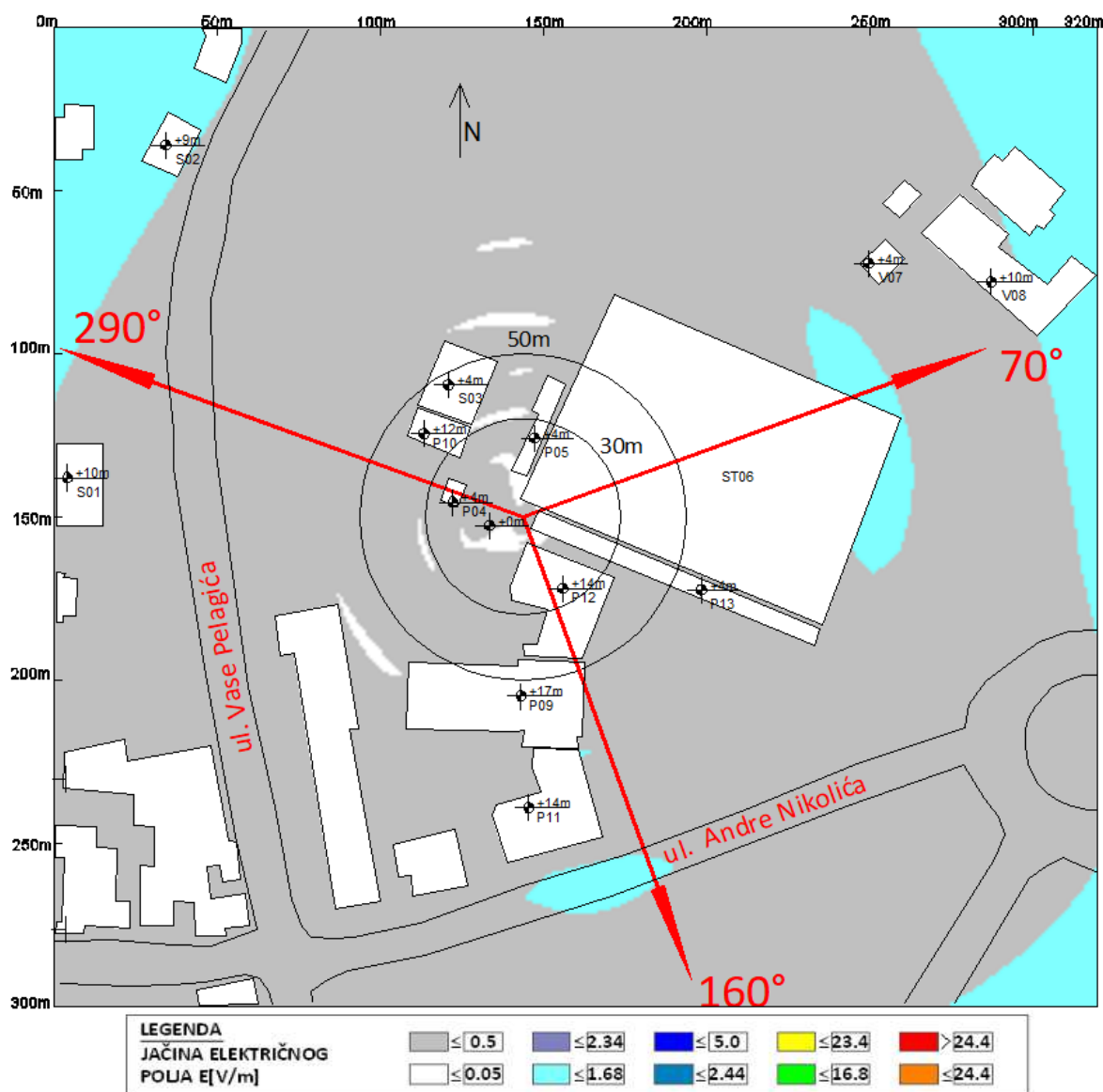
Slika 6.12 Maksimalna proračunata vrednost električnog polja na nivou tla u slučaju rada sistema LTE1800 (10MHZ) operatora A1 Srbija iznosi: 0.87 V/m
