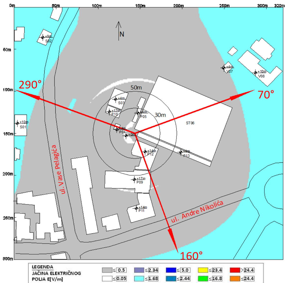
Slika 6.14 Maksimalna proračunata vrednost jačine električnog polja na nivou tla u slučaju rada sistema LTE800 na predmetnoj lokaciji operatora A1 Srbija iznosi: 0,83 V/m
