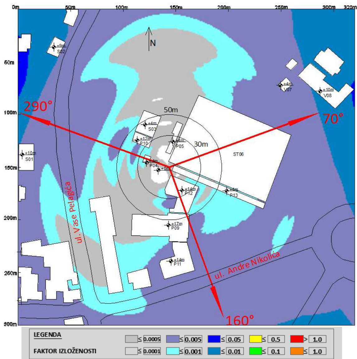
Slika 6.16 Rezultati proračuna faktora izloženosti u široj okolini lokacije bazne stanice na visini +1.70m (prosečna visina čoveka) u odnosu na nivo tla za slučaj rada svih sistema operatora A1 . Maksimalna proračunata vrednost faktora izloženosti iznosi FI=0.0115 .
