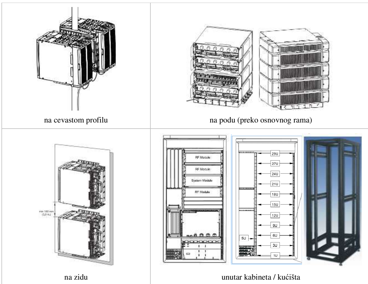
Slika 3.5 Mogući scenariji montaže Flexi modula
