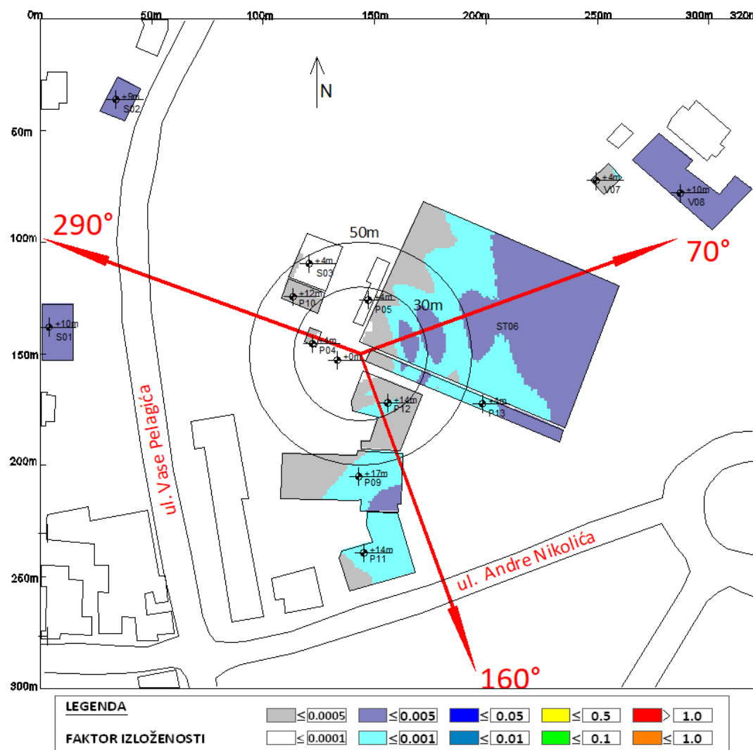
Slika 6.8 Rezultati proračuna faktora izloženosti u objektima na najizloženijim spratovima za slučaj rada svih sistema operatora A1
