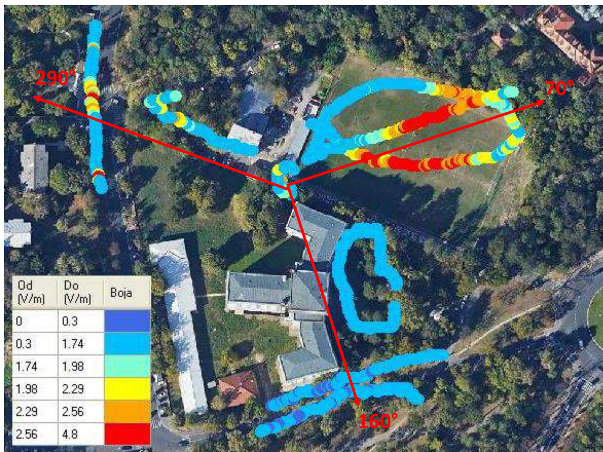
Prostorna raspodela polja u okolini antenskog sistema
