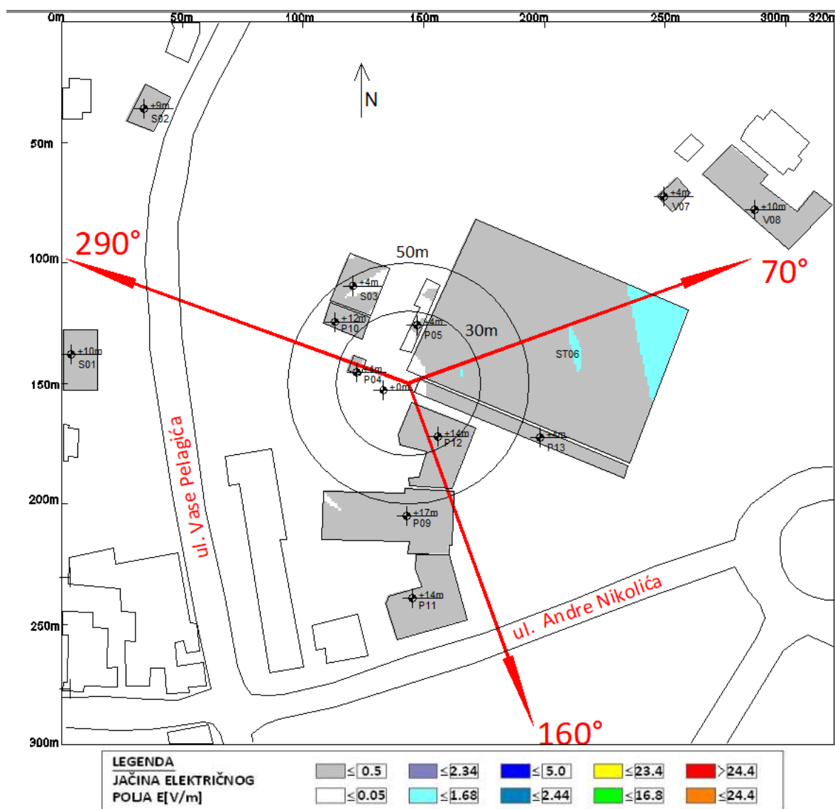
Slika 6.5 Rezultati proračuna jačine električnog polja u objektima na najizloženijim spratovima za slučaj rada sistema LTE1800 (20MHZ) operatora A1 Srbija
