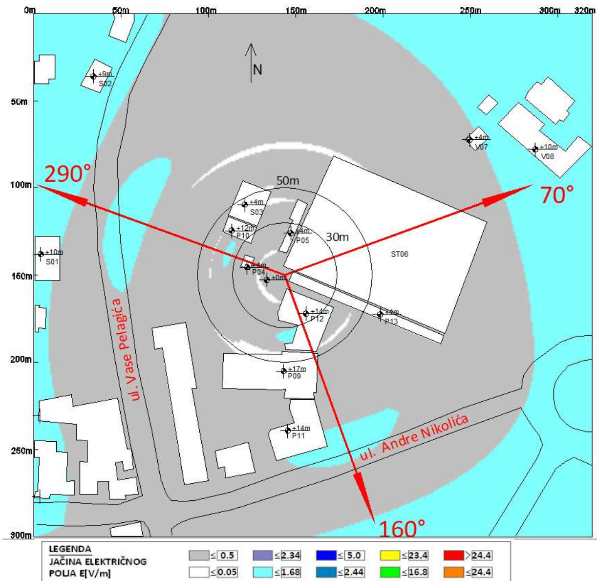
Slika 6.9 Maksimalna proračunata vrednost električnog polja na nivou tla u slučaju rada sistema GSM900 operatora A1 Srbija iznosi: 1.14 V/m
