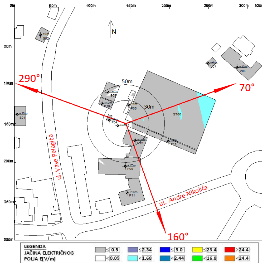
Slika 6.4 Rezultati proračuna jačine električnog polja u objektima na najizloženijim spratovima za slučaj rada sistema LTE1800 (10MHZ) operatora A1 Srbija
