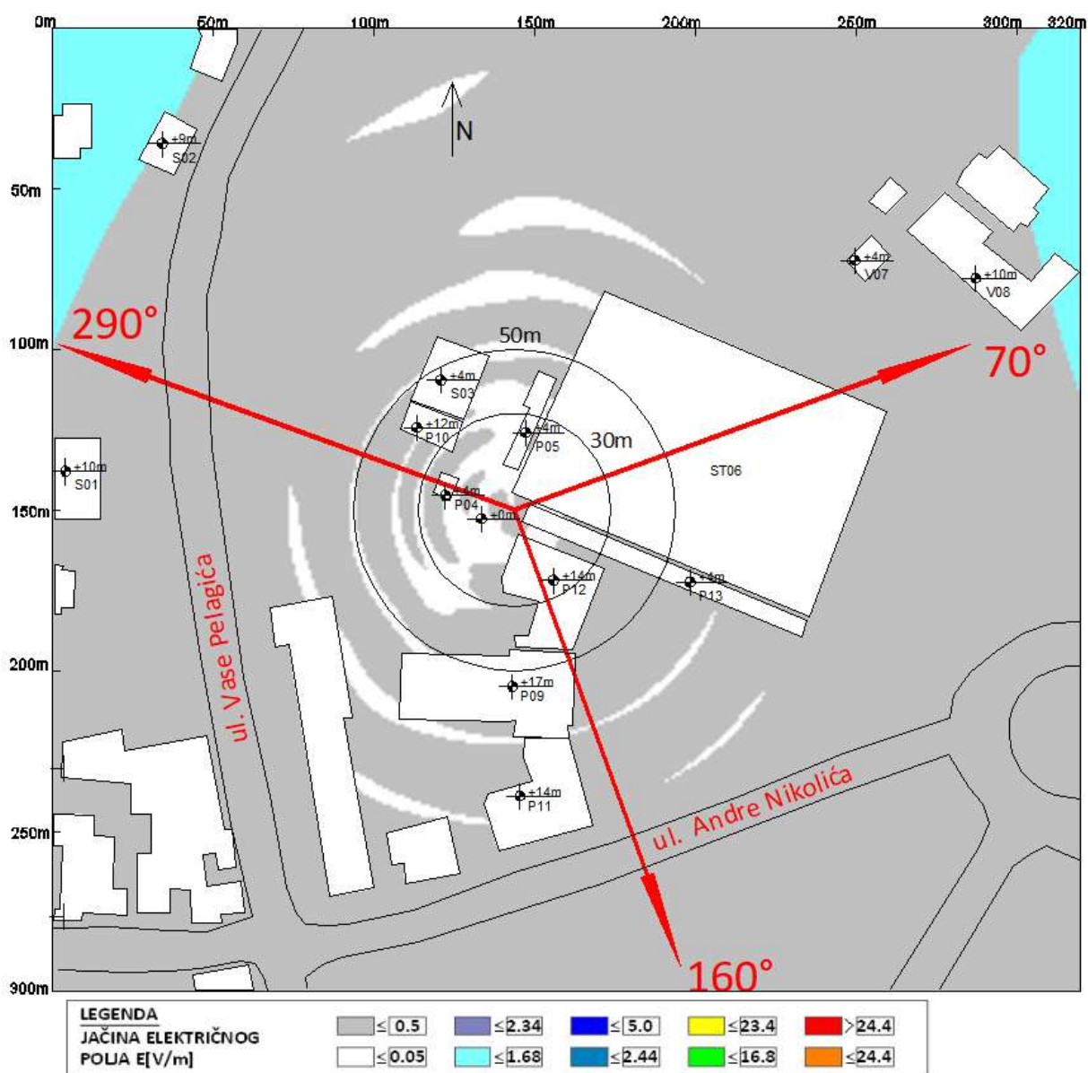
Slika 6.10 Maksimalna proračunata vrednost električnog polja na nivou tla u slučaju rada sistema UMTS2100 operatora A1 Srbija iznosi: 0.73 V/m
