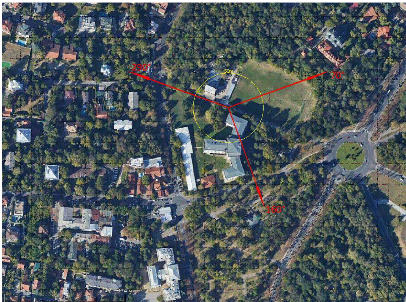
Slika 2.1 Dijagram zračenja radio bazne stanice „BG0916_01 BG_FK_Graficar“
