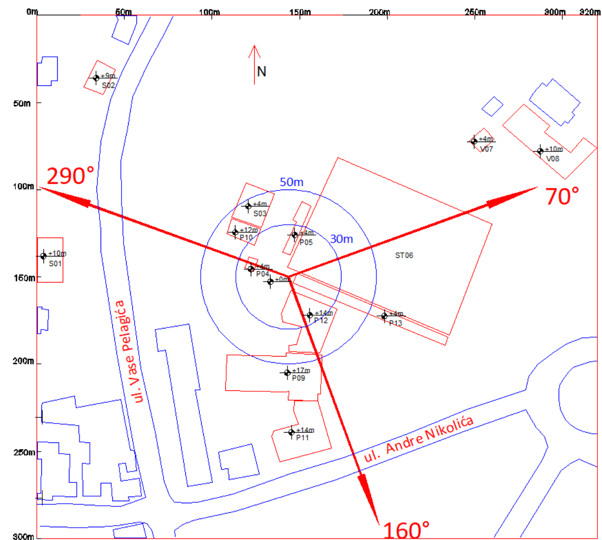
Slika 5.2 Dijagram objekata u okruženju radio bazne «BG0916_01 BG_FK_Graficar»
