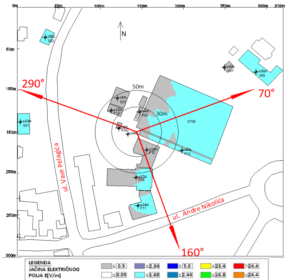
Slika 6.7 Rezultati proračuna jačine električnog polja u objektima na najizloženijim spratovima za slučaj rada svih sistema operatora A1
