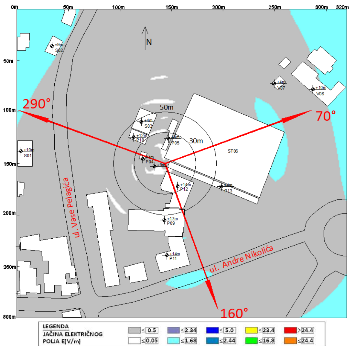
Slika 6.13 Maksimalna proračunata vrednost električnog polja na nivou tla u slučaju rada sistema LTE1800 (20MHZ) operatora A1 Srbija iznosi: 0.87 V/m
