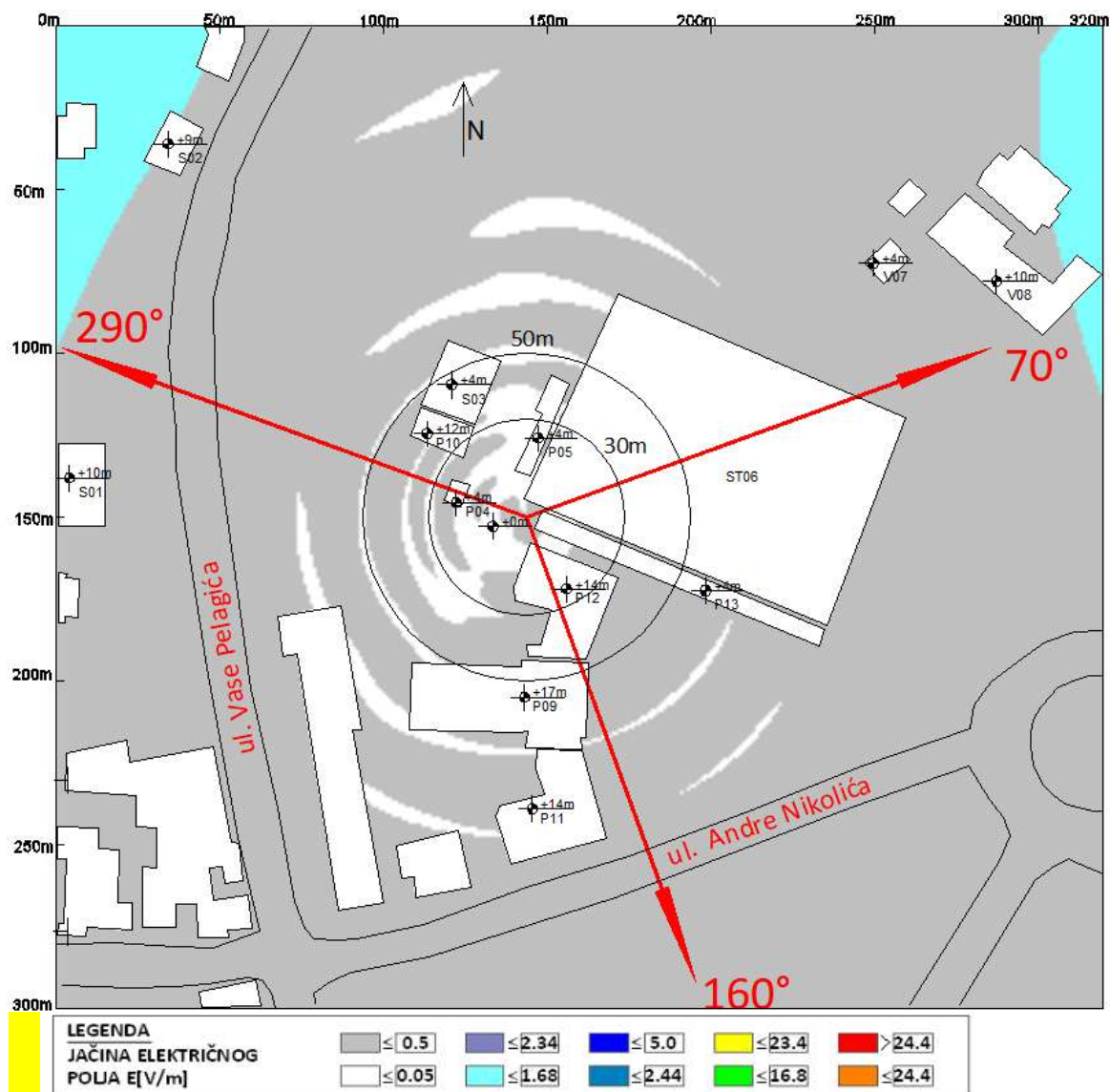
Slika 6.11 Maksimalna proračunata vrednost električnog polja na nivou tla u slučaju rada sistema LTE2100 operatora A1 Srbija iznosi: 0.73 V/m
