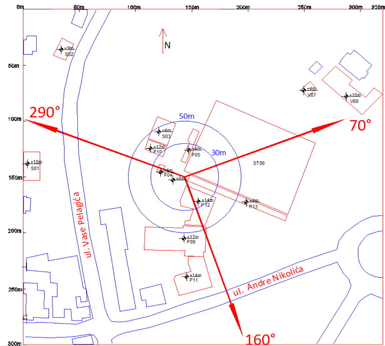
Slika 2.2 Dijagram objekata u okruženju radio bazne stanice „BG0916_01 BG_FK_Graficar“
