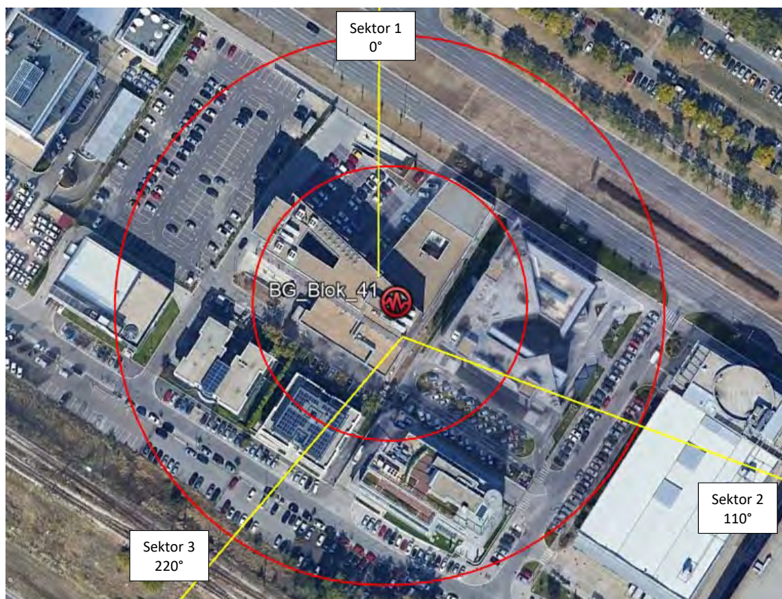
Slika 2.9 Pravci zračenja antenskih sistema predmetne bazne stanice
