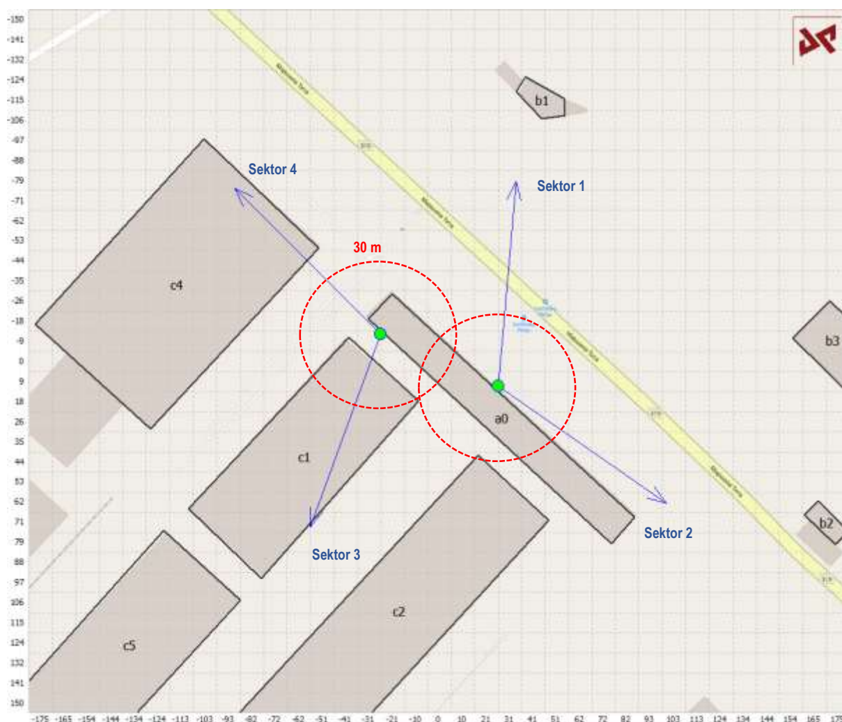
Slika 2.6 Prikaz pravaca zračenja antena i pozicije okolnih objekata
