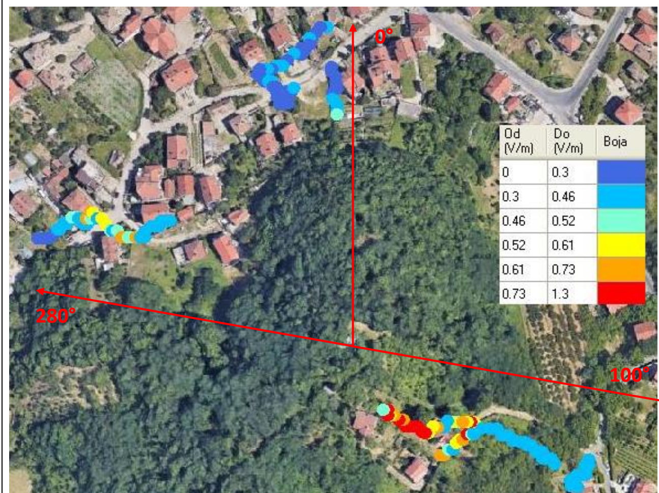
Prostorna raspodela polja u okolini antenskog sistema
