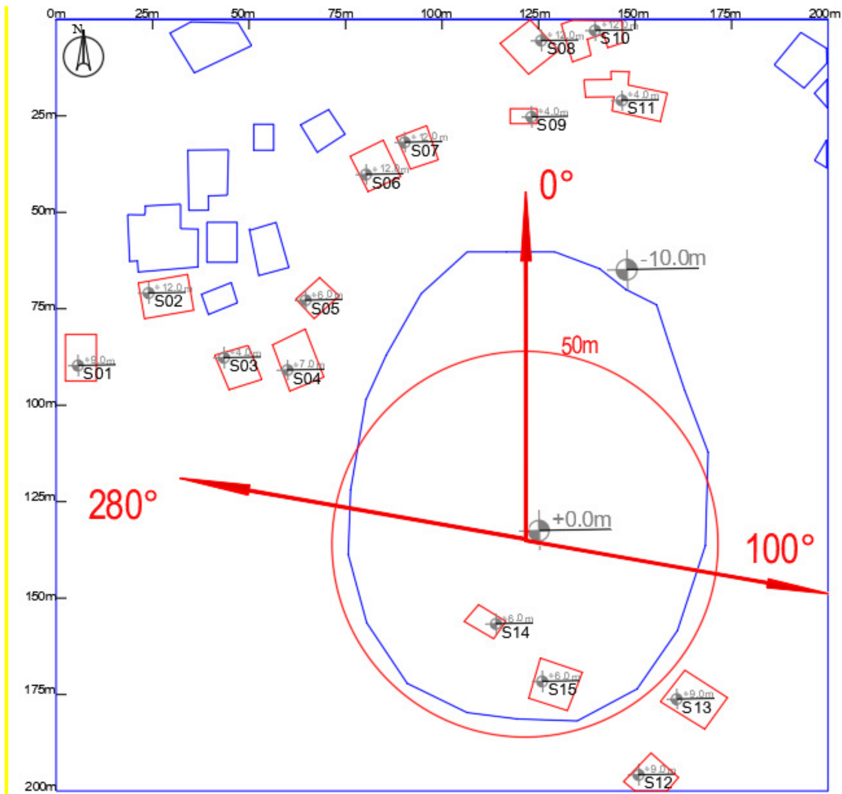
Slika 2.2 Dijagram objekata u okruženju radio bazne stanice „BG - Kaluđerica 3” - BG560/BGU560/BGL560/BGO560/BGJ560
