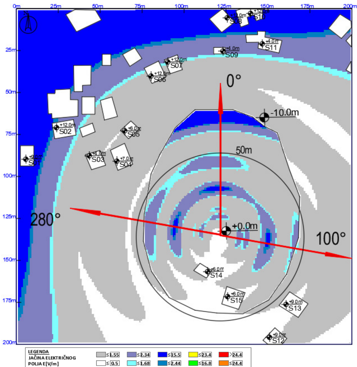
Slika 6.14 Maksimalna proračunata vrednost električnog polja na nivou tla u slučaju rada svih sistema na predmetnoj lokaciji operatora Telekom iznosi: 3.83 V/m .
