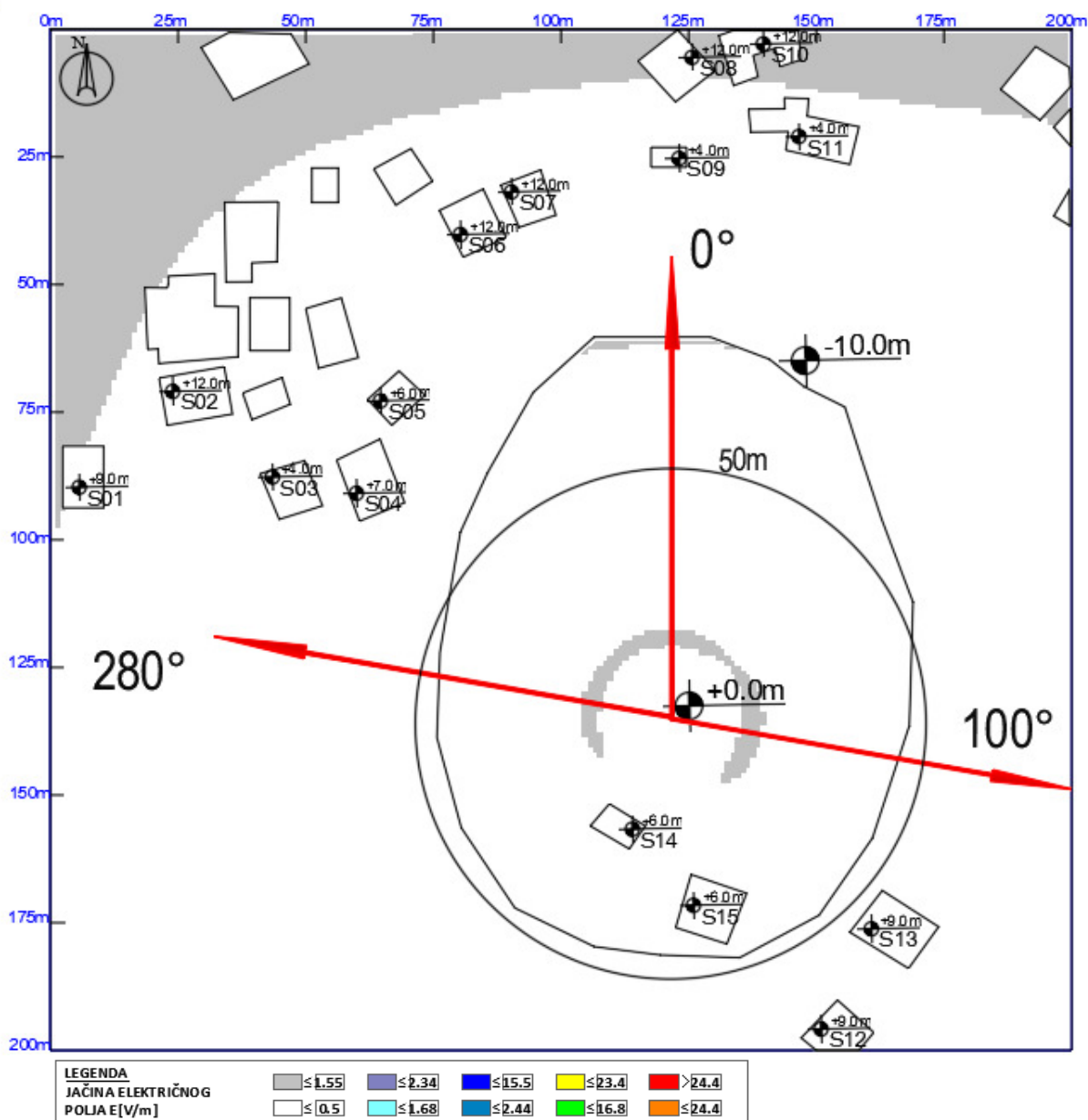
Slika 6.13 Maksimalna proračunata vrednost električnog polja na nivou tla u slučaju rada sistema LTE2100 operatora Telekom iznosi: 0.99 V/m
