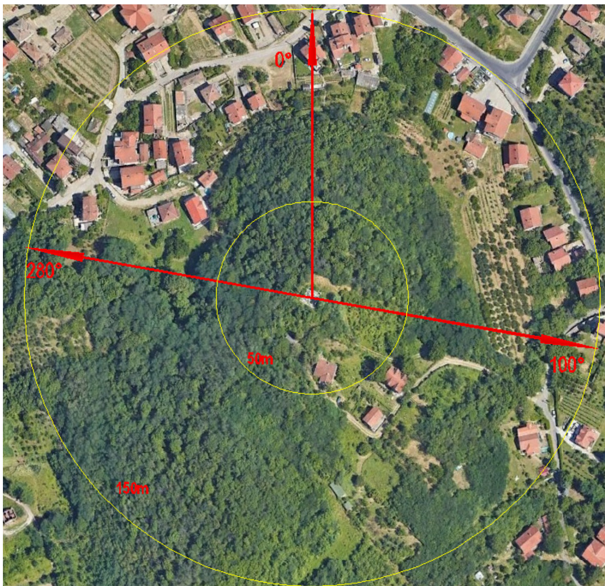
Slika 2.1 Dijagram zračenja radio bazne stanice „BG - Kaluđerica 3” - BG560/BGU560/BGL560/BGO560/BGJ560
