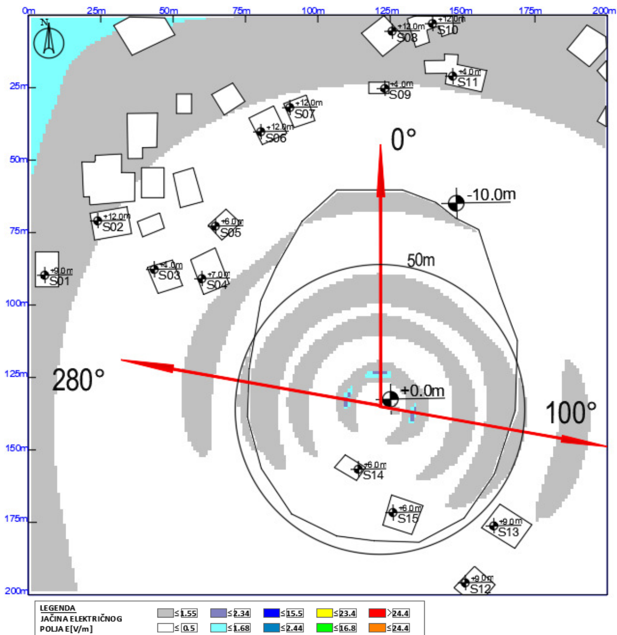
Slika 6.11 Maksimalna proračunata vrednost električnog polja na nivou tla u slučaju rada sistema LTE1800 operatora Telekom iznosi: 1.77 V/m
