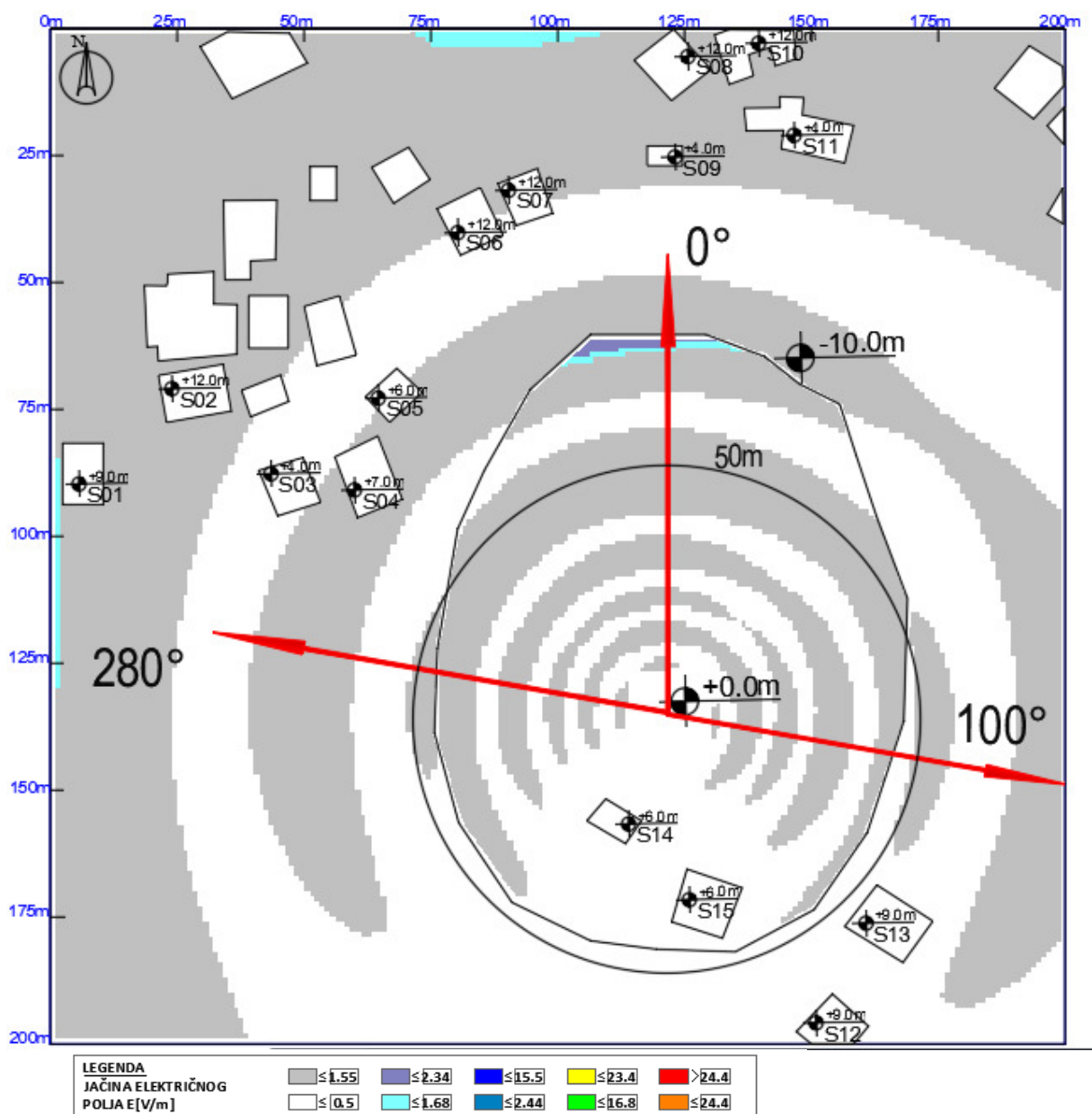
Slika 6.9 Maksimalna proračunata vrednost električnog polja na nivou tla u slučaju rada sistema GSM900 operatora Telekom iznosi: 1.93 V/m
