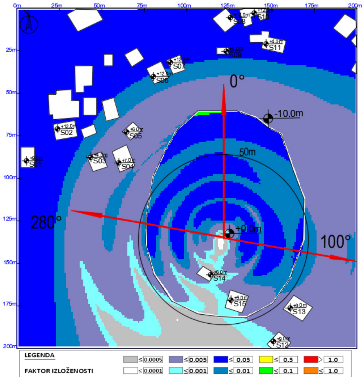
Slika 6.16 Maksimalna proračunata vrednost ukupnog faktora izloženosti na nivou tla u slučaju rada svih sistema na predmetnoj lokaciji operatora Telekom i A1 SRBIJA iznosi: 0.0552 .
