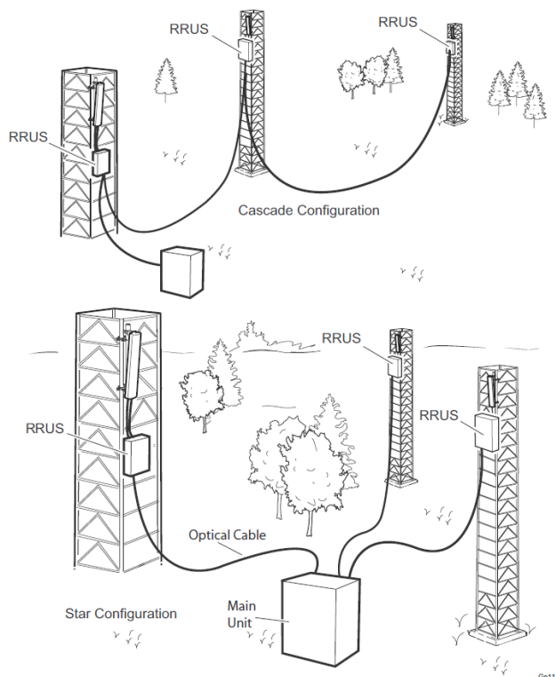
Slika 10.4 Povezivanje BS 6601 sa RRUS jedinicama
