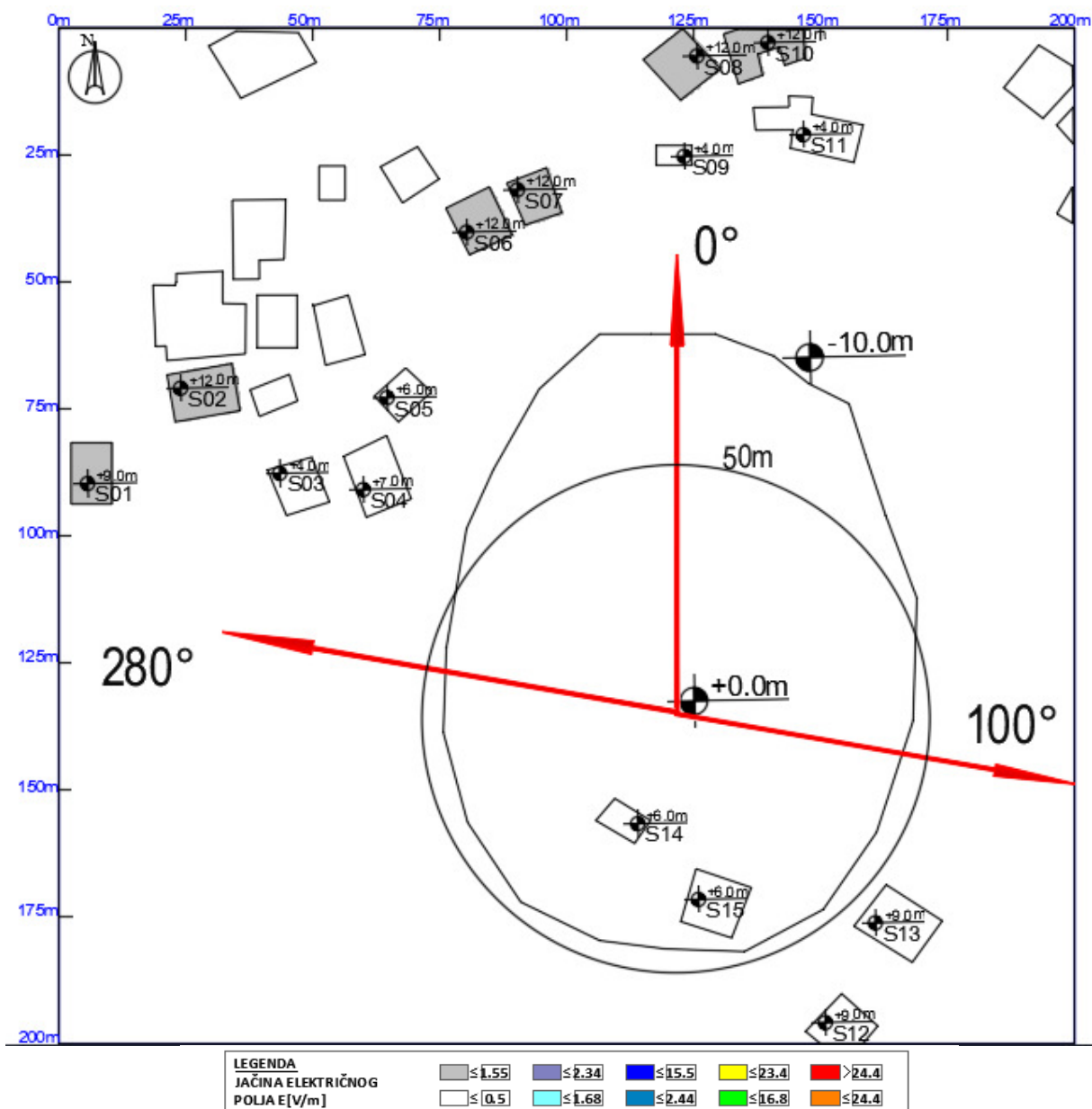
Slika 6.3 Rezultati proračuna jačine električnog polja u objektima na najizloženijim spratovima za slučaj rada sistema LTE1800 operatora Telekom Srbija
