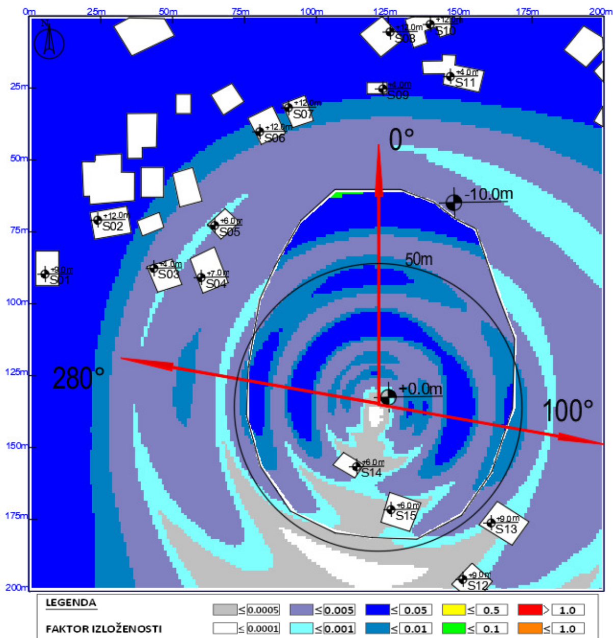
Slika 6.15 Maksimalna proračunata vrednost ukupnog faktora izloženosti na nivou tla u slučaju rada svih sistema na predmetnoj lokaciji operatora Telekom iznosi: 0.0533 .
