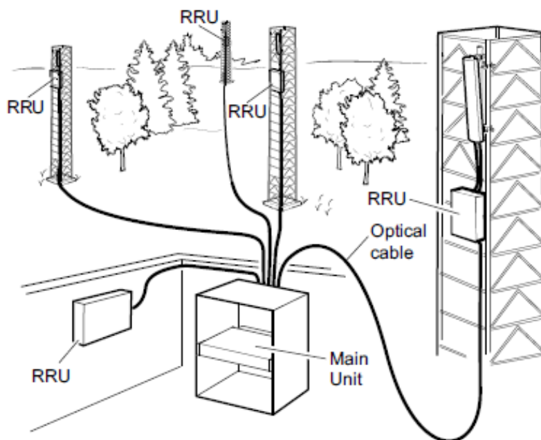
Slika 10.1 RBS6601, centralna jedinica i RRU
