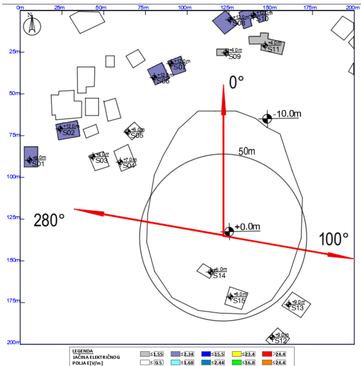
Slika 6.7 Rezultati proračuna jačine električnog polja u objektima na najizloženijim spratovima za slučaj rada svih sistema operatora Telekom
