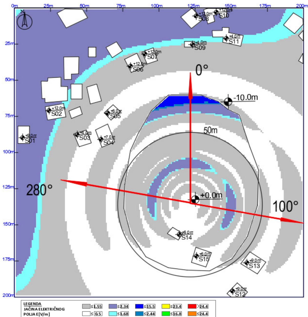
Slika 6.12 Maksimalna proračunata vrednost električnog polja na nivou tla u slučaju rada sistema LTE800 operatora Telekom iznosi: 2.93 V/m
