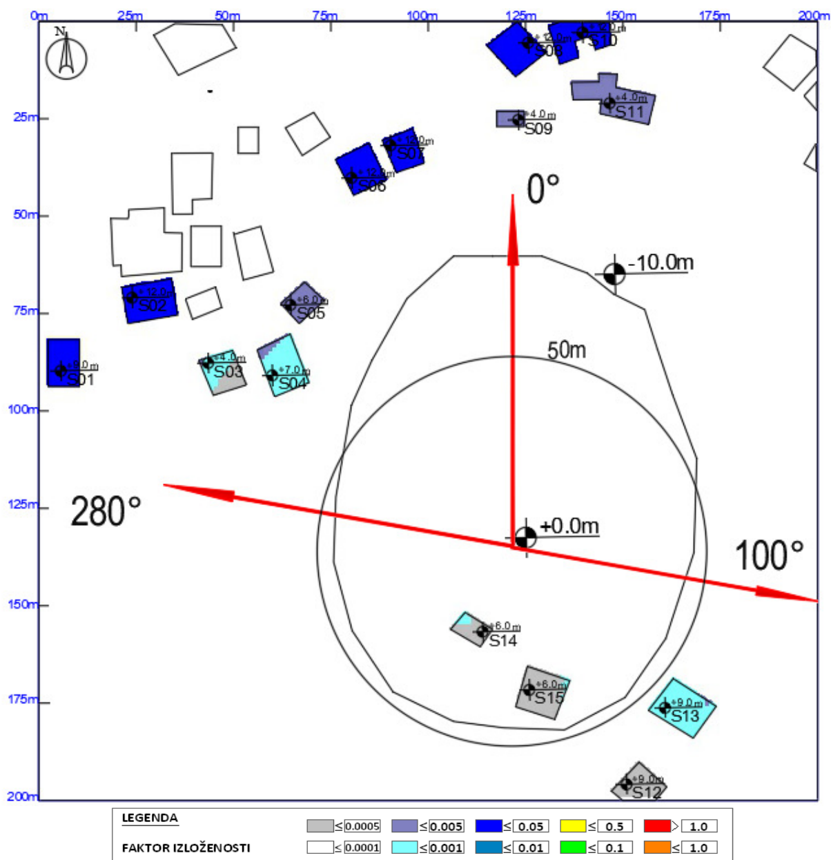
Slika 6.8 Rezultati proračuna faktora izloženosti u objektima na najizloženijim spratovima za slučaj rada svih sistema operatora Telekom i A1
