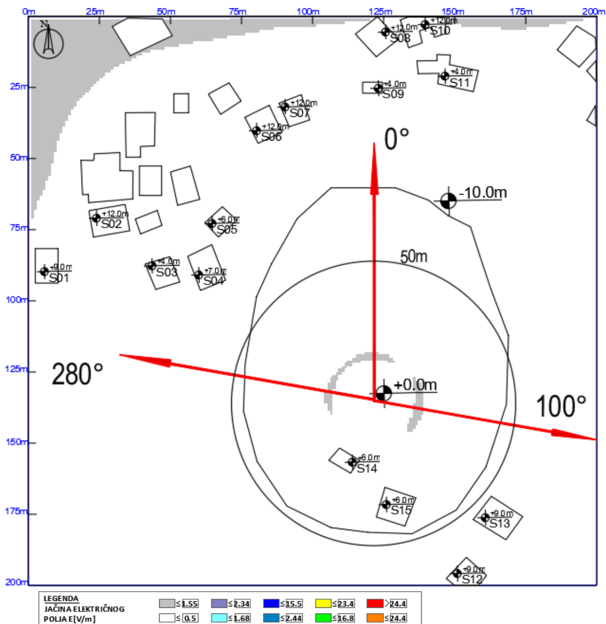
Slika 6.10 Maksimalna proračunata vrednost električnog polja na nivou tla u slučaju rada sistema UMTS2100 operatora Telekom iznosi: 0.76 V/m
