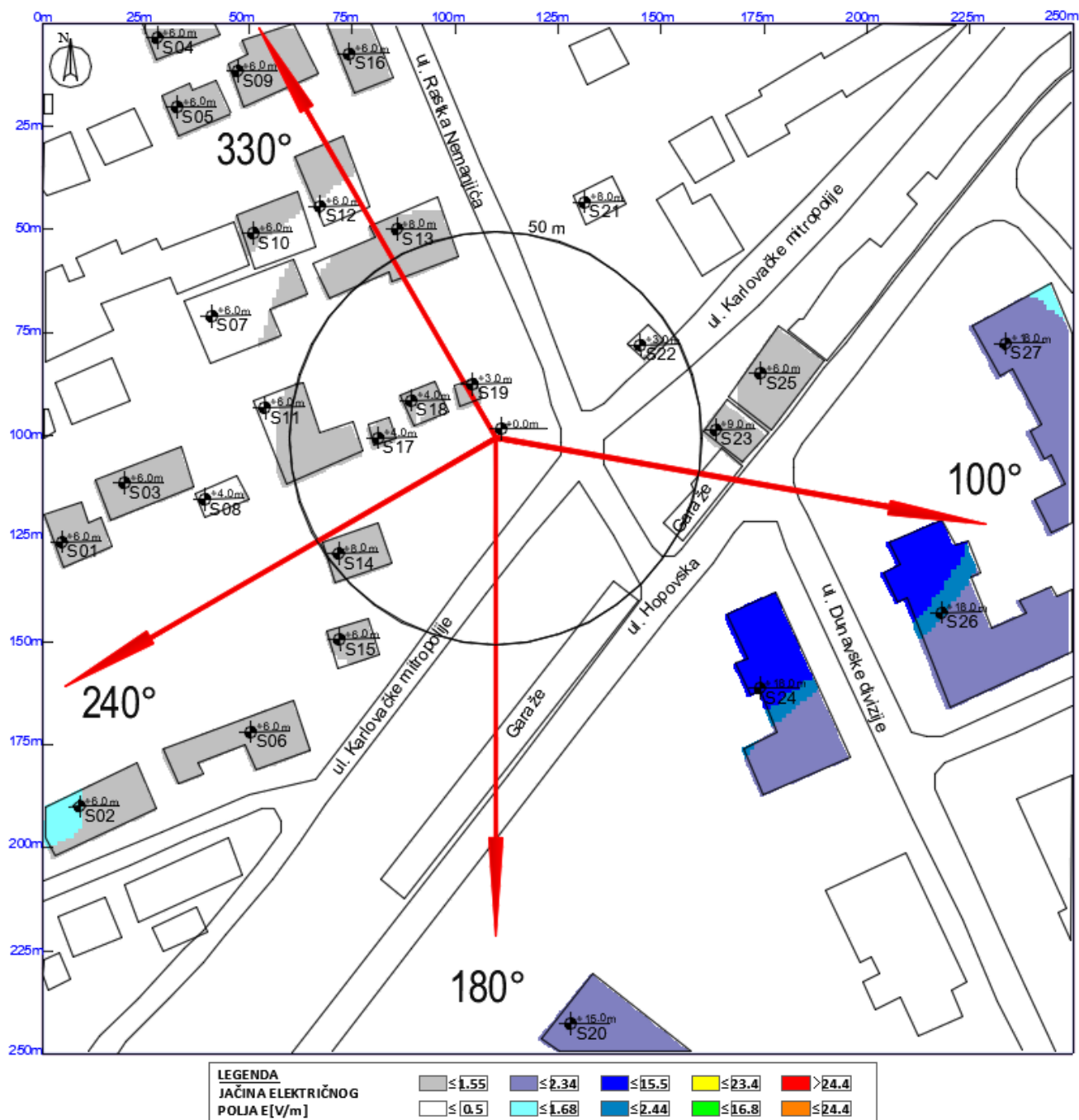
Slika 6.7 Rezultati proračuna jačine električnog polja u objektima na najizloženijim spratovima za slučaj rada svih sistema operatora Telekom
