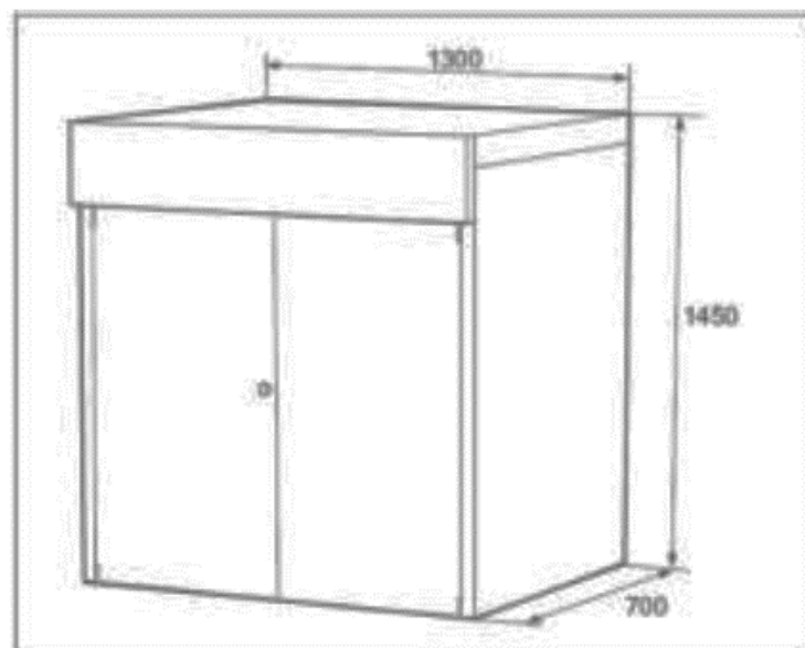
Slika 10.2 Dimenzije RBS6101
