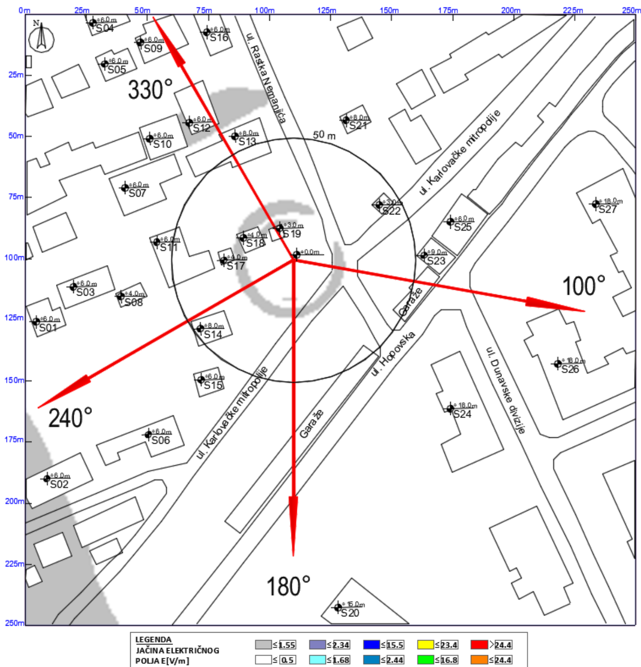
Slika 6.10 Maksimalna proračunata vrednost električnog polja na nivou tla u slučaju rada sistema UMTS2100 operatora Telekom iznosi: 1.33 V/m
