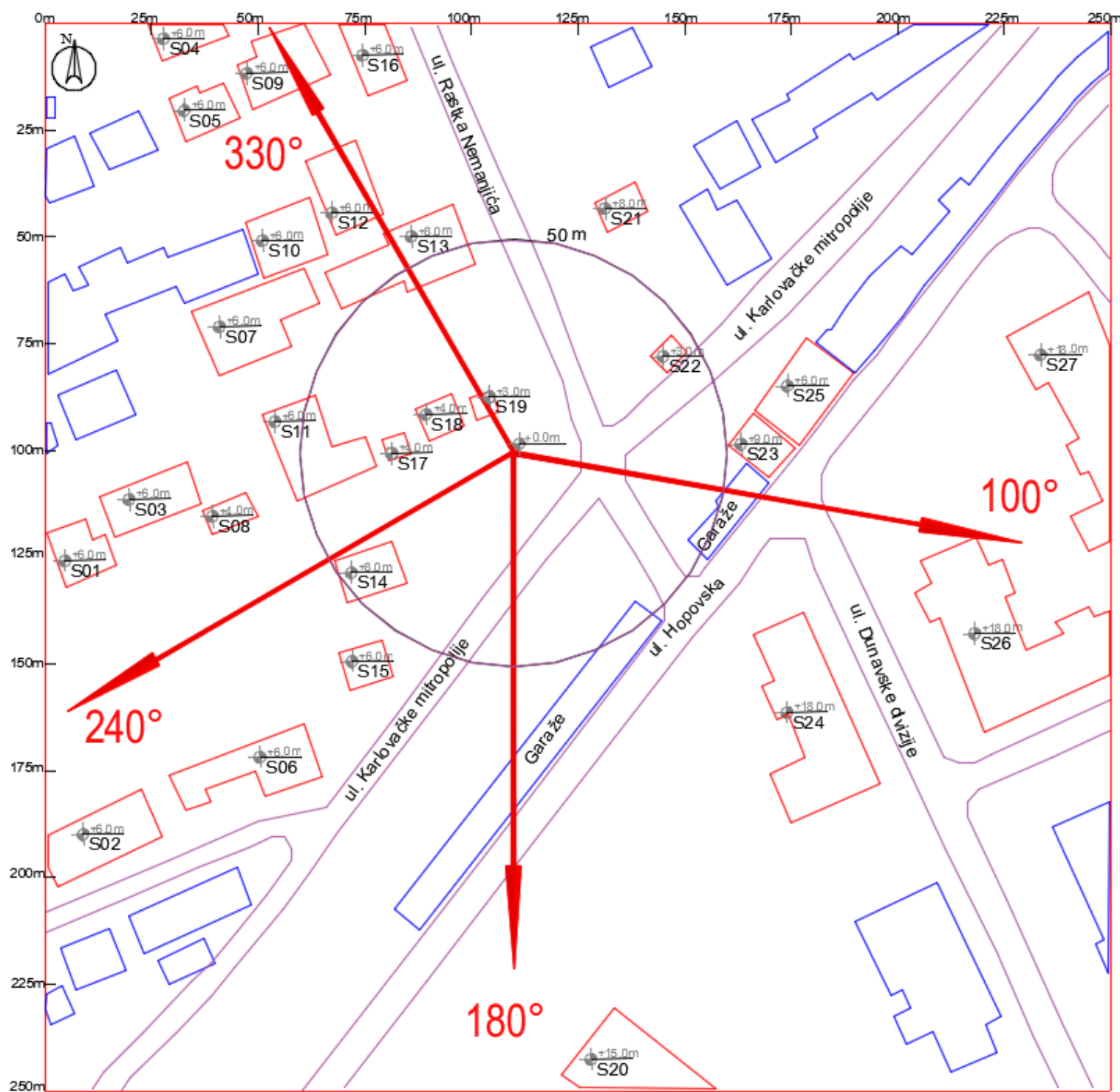
Slika 2.2 Dijagram objekata u okruženju radio bazne stanice „BG - Borca Greda“ - BG589/BGU589/BGL589/BGO589/BGJ589
