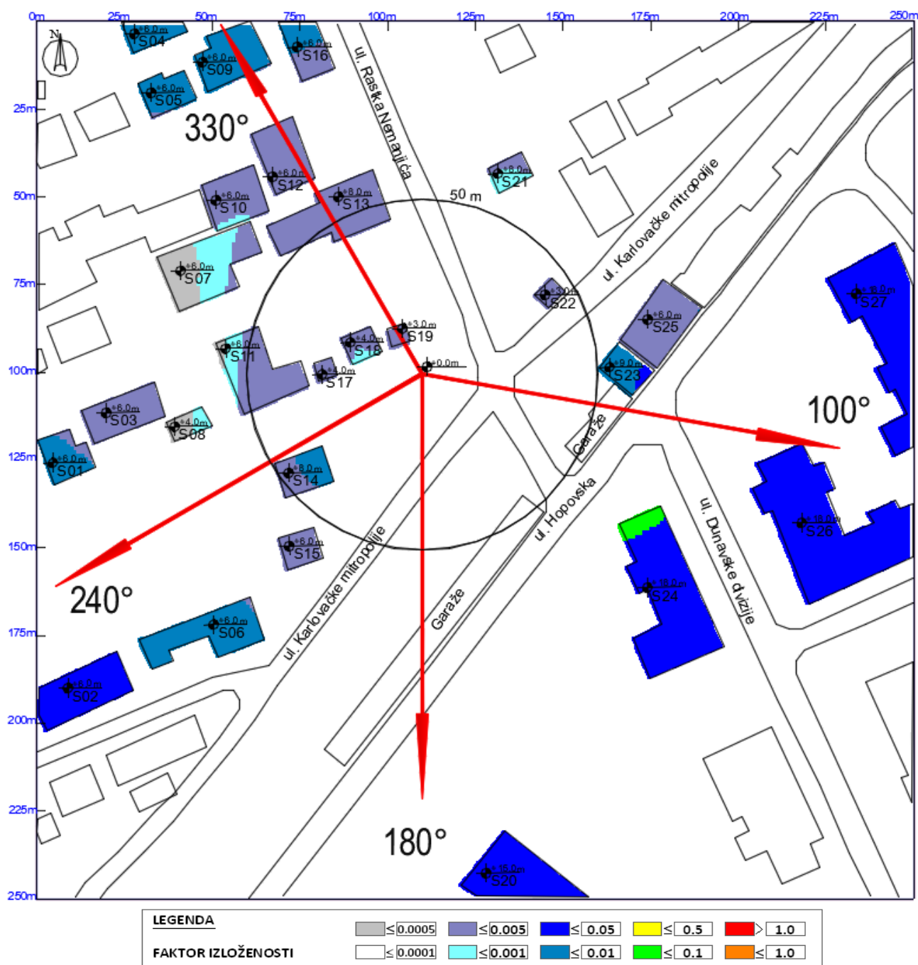
Slika 6.8 Rezultati proračuna faktora izloženosti u objektima na najizloženijim spratovima za slučaj rada svih sistema operatora Telekom, Yettel i A1
