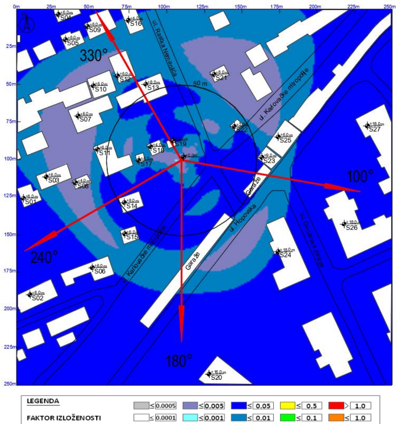
Slika 6.16 Maksimalna proračunata vrednost ukupnog faktora izloženosti na nivou tla u slučaju rada svih sistema na predmetnoj lokaciji operatora Telekom, Yettel i A1 SRBIJA mobile iznosi: 0.0421 .
