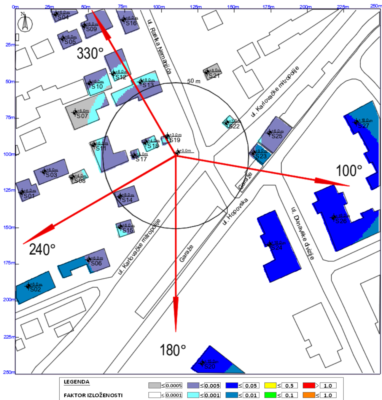
Slika 6.6 Rezultati proračuna faktora izloženosti u objektima na najizloženijim spratovima za slučaj rada sistema GSM900/UMTS2100/LTE1800/LTE800/LTE2100 operatora Telekom Srbija
