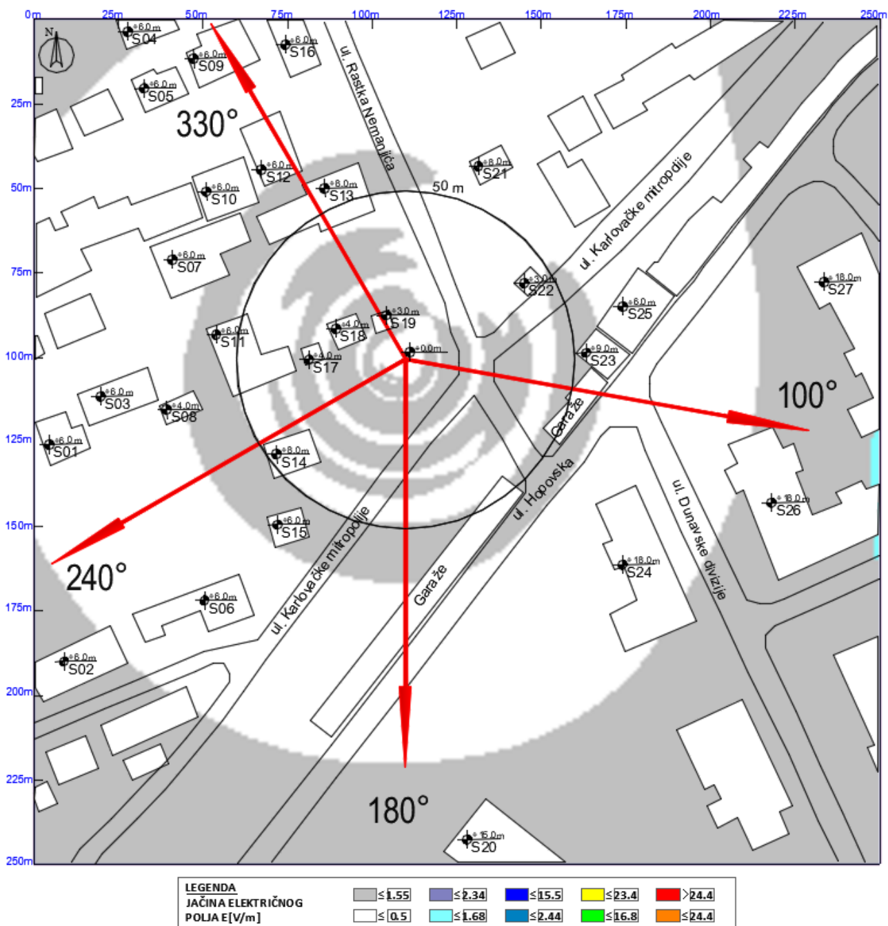
Slika 6.11 Maksimalna proračunata vrednost električnog polja na nivou tla u slučaju rada sistema LTE1800 operatora Telekom iznosi: 1.56 V/m
