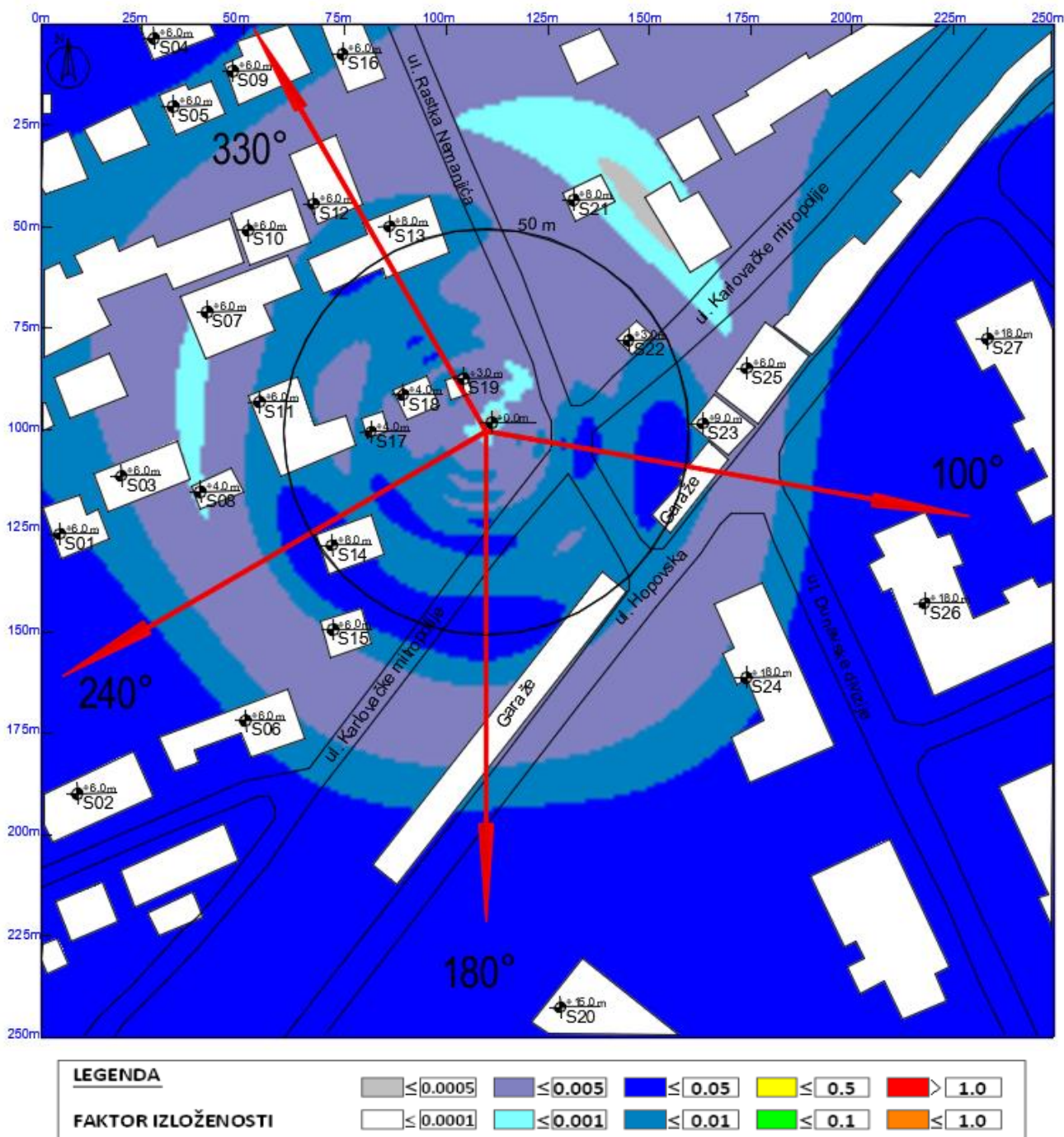
Slika 6.15 Maksimalna proračunata vrednost ukupnog faktora izloženosti na nivou tla u slučaju rada svih sistema na predmetnoj lokaciji operatora Telekom iznosi: 0.0276 .
