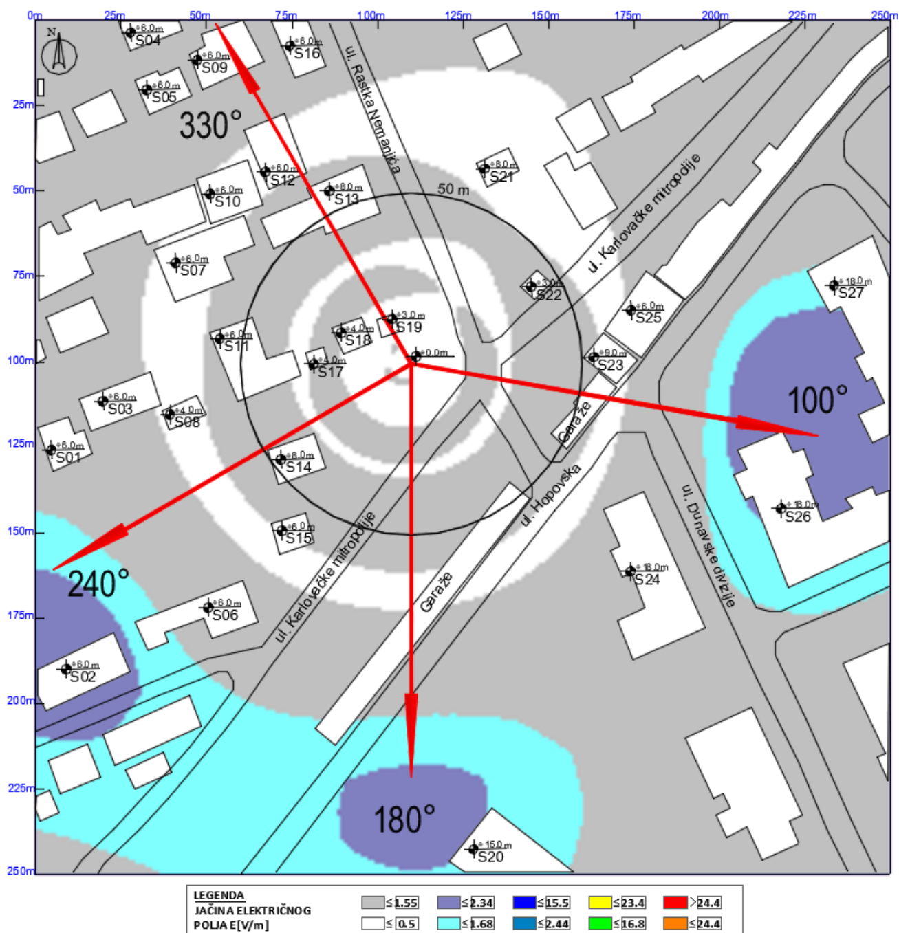
Slika 6.12 Maksimalna proračunata vrednost električnog polja na nivou tla u slučaju rada sistema LTE800 operatora Telekom iznosi: 1.83 V/m
