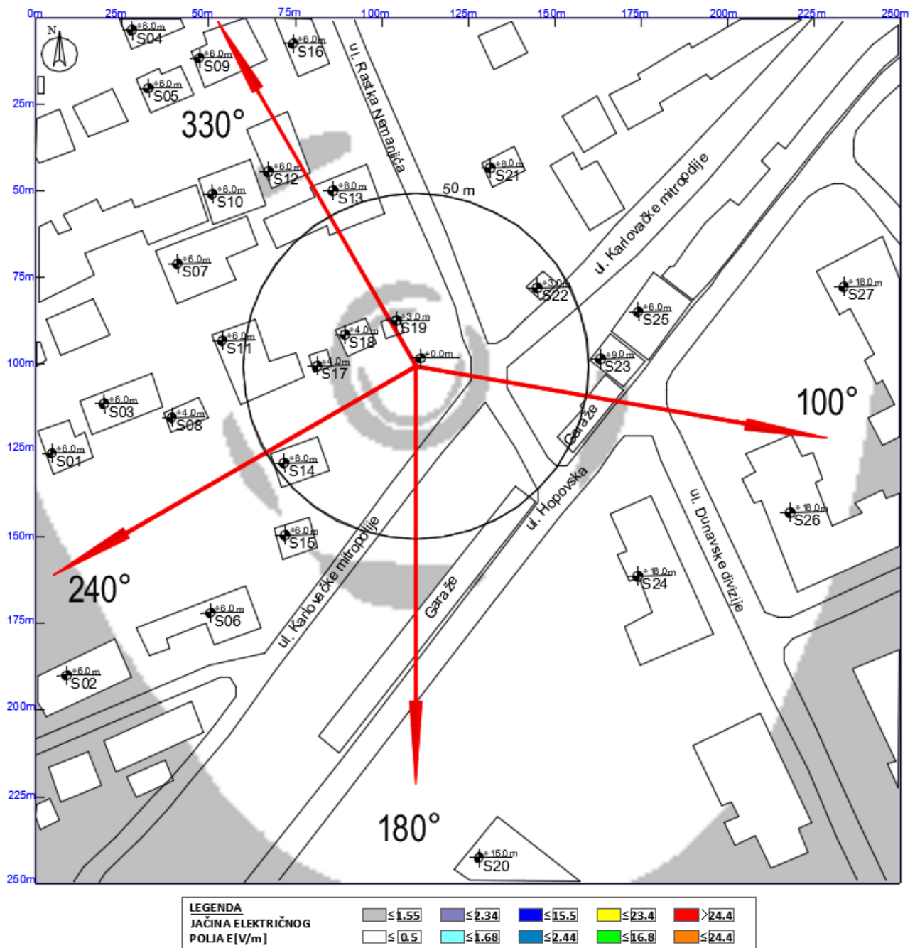
Slika 6.13 Maksimalna proračunata vrednost električnog polja na nivou tla u slučaju rada sistema LTE2100 operatora Telekom iznosi: 1.26 V/m
