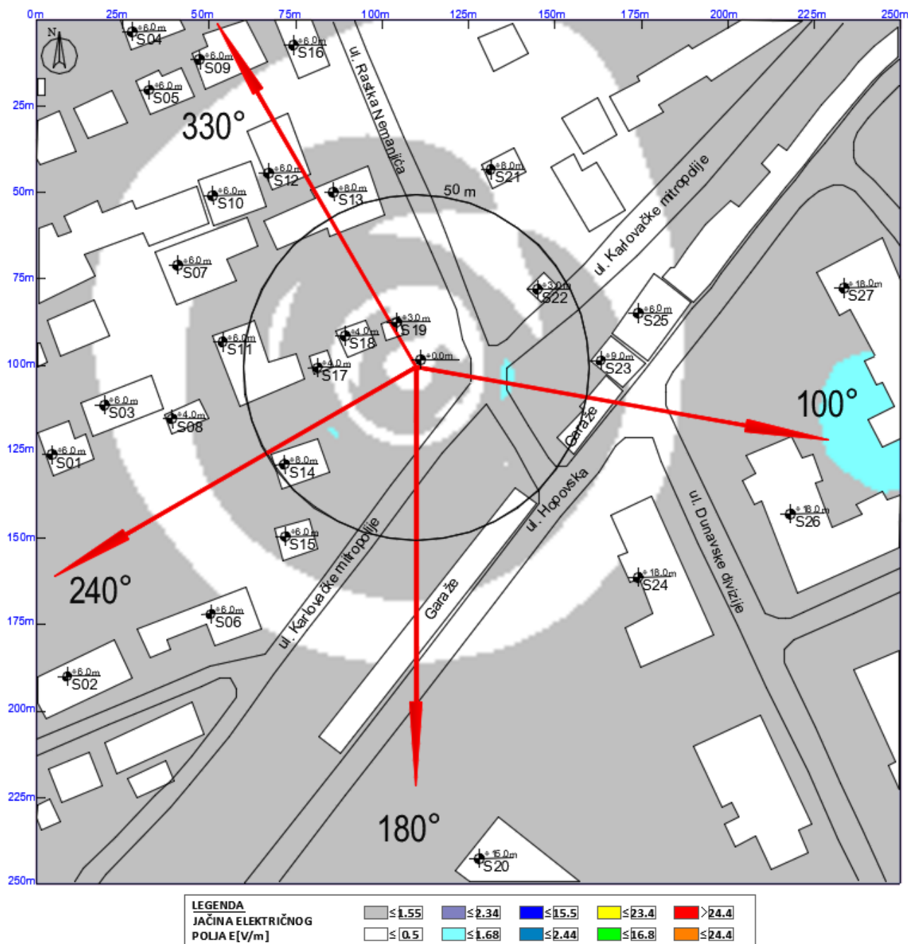
Slika 6.9 Maksimalna proračunata vrednost električnog polja na nivou tla u slučaju rada sistema GSM900 operatora Telekom iznosi: 1.65 V/m
