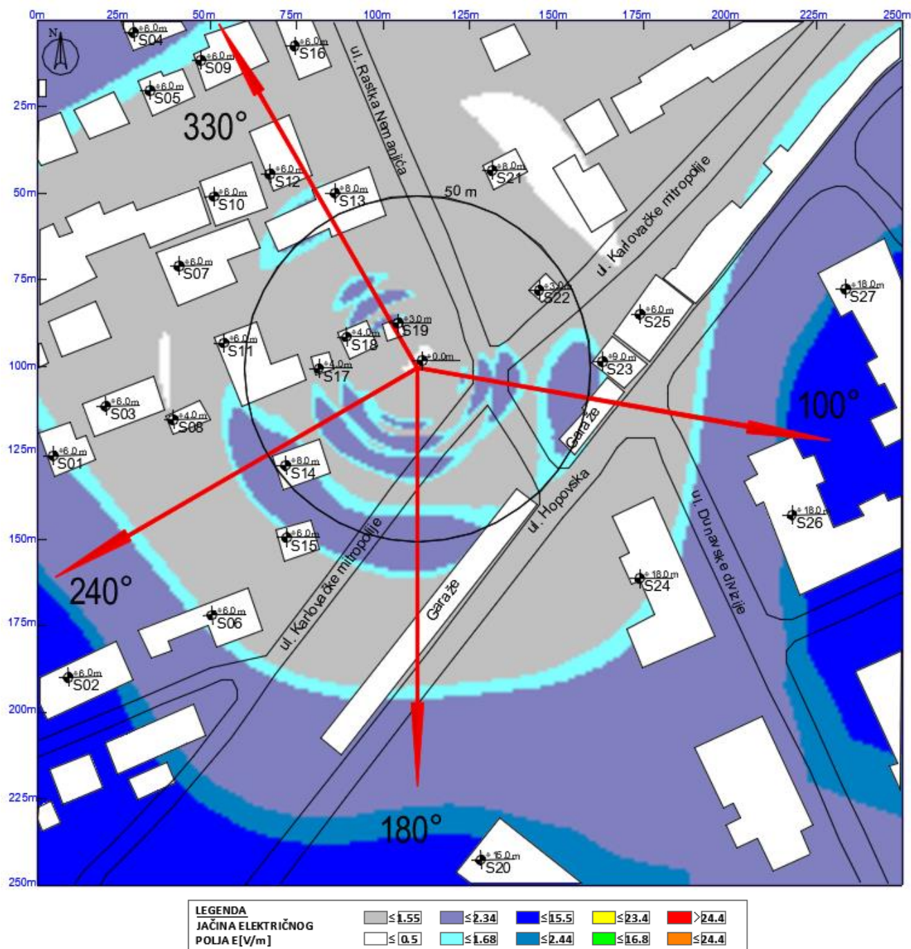
Slika 6.14 Maksimalna proračunata vrednost električnog polja na nivou tla u slučaju rada svih sistema na predmetnoj lokaciji operatora Telekom iznosi: 2.95 V/m .
