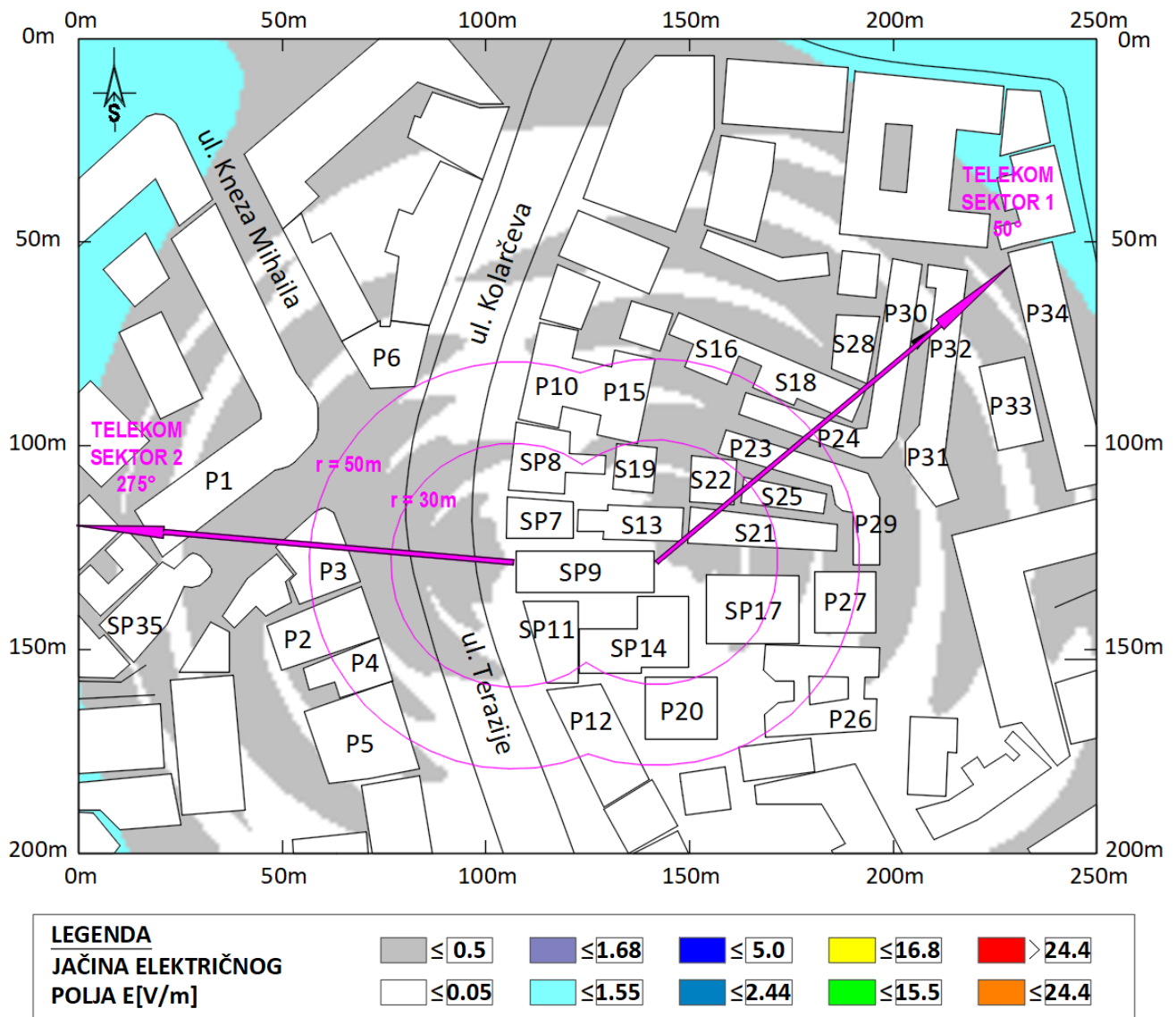
Slika 6.13 Rezultati proračuna jačine električnog polja u široj okolini lokacije bazne stanice na visini +1.70m (prosečna visina čoveka) u odnosu na nivo tla za slučaj rada sistema LTE2100 operatera Telekom . Maksimalna proračunata vrednost jačine električnog polja iznosi E=1.25 V/m
