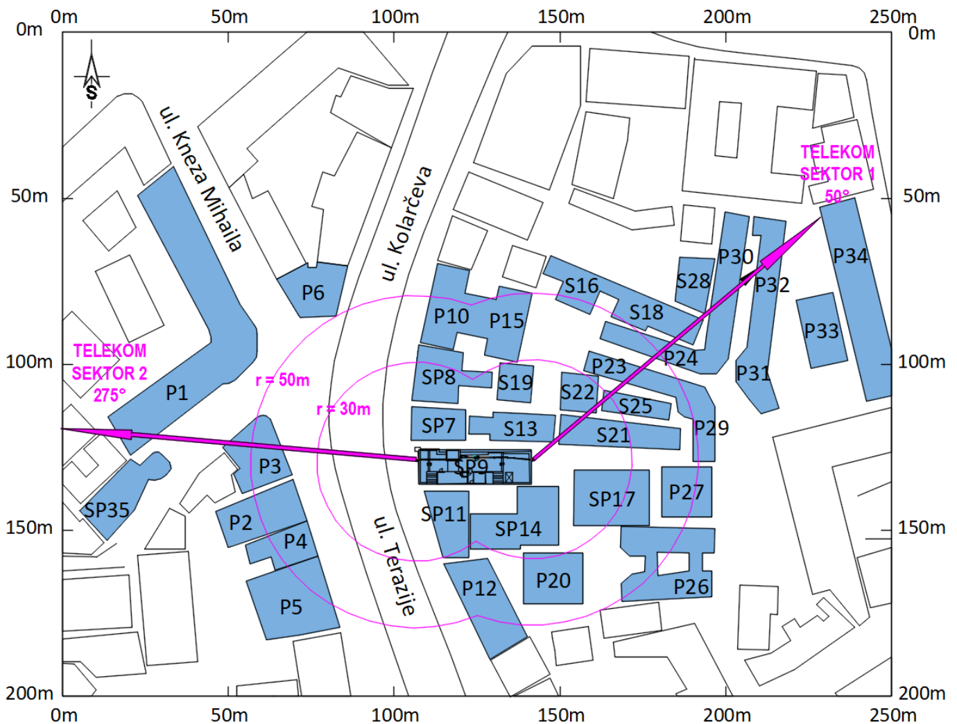
Slika 2.2 Dijagram objekata u okruženju radio bazne stanice "BG - Terazije III" – BG128/BGU128/BGL128/BGO128/BGJ128
