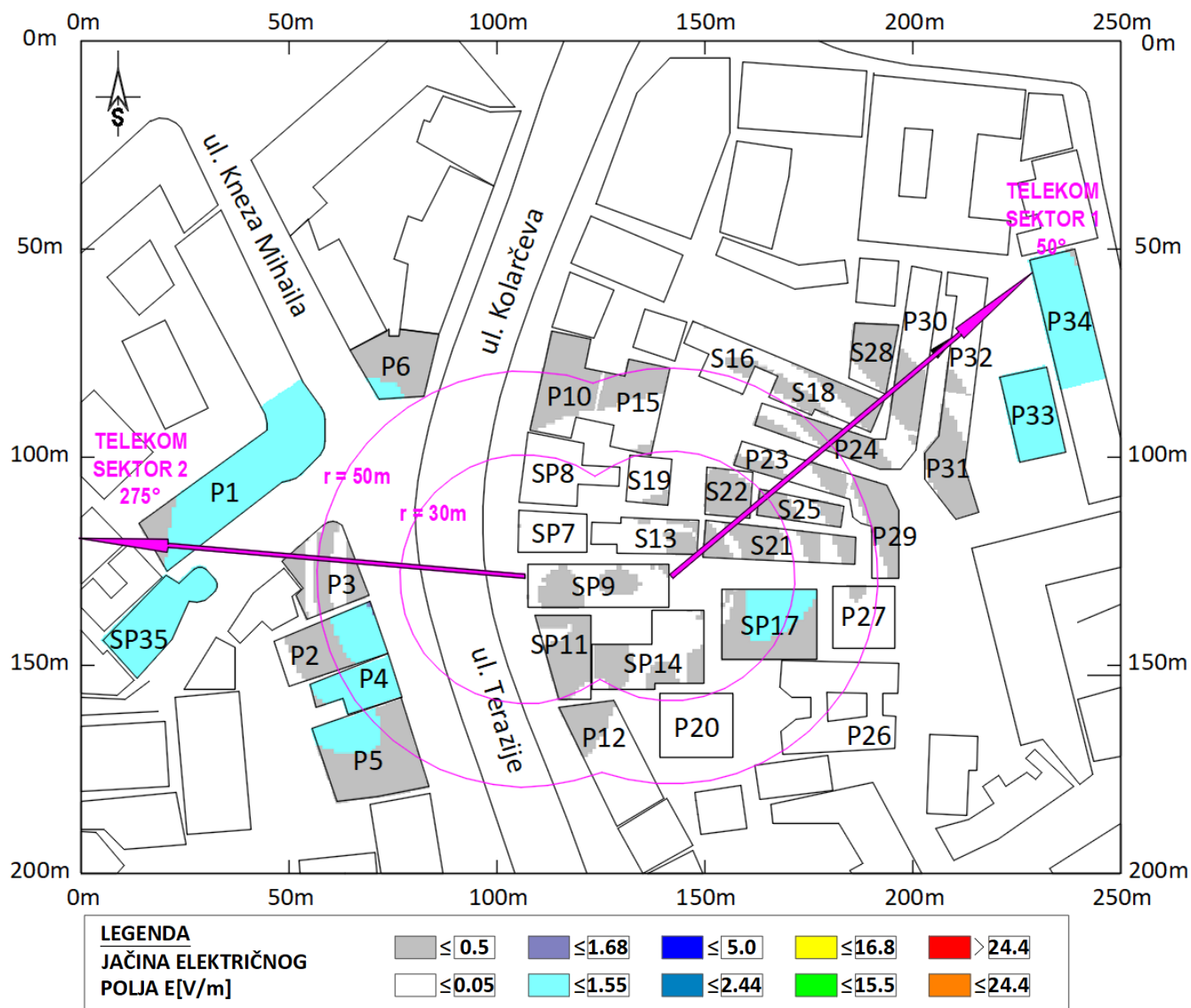
Slika 6.3 Rezultati proračuna jačine električnog polja u objektima na najizloženijim spratovima za slučaj rada sistema UMTS2100 operatora Telekom Srbija
