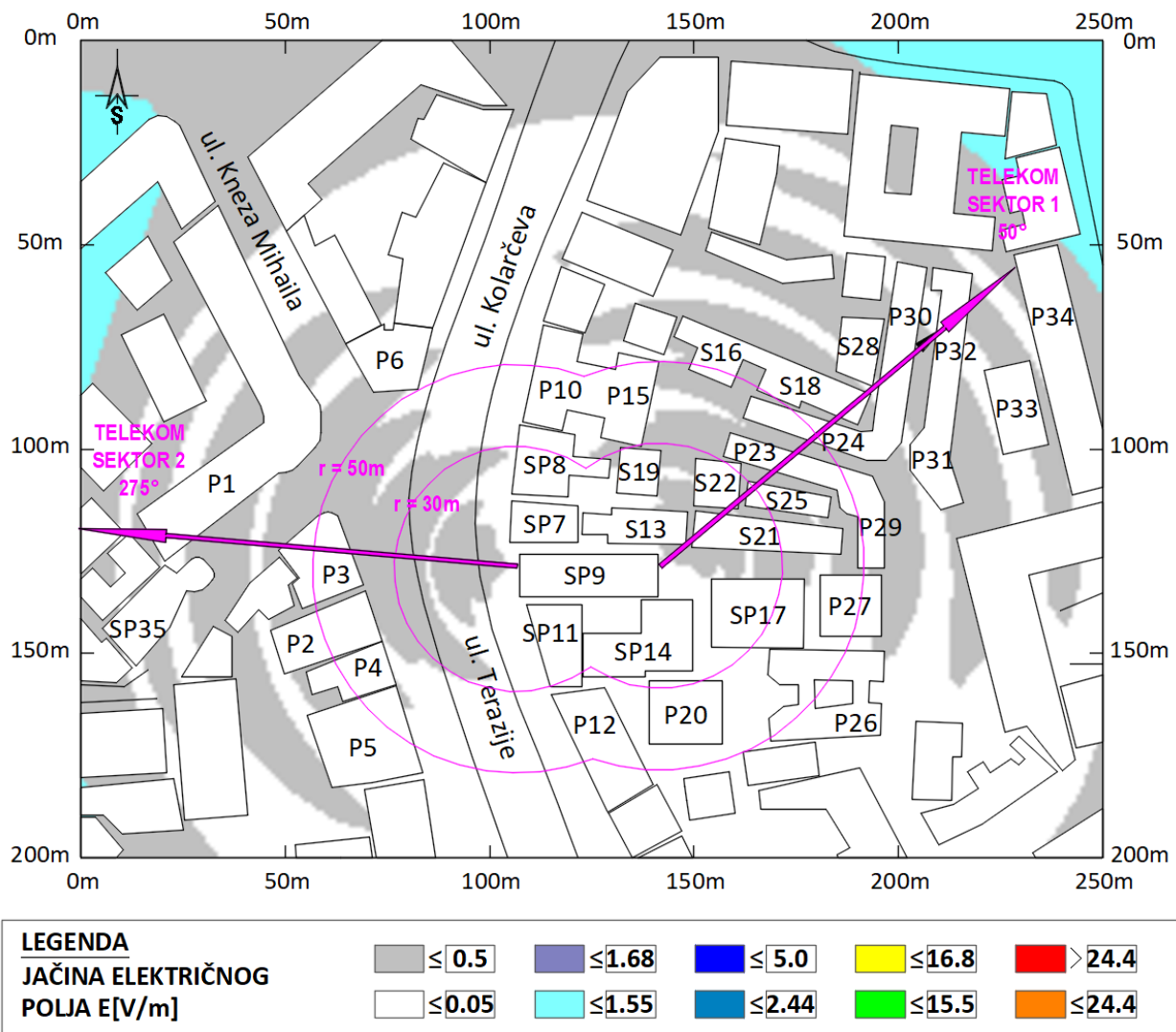
Slika 6.10 Rezultati proračuna jačine električnog polja u široj okolini lokacije bazne stanice na visini +1.70m (prosečna visina čoveka) u odnosu na nivo tla za slučaj rada sistema UMTS2100 operatera Telekom . Maksimalna proračunata vrednost jačine električnog polja iznosi E=0.99 V/m
