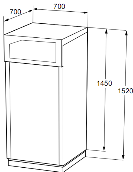
Slika 10.2 Dimenzije RBS6101
