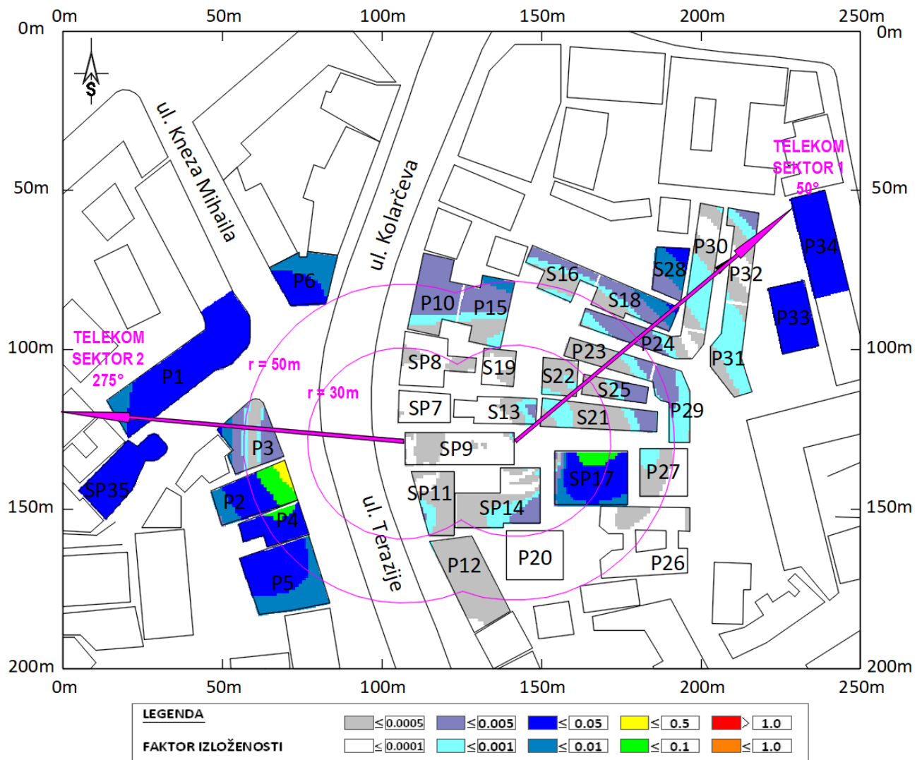
Slika 6.8 Rezultati proračuna ukupnog faktora izloženosti u objektima na najizloženijim spratovima za slučaj rada svih sistema operatora Telekom Srbija
