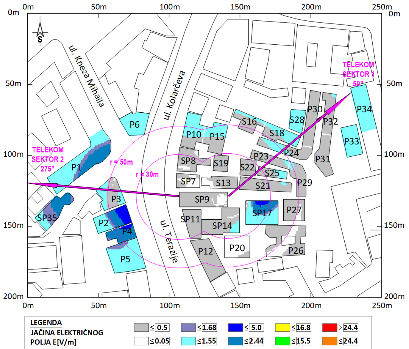
Slika 6.6 Rezultati proračuna jačine električnog polja u objektima na najizloženijim spratovima za slučaj rada sistema LTE800 operatora Telekom Srbija
