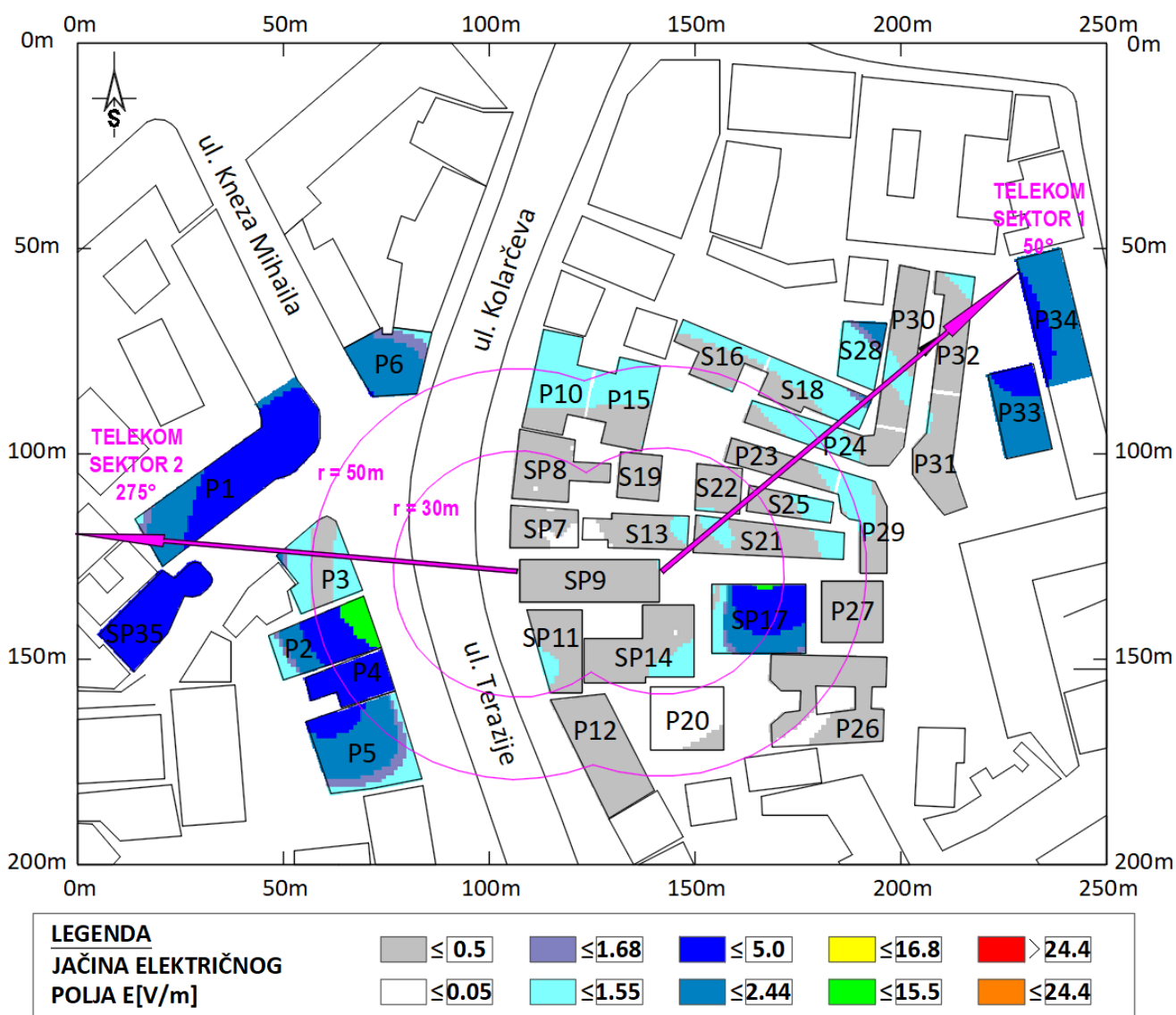
Slika 6.7 Rezultati proračuna jačine električnog polja u objektima na najizloženijim spratovima za slučaj rada svih sistema operatora Telekom Srbija
