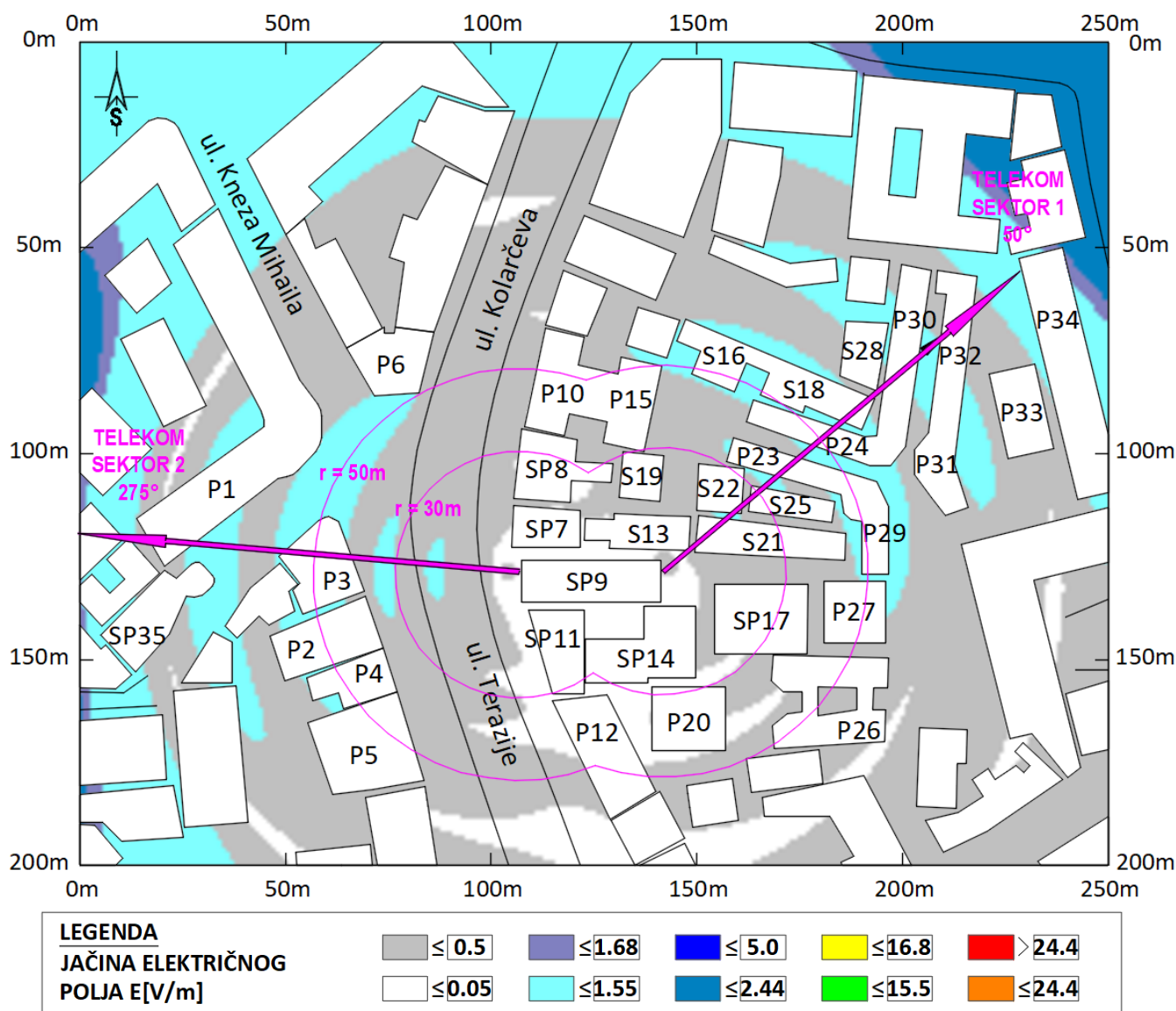
Slika 6.12 Rezultati proračuna jačine električnog polja u široj okolini lokacije bazne stanice na visini +1.70m (prosečna visina čoveka) u odnosu na nivo tla za slučaj rada sistema LTE800 operatera Telekom . Maksimalna proračunata vrednost jačine električnog polja iznosi E=2.12V/m
