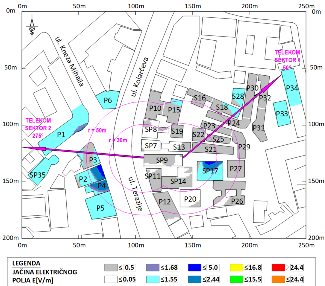
Slika 6.1 Rezultati proračuna- jačine električnog polja -u objektima na najizloženijim spratovima za slučaj rada za slučaj rada sistema GSM900 operatera Telekom Srbija .
