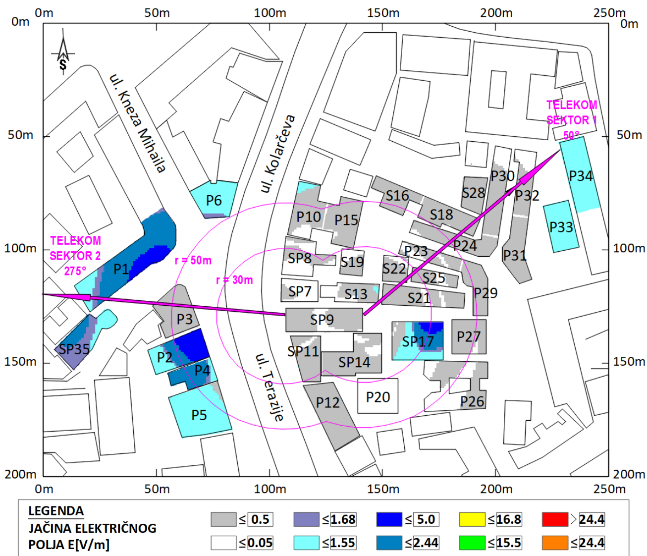
Slika 6.4 Rezultati proračuna jačine električnog polja u objektima na najizloženijim spratovima za slučaj rada sistema LTE1800 operatora Telekom Srbija
