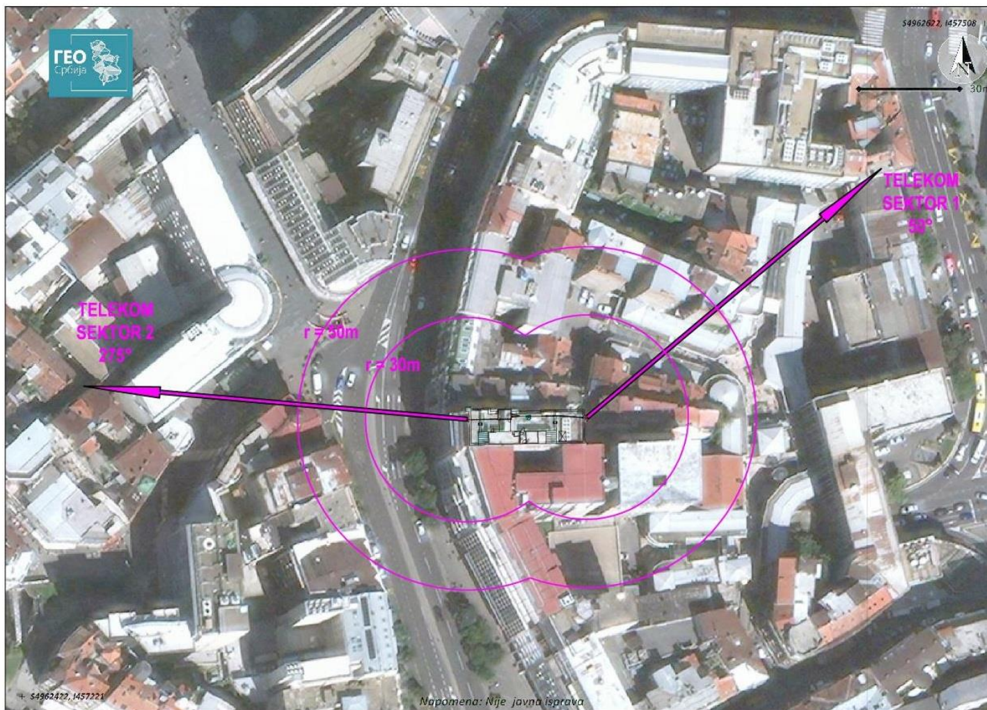
Slika 2.1 Dijagram zračenja radio bazne stanice "BG - Terazije III" – BG128/BGU128/BGL128/BGO128/BGJ128
