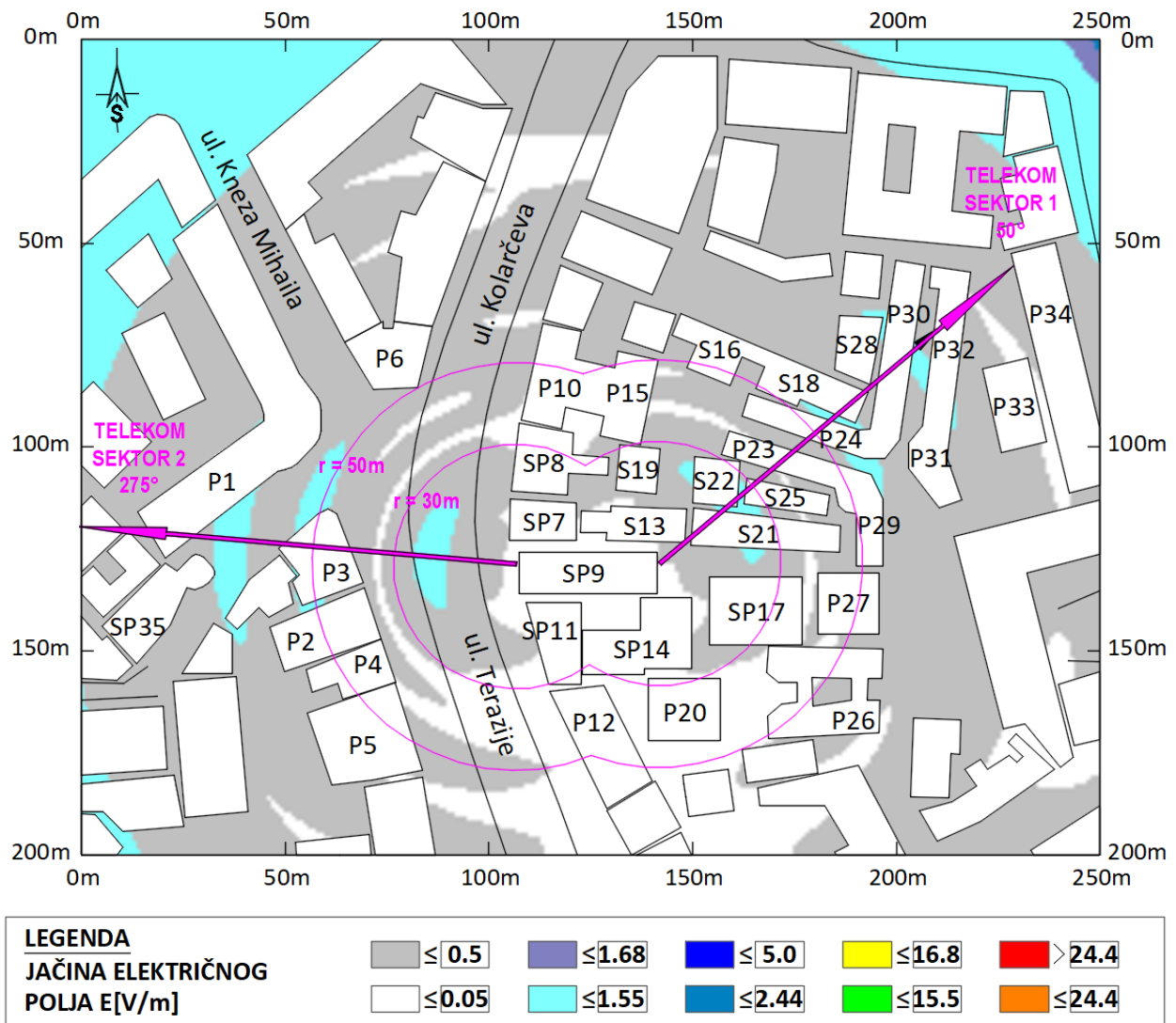
Slika 6.11 Rezultati proračuna jačine električnog polja u široj okolini lokacije bazne stanice na visini +1.70m (prosečna visina čoveka) u odnosu na nivo tla za slučaj rada sistema LTE1800 operatera Telekom . Maksimalna proračunata vrednost jačine električnog polja iznosi E=1.71 V/m
