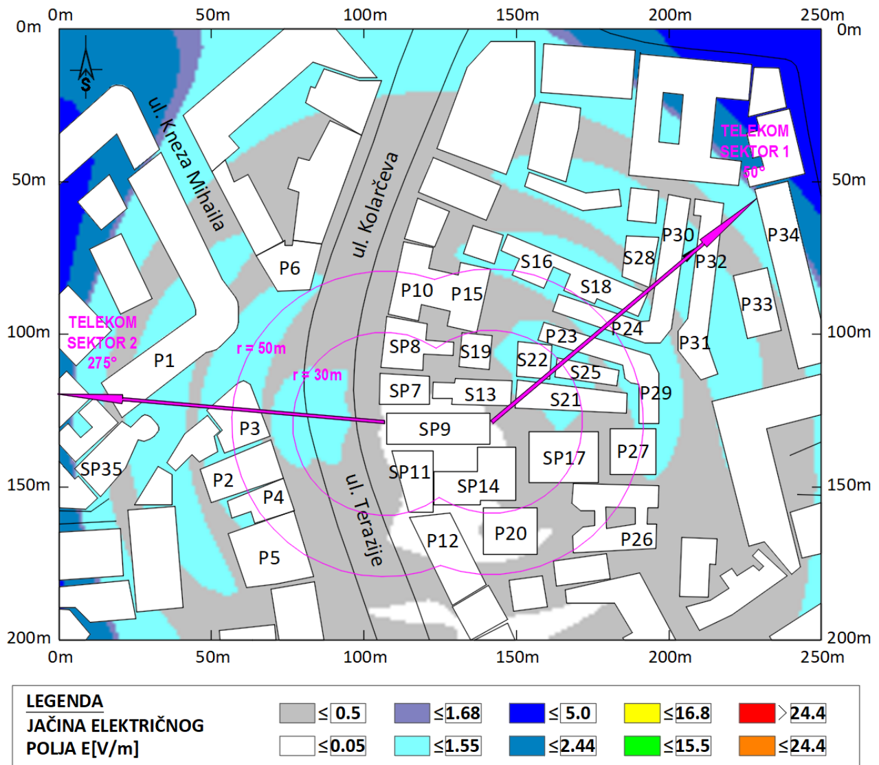
Slika 6.14 Rezultati proračuna jačine električnog polja u široj okolini lokacije bazne stanice na visini +1.70m (prosečna visina čoveka) u odnosu na nivo tla za slučaj rada svih sistema operatera Telekom . Maksimalna proračunata vrednost jačine električnog polja iznosi E=3.52 V/m
