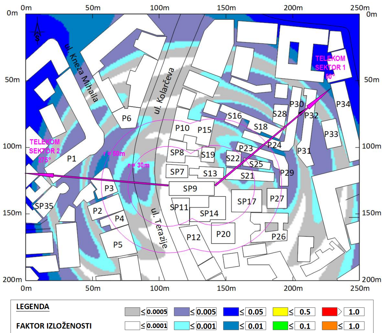
Slika 6.15 Rezultati proračuna faktora izloženosti u široj okolini lokacije bazne stanice na visini +1.70m (prosečna visina čoveka) u odnosu na nivo tla za slučaj rada svih sistema operatera Telekom. Maksimalna proračunata vrednost faktora izloženosti iznosi: F.I=0.0381 .
