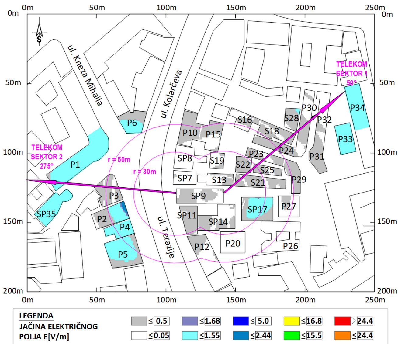
Slika 6.6 Rezultati proračuna jačine električnog polja u objektima na najizloženijim spratovima za slučaj rada sistema LTE2100 operatora Telekom Srbija
