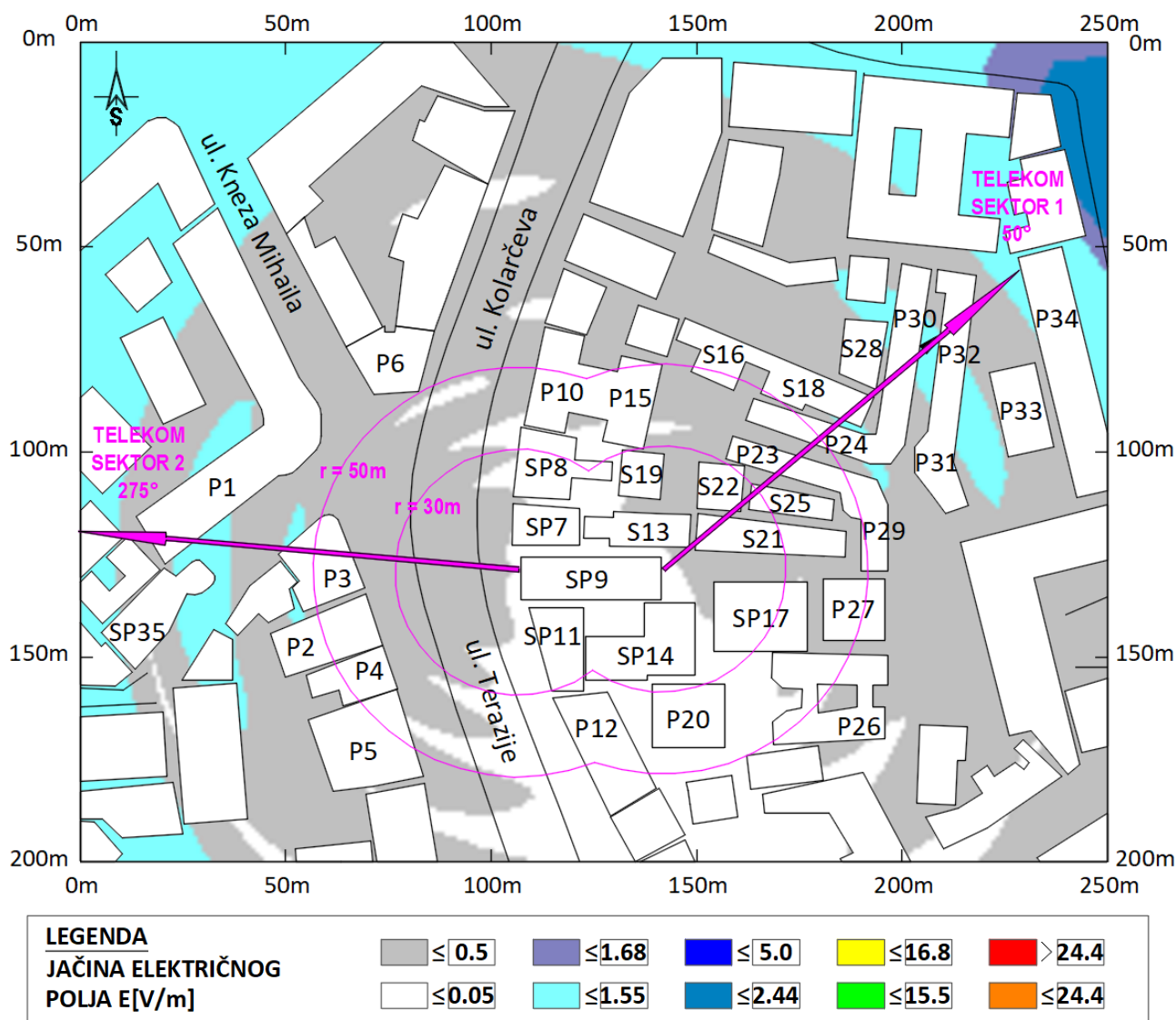
Slika 6.9 Rezultati proračuna jačine električnog polja u široj okolini lokacije bazne stanice na visini +1.70m (prosečna visina čoveka) u odnosu na nivo tla za slučaj rada sistema GSM900 operatera Telekom. Maksimalna proračunata vrednost jačine električnog polja iznosi E=1.79 V/m .
