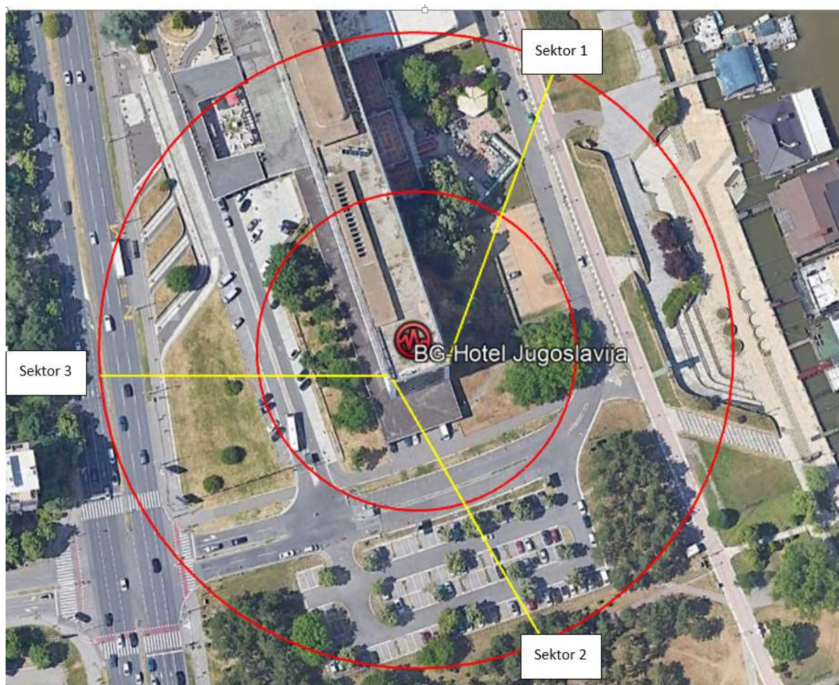
Slika 2.7 Pravci zračenja antenskih sistema predmetne bazne stanice
