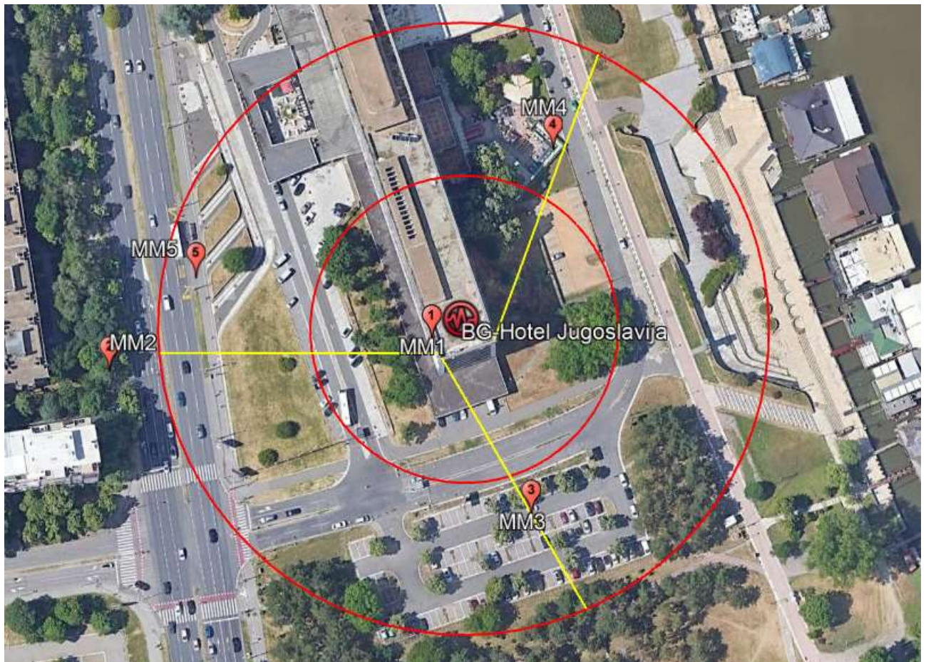
Slika 8: Prikaz Mernih Mesta u lokalnoj zoni BS Telekom Srbija BG-Hotel Jugoslavija
