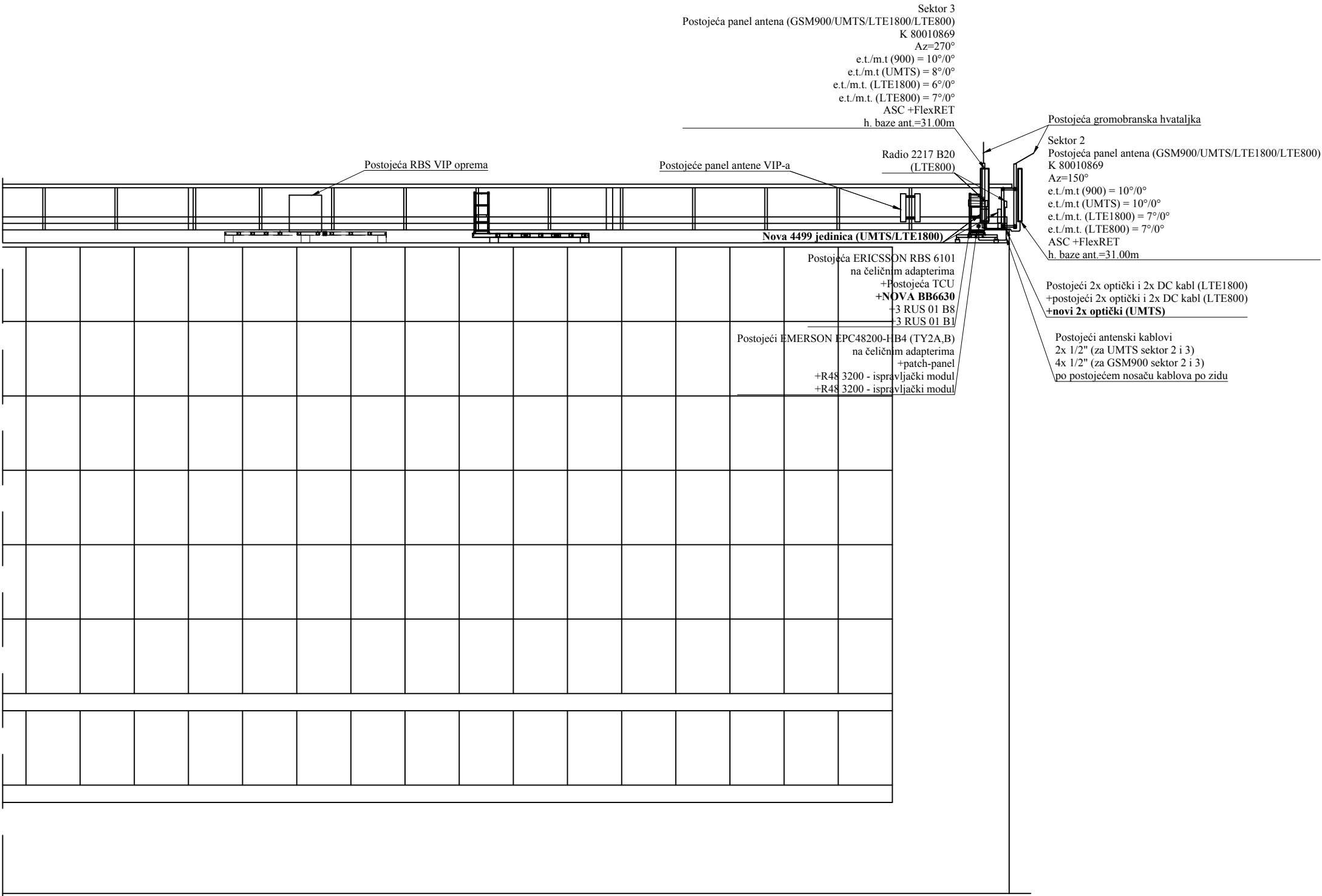
Izgled A-A
