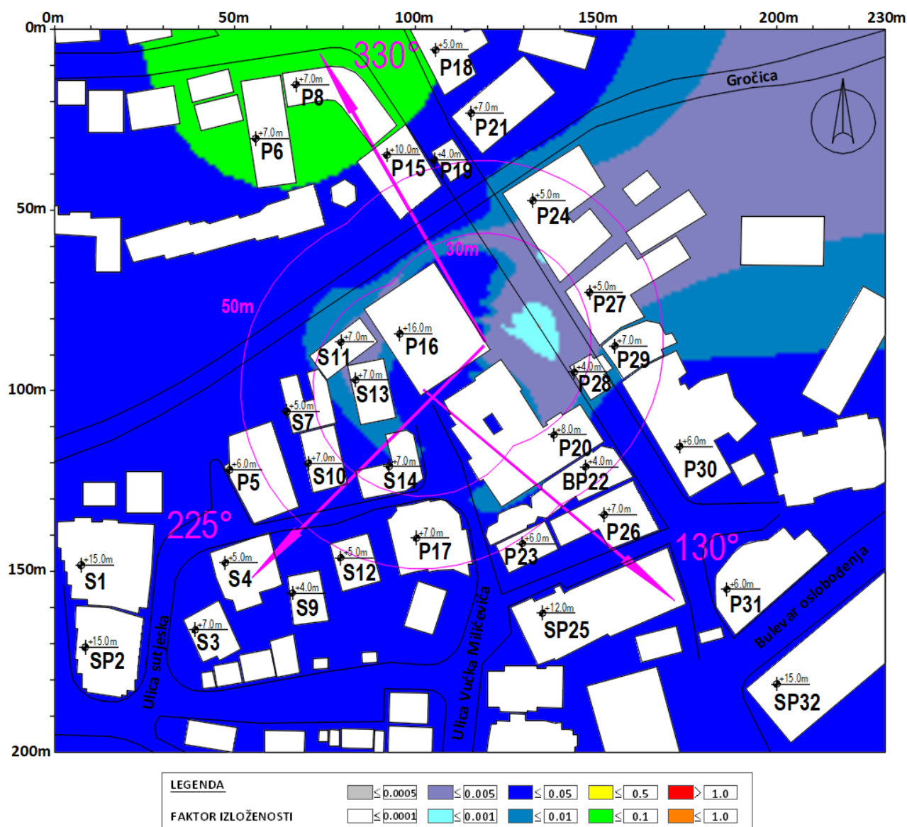
Slika 4.14 Rezultati proračuna faktora izloženosti u široj okolini lokacije bazne stanice na visini +1.70m (prosečna visina čoveka) u odnosu na nivo tla za slučaj rada svih sistema operatera Telekom. Maksimalna proračunata vrednost faktora izloženosti iznosi: F.I=0.0738 .
