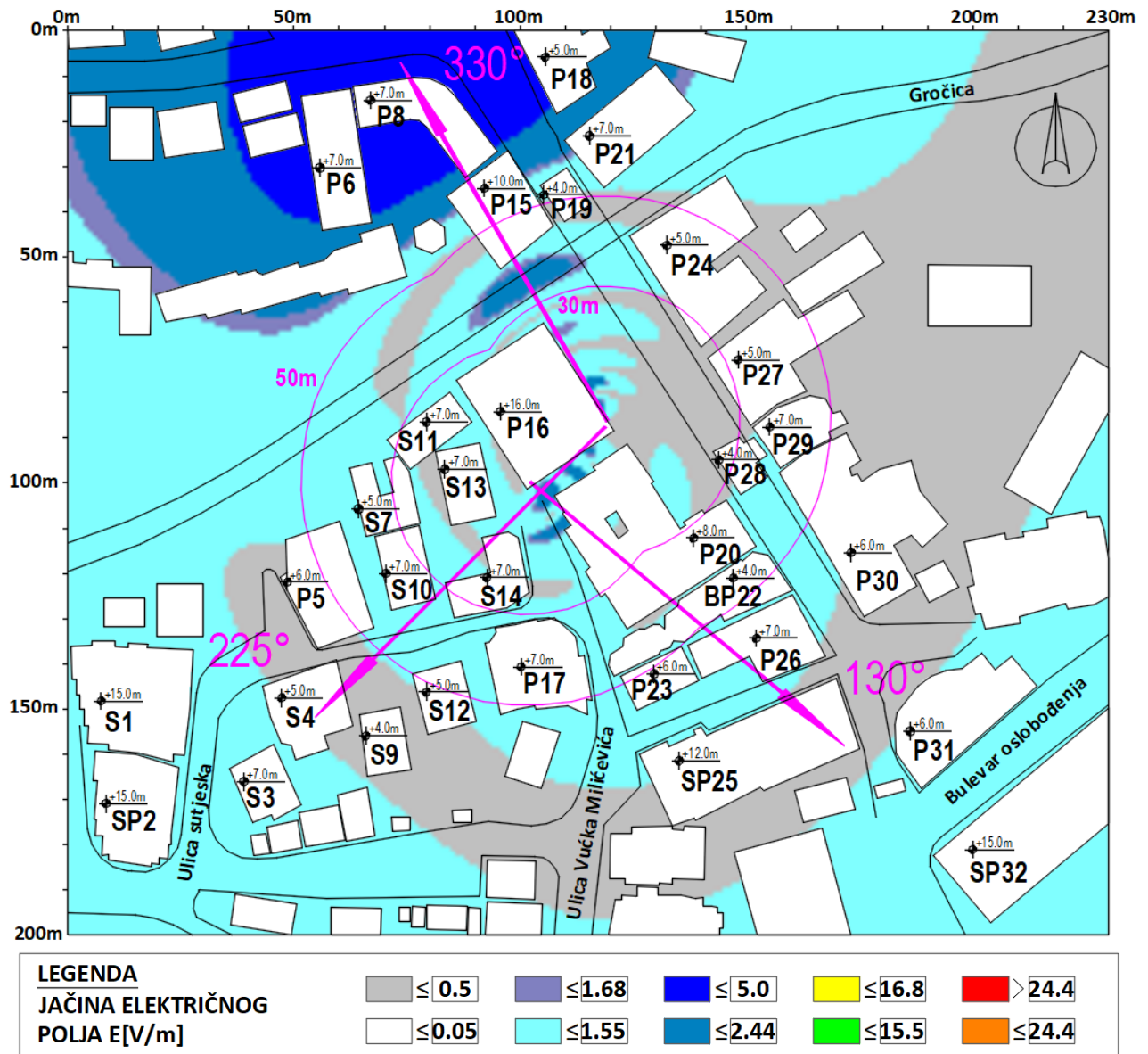
Slika 4.10 Rezultati proračuna jačine električnog polja u široj okolini lokacije bazne stanice na visini +1.70m (prosečna visina čoveka) u odnosu na nivo tla za slučaj rada sistema GSM900 operatera Telekom. Maksimalna proračunata vrednost jačine električnog polja iznosi E=3.09 V/m.
