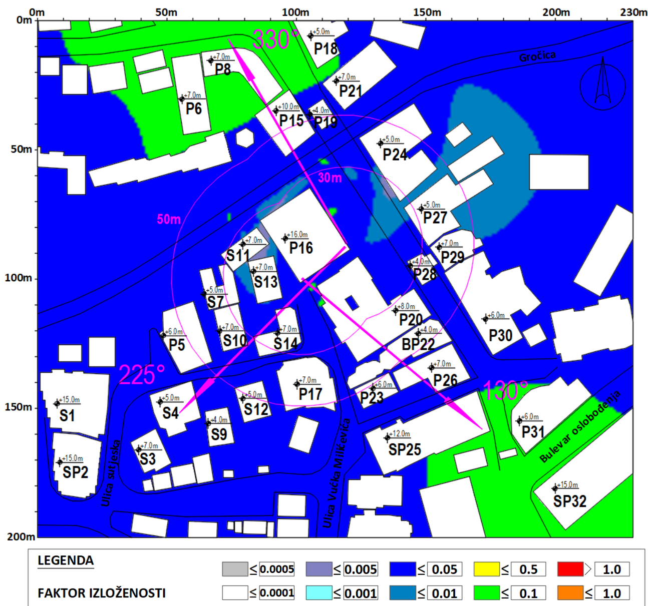
Slika 4.5 Rezultati proračuna faktora izloženosti u široj okolini lokacije bazne stanice na visini +1.70m (prosečna visina čoveka) u odnosu na nivo tla za slučaj rada svih sistema operatora Telekom I Cetin(Yettel). Maksimalna proračunata vrednost faktora izloženosti iznosi FI=0.0748 .
