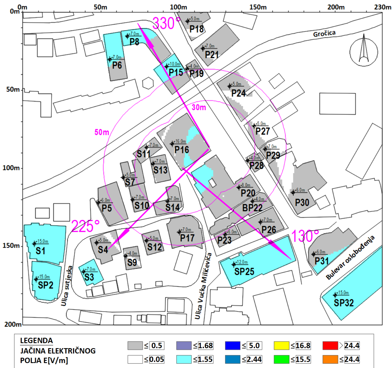
Slika 4.3 Rezultati proračuna jačine električnog polja u objektima na najizloženijim spratovima za slučaj rada sistema UMTS2100 operatora Telekom Srbija
