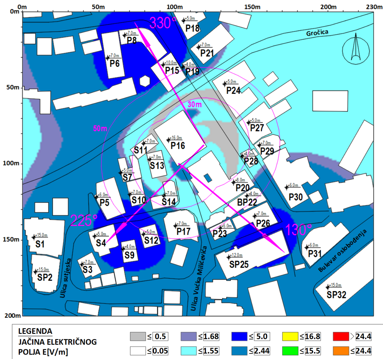
Slika 4.14 Rezultati proračuna jačine električnog polja u široj okolini lokacije bazne stanice na visini +1.70m (prosečna visina čoveka) u odnosu na nivo tla za slučaj rada sistema LTE800 operatora Telekom . Maksimalna proračunata vrednost jačine električnog polja iznosi E=2.92 V/m .
