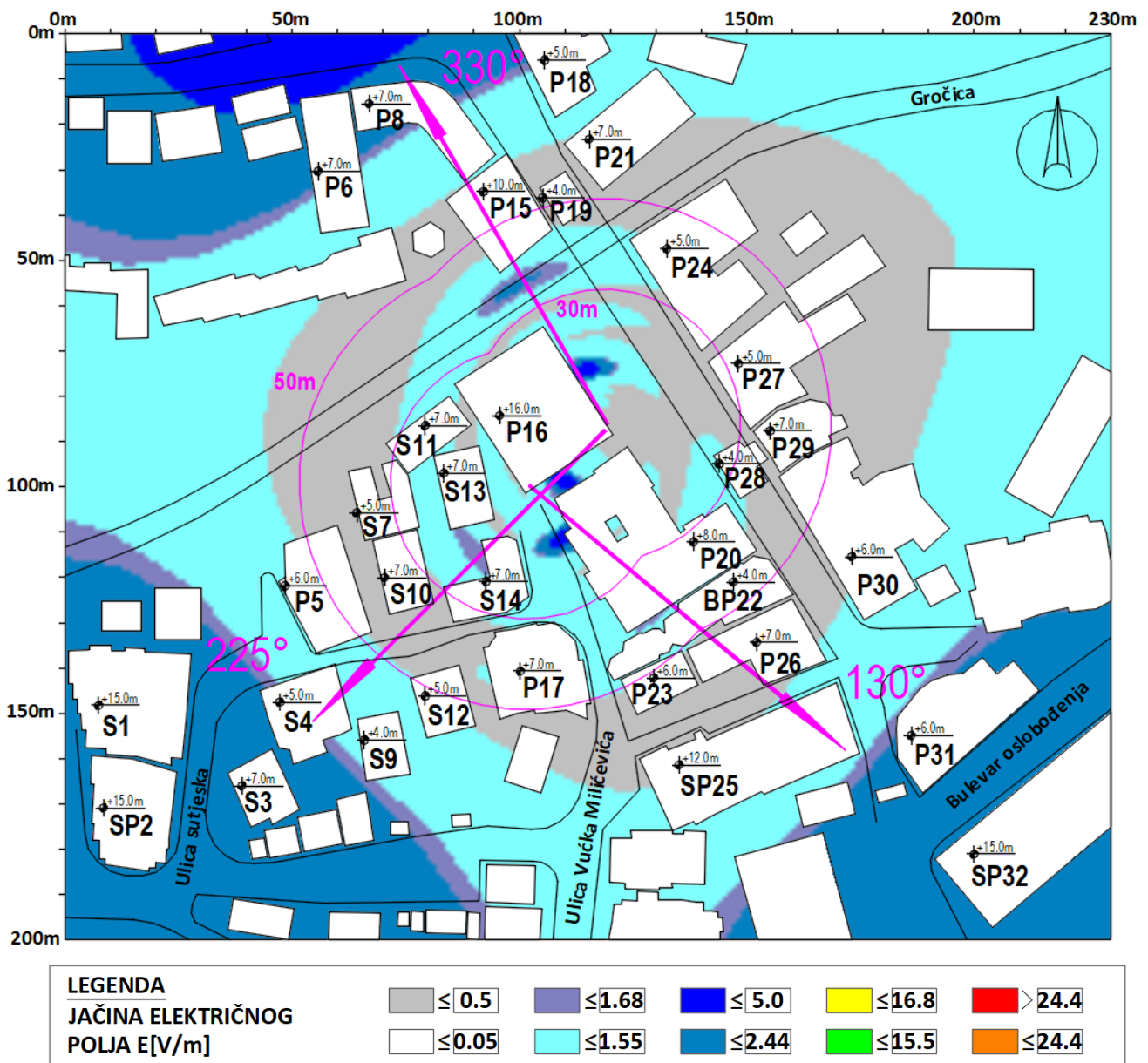
Slika 4.13 Rezultati proračuna jačine električnog polja u široj okolini lokacije bazne stanice na visini +1.70m (prosečna visina čoveka) u odnosu na nivo tla za slučaj rada sistema LTE1800 operatora Telekom . Maksimalna proračunata vrednost jačine električnog polja iznosi E=3.08 V/m .
