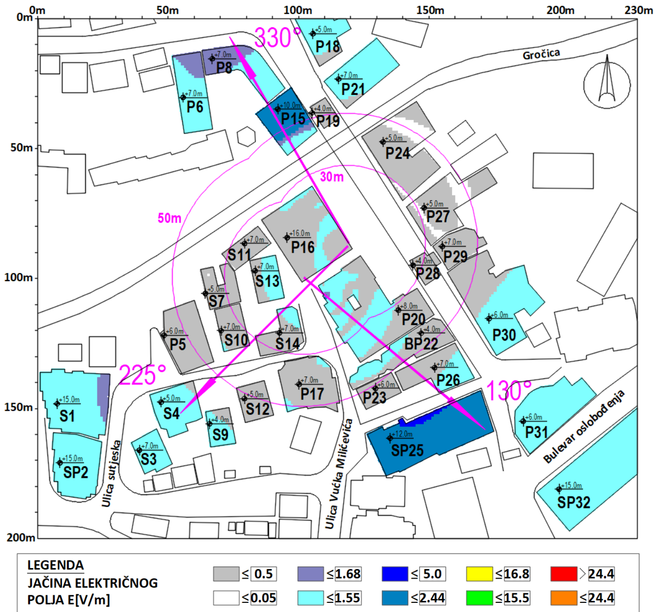
Slika 4.5 Rezultati proračuna jačine električnog polja u objektima na najizloženijim spratovima za slučaj rada sistema LTE1800 operatora Telekom Srbija
