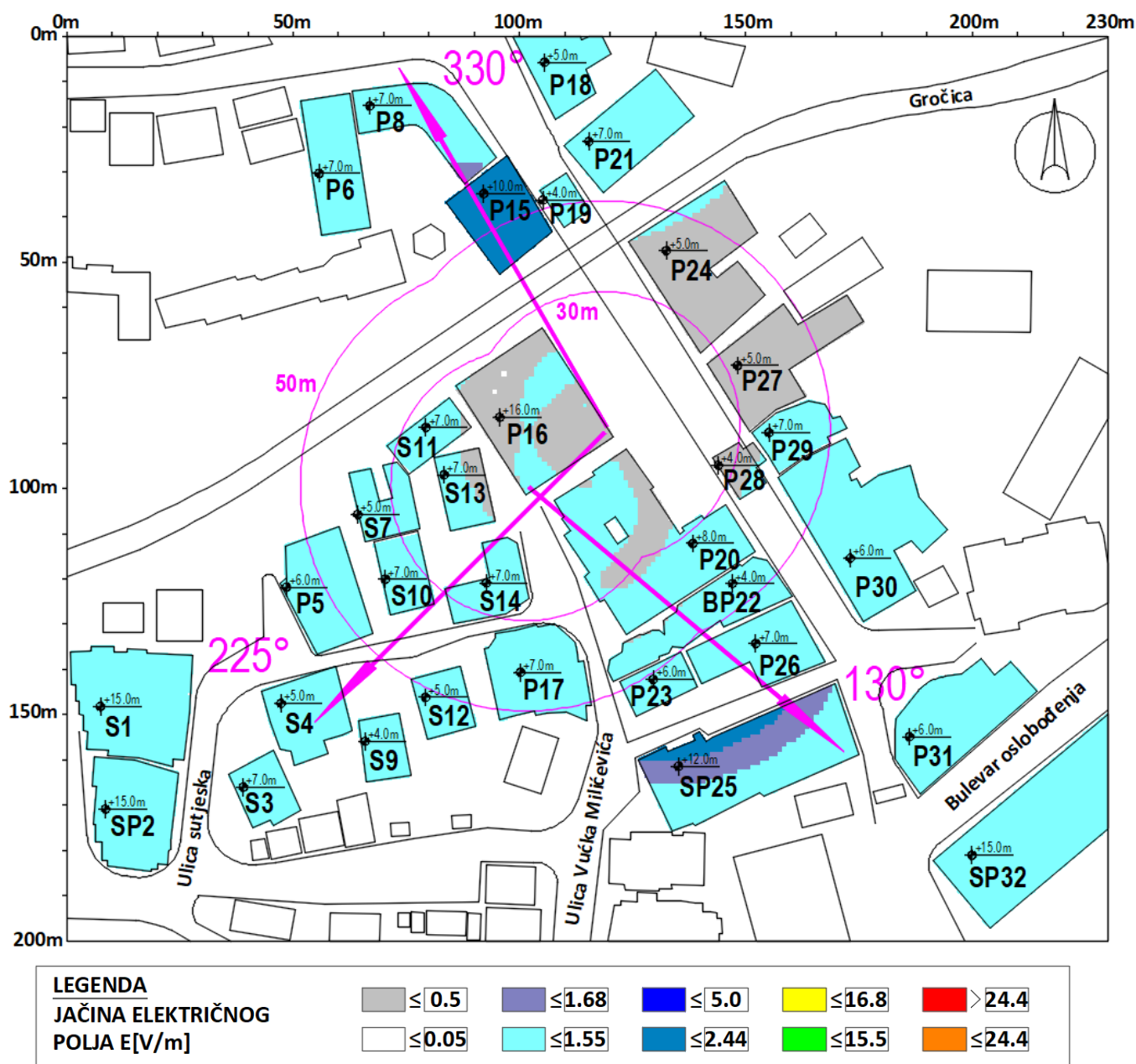
Slika 4.6 Rezultati proračuna jačine električnog polja u objektima na najizloženijim spratovima za slučaj rada sistema LTE800 operatora Telekom Srbija
