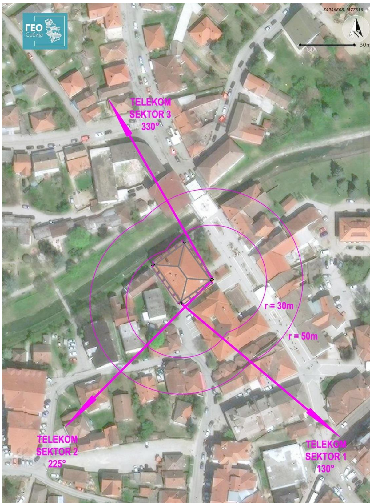
Slika 2.1 Dijagram zračenja radio bazne stanice "Grocka PTT" – BG229/BGU229/BGL229/BGO229/BGJ229
