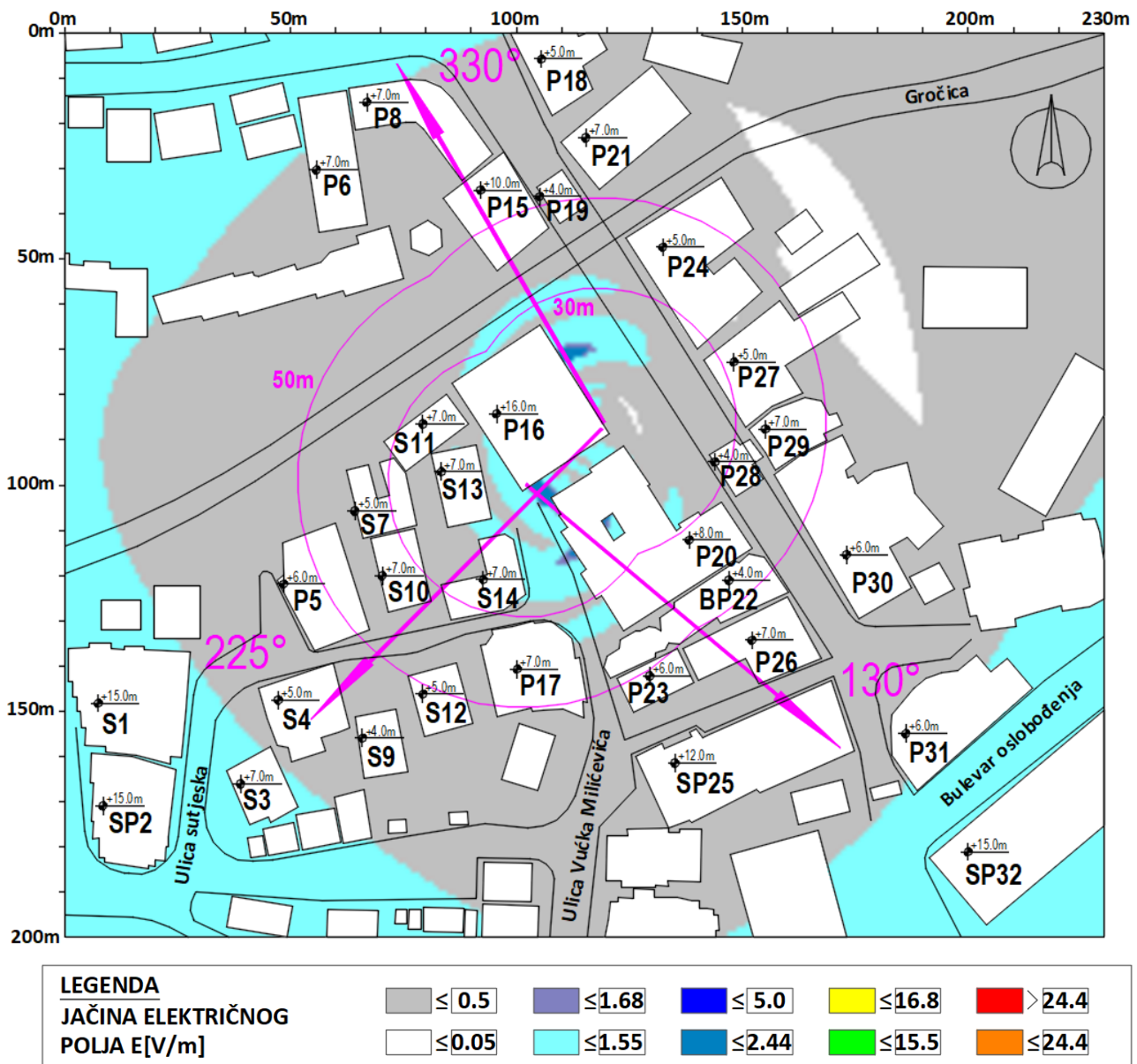
Slika 4.1 Rezultati proračuna jačine električnog polja u široj okolini lokacije bazne stanice na visini +1.70m (prosečna visina čoveka) u odnosu na nivo tla za slučaj rada sistema UMTS2100 operatora Telekom . Maksimalna proračunata vrednost jačine električnog polja iznosi E=2.00 V/m .
