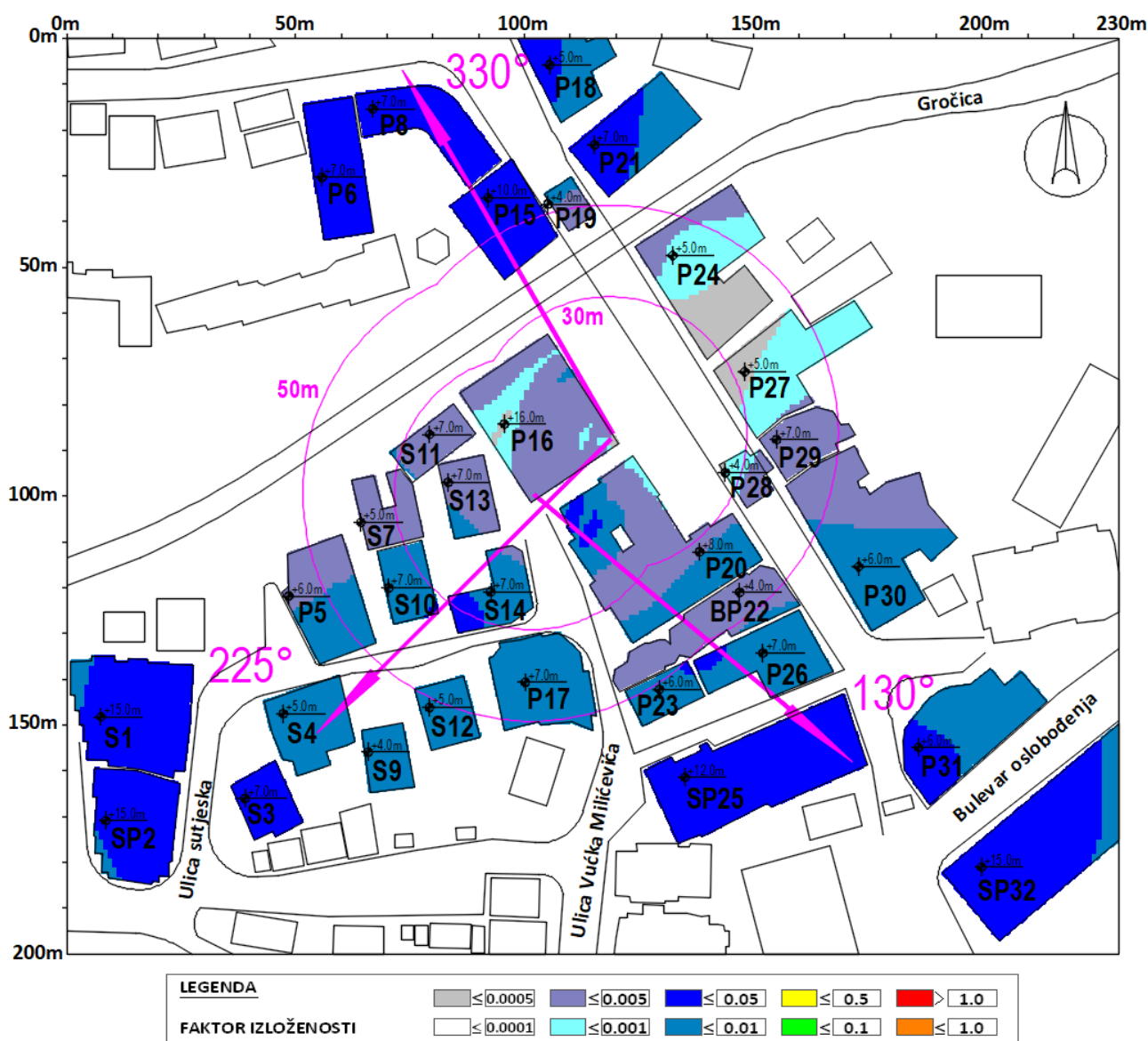
Slika 4.8 Rezultati proračuna ukupnog faktora izloženosti u objektima na najizloženijim spratovima za slučaj rada svih sistema operatora Telekom Srbija
