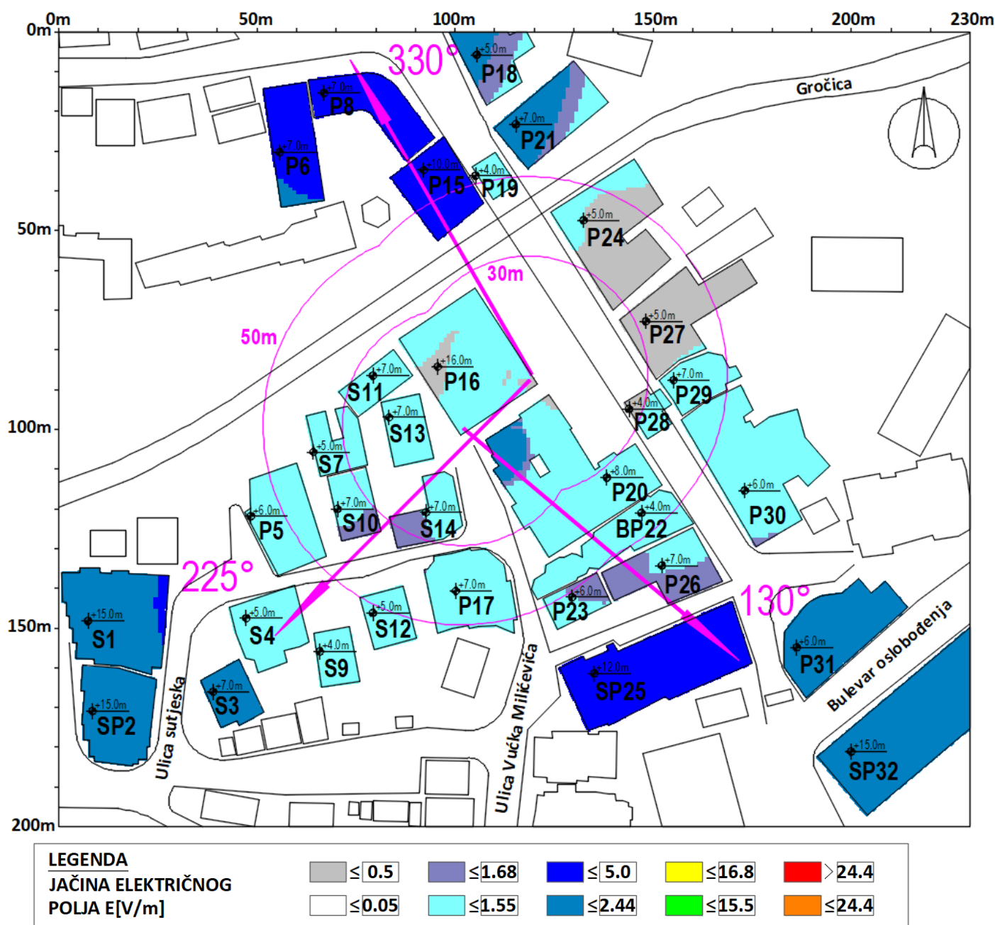
Slika 4.7 Rezultati proračuna jačine električnog polja u objektima na najizloženijim spratovima za slučaj rada svih sistema operatora Telekom Srbija
