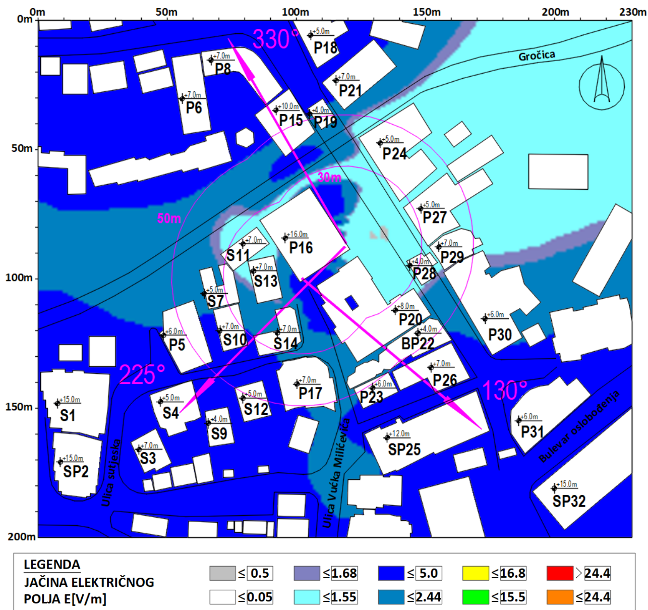
Slika 4.13 Rezultati proračuna jačine električnog polja u široj okolini lokacije bazne stanice na visini +1.70m (prosečna visina čoveka) u odnosu na nivo tla za slučaj rada svih sistema operatera Telekom . Maksimalna proračunata vrednost jačine električnog polja iznosi E=4.83 V/m
