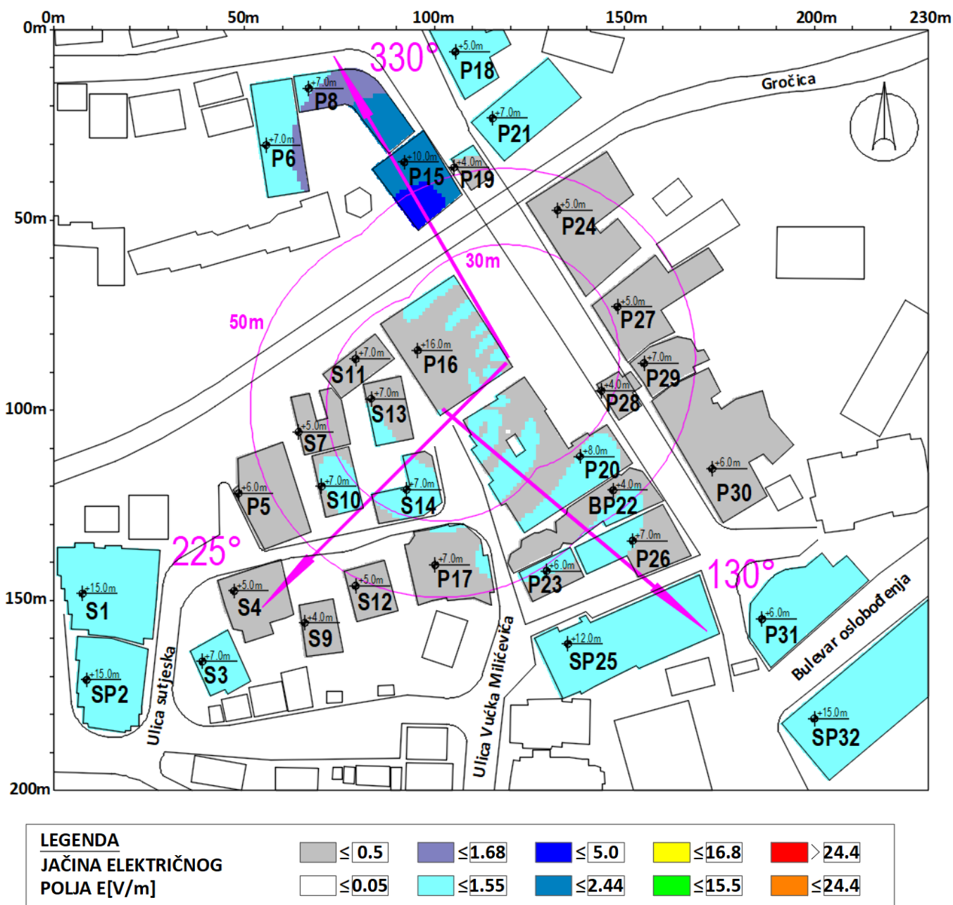
Slika 4.1 Rezultati proračuna- jačine električnog polja -u objektima na najizloženijim spratovima za slučaj rada za slučaj rada sistema GSM900 operatera Telekom Srbija .
