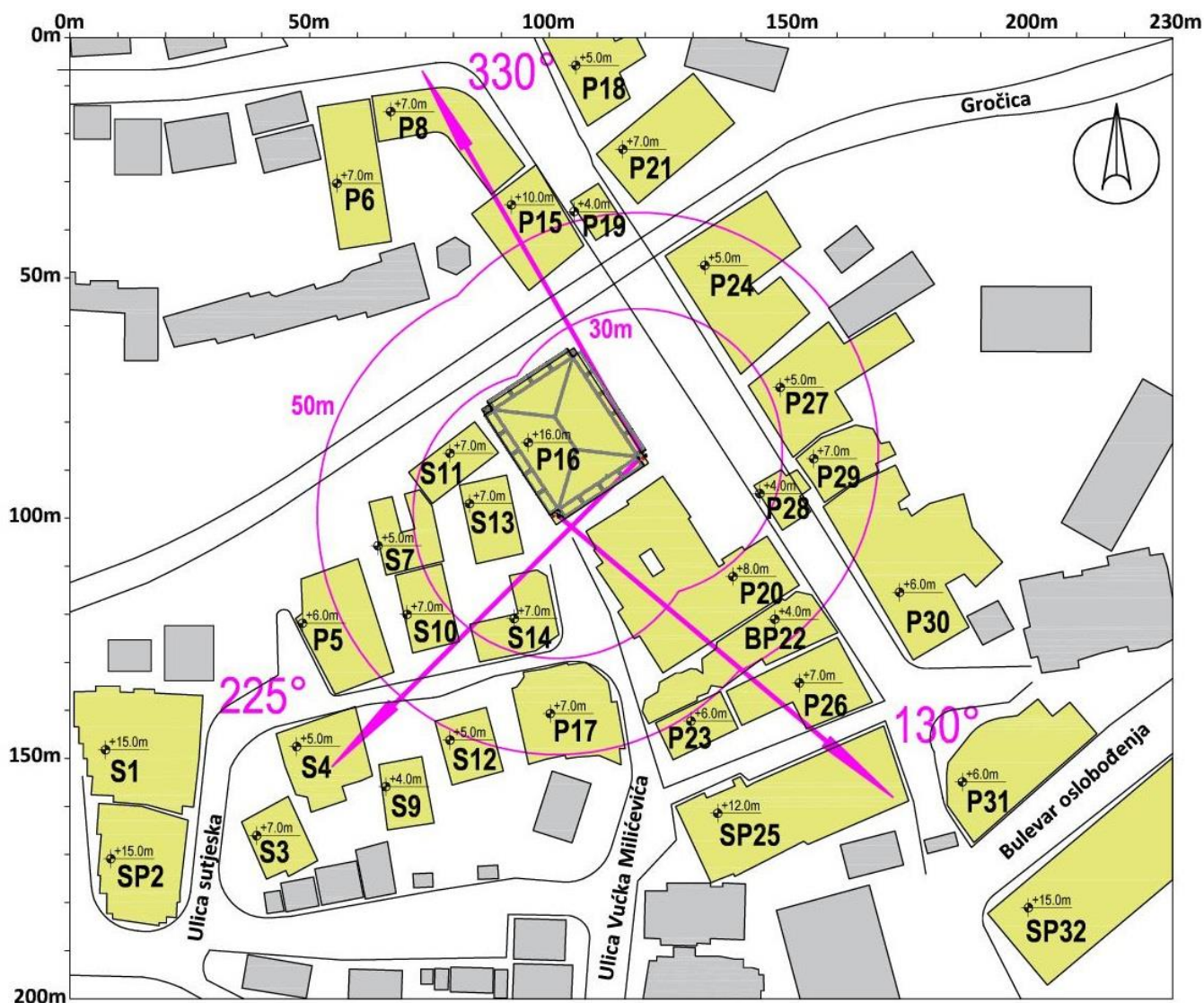
Slika 2.2 Dijagram objekata u okruženju radio bazne stanice "Grocka PTT" – BG229/BGU229/BGL229/BGO229/BGJ229
