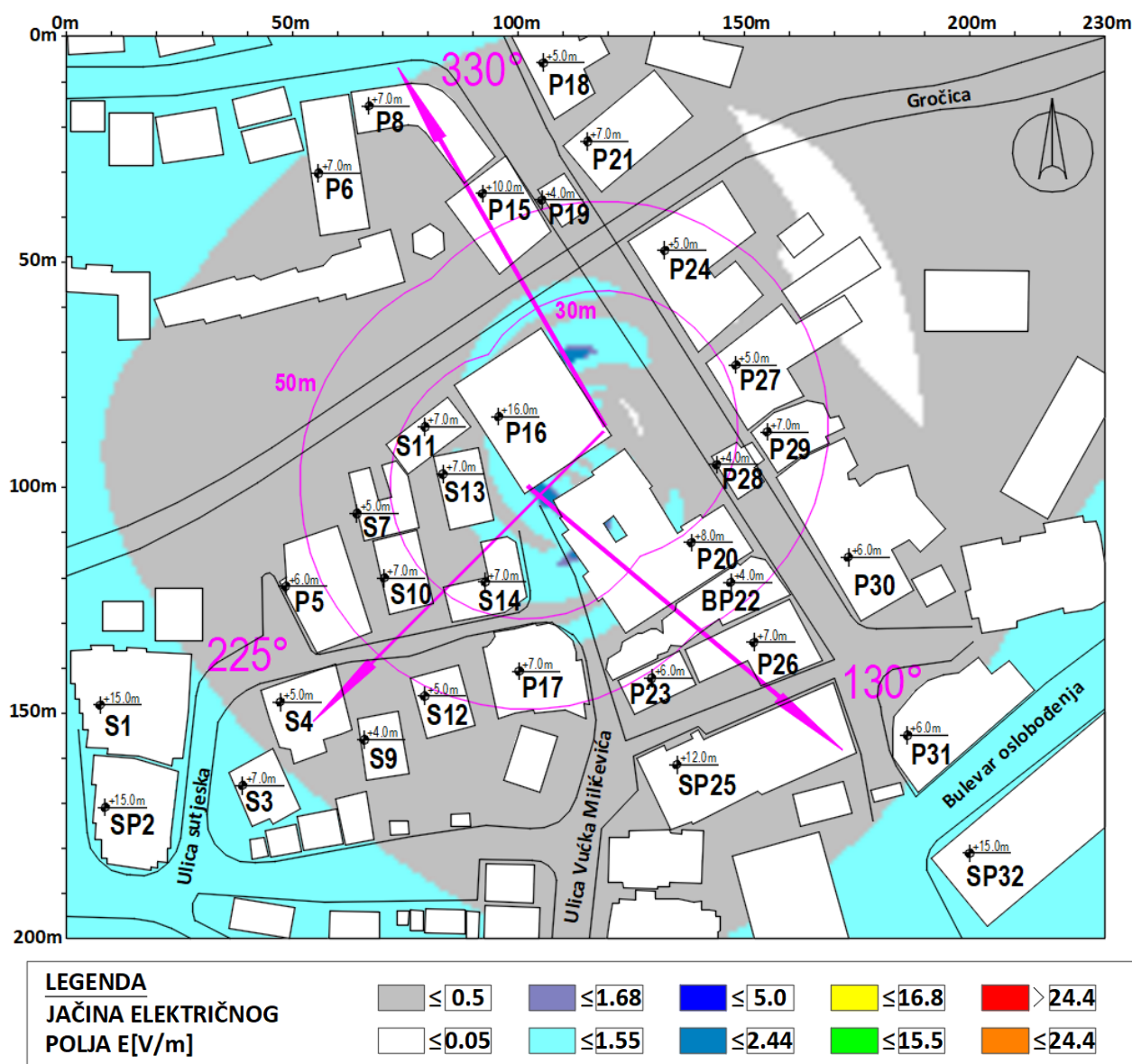
Slika 4.2 Rezultati proračuna jačine električnog polja u široj okolini lokacije bazne stanice na visini +1.70m (prosečna visina čoveka) u odnosu na nivo tla za slučaj rada sistema LTE2100 operatora Telekom . Maksimalna proračunata vrednost jačine električnog polja iznosi E=2.00 V/m .
