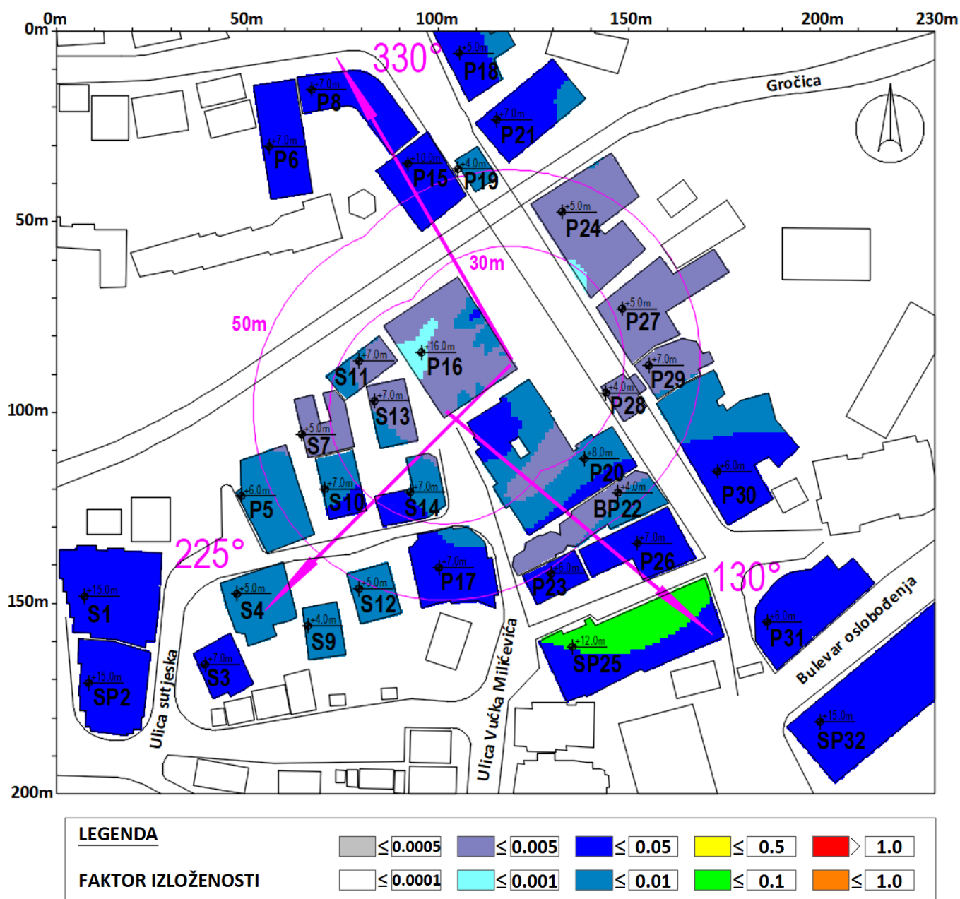
Slika 4.9 Rezultati proračuna ukupnog faktora izloženosti u objektima na najizloženijim spratovima za slučaj rada svih sistema operatora Telekom Srbija i Cetin(Yettel)
