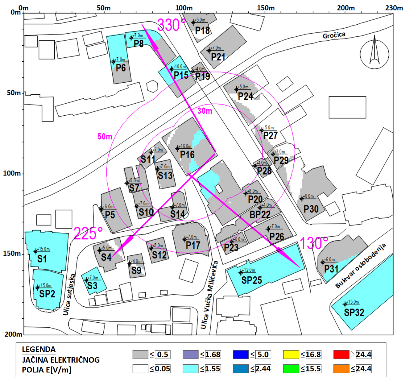
Slika 4.4 Rezultati proračuna jačine električnog polja u objektima na najizloženijim spratovima za slučaj rada sistema LTE2100 operatora Telekom Srbija
