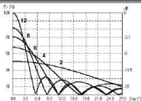
Diagrammi di ampiezza verticali di sistemi collineari in fase con 2, 4, 6, 8, 12 piani. Amplitude vertical diagrams of phased stacked-arrays with 2, 4, 6, 8, 12 bays.
