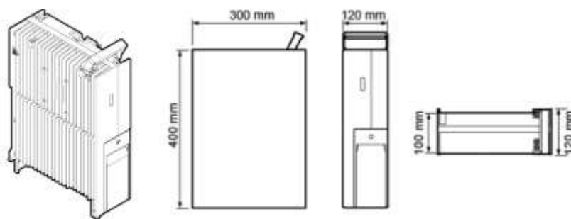
Slika 3.8 RRU jedinica
