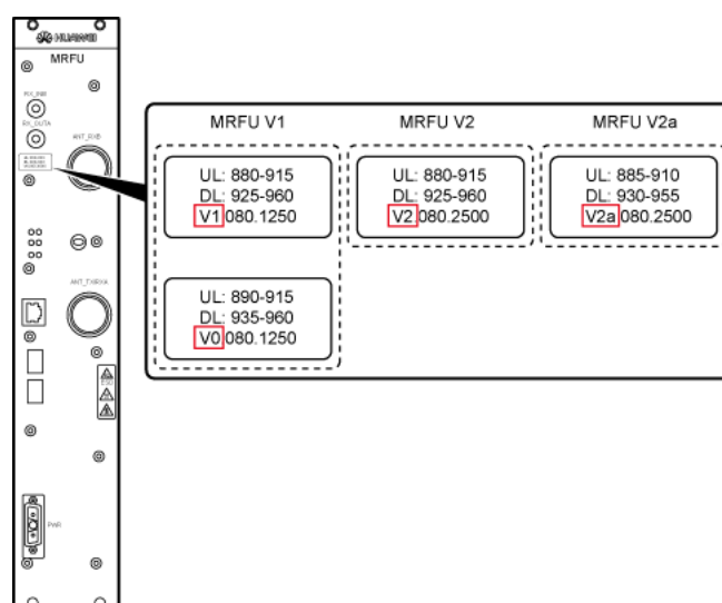
Slika 3.12 MRFU jedinica
