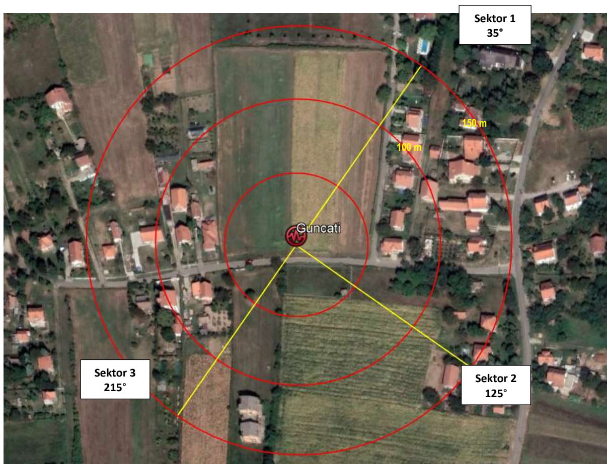
Slika 2.7 Pravci zračenja antenskih sistema GUNCATI
