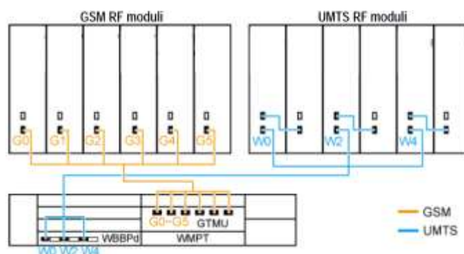
Slika 3.1 Povezivanje BBU3900 i RF modula
