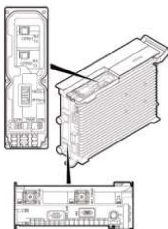
Slika 3.9 Portovi RRU jedinice 3268
