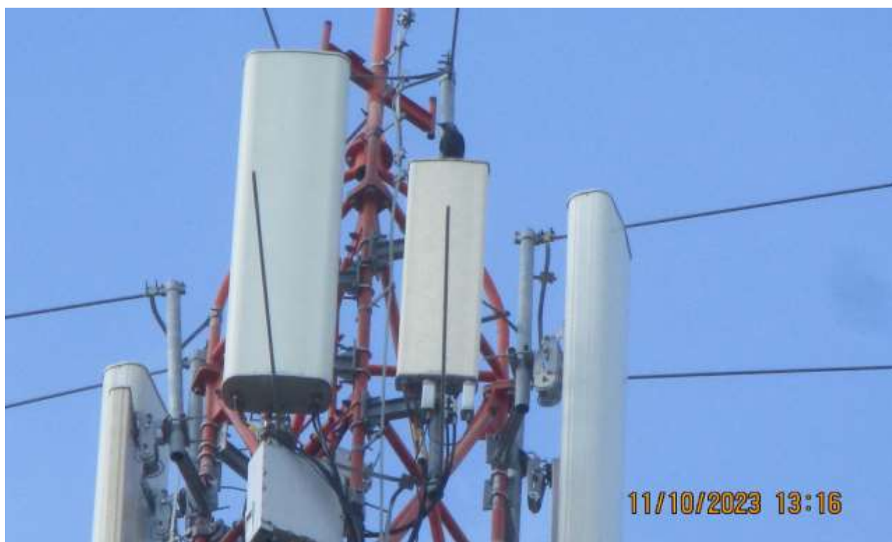
Slika 5 : Prikaz antena i radio modula sektora 2
