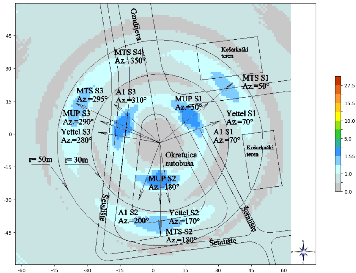
Slika 6.4. Rezultati proračuna jačine električnog polja na tlu sa uračunatom prosečnom visinom čoveka, za slučaj kada bazna stanica LTE800 Telekom Srbija radi sa maksimalnim kapacitetom.
