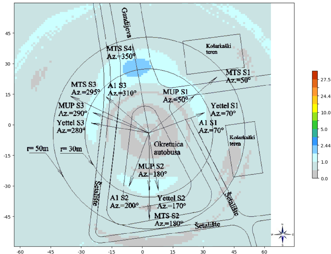
Slika 6.6. Rezultati proračuna jačine električnog polja na tlu sa uvažanom prosečnom visinom čoveka, za slučaj kada bazna stanica LTE2100 Telekom Srbija radi sa maksimalnim kapacitetom.
