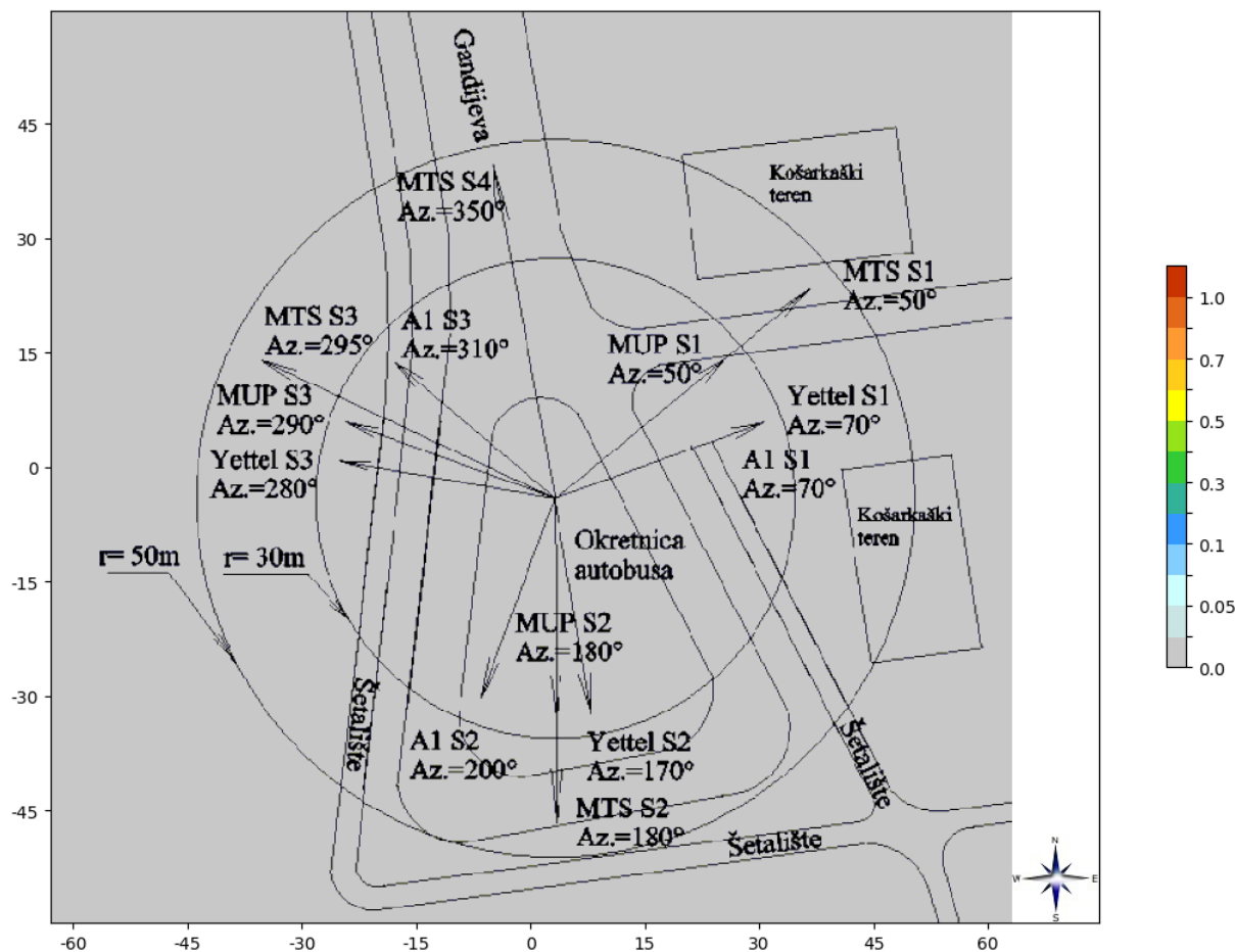
Slika 6.7. Rezultati proračuna faktora izlaganja na tlu sa uračunatom prosečnom visinom čoveka, za slučaj kada svi sistemi Telekom Srbija na lokaciji rade sa maksimalnim kapacitetom.
