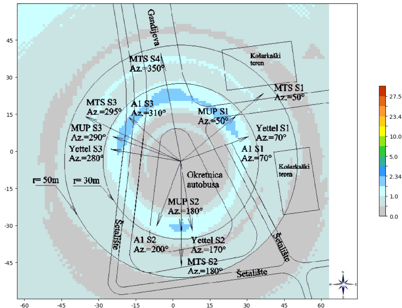
Slika 6.3. Rezultati proračuna jačine električnog polja na tlu sa uvažanom prosečnom visinom čoveka, za slučaj kada bazna stanica LTE1800 Telekom Srbija radi sa maksimalnim kapacitetom.
