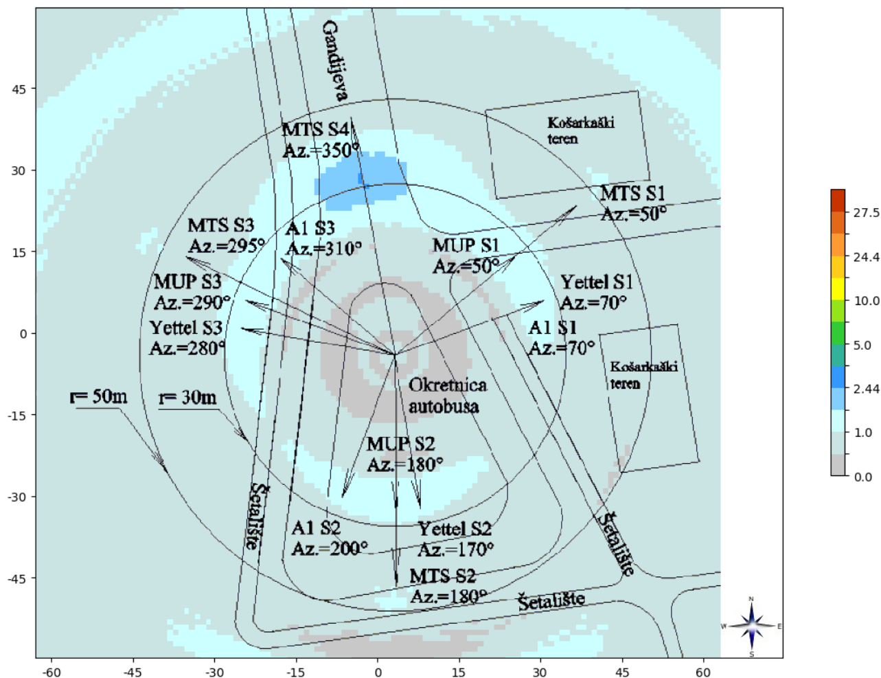
Slika 6.5. Rezultati proračuna jačine električnog polja na tlu sa uvažavanom prosečnom visinom čoveka, za slučaj kada bazna stanica UMTS2100 Telekom Srbija radi sa maksimalnim kapacitetom.
