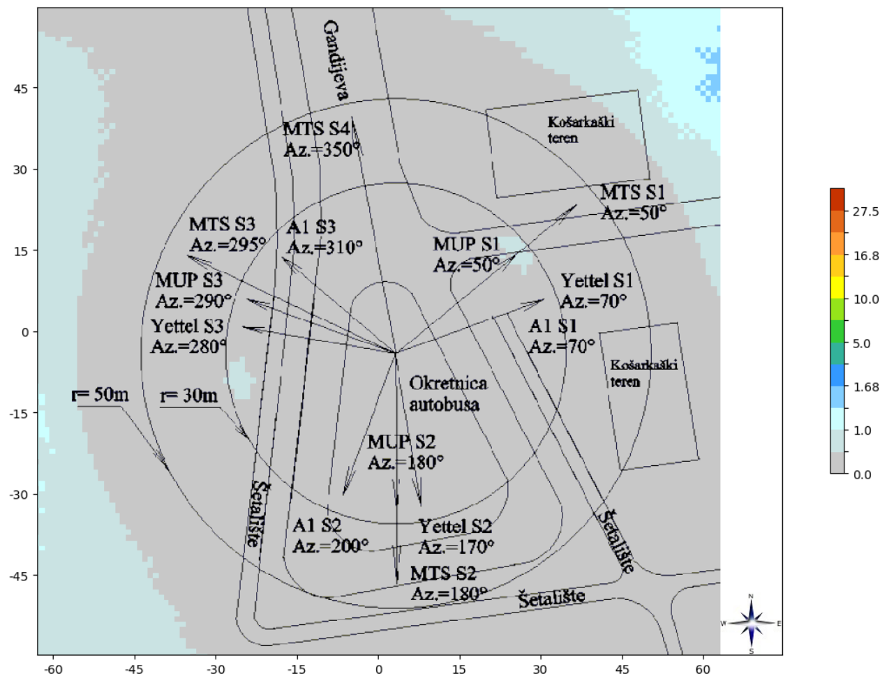
Slika 6.2. Rezultati proračuna jačine električnog polja na tlu sa uvažavanom prosečnom visinom čoveka, za slučaj kada bazna stanica GSM900 Telekom Srbija radi sa maksimalnim kapacitetom.
