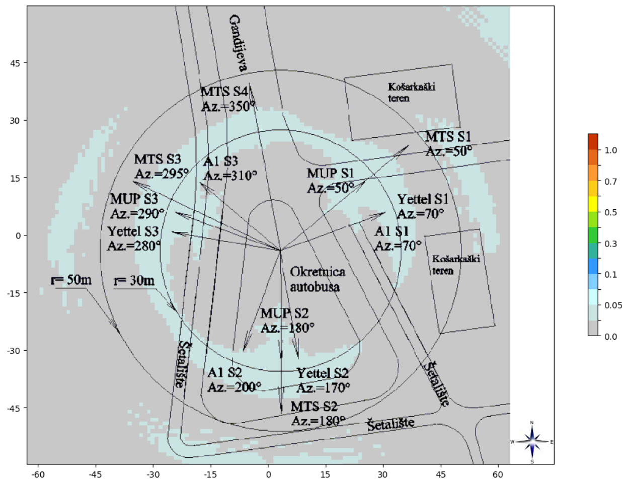
Slika 6.8. Rezultati proračuna faktora izlaganja na tlu sa uračunatom prosečnom visinom čoveka, za slučaj kada svi sistemi svih operatora na lokaciji rade sa maksimalnim kapacitetom.
