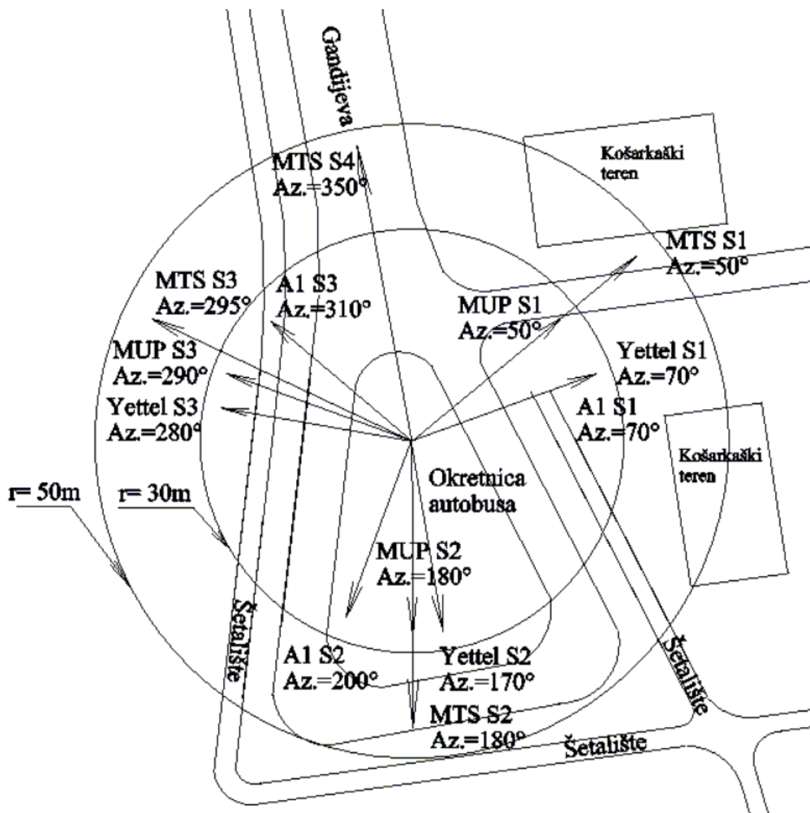
Slika 2.1.1. Dijagram objekata u okruženju predmetne bazne stanice u krugu poluprečnika 50m
