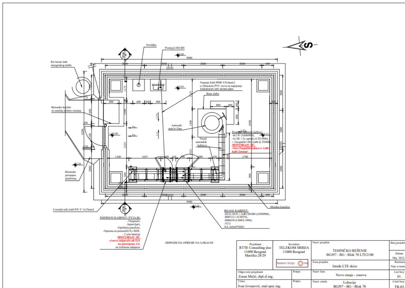
Slika 3.2.1. Izgled novoprojektovanog stanja - osnova
